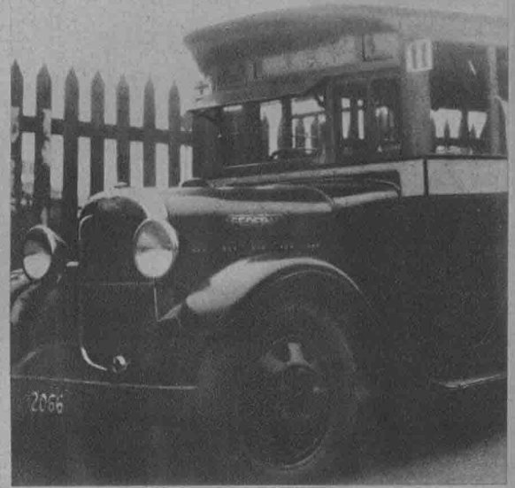
廣州製之木炭瓦斯汽車試驗情形
