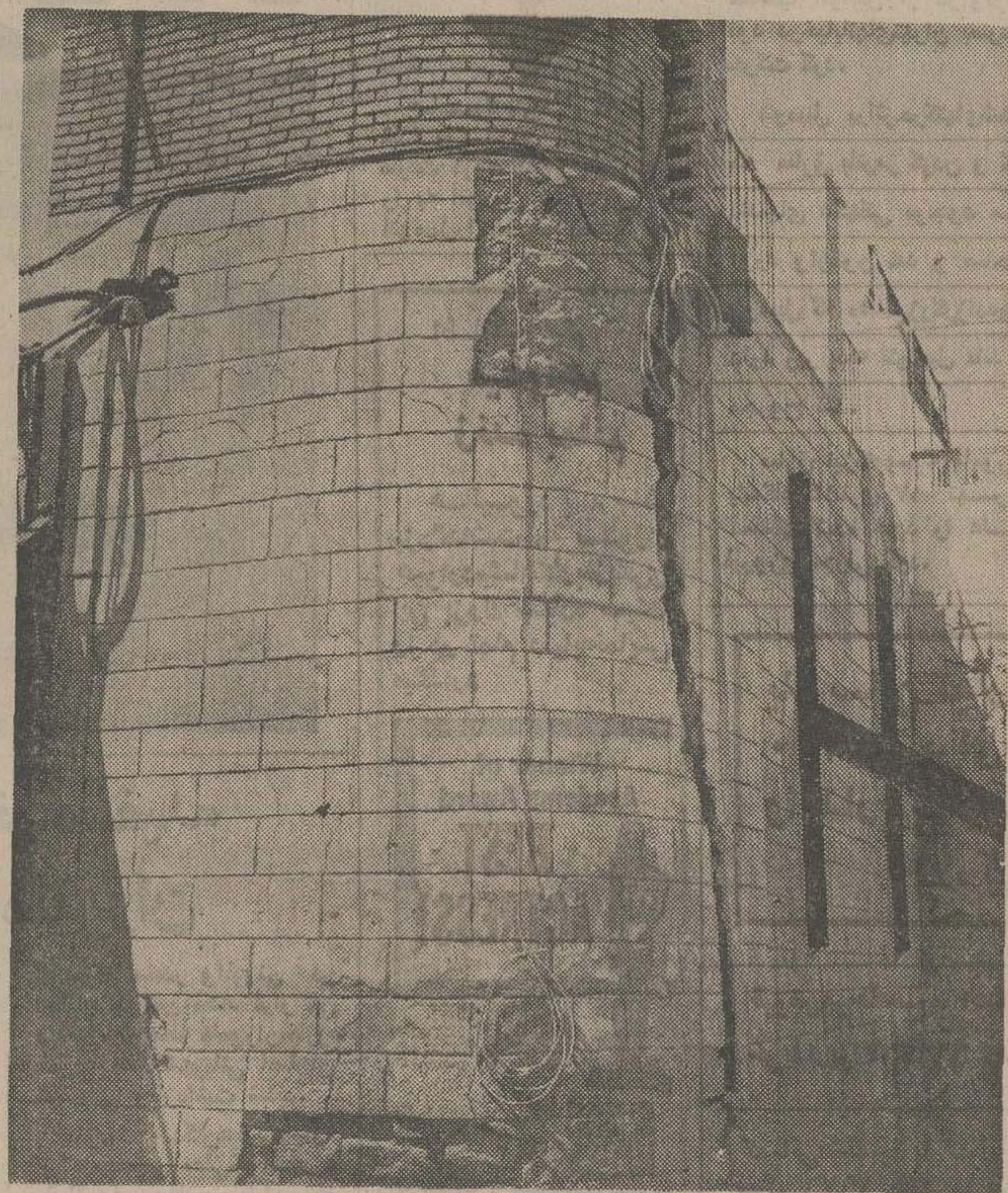
پایه بل معلق (سفید) اهواز که بطرز عجیبی شکاف برداشته در این عکس مشخص است . عکس از : غلامرضا یزدانی خبرنگار عکاس اطلاعات در اهواز
