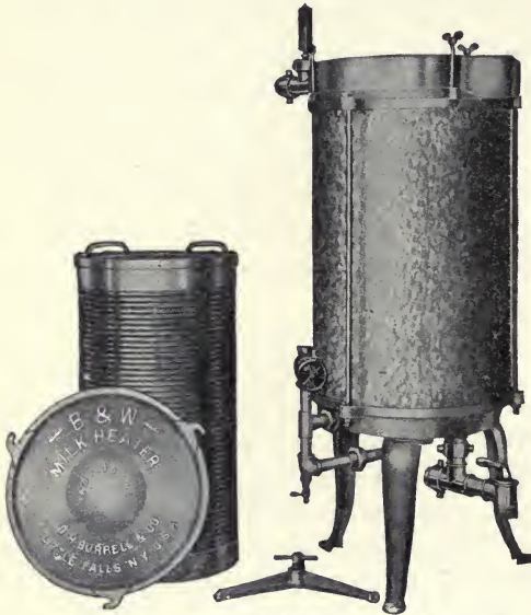
Fig. 24. Simplex regeneration pasteurizer Courtesy D. H. Burrell & Co.
