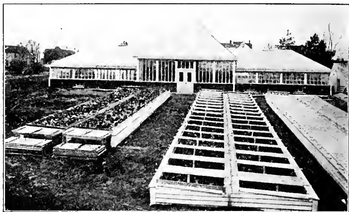
FIG. 24. PERMANENT COLD FRAMES
