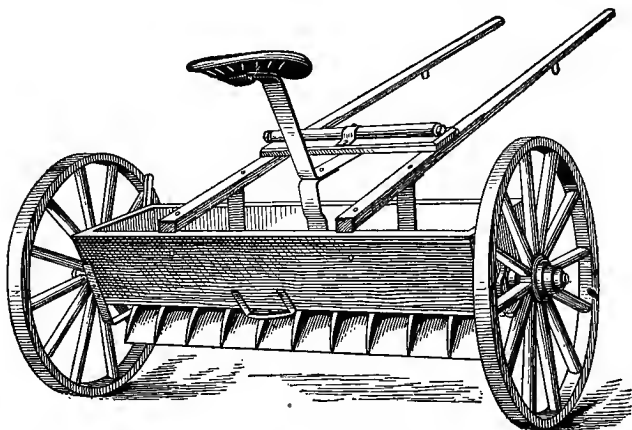
FIG. 14. LIME SPREADER
