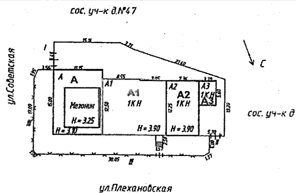
План-схема участка с объектом
