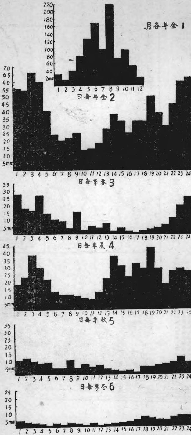
(五) 遼義雨量變化柱狀圖
