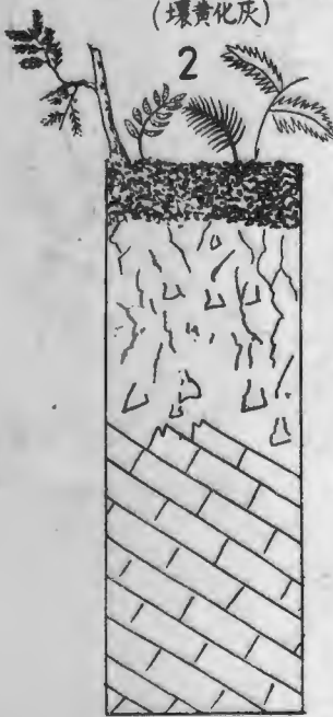
面剖土壤粘砂粉山東 (上灰石色黑)
