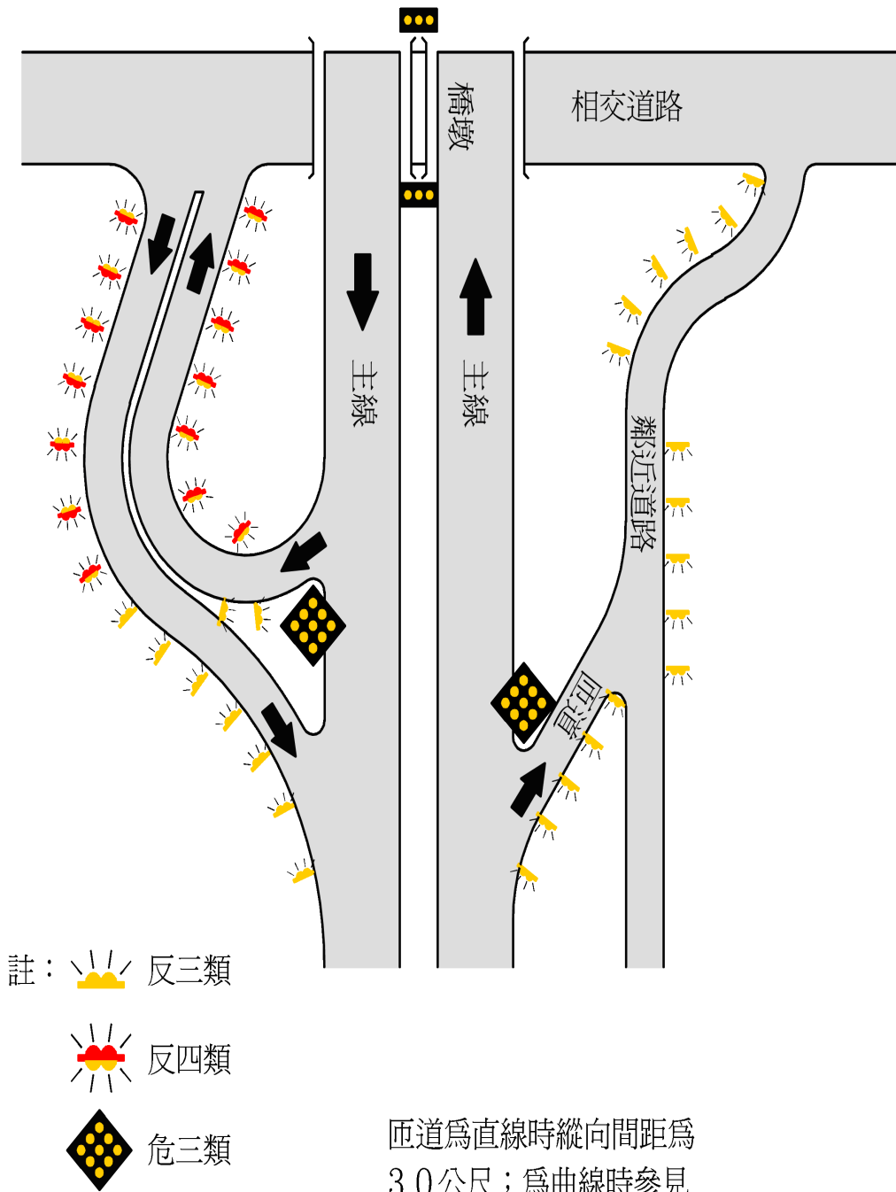
圖四 高(快)速公路匝道上反光導標及危險標記之設置
