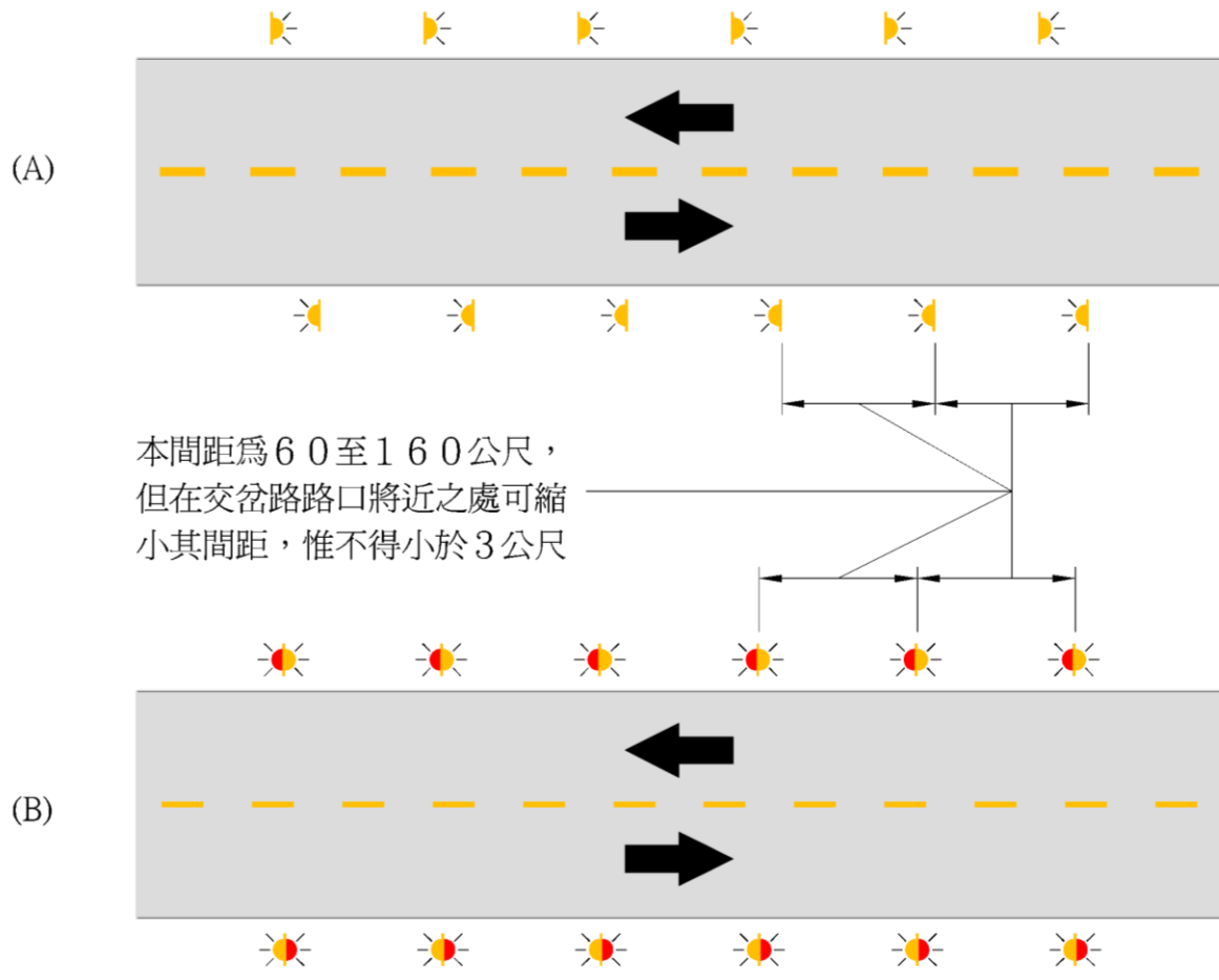
圖一 公路直線上反光導標之位置
