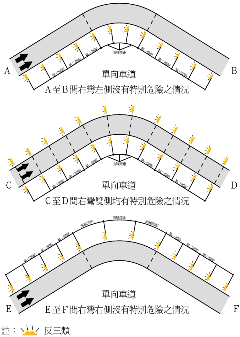
圖二 單向車道曲線上反光導標之設置
