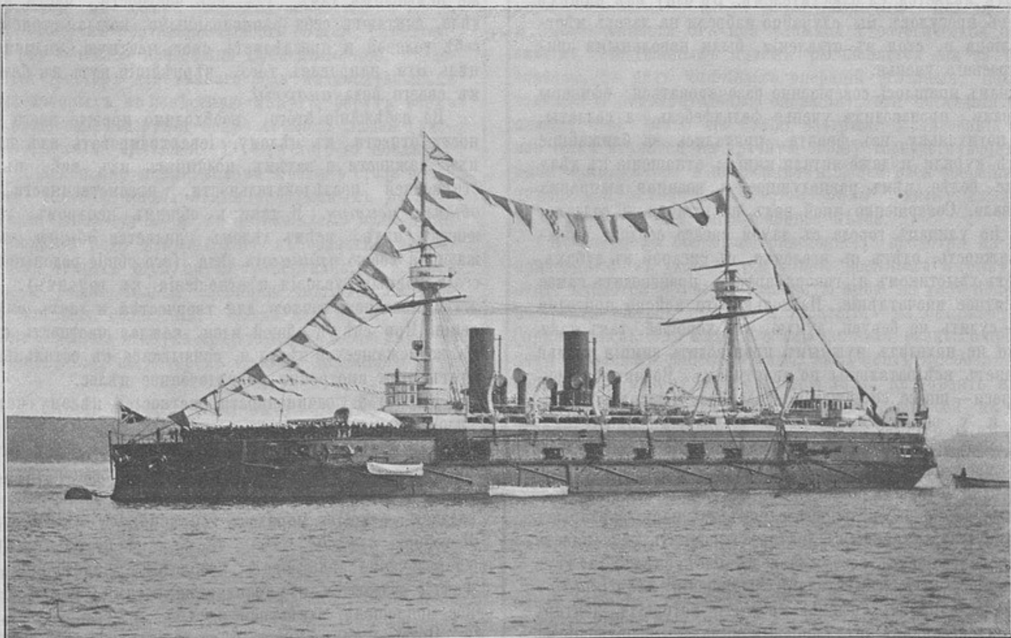
Эскадренный броненосецъ «Императоръ Александръ II.» Построенъ въ 1887 г. Длина 326 ф.; ширина 67 ф.; углубленіе 23 ф. водоизмѣщеніе 84400 тоннъ.; машина 8000 индикаторныхъ силъ. Ходъ 15 узловъ. Орудія: 2—12 дюйм. 4—9 дюйм. 8—6 дюйм. 24 скорострѣльныхъ, 4 минныхъ аппарата.
