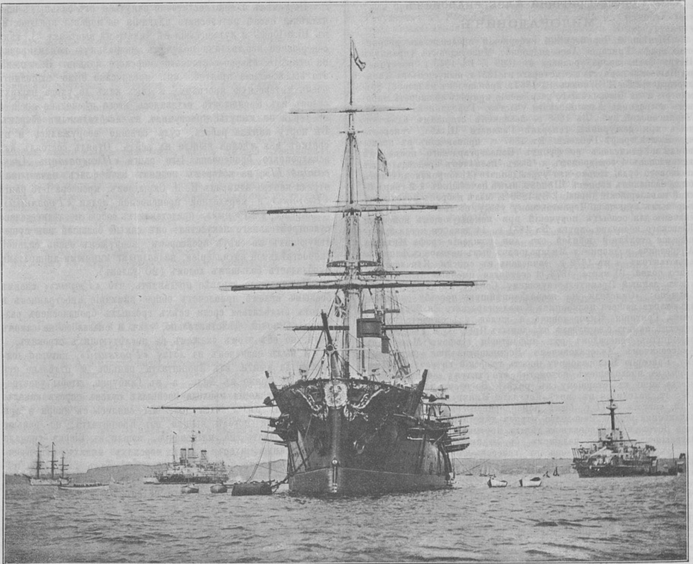
Крейсеръ 1-го ранга «Рюрикъ». Построенъ въ 1892 г. Длина 426 ф.; ширина 67 ф. углубленіе 26 ф. водоизмѣщеніе 11000 тоннъ. Машины 13,250 индикаторныхъ силъ. Ходъ 20 узловъ. Орудія: 4—8"; 16—6" скорострѣльныхъ системы Кана; 6—5" тоже скорострѣльныхъ; 20 скорострѣльныхъ пушекъ малаго калибра; 6 минныхъ аппаратовъ.
