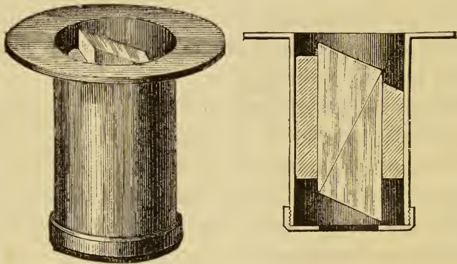
Fig. 32. — Polarizador. La figura de la derecha representa un corte vertical del aparato y muestra el prisma de nicol ; la figura de la izquierda representa el nicol en su montura.
