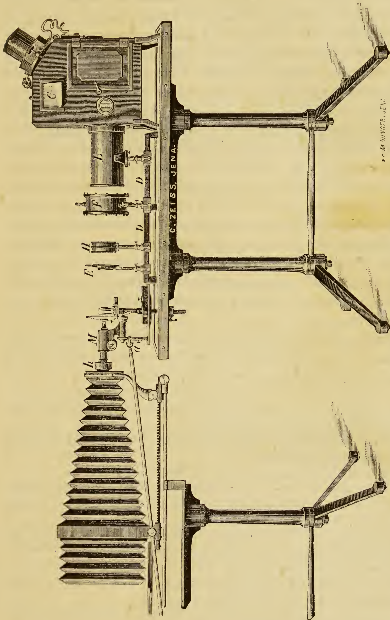
Fig. 30. — Gran aparato microfotográfico de Zeiss, dispuesto para la iluminación con luz eléctrica ó la luz del magnesio.
