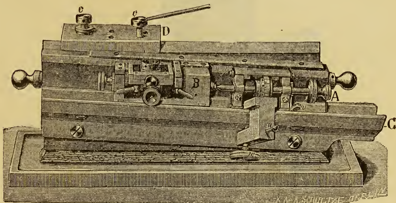
Fig. 38. — Microtomo por deslizamiento. Modelo Thoma Jung: A, tornillo micrométrico; B, bloque portador del porta-piezas; C, plano inclinado; D, pieza sobre la que se fija la navaja.
