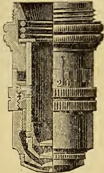
Fig. 17.—Corte vertical de un objetivo apocromático y de corrección.
