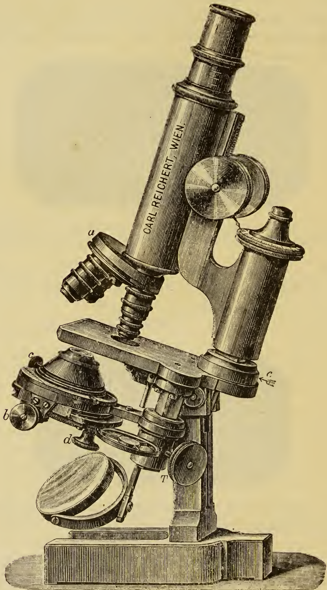
Fig. 21. — Microscopio modelo II, b , de Reichert, provisto del iluminador Abbe y del revólver porta-objetivo.
