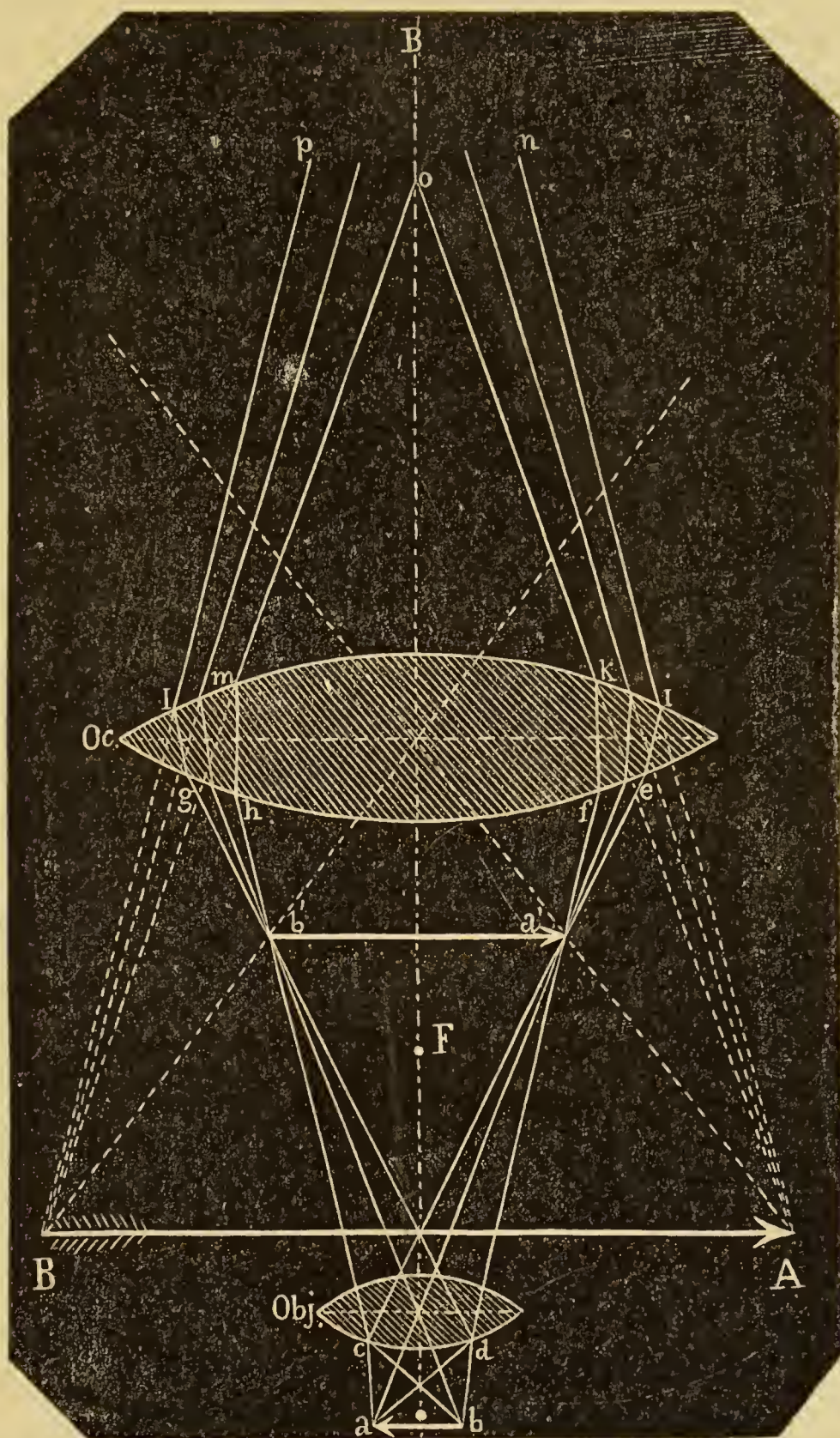
Fig. 6. — Marcha de los rayos y formación de las imágenes en el microscopio compuesto: Obj. , objetivo; Oc. , ocular; a b , objeto microscópico; b' a' , imagen real proyectada por el objetivo; A B , imagen virtual engendrada por el ocular.
