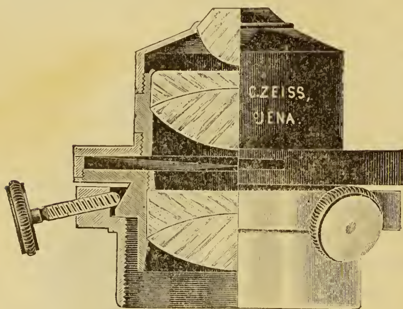
Fig. 14. — Corte del concentrador Abbe acromático.
