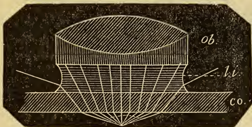
Fig. 20. — Marcha de los rayos emanados de la preparación en un objetivo de inmersión homogénea: ob. , objetivo; co. , cubre-objeto; li. , líquido de inmersión. (Tomadas de Ellenberger).
