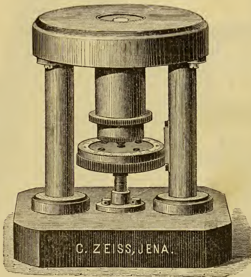
Fig. 35. — Microtomo de Ranvier perfeccionado por Zeiss.
