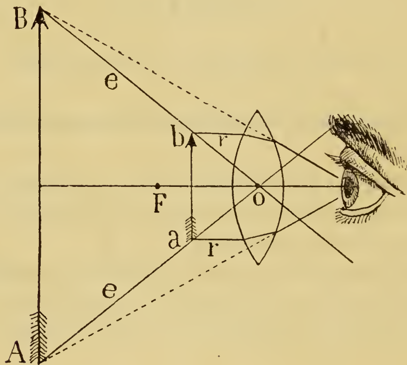
Fig. 1. — Formación de las imágenes en el microscopio simple.
