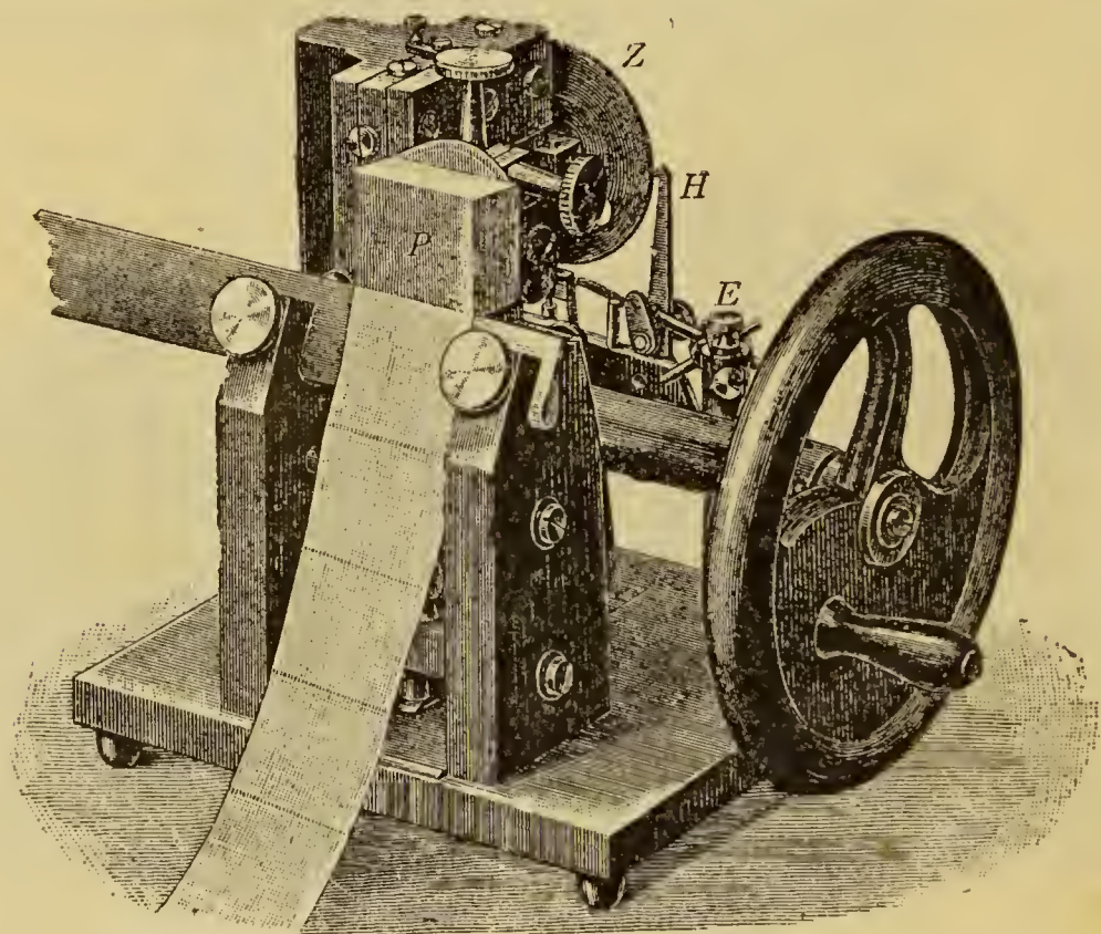
Fig. 39. — Microtomo automático de Minot para practicar secciones en parafina: P, parafina; Z, rueda dentada unida al tornillo micrométrico.
