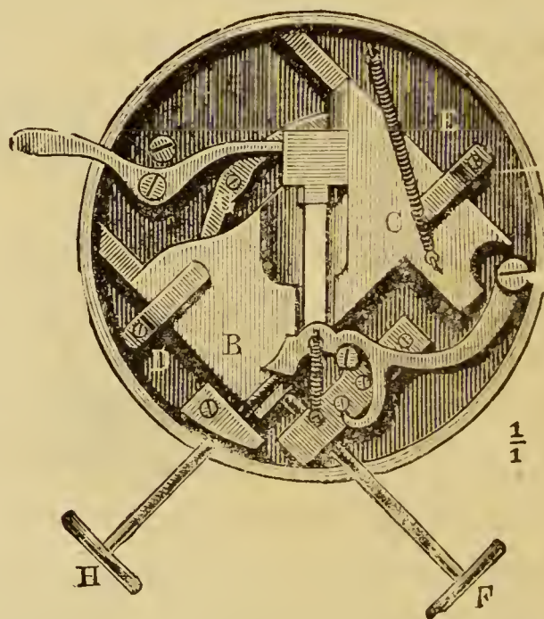
Fig. 34. — Detalles del aparato destinado á estrechar la hendidura del microespectroscopio.
