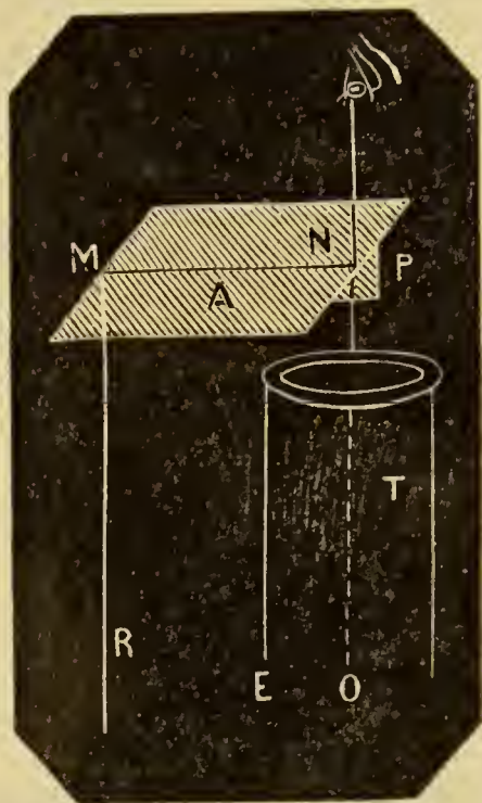
Fig. 24. — Esquema de la cámara de Nachet: T, tubo del microscopio; A, el paralelepípedo de cristal; R, rayo que llega del papel; O, rayo emanado del microscopio.
