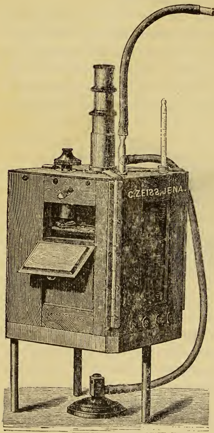
Fig. 41. — Cámara caliente de Pfeiffer.
