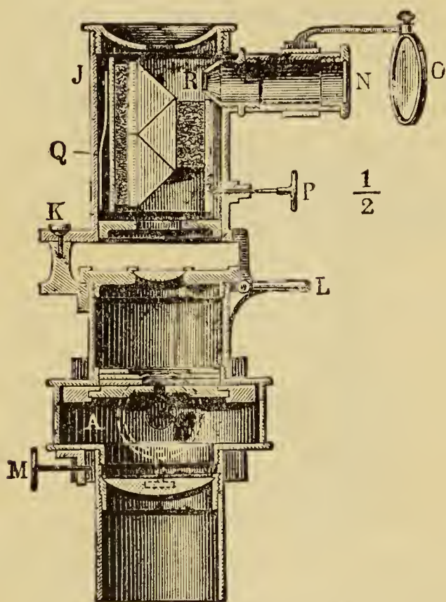
Fig. 33. — Microespectroscopio de Sorby construido por Zeiss.
