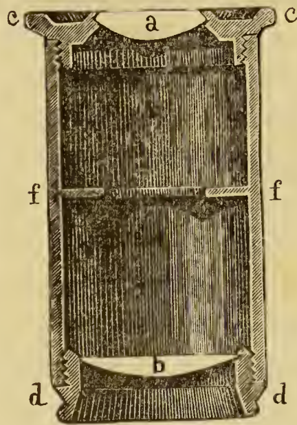
Fig. 22. — Corte vertical del ocular: a , ocular propiamente dicho; b , lente del campo; f , diafragma.
