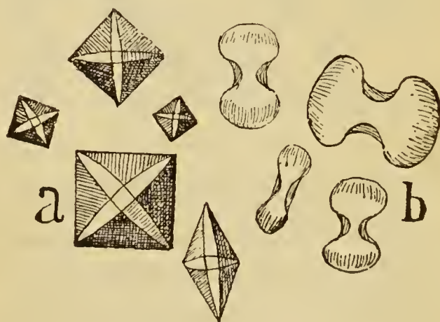
Fig. 44. — Cristales de oxalato de cal. — a , cristales octaédricos; b , cristales en forma de reloj de arena.
