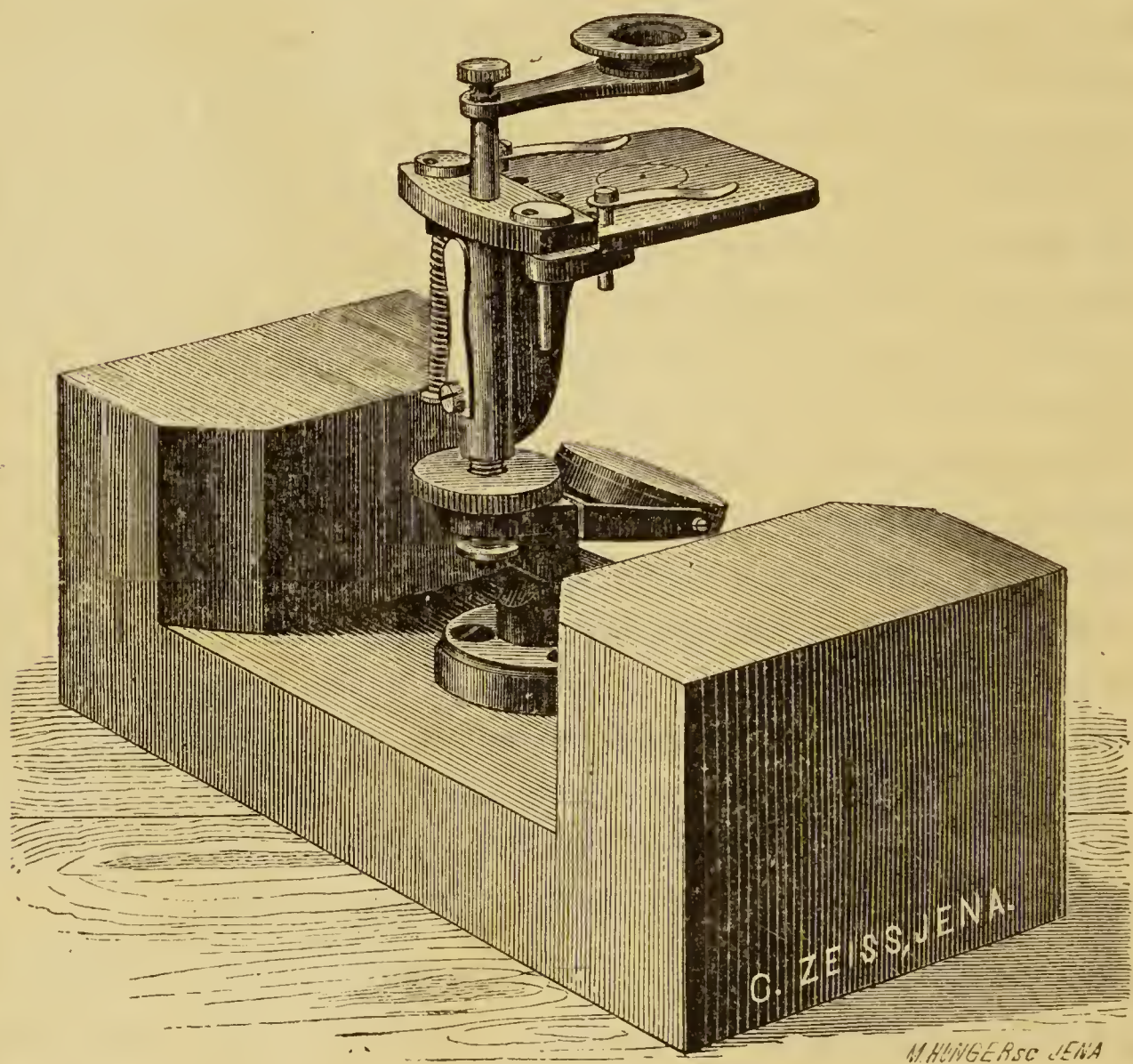
Fig. 2. — Modelo de microscopio simple según Zeiss. El descenso de la lente se opera por tornillo micrométrico.
