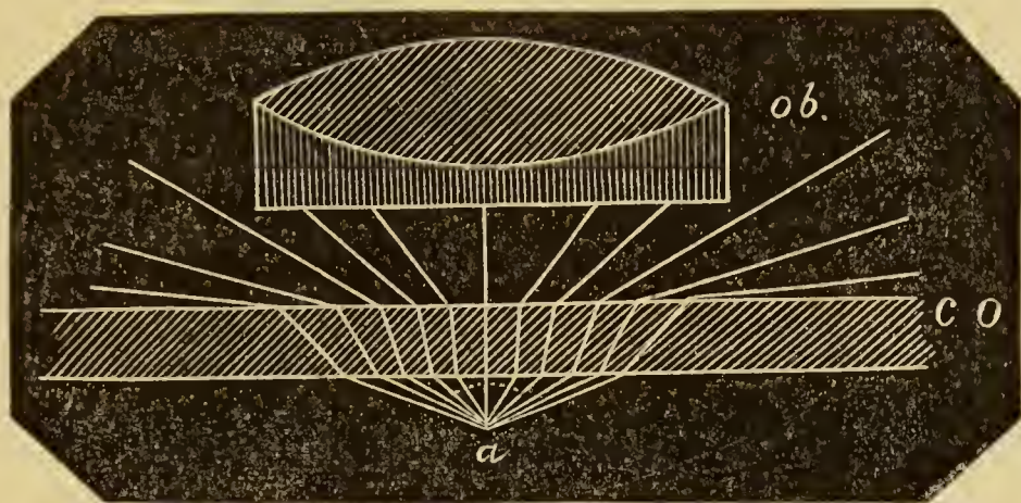
Fig. 19. — Marcha de los rayos luminosos emanados de un punto en los objetivos á seco: ob. , lente frontal del objetivo; co. , cubre-objeto.
