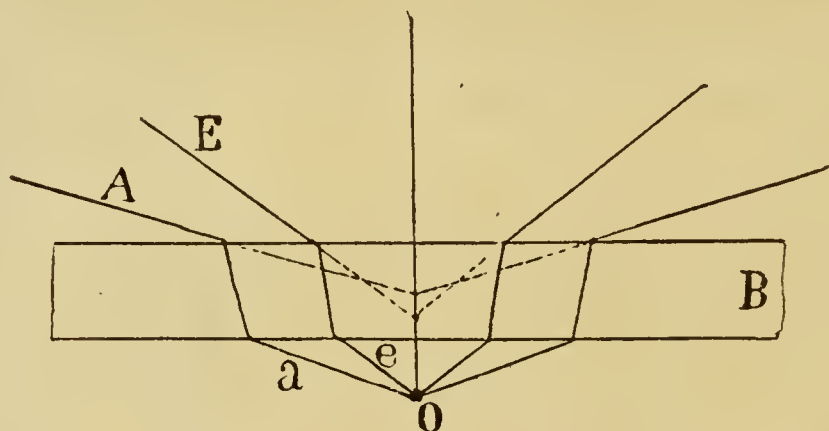
Fig. 18. — Influencia del espesor de la lámina cubre-objetos (B) en la marcha de los rayos luminosos emanados de un punto O de la preparación.
