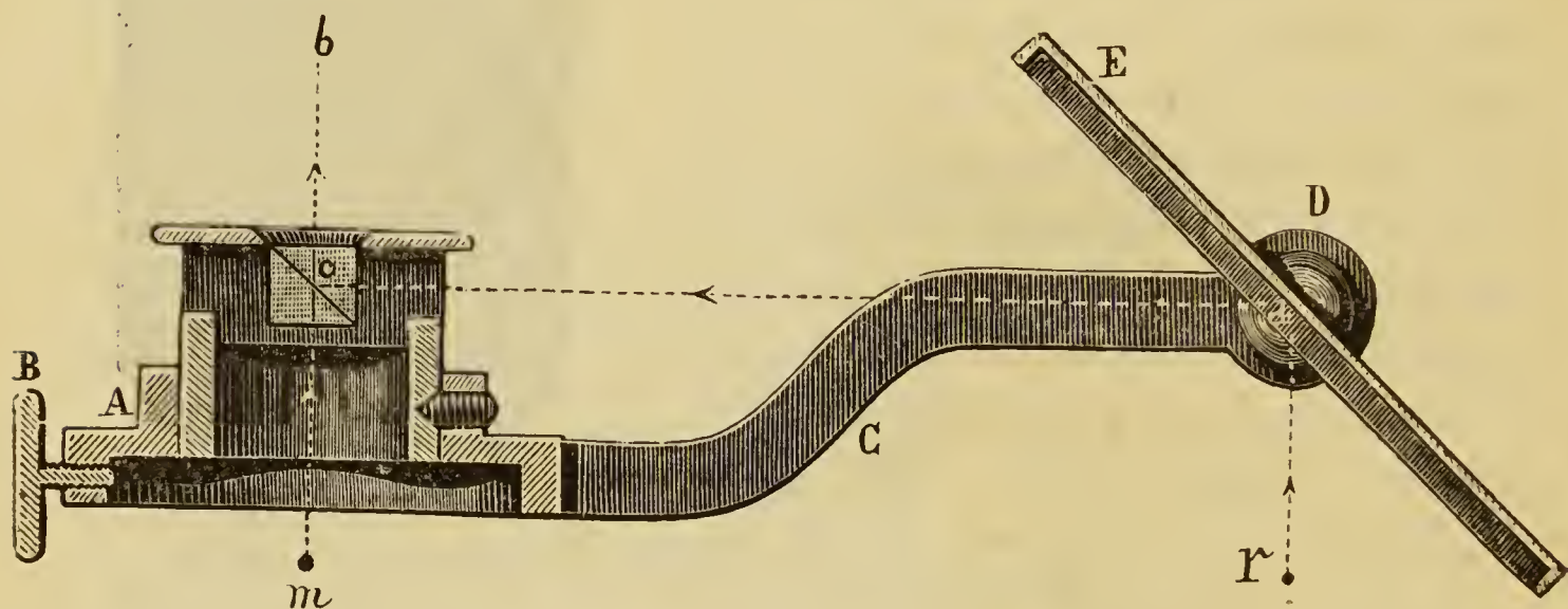
Fig. 25. — Marcha de los rayos luminosos en la cámara clara de Abbe : r , rayo emanado del papel ; m , rayo llegado del microscopio ; E, espejo ; c , cubo de cristal.
