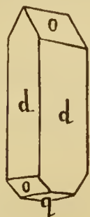
Fig. 46.—Forma ideal de los cristales de urea (Kössel).
