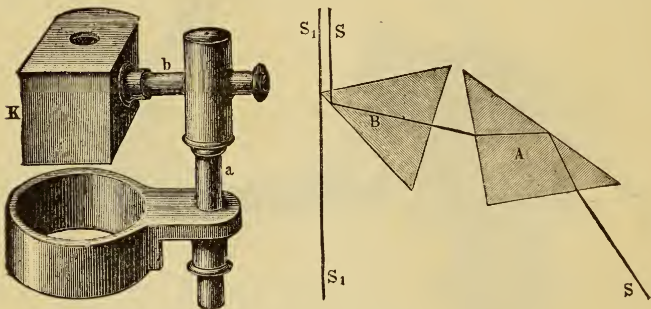
Fig. 27. — Cámara clara de Zeiss: á la izquierda se ve el aparato completo; á la derecha, su esquema: S, rayo dimanado del papel; S 1 , rayo llegado del microscopio.
