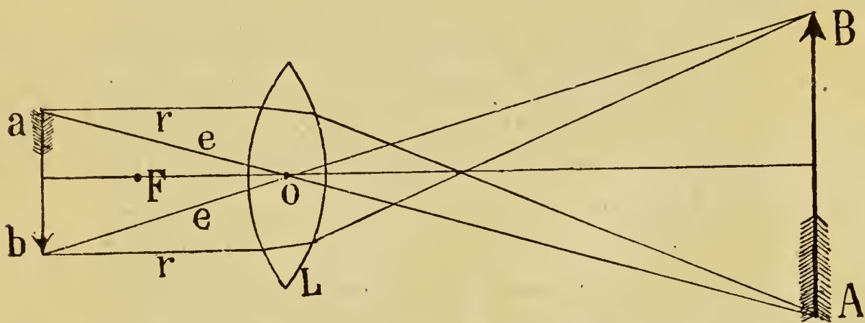
Fig. 5. — Marcha de los rayos luminosos en el objetivo: A, B, imagen; F, foco; e, e , ejes secundarios.
