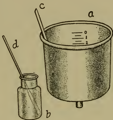
FIG. 47 MARSCHALL RENNET-TEST
