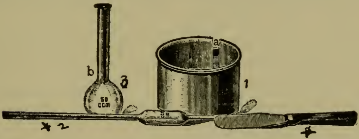
FIG. 46—MONRAD RENNET-TEST
