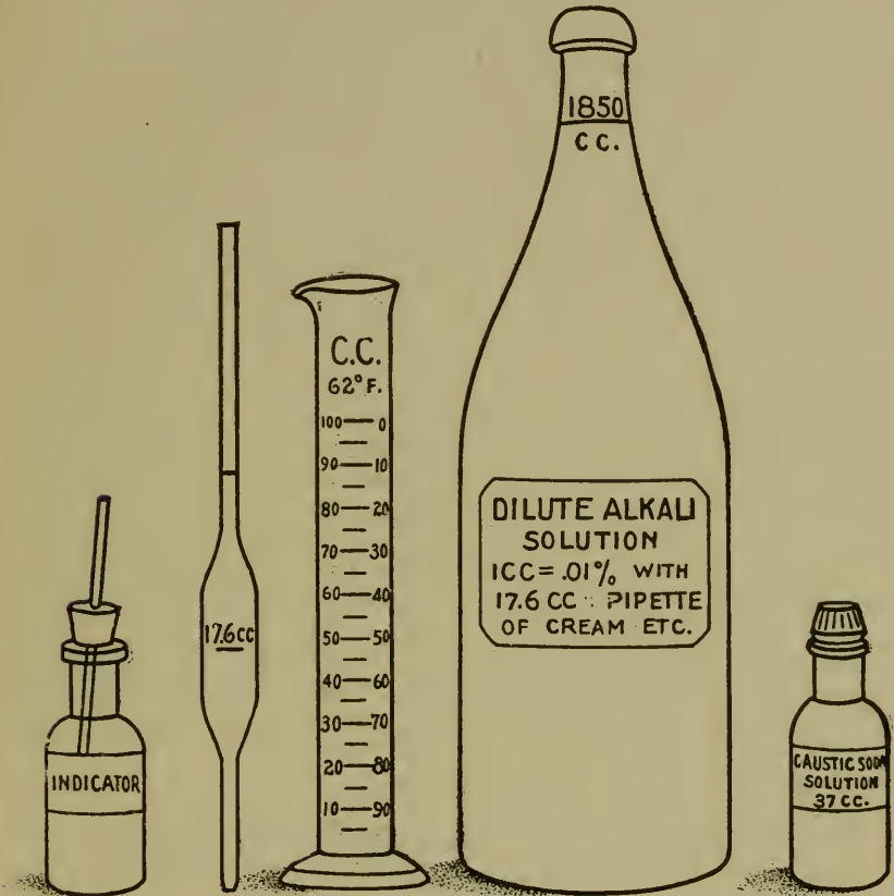
FIG. 40—PURDUE ALKALI TEST
