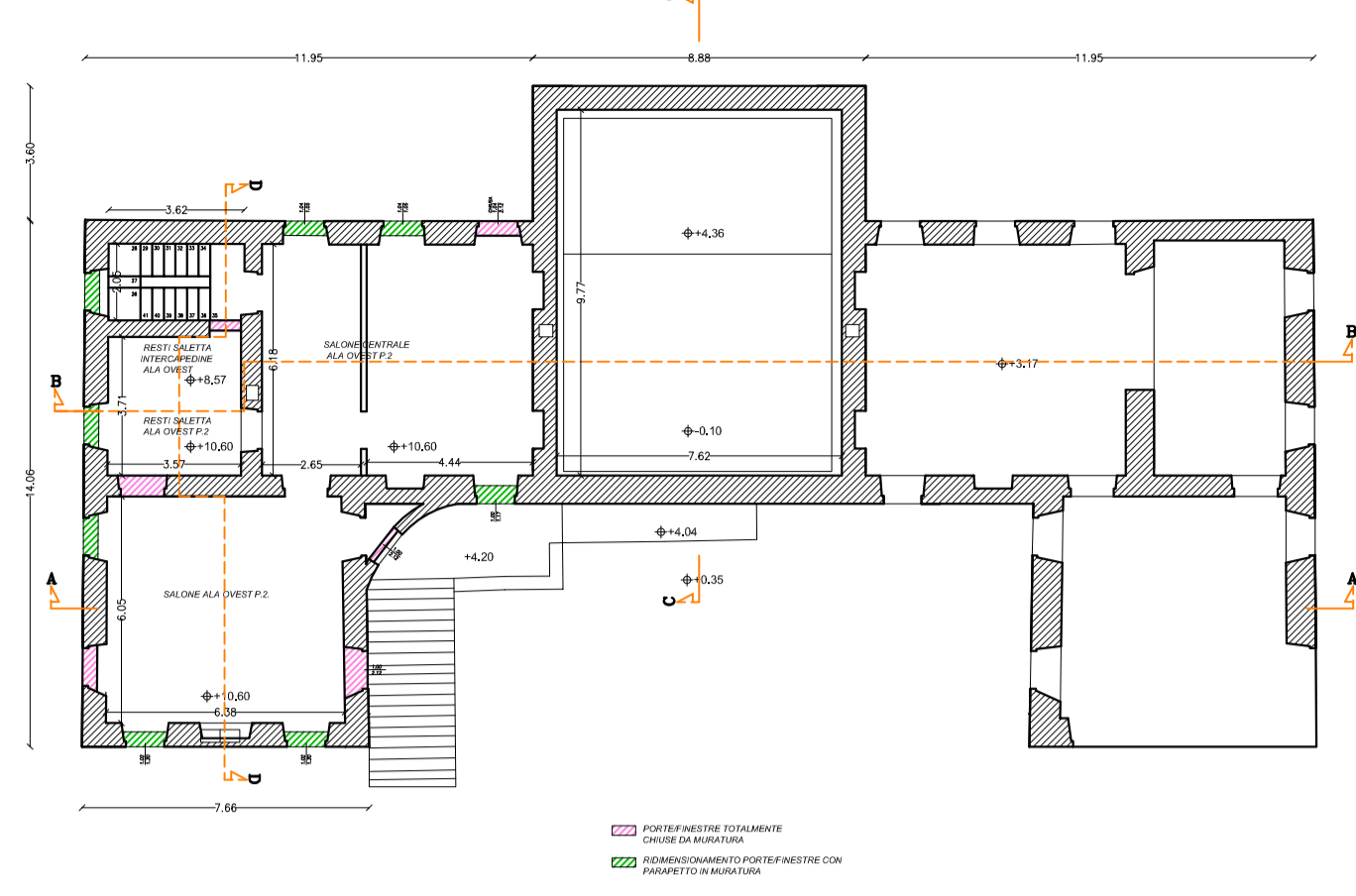
PIANO SECONDO
