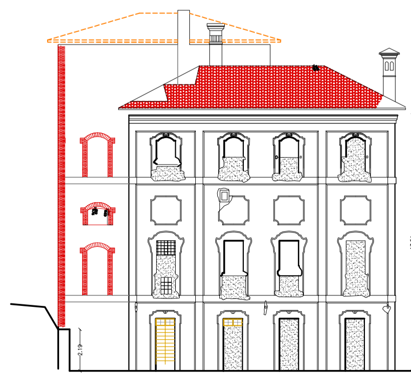
PROSPETTO OVEST
