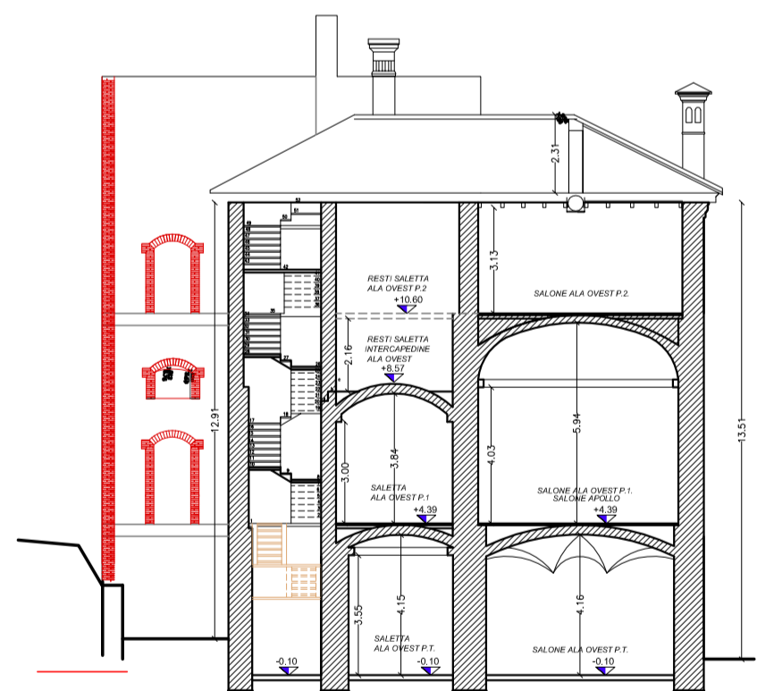
SEZIONE D-D
