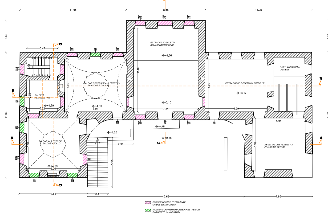
PIANO PRIMO
