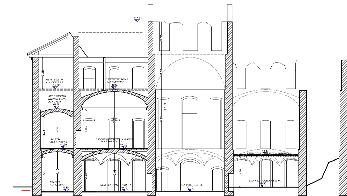
SEZIONE B-B
