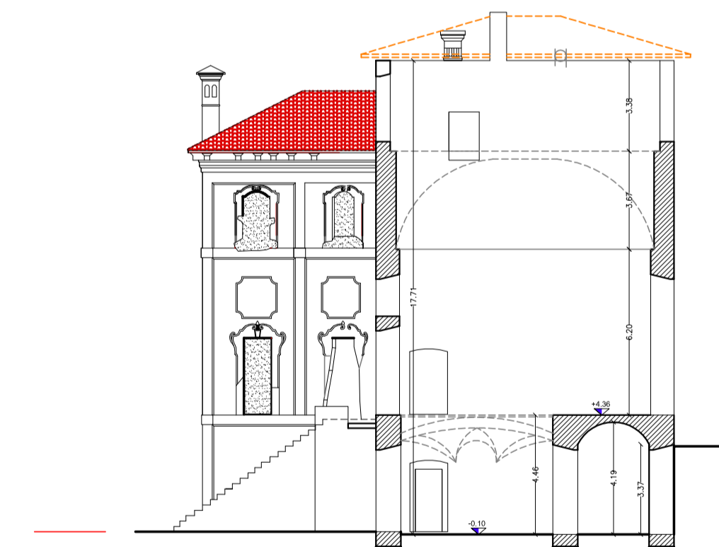
SEZIONE C-C
