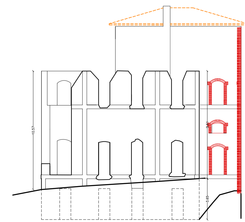
PROSPETTO EST
