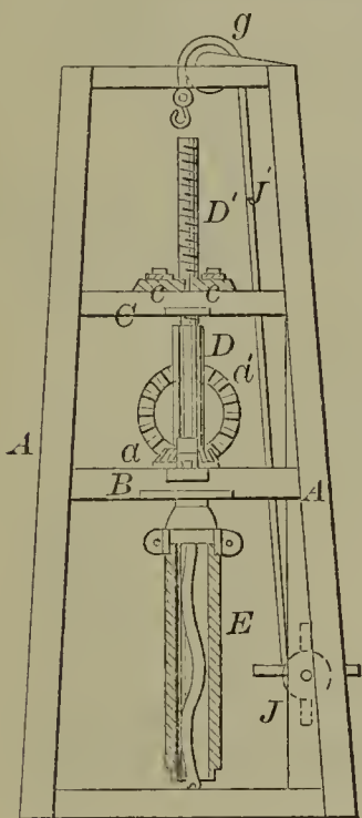
52102—G. L. Witsill—Well Boring.
