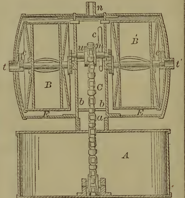
56116—L. Stevens— Treating Gas.
