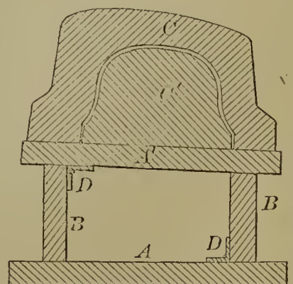
54601—H. A. Robison— Hat Block.
