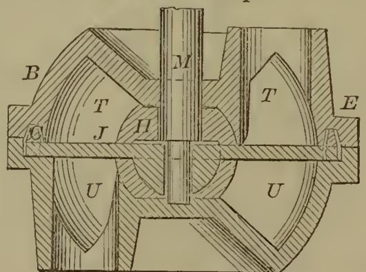
55318—H. Maas— Pump.
