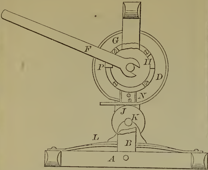
55226—W. O. Bartlett— Bridle.
