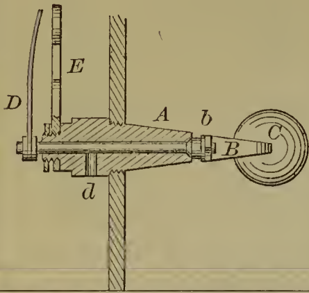
53351—F. Schweizer—Bolt Heading Machine.
