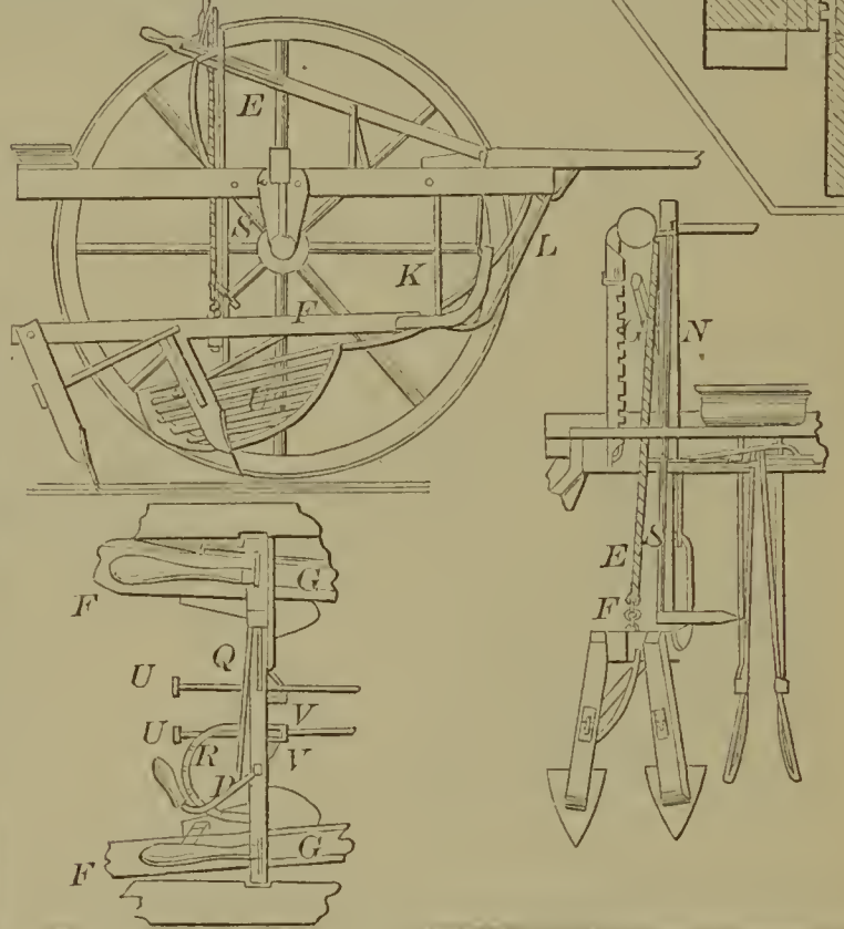
59231—W. Kiddoo—Cultivator.
