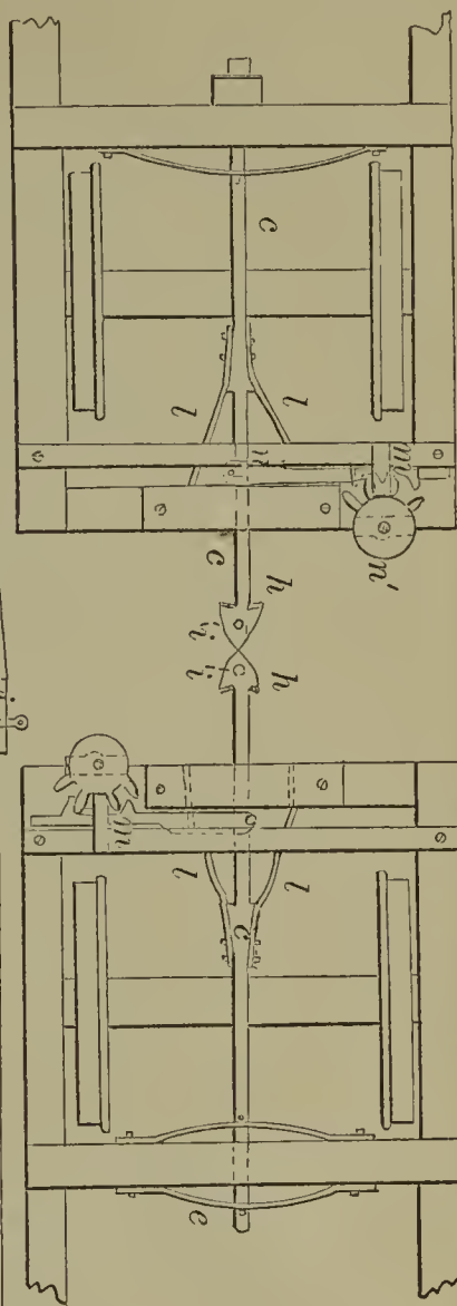
60093—J. D. Van Hoevenbergh—Carriage.
