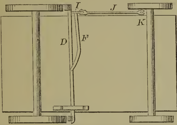
57625—G. W. Crowe—Brake.
