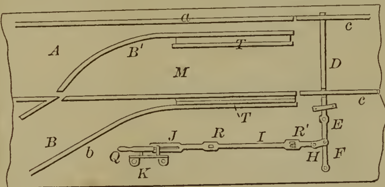
56432—T. S. Mitchell— Railroad Switch.
