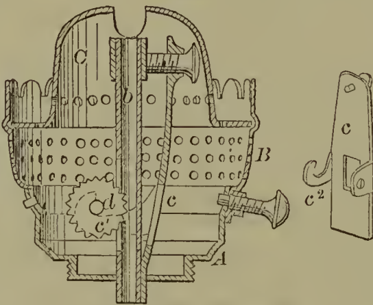
60263—J. F. Sanford—Lamp Burner.
