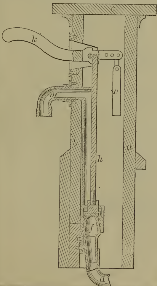
55893—J. Old—Hydrant.
