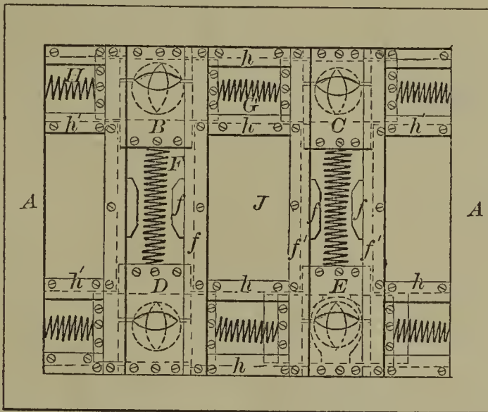
58049—W. N. Barr— Cane Stripper.
