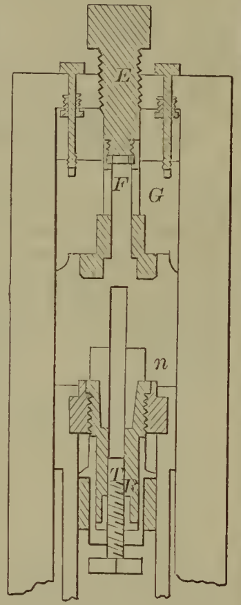
55597—H. E. Anthony— Bolt Heading Machine.
