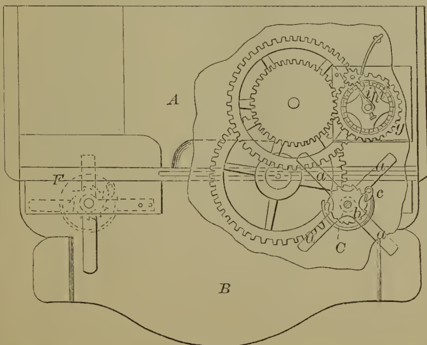
59387—J. & C. Gschwind—Car Register.
