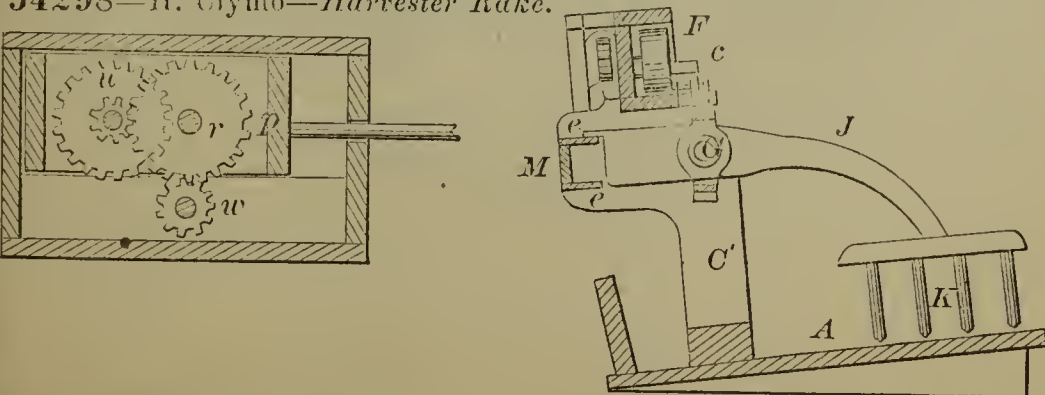
54298—H. Clymo— Harvester Rake.
