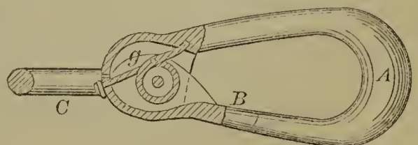
56951—O. S. Judd—Snap Hook.
