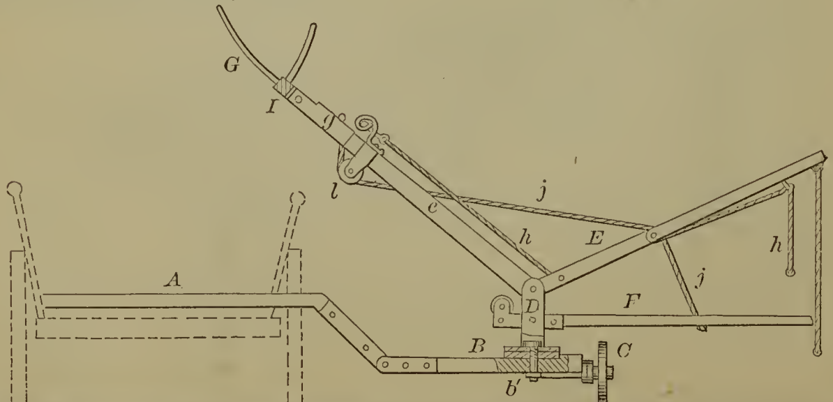
54627—F. Van Etten—Hay Loader.
