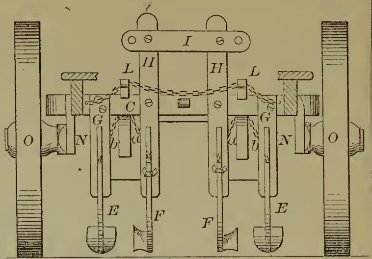
53403—W. R. Brooks—Wick Trimmer.
