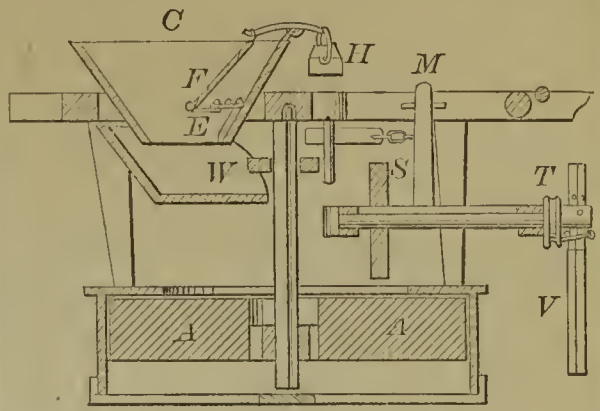
59435—S. M. Miller— Grinding Mill.
