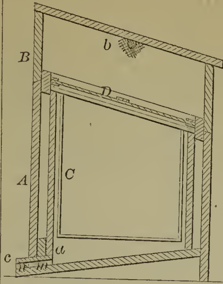
56782—M. D. Mulford, Jr.— Beehive.
