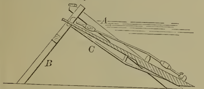
56962—J. Malby—Flood Gate.
