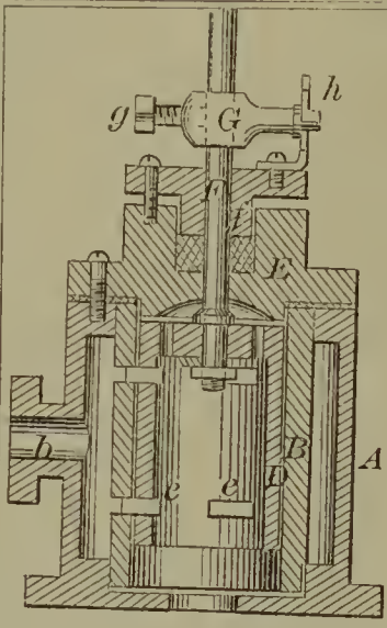
60378—G. G. Hunt— Steam Valve.
