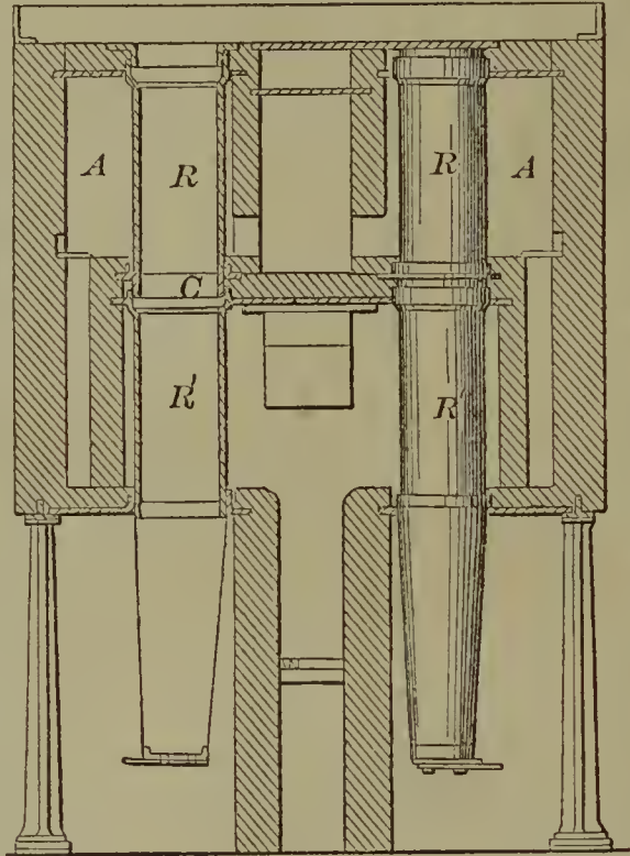
60492—E. P. Eastwick—Bone Black Kiln.
