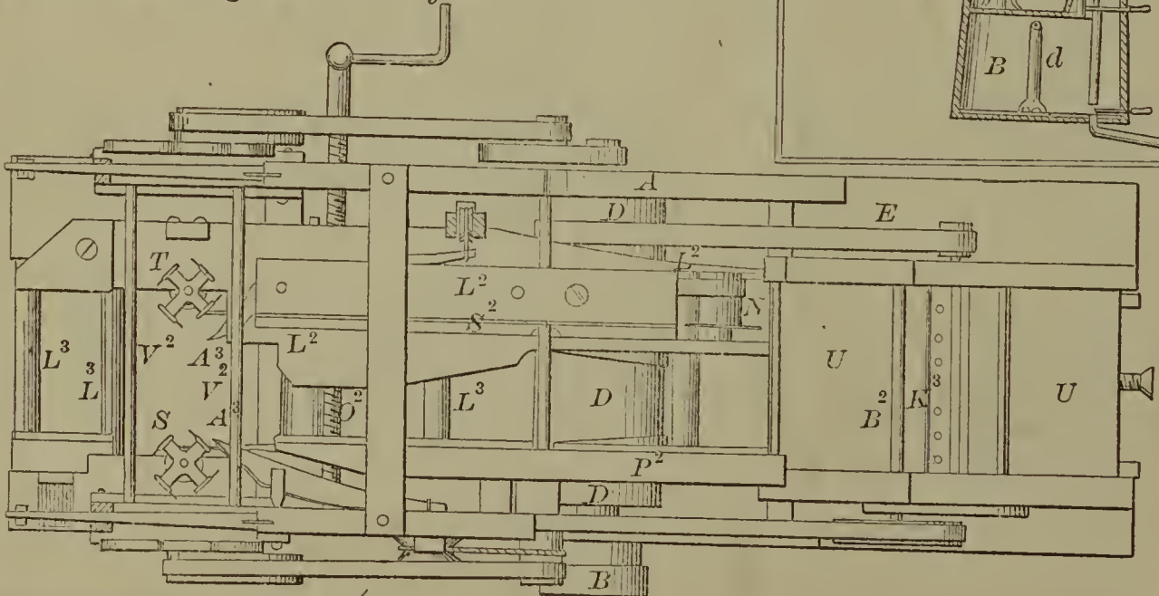
60332—O. Bridgeman—Planing Machine.
