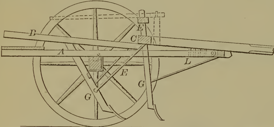
57700—G. T. Gifford— Cultivator.
