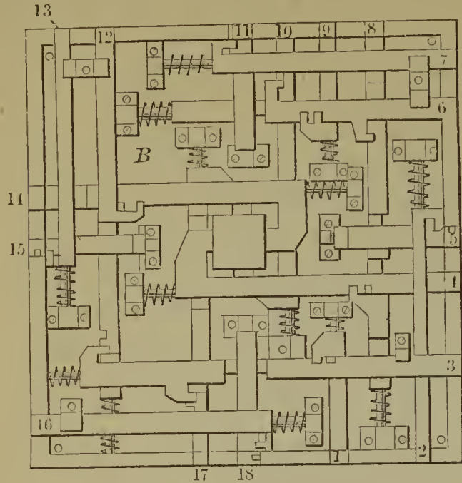
56790—A. A. Oat—Safe Lock.
