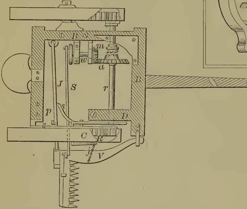
54946—J. G. Perry—Harvester.
