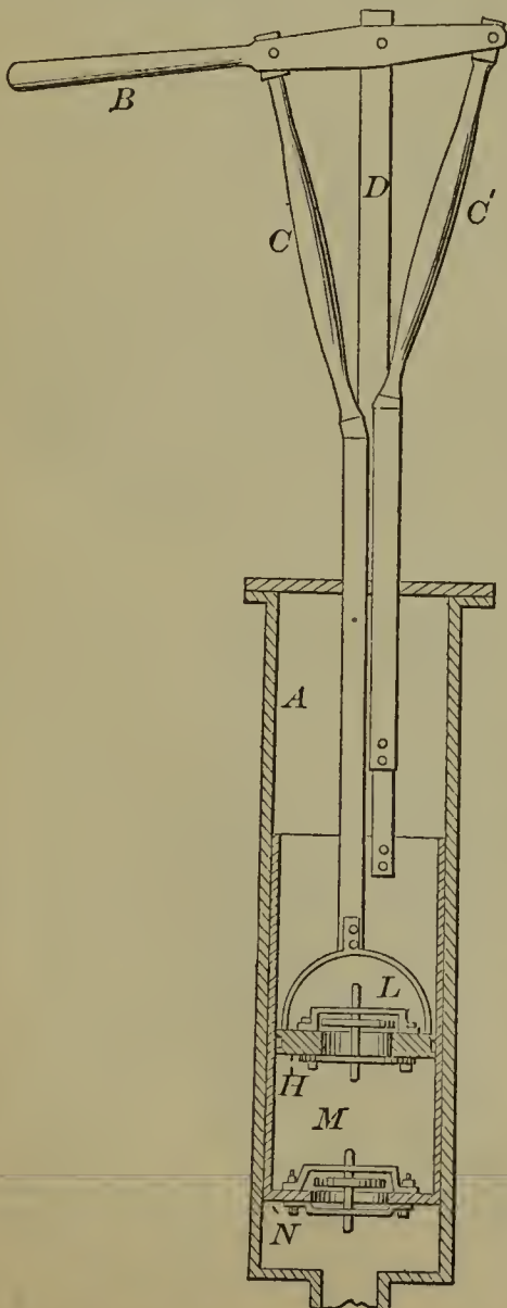
53185—A. Rewerick— Pump.
