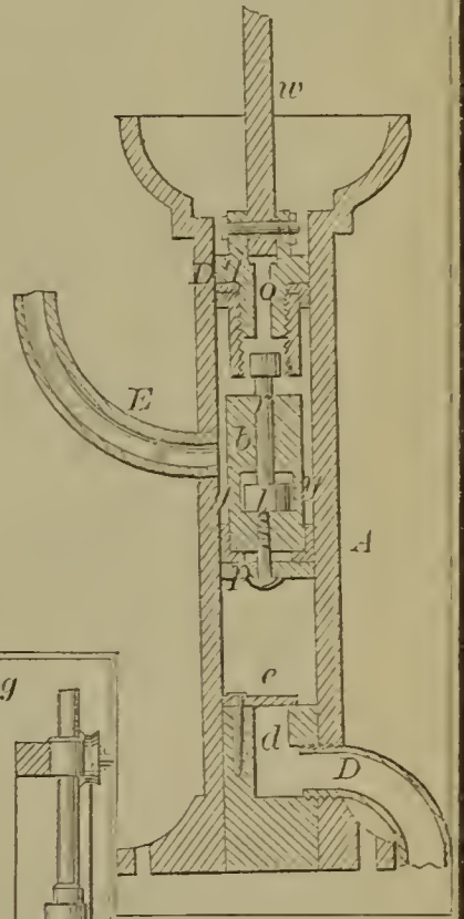
59030—D. L. Jaques— Pump.
