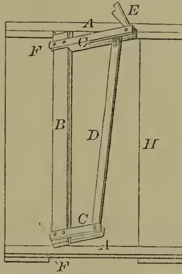
59662—L. S. Safford—Stanchion.
