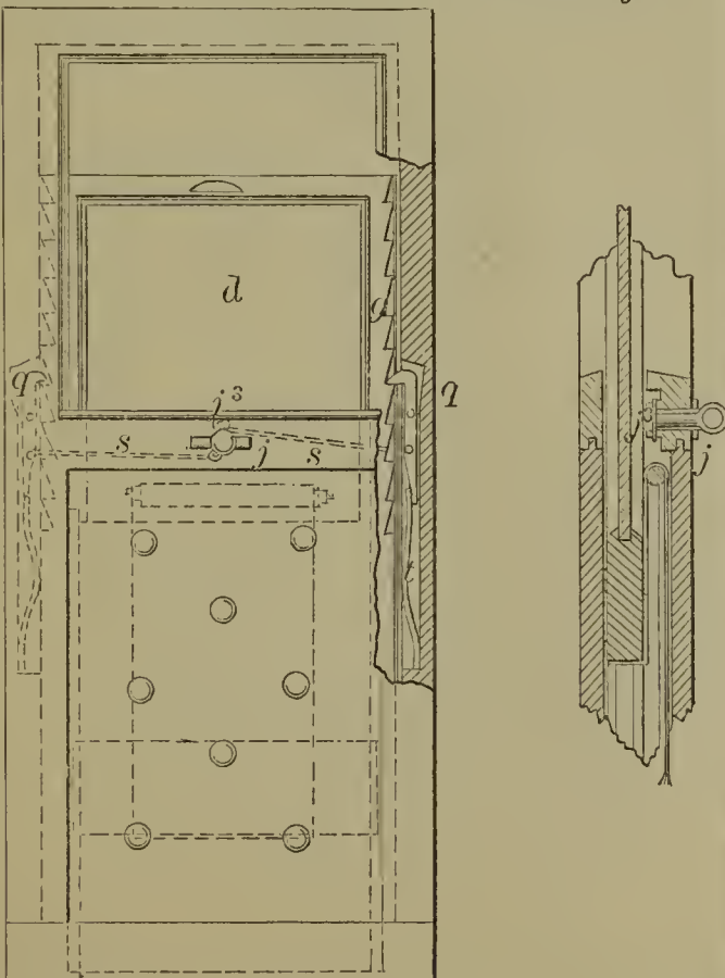
59521—J. K. Farnworth—Sash Fastening.
