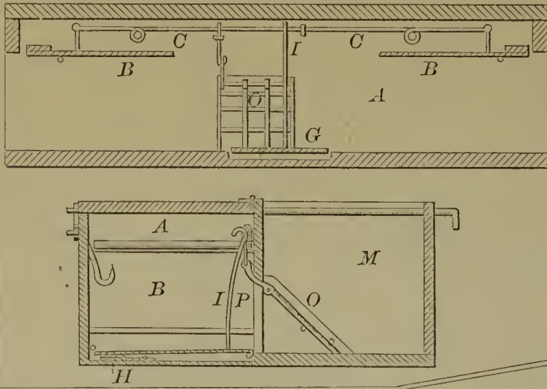
56736—W. A. Ellis—For Forming Plow Handles.
