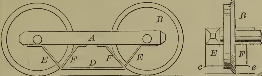
55350—J. Nusbaum—Car Truck.
