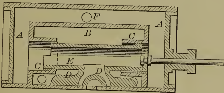
53707—R. D. Turner— Slide Valve.
