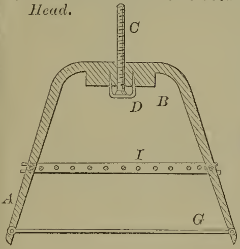
55857—W. H. Hart— Butter Worker.
