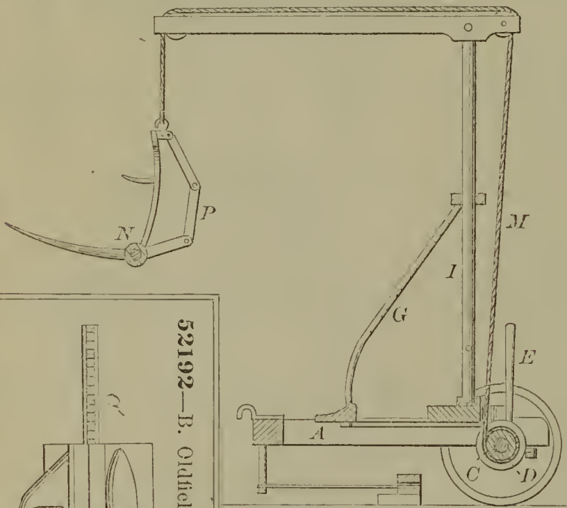
52190—Niles & Gillett—Loading Hay Wagons.
