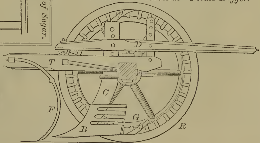
52428—A. Marcellus—Potato Digger.
