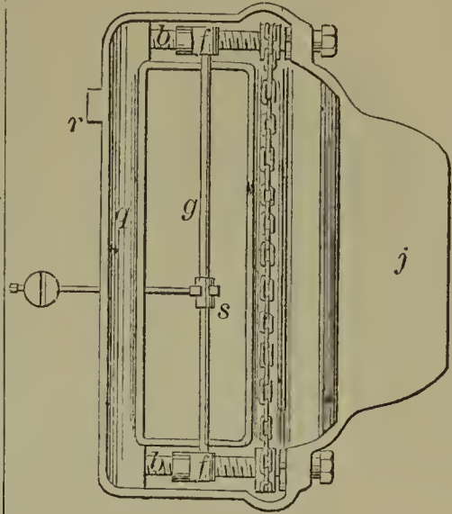
60176—J. H. Gray—For Picking Mill Stones.
