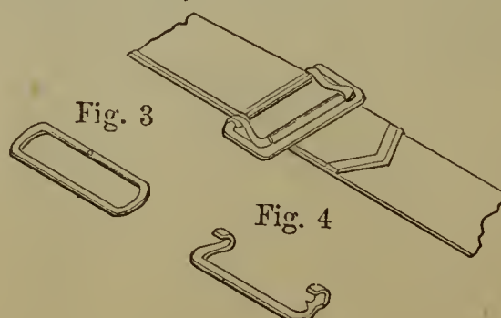
55113—G. R. Kelsey— Buckle.
