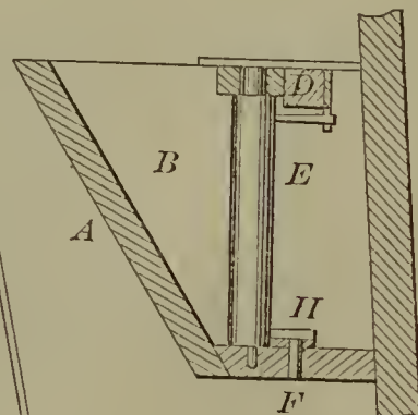
52295—W. S. & J. S. Lakin— Fertilizer Sower.
