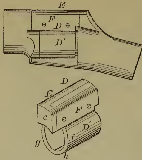
53521—J. E. Casey—Churn.
