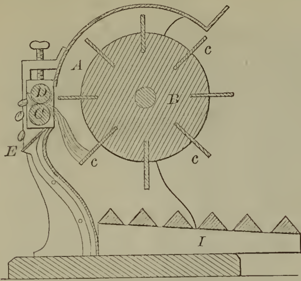
51892—J. E. Carver—Cotton Gin.
