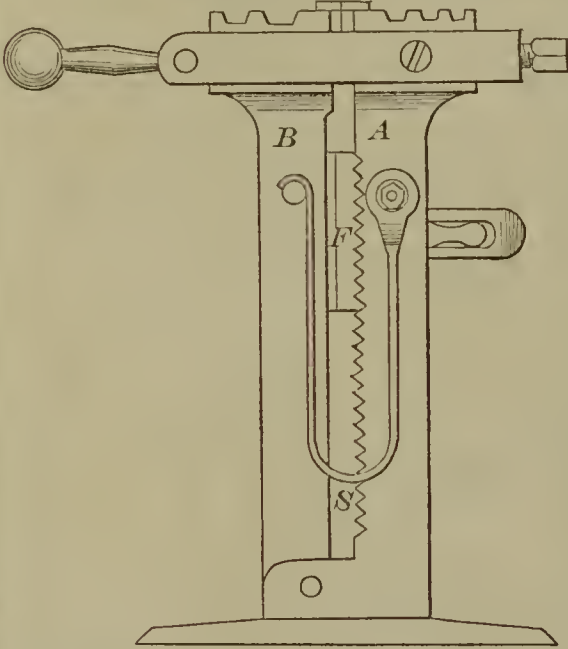
52394—N. Day— Boot Crimp.
