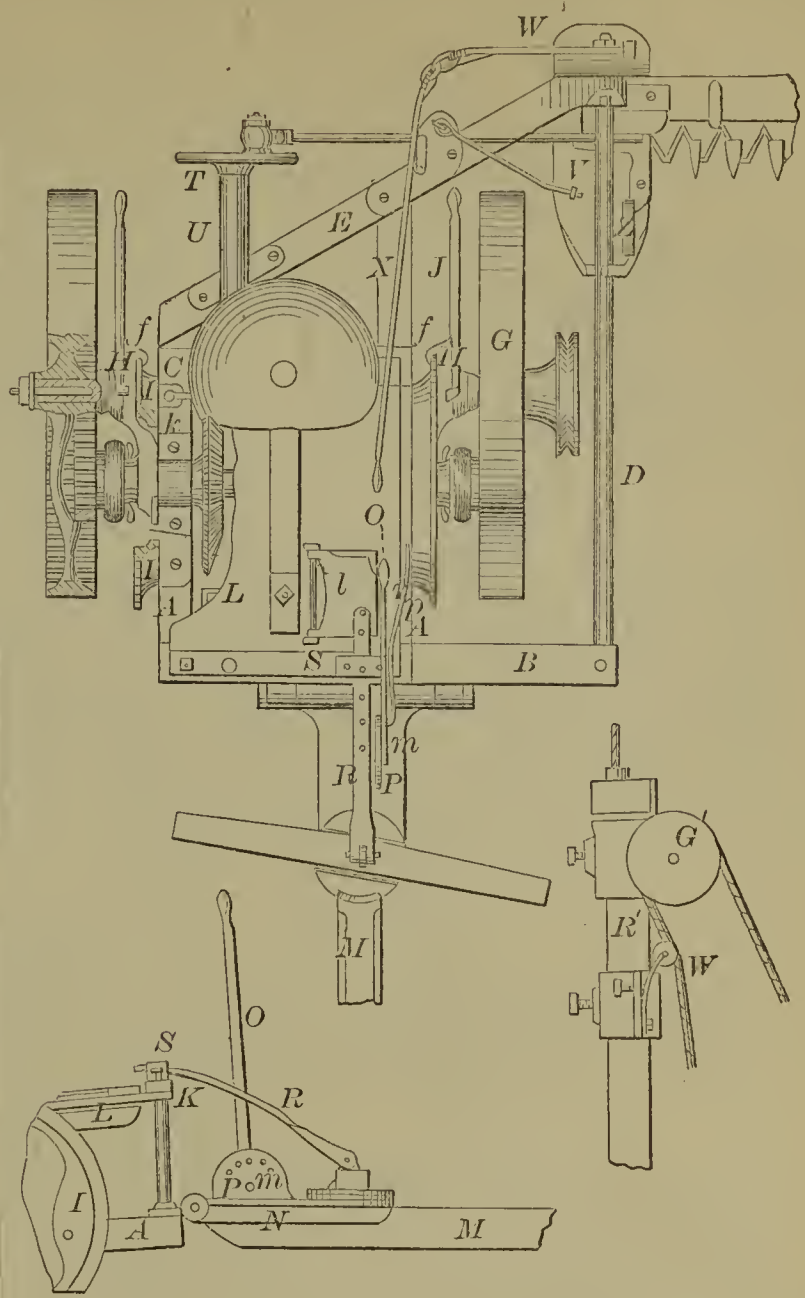
59302—W. N. Whiteley, Jr.—Harvester.
