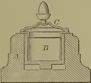
59223—P. K. Holbrook—Ink Cup.
