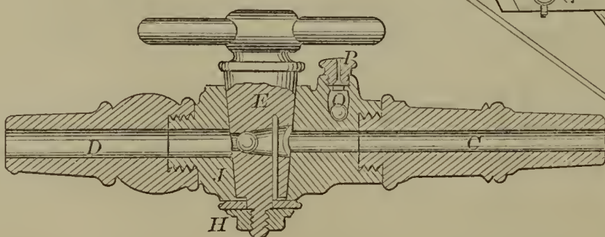
55527—C. L. Munns—Gas Inhaler.
