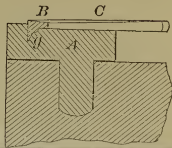
55221—J. Ashcroft—Low Water Detector.
