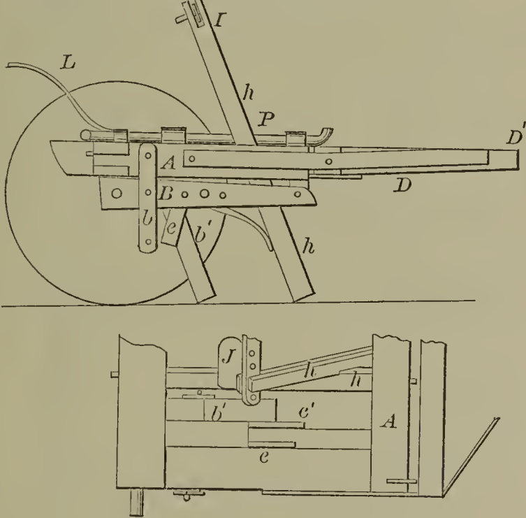
52049—G. L. Hutchinson— Cultivator.
