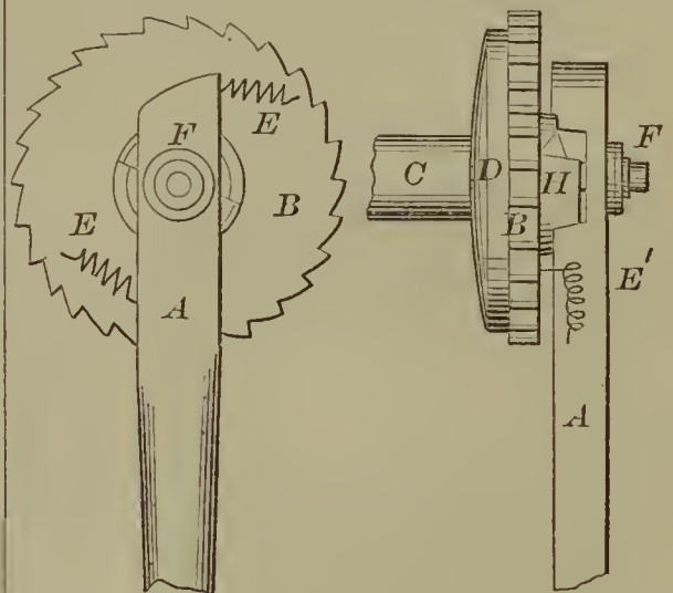
55977—A. S. Babbit—Water Elevator.
