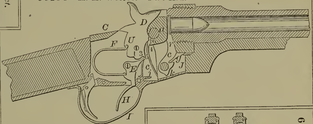
60106—H. H. Wolcott—Fire Arm.
