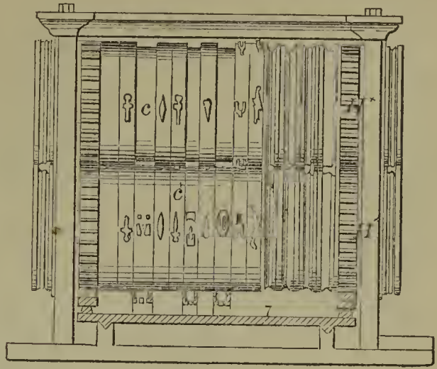
60322—H. Baines—For Rolling Metal.
