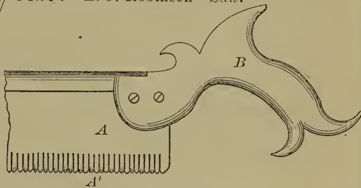
58297—E. J. Robinson— Saw.
