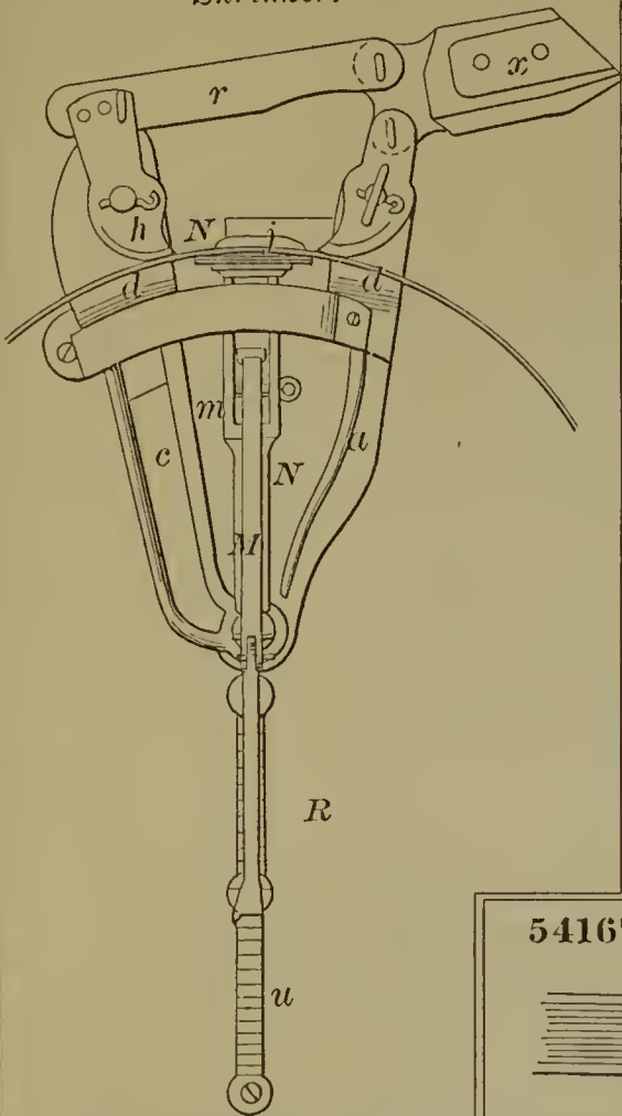
54166—W. W. Hubbard— Corn Planter.
