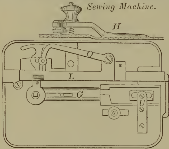
55865—J. A. & H. A. House—Button Hole Sewing Machine.
