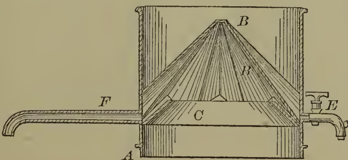
60079—B. P. Stebbins— Still.
