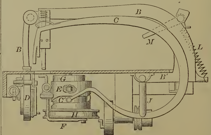
54577—T. L. Melone—Sewing Machine.
