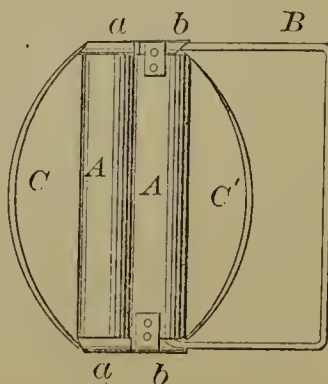
54164—L. Hover— Sad Iron Holder.
