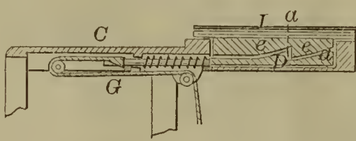
57394—G. B. Simpson—For Reducing Ores.
