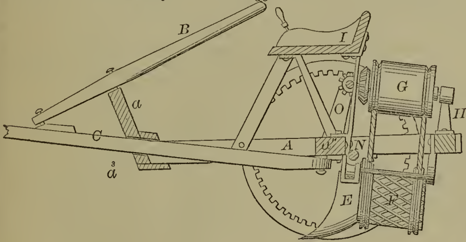
55206—F. A. Morley—Potato Digger.
