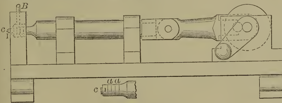
54468—E. E. Marsh— Eyelet Machine.
