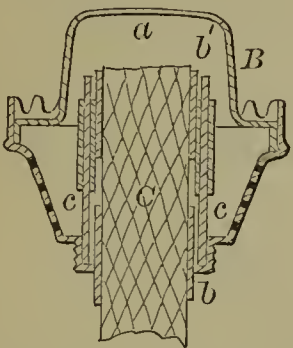
53953—P. Crans, Jr.— Lamp Burner.
