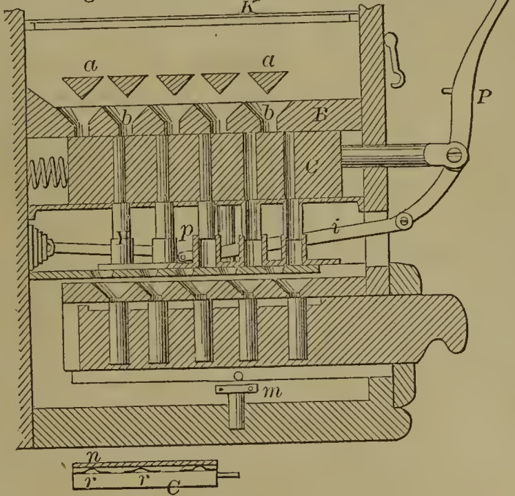
56489—Dodge & Smith—Cartridge Filling Machine.
