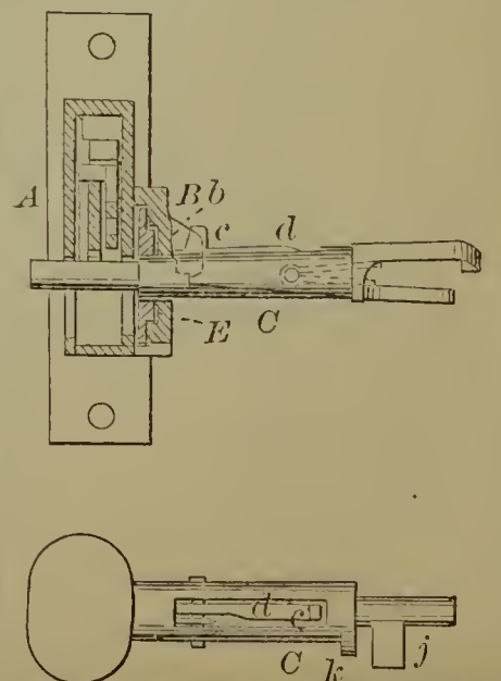
54952—D. A. Pratt—Lock.
