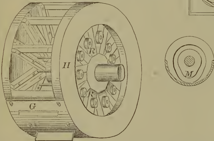
56973—J. Merkel—Paddle Wheel.
