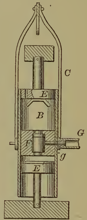
53750—H. M. Stoker—Pump.
