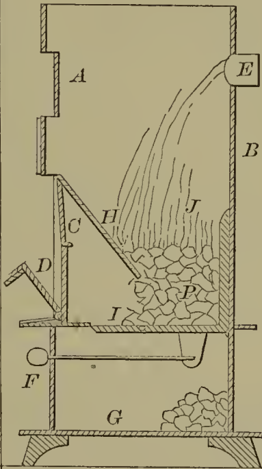
54943—H. Pelton— Lime Kiln.
