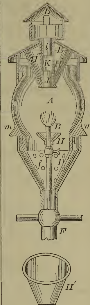
55686—T. T. Markland—Street Lamp.
