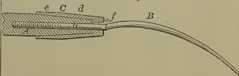
60065—W. F. Rundell—Hay Fork.
