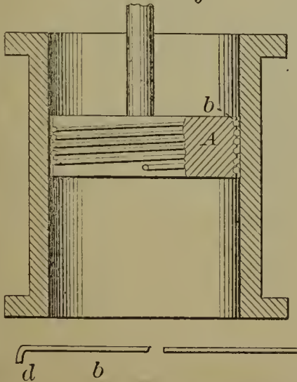
56699—A. S. Cameron— Piston Packing
