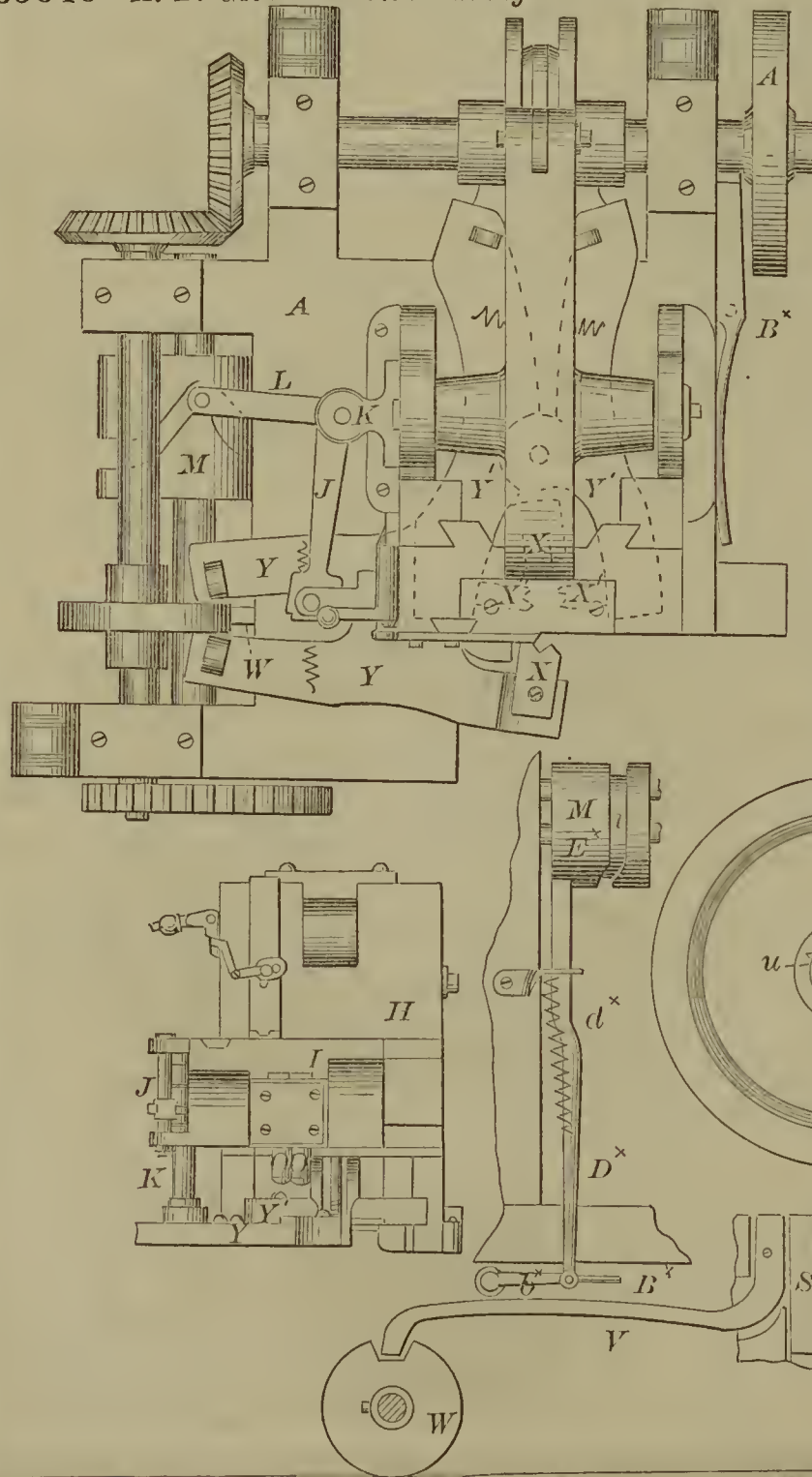
55646—A. B. Glover— Bolt Heading Machine.
