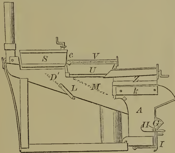
58331--J. E. Youngman--Evaporator.
