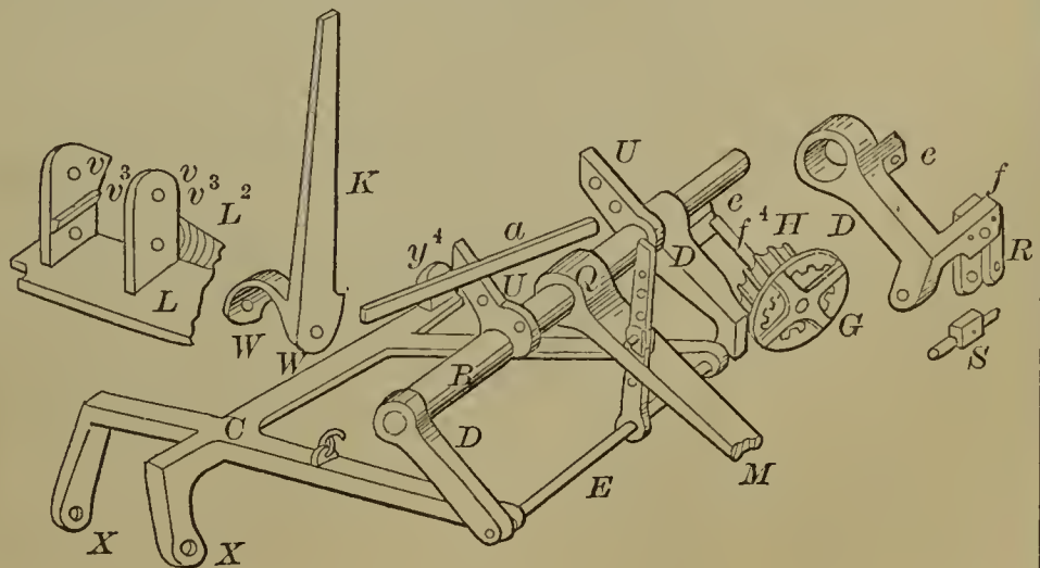
56397—E. T. Ford— Harvester.
