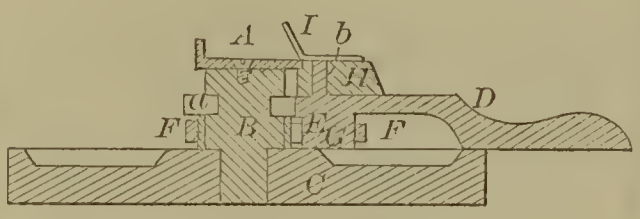
52430—O. H. & J. A. Marston—Heel Cutter.
