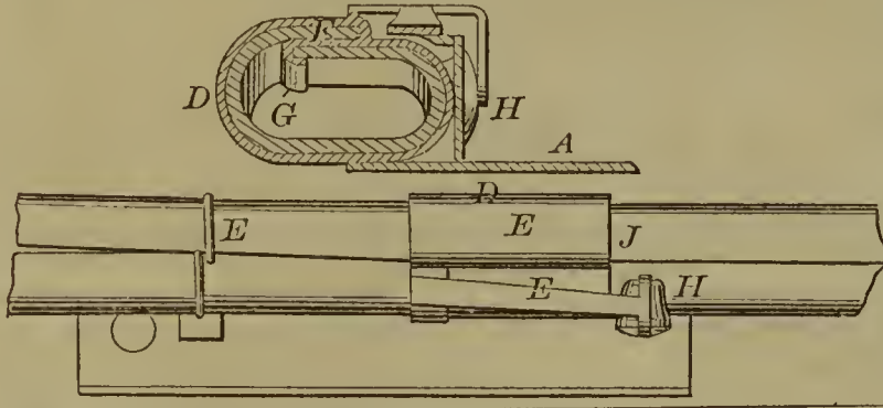
56530—S. Child, Jr.— Vapor Stove.
