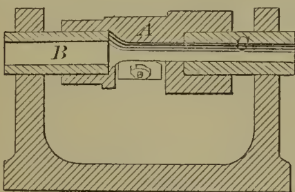
59552—J. Burt— Turning Lathe.
