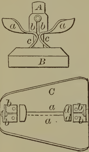
58070—E. T. Colburn— Sad Iron.
