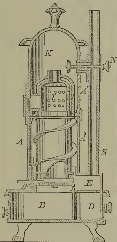
52033—J. D. Conner—Coal Stove.
