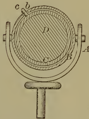
58402—M. Fryer—Oar Swivel.
