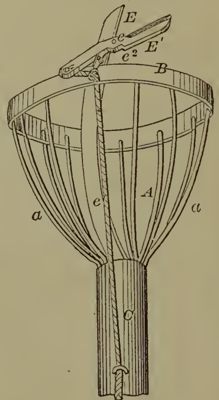
60565—H. L. Scott— Fruit Gatherer.
