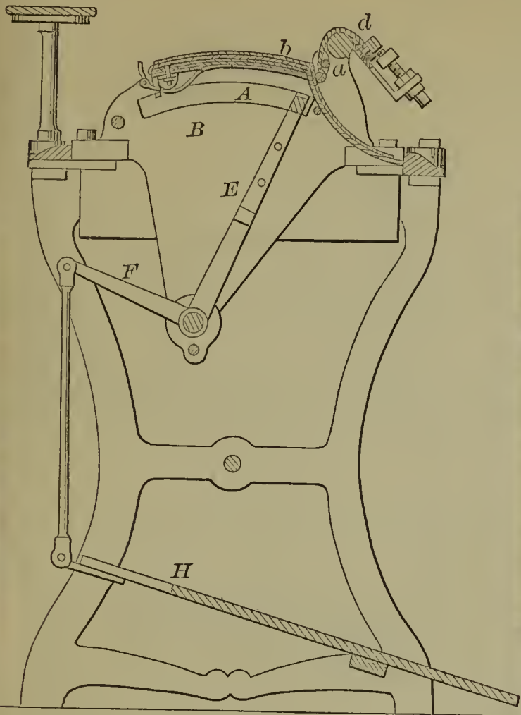
55217—G. A. Reiniger—Cigar Machine.
