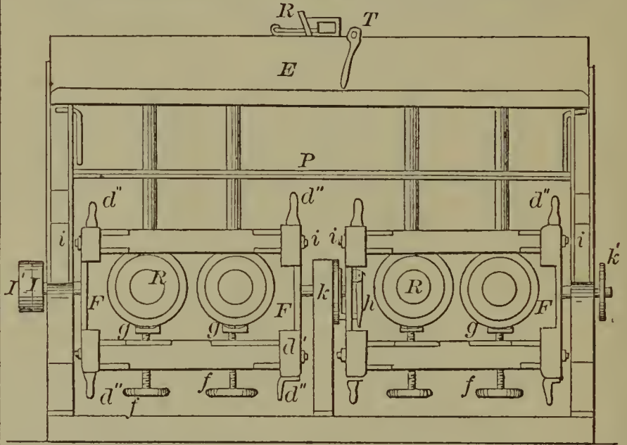
53180 I. Philbrook— Corn Husker.
