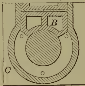
59632—C. M. Oliver— Axle Box.
