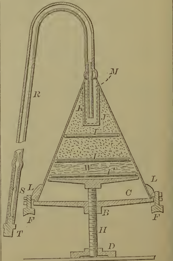
59467—T. Simmons—Filter.
