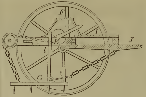
57222—J. W. Tyson—Cultivator.
