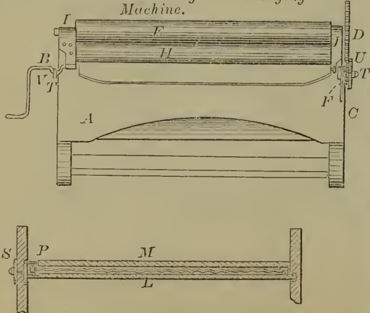
59041—J. S. Lash—Clothes Wringer.
