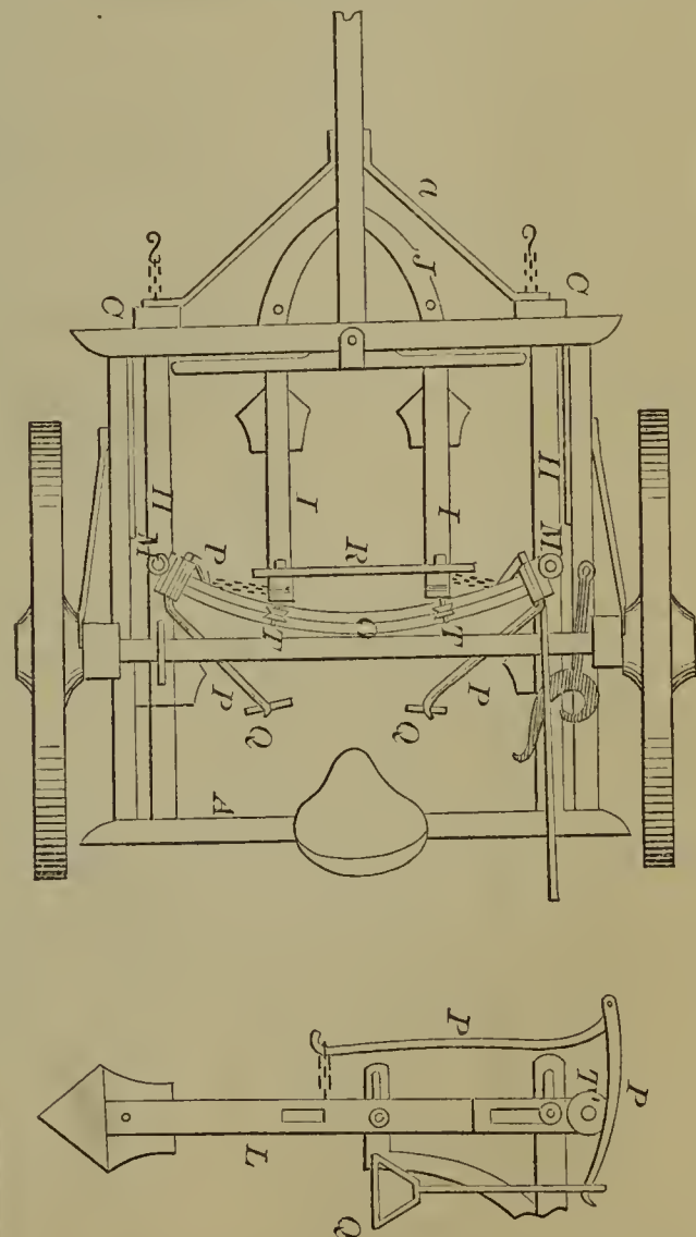
53303—M. H. Hullinger— Cultivator.
