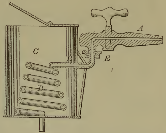
55962—J. R. B. Schwarze— Liquid Cooler.
