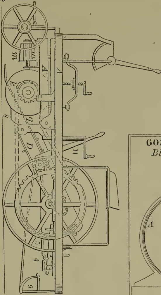
Sled Brake.
