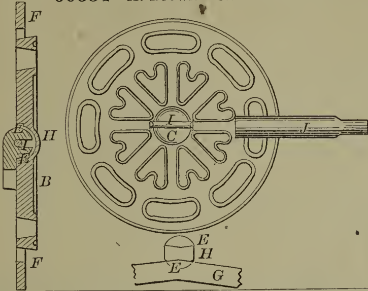
60336—J. H. Brown— Spring Toy.
