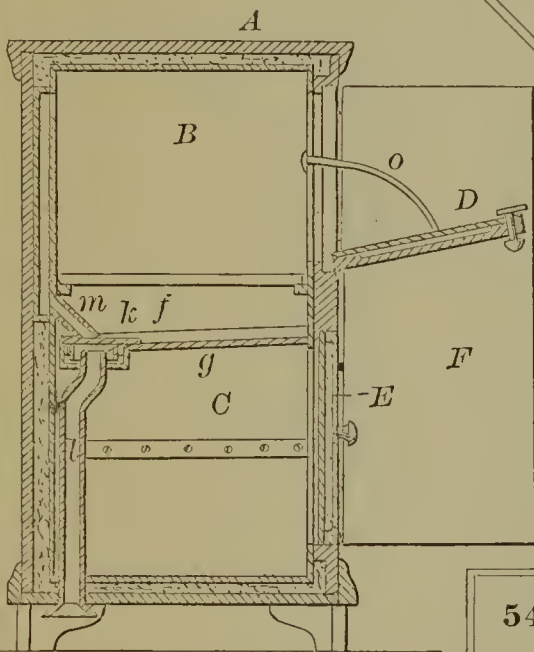
54980—P. A. Vogt— Refrigerator.
