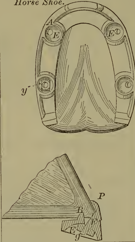
55045—Behel & Buell— Horse Shoe.
