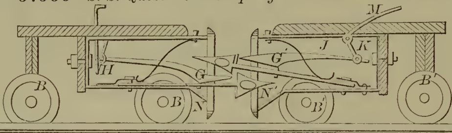
57566—S. S. Quest—Car Coupling.
