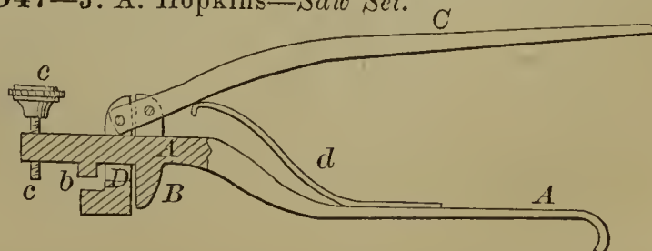
54547—J. A. Hopkins— Saw Set.
