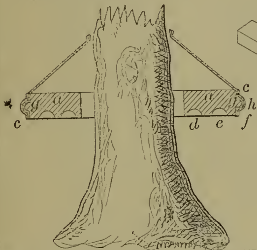
59623—B. Merritt, Jr.—Tree Protector.
