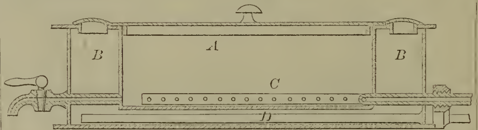
52277—S. B. Ellithorp—Refrigerator.
