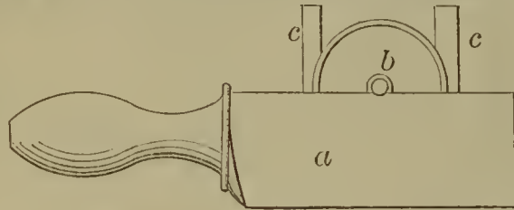
56264—J. B. Pratt— Knife Sharpener.
