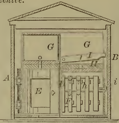
57272—L. W. & S. W. Albee— —Beehive.
