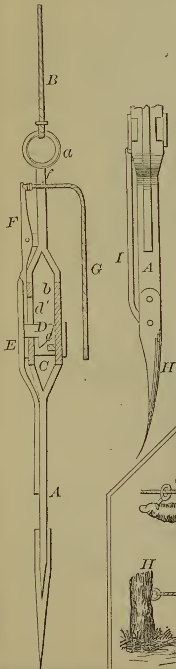
52805—B. F. Hisert—Horse Hay Fork.
