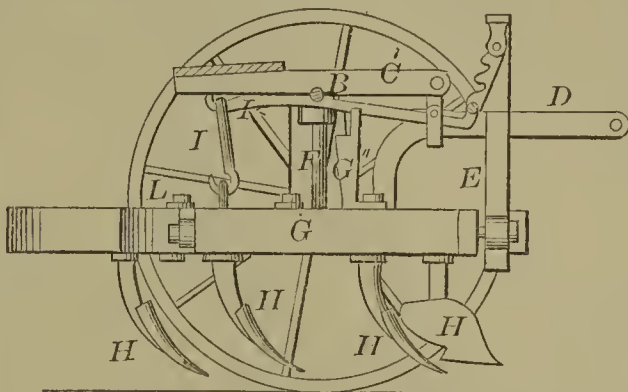
59454—C. S. Roberts—Cultivator.
