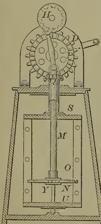
60289—A. J. Vanatta— Churn.
