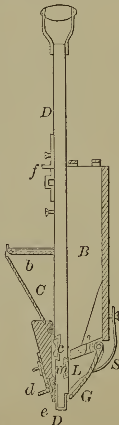
60200—J. H. Latimer— Hand Seed Planter.
