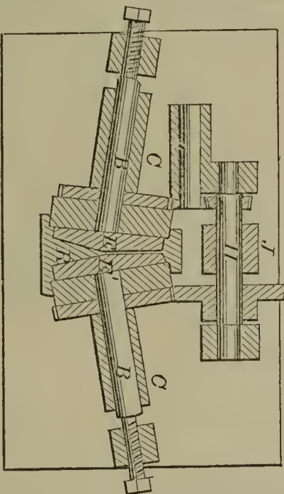
52363—H. Kellogg—Quartz Mill.
