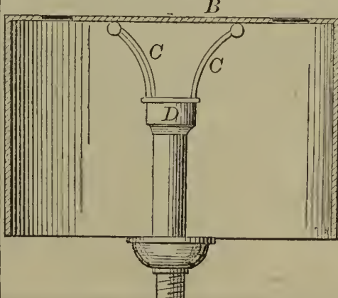
57578—H. S. Saroni—Vapor Burner.
