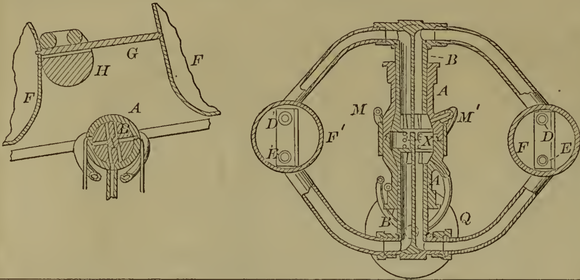
56096—G. A. Riedel—Automatic Boiler Feeder.
