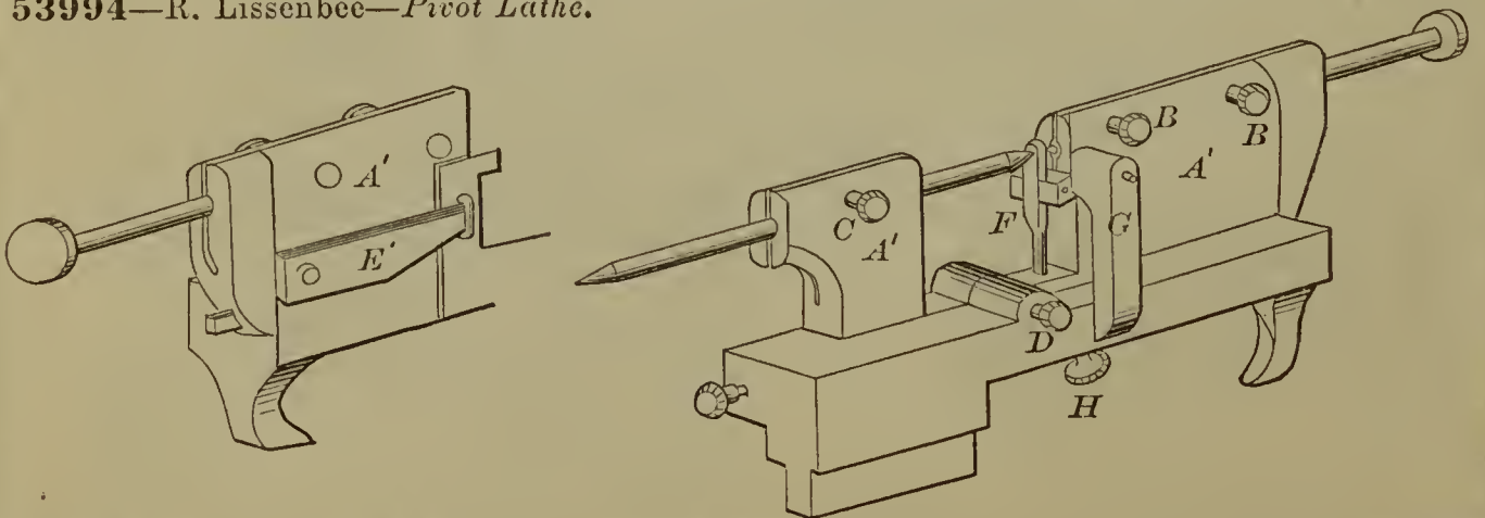
53994—R. Lissenbee— Pivot Lathe.
