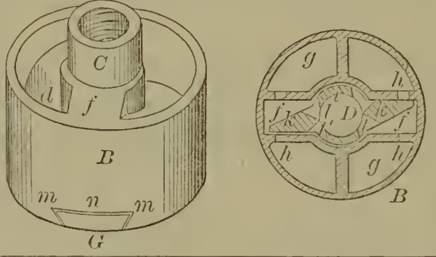
52431—Mason & Gill—Pump.
