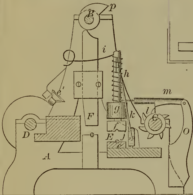
53351—F. Schweizer—Bolt Heading Machine.
