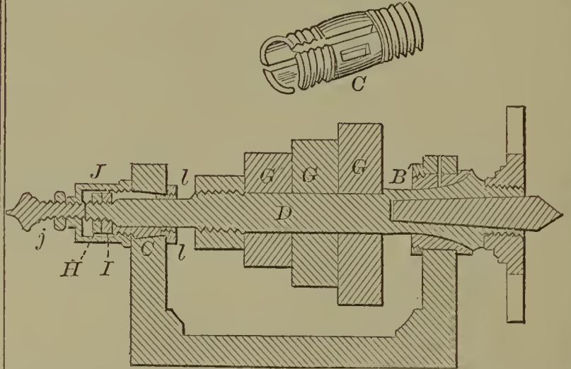
60155—R. W. Drew— Turning Lathe.
