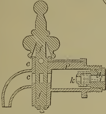
58356—E. Candler— Faucet.
