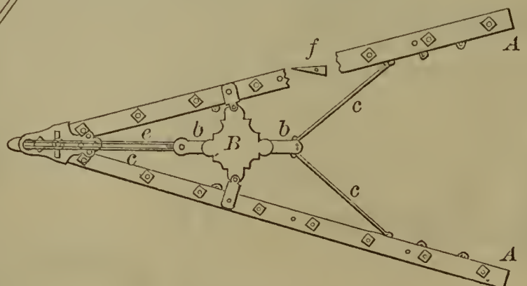
56286—E. M. Sorley— Cultivator.
