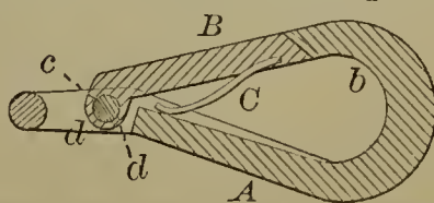
53122—E. S. Dawson— Snap Hook.
