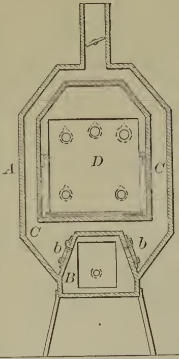
51792—J. I. Boone—Fruit Dryer.
