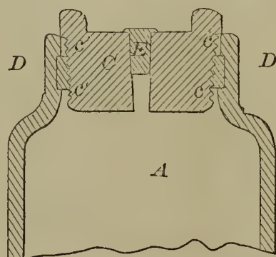
52379—E. Bennett— Fruit Jar.
