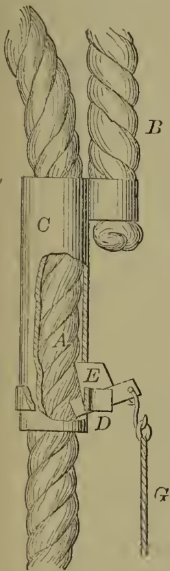
59585—J. Gifford, Jr.— Hay Elevator.
