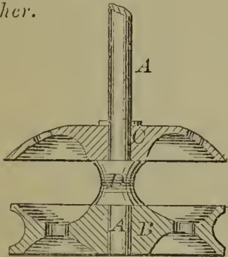
56730—A. L. Dewey—Sewing Machine.
