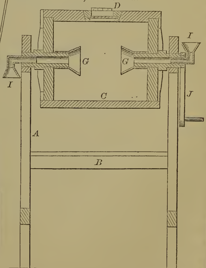
54861—A. Clift, Jr.— Churn.
