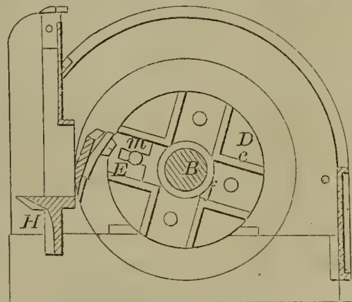
57363—J. H. Mumma— Straw Cutter.
