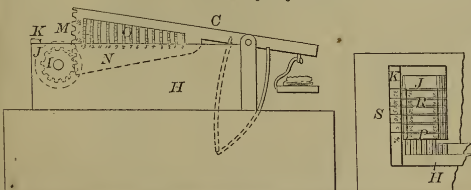
55503—J. S. & E. B. Lake— Weighing Scale.
