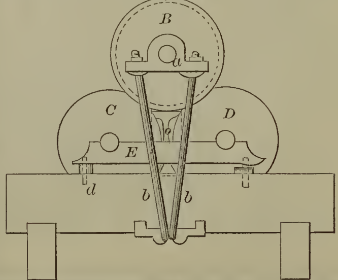
52127—G. Bevitt—Sugar Mill.
