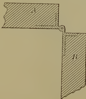
54171—D. C. Jordan, Sr.— Hinge.
