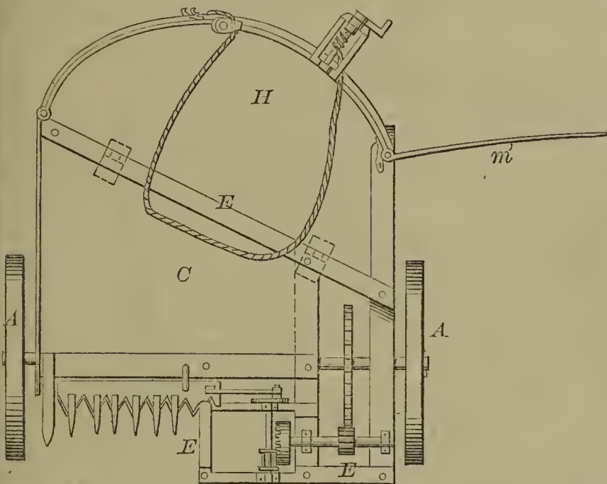
57114—F. F. Fowler—Horse Hay Fork.
