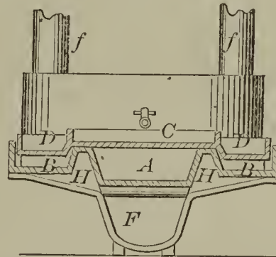
52022—A. L. Brink— Sugar Evaporator.
