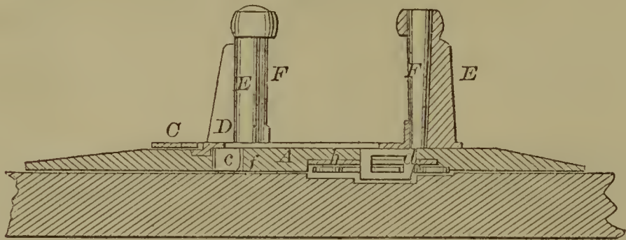
56086—J. W. Norcross— Row Lock .
