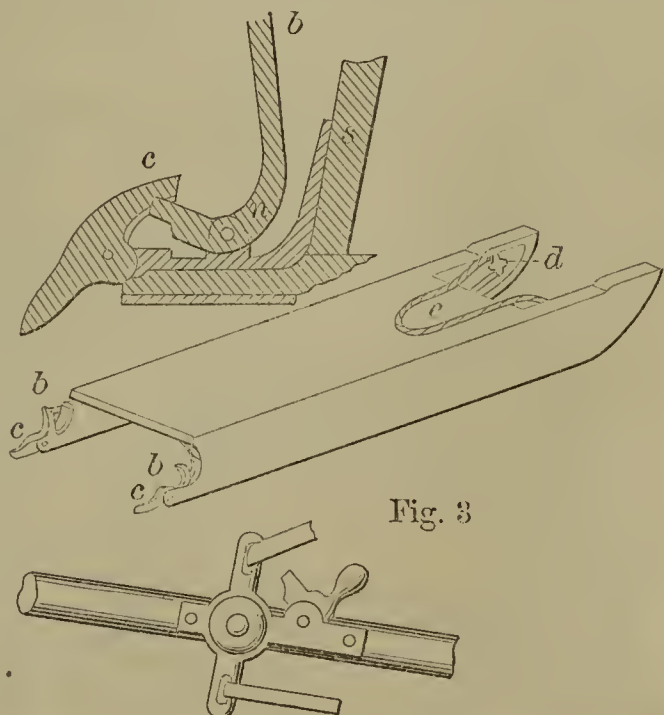
52663—S. R. Boure—Sled.
