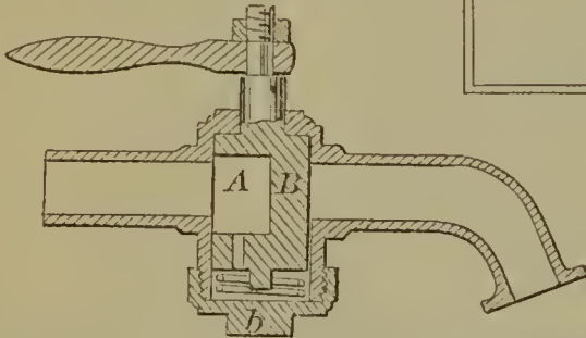
54305—W. H. De Valin— Stop Cock.
