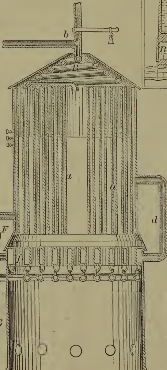
60562—H. S. Saroni— Steam Generator.
