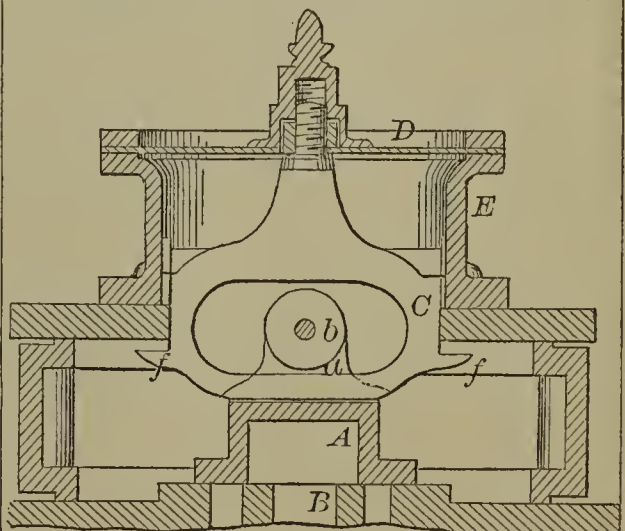
60081—W. J. Stevens— Slide Valve.
