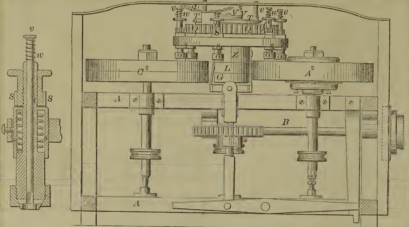
57472—P. Carbach—Melodeon.
