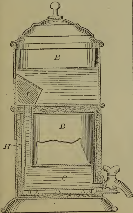
53998—T. T. Markland, Jr.— Water Cooler.
