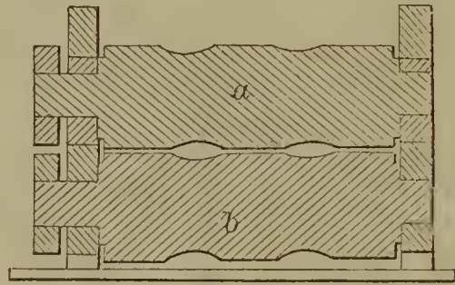
57388—J. S. Seaman—Rolling Iron or Steel.
