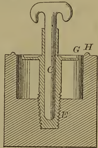
56542—A. B. Ely— Telegraphic Insulator.
