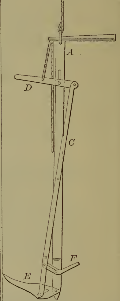
55035—T. H. Arnold— Horse Hay Fork.
