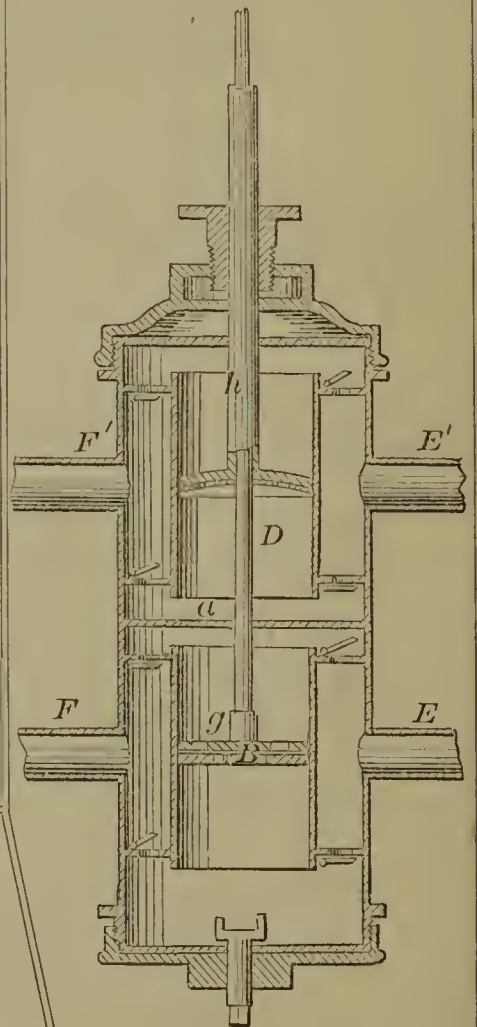
59125—J. N. Dennison—Pump.
