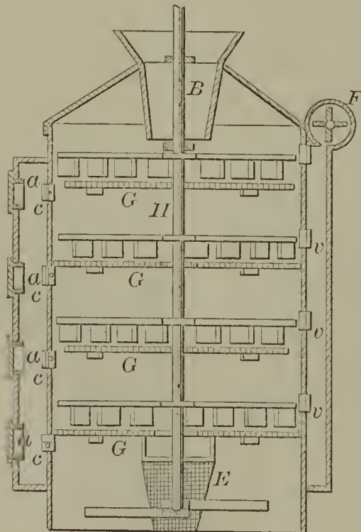
51880—R. T. Sutton—Grain Dryer.
