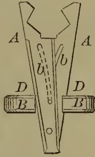
60625—A. K. & B. H. Foster— Cotton Cultivator.
