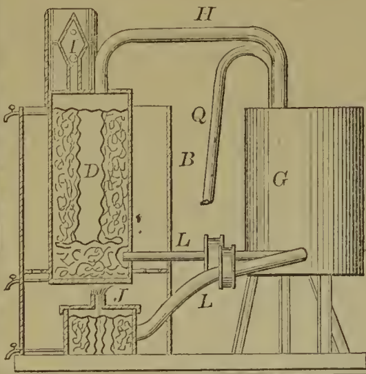
57684—F. A. Deutenberg—Tuyere.
