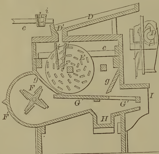
55362—D. K. Reeder—Corn Sheller.
