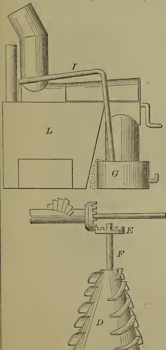
54028—G. B. Simpson— Amalgamator.
