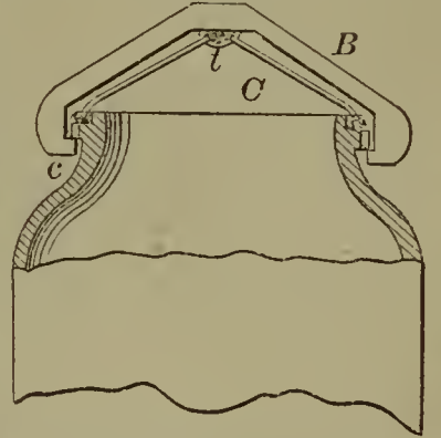
58674—G. A. Reynolds—Fruit Jar.
