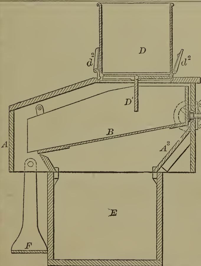
58132—C. L. Pierce— Ash Sifter.
