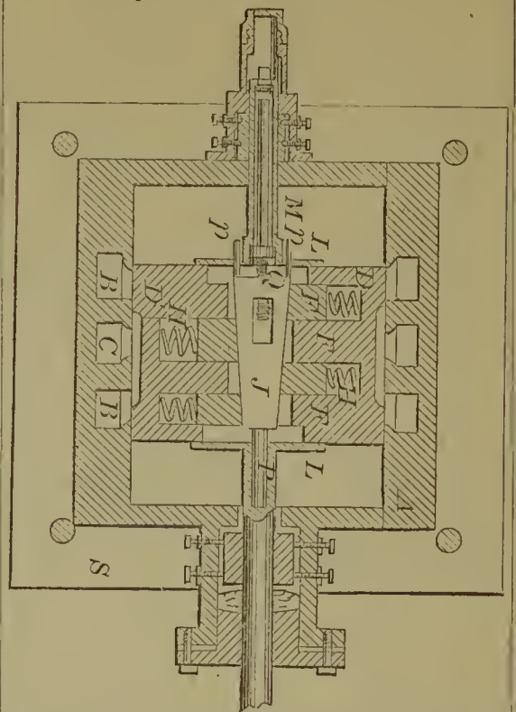
59478—J. M. Talbott— Tobacco Press.
