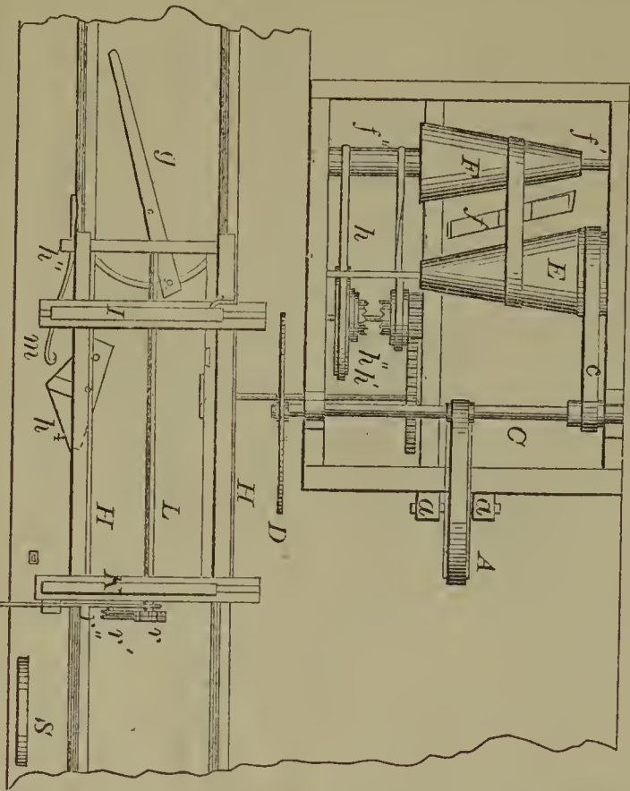
60374—J. A. Holford— Saw Mill.
