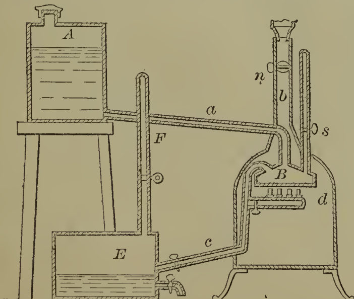
57915—J. H. Irwin— Retort for Generating Gas.
