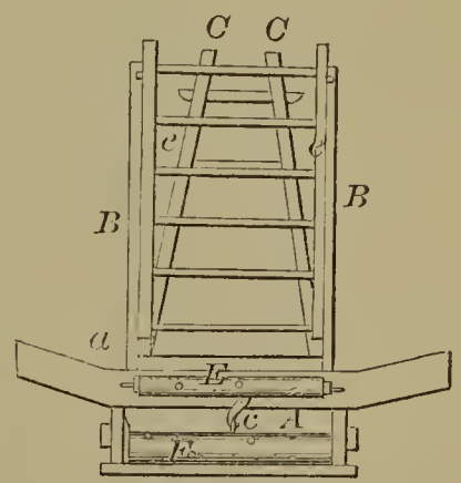
58280—A. Naramor—Wagon Hay Rack.
