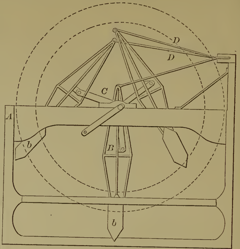
54801—A. A. Wilder—Propeller.
