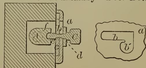
57616—G. T. Allamby—Door Bolt.
