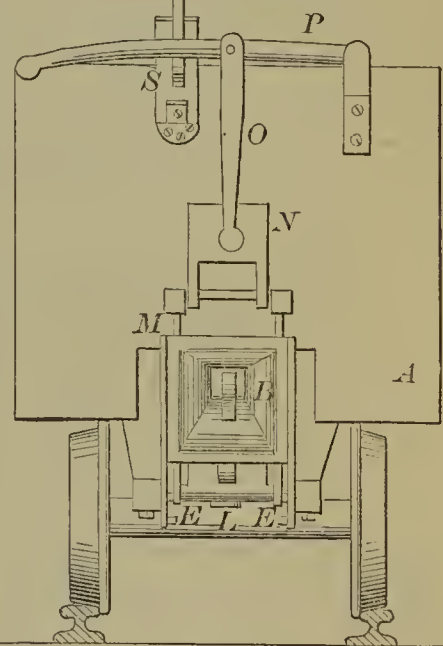
56837—W. Van Valkenburgh—Car Coupling.
