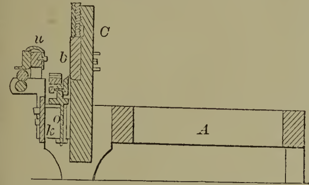
58642—G. M. Heim—Washing Machine.
