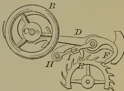
54277—B. Bacon—Clock Escapement.
