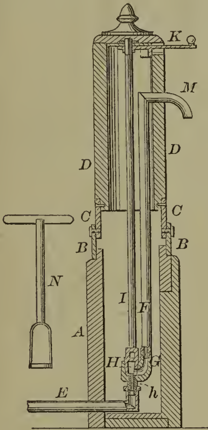
60423—J. P. Riley—Hydrant.
