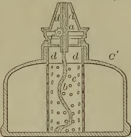
52369—E. F. Rogers—Lamp.
