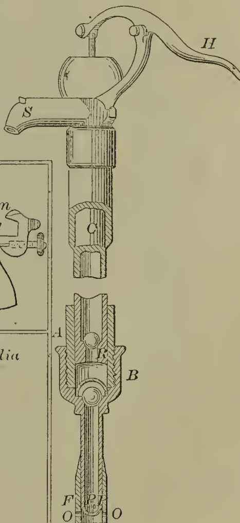
57595—R. E. Strait—Pump.
