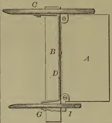
57582—O. W. Seely—Churn.
