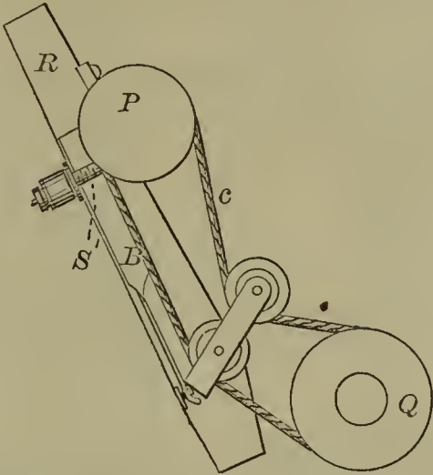
52330—J. E. Short—Broom Head.
