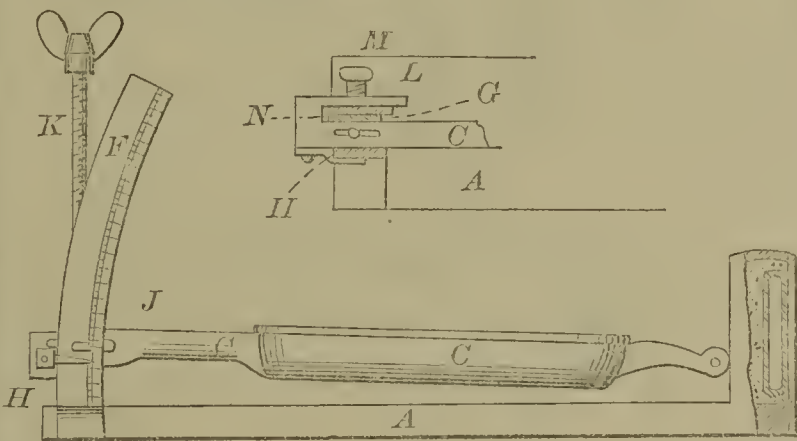
52579—R. Ledig— Spirit Level.
