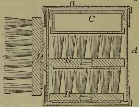
53111—E. S. Carter—Boot Blacking Case.
