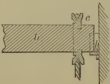
55454—J. B. Bailey— Curtain Fixture.
