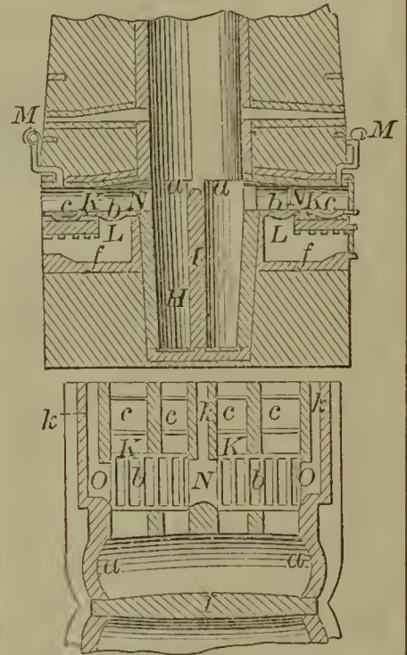
55701—J. Perkins— Cotton Seed Huller.
