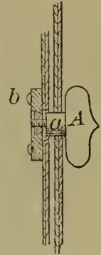
53333—E. H. Porter—Swivel Button.
