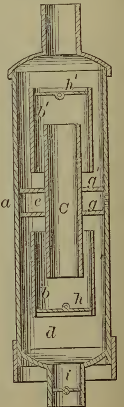
55419—W. Kroeger—Stove Pipe Drum.
