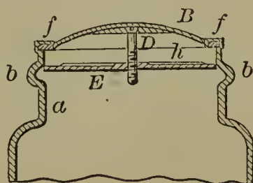
60468—J. Borden— Fruit Jar.
