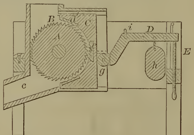
55701—J. Perkins— Cotton Seed Huller.
