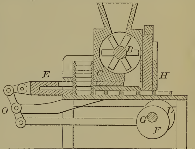
54752—A. R. McNair—Brick Machine.
