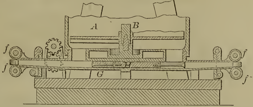
57415—R. L. Walker— Brick Machine.
