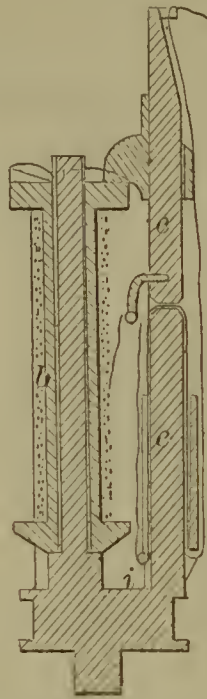
57201—T. J. Sloan— Braiding Machine.
