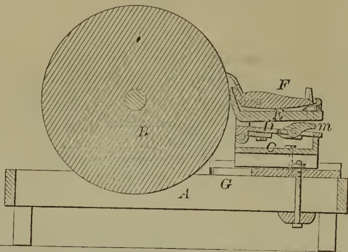
57566—S. S. Quest—Car Coupling.
