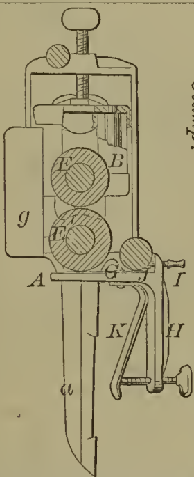
58698—C. W. Wailey— Cotton Tie.
