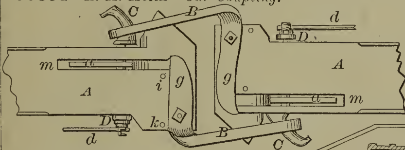
60384—E. H. Keith—Car Coupling.
