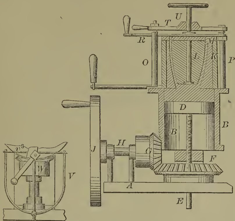
60091—W. W. Tice—Moulder's Clamp.
