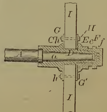
57855—H. B. Buch—Metallic Hub.
