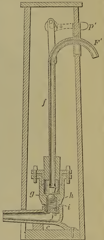
55136—R. A. McCauley—Hydrant.
