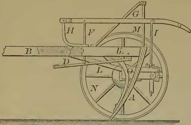
57757—N. Peck— Earth Scraper.
