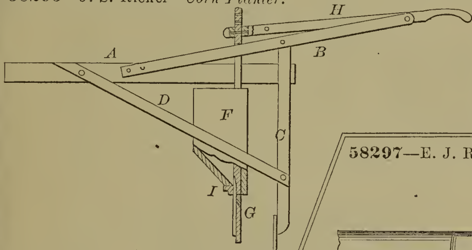
58295—J. S. Rickel— Corn Planter.
