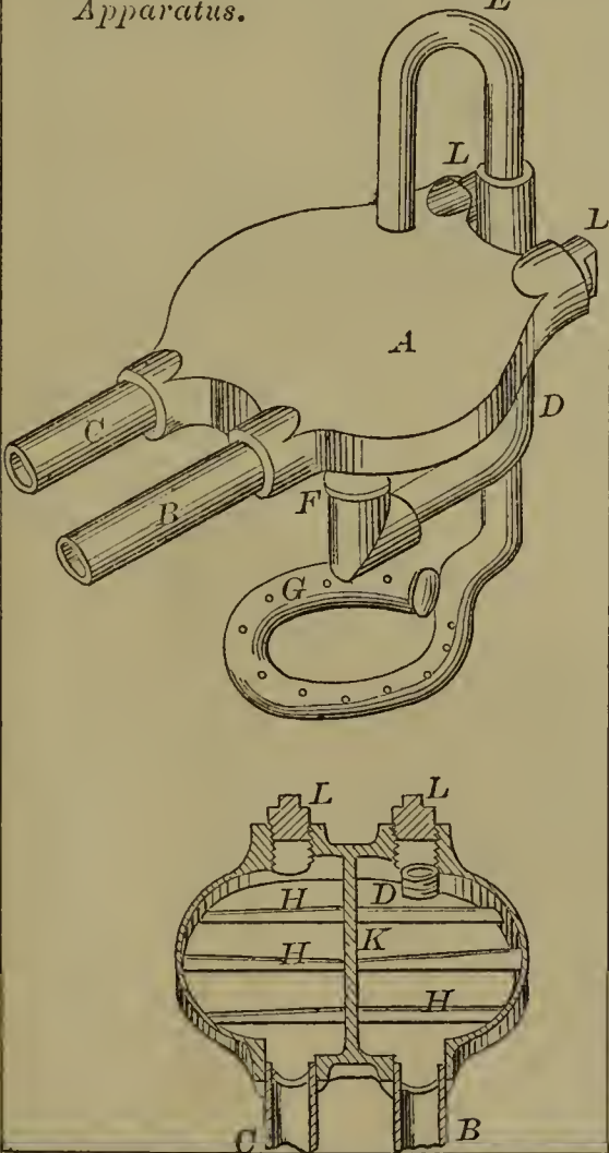
56143—A. J. Griffin—Gas Burning Apparatus.
