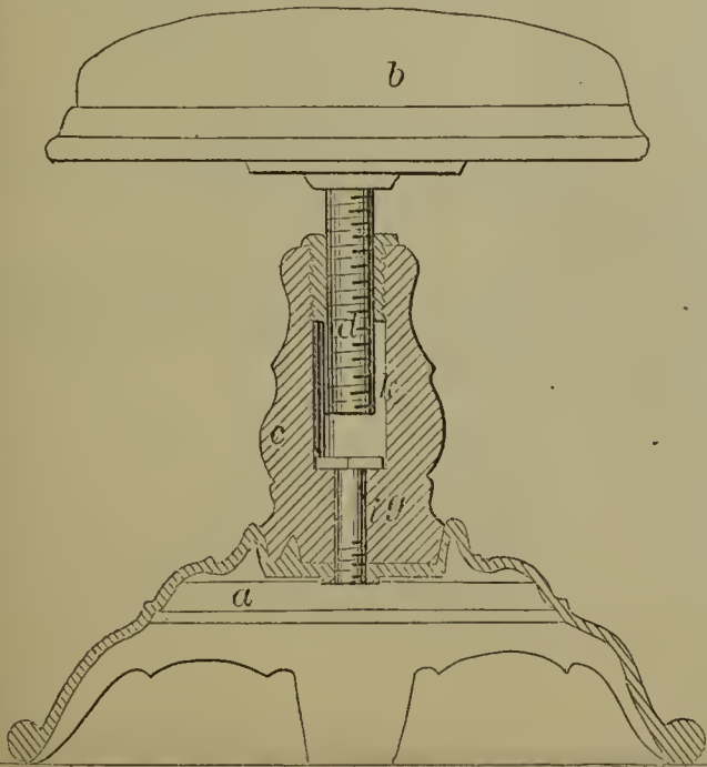
58979—J. Briggs— Piano Stool.
