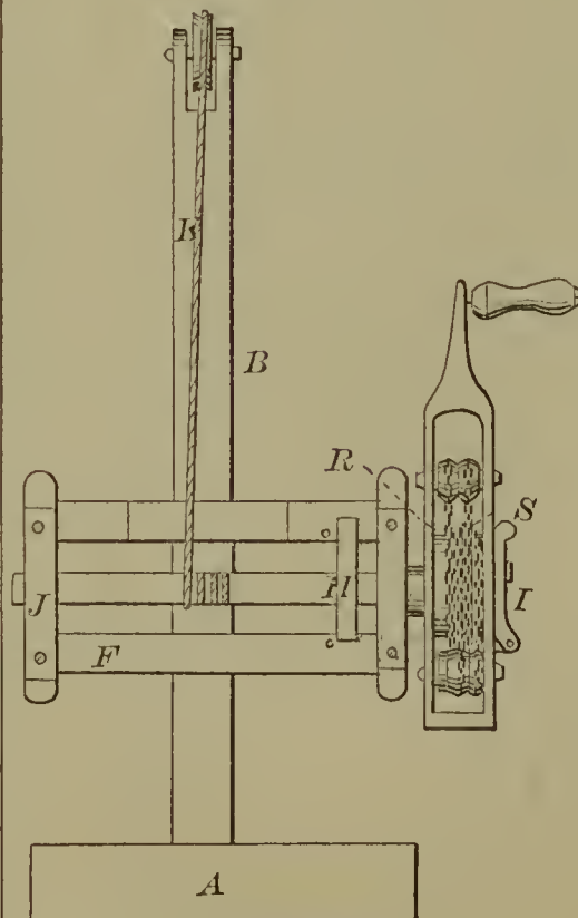
54419—H. F. Shaw— Hoisting Apparatus.
