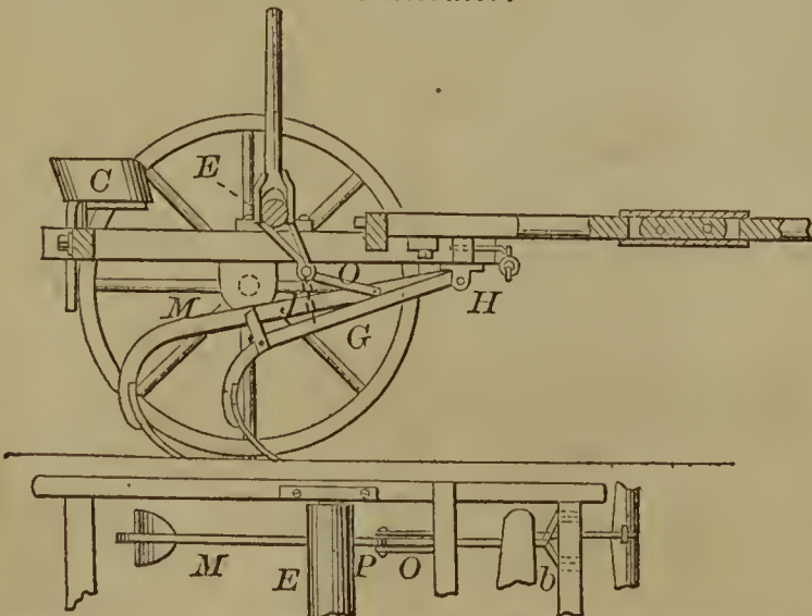
56511—J. N. Arvin—Cultivator.
