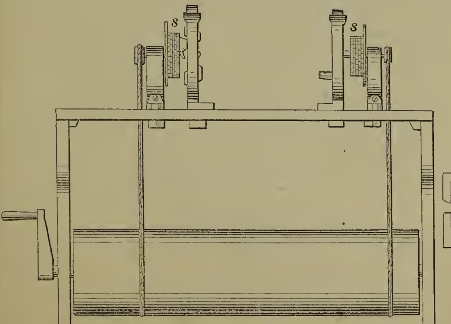
54222—J. M. Seymour— For Tenoning Blind Slats.
