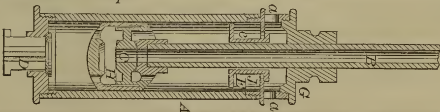
52709—H. A. M. Harris— Pump.
