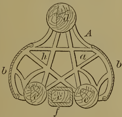
54781—W. H. Sargent— Washing Machine.
