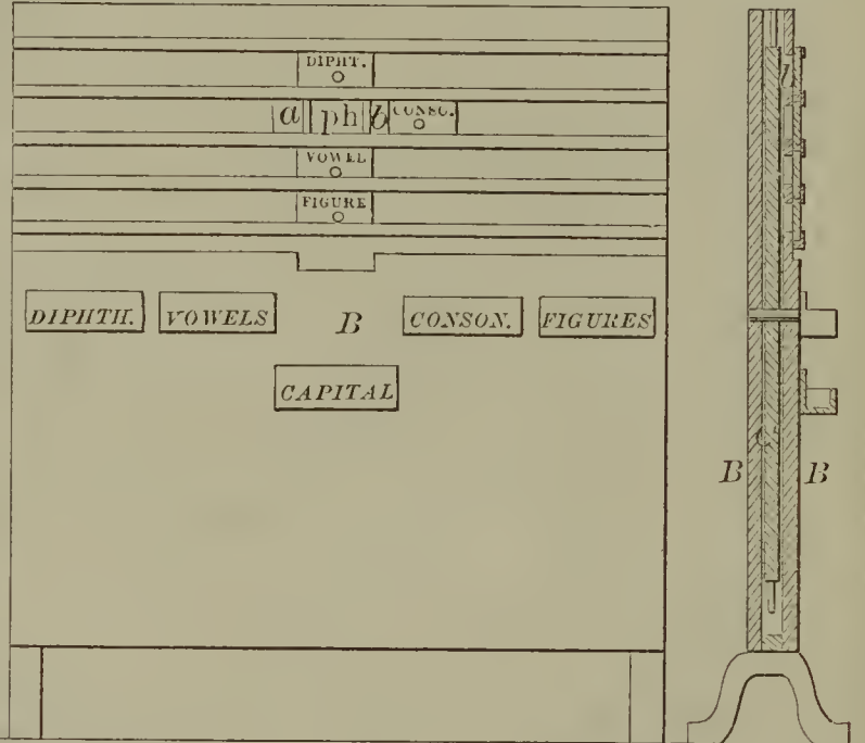
51864—J. H. R. Reffelt— Alphabeticon.
