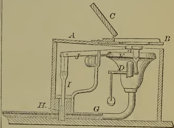
55766—O. S. Pettit—Water Closet.
