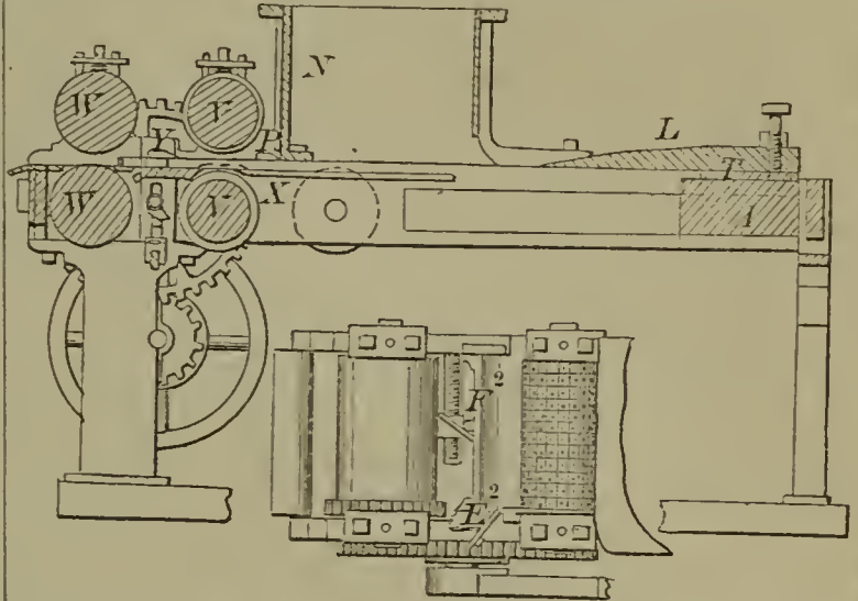
58938—A. M. Connett—Shingle Machine.
