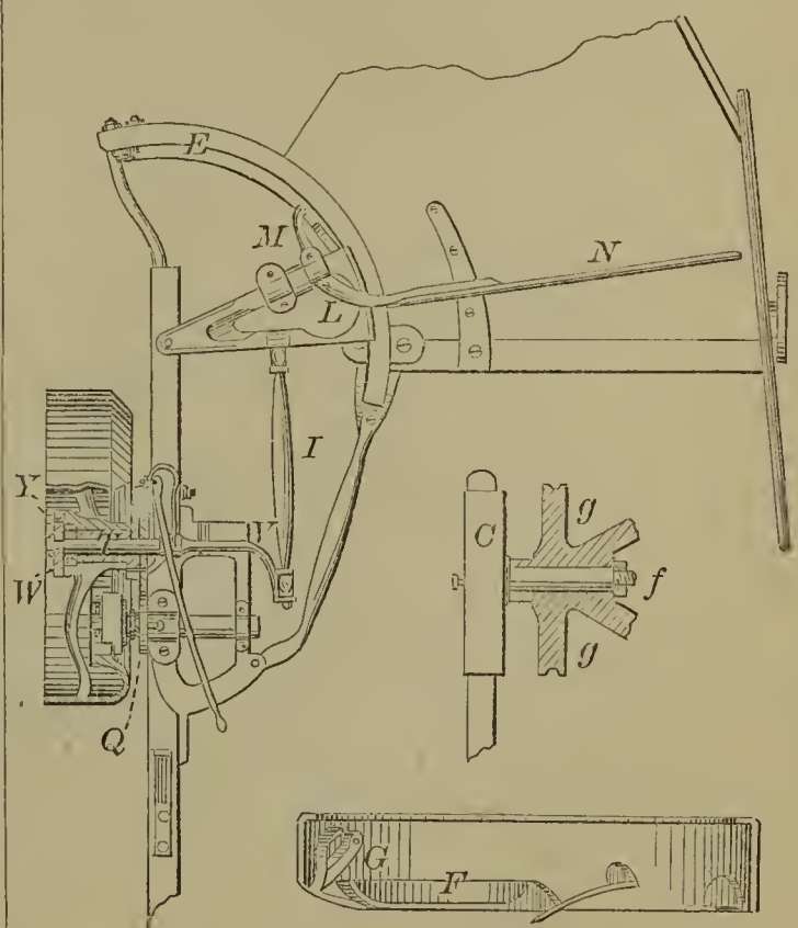
59303—W. N. Whiteley, Jr.—Harvester.
