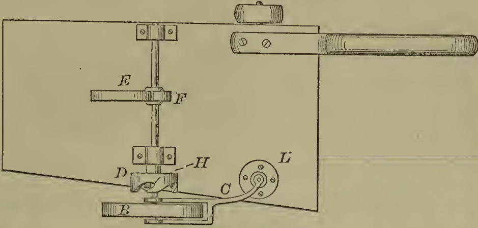
52396—N. A. Dederer—Harvester Rake.
