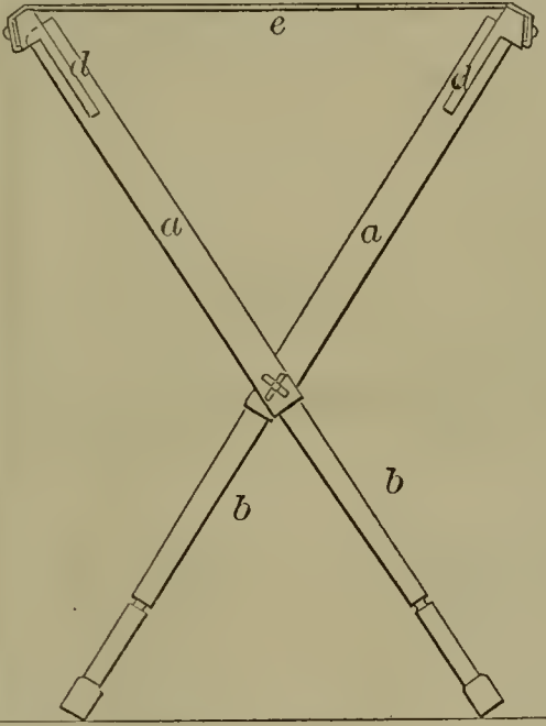
52412—C. G. Herbert— Camp Stool.
