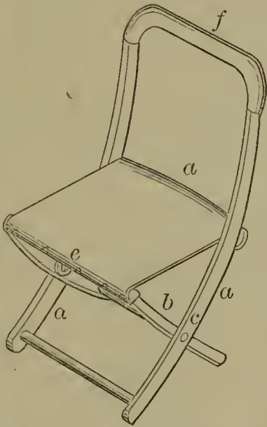
52488—I. N. Dann— Folding Chair.
