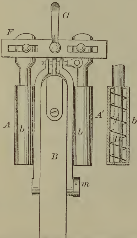
52123—L. W. Alden—Plow Clevis.
