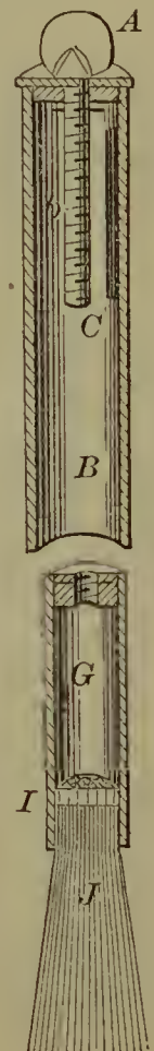
53923—D. K. Herr—Stencil Brush.
