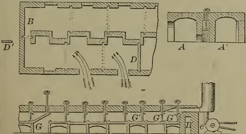
58941—Haueisen, Wagner & Nulsen—Brick Kiln.
