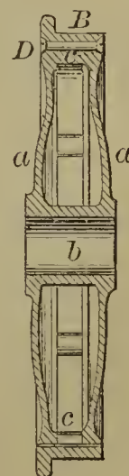
85298—E. S. Robinson— Car Wheel.
