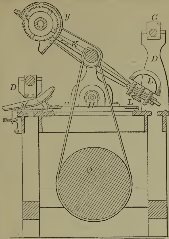
60321—J. E. Atwood—Saw.
