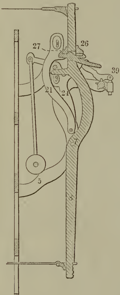
51928—G. Crompton— Fancy Loom.
