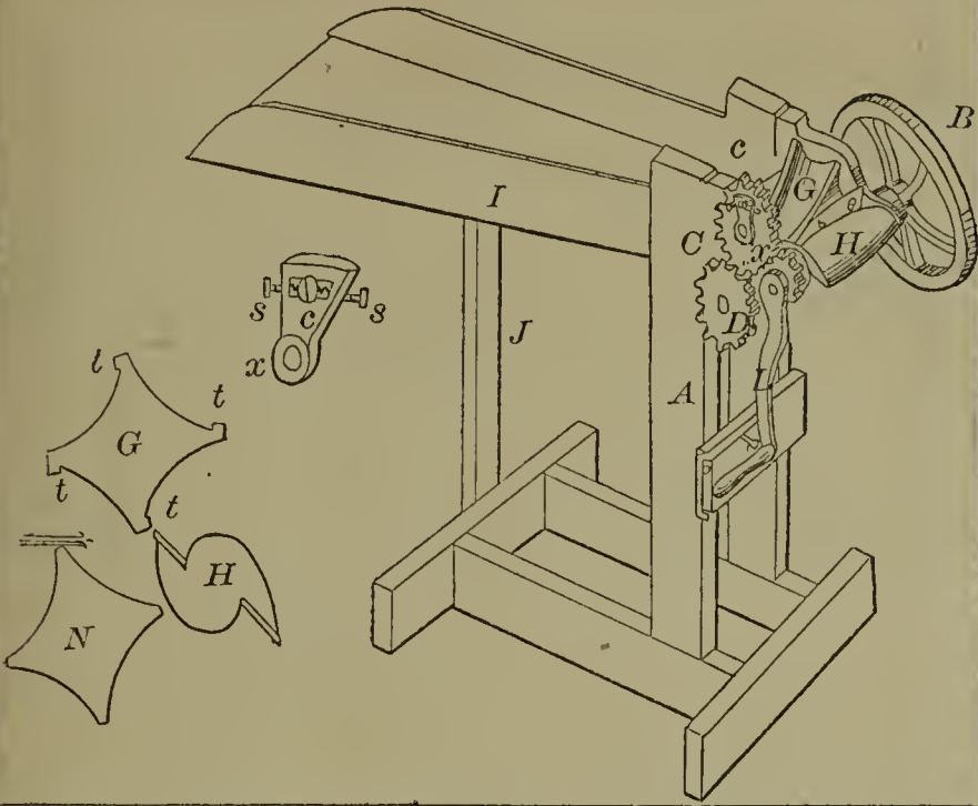
60551—Petveys & Leggett— Gate.
