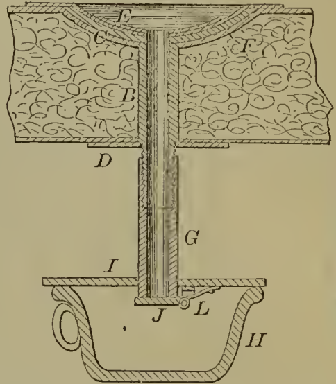
56376—H. Cordes—Invalid Bedstead.
