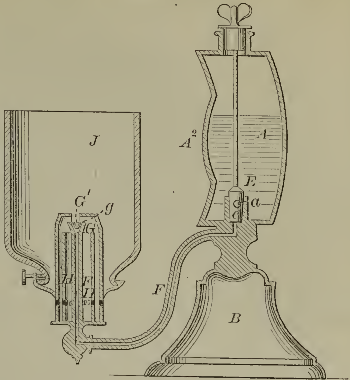
51852—G. W. Mitchell—Lamp.
