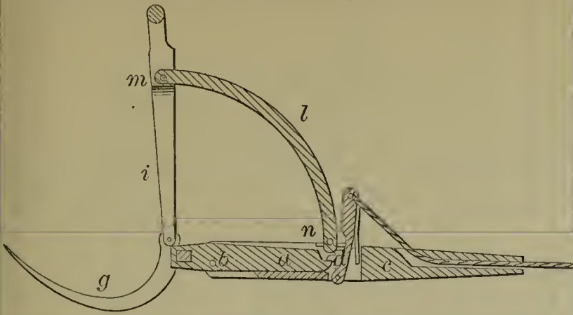
55408—P. A. Wise—Horse Hay Fork.
