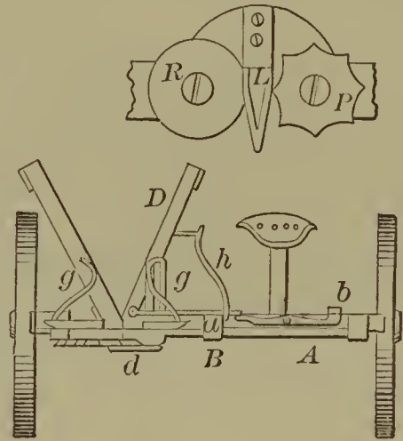
58706—J. F. Winchell— Corn Harvester.
