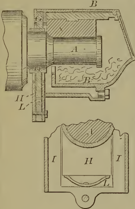
59616—F. Leppens—Axe Box.
