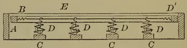
54545—A. Hitchcock— Bed Bottom.
