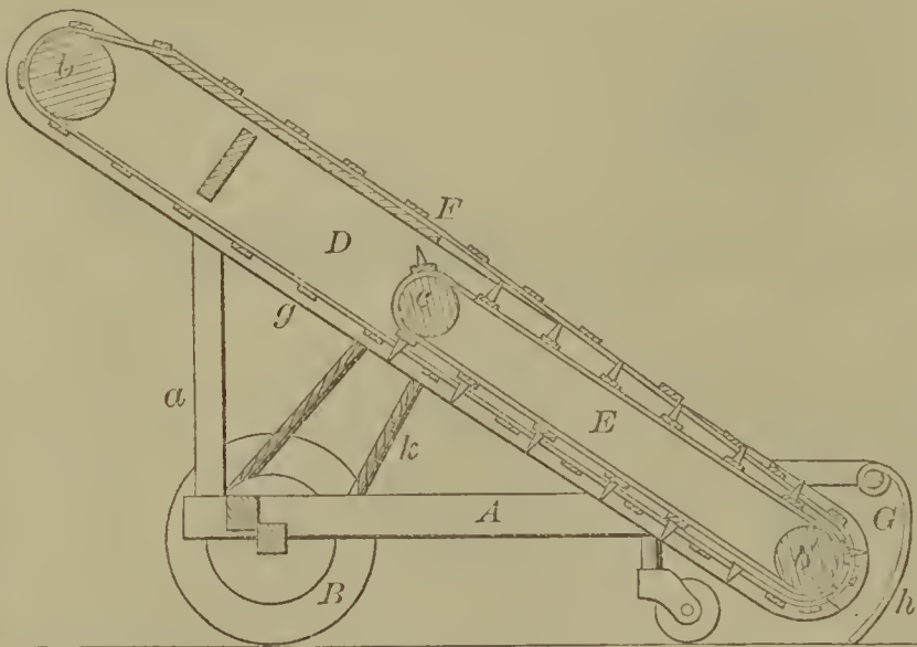
52602—A. Raffel— Hoop Skirt Former.
