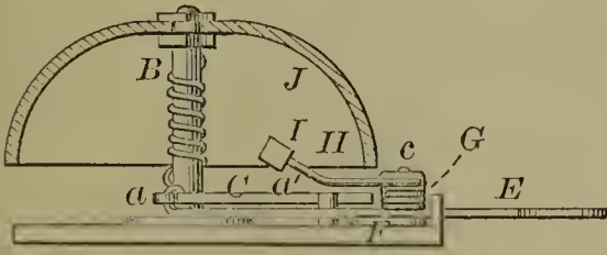
53366—W. H. Watrous— Door Bell.
