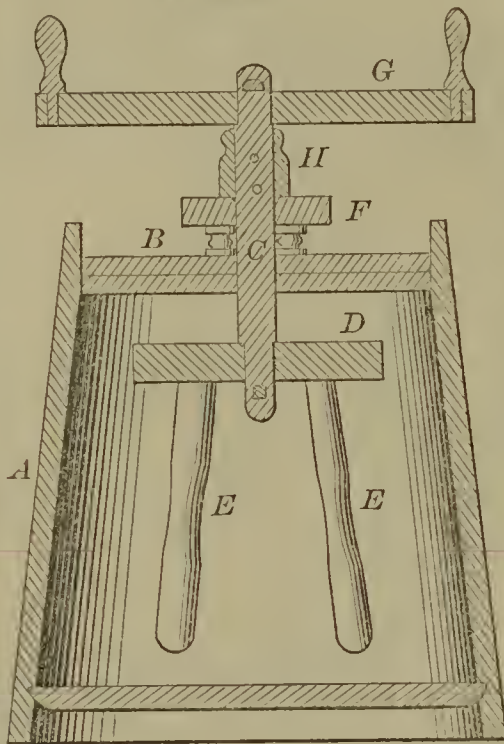
52550—J. & J. Ehart—Washing Machine.
