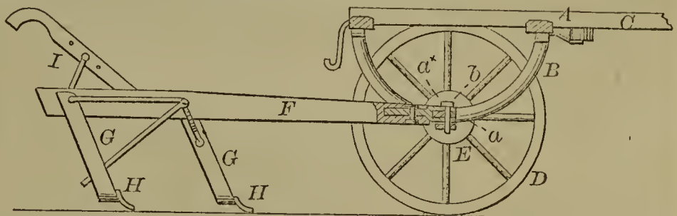
56122—C. W. Taliaferro— Corn Cultivator.
