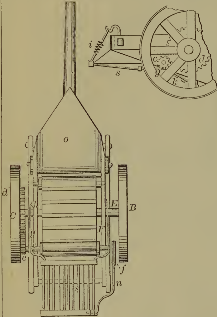
56366—W. F. Caldwell—Potato Digger.
