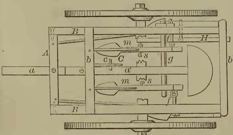
55993—A. M. Black—Cultivator.
