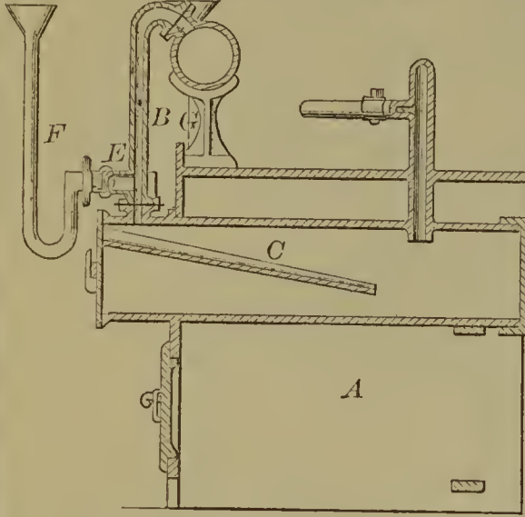
58221—J. H. Connelly—Making Gas.
