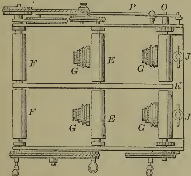
60202—W. & J. Leach— Hand Spinning Machine.
