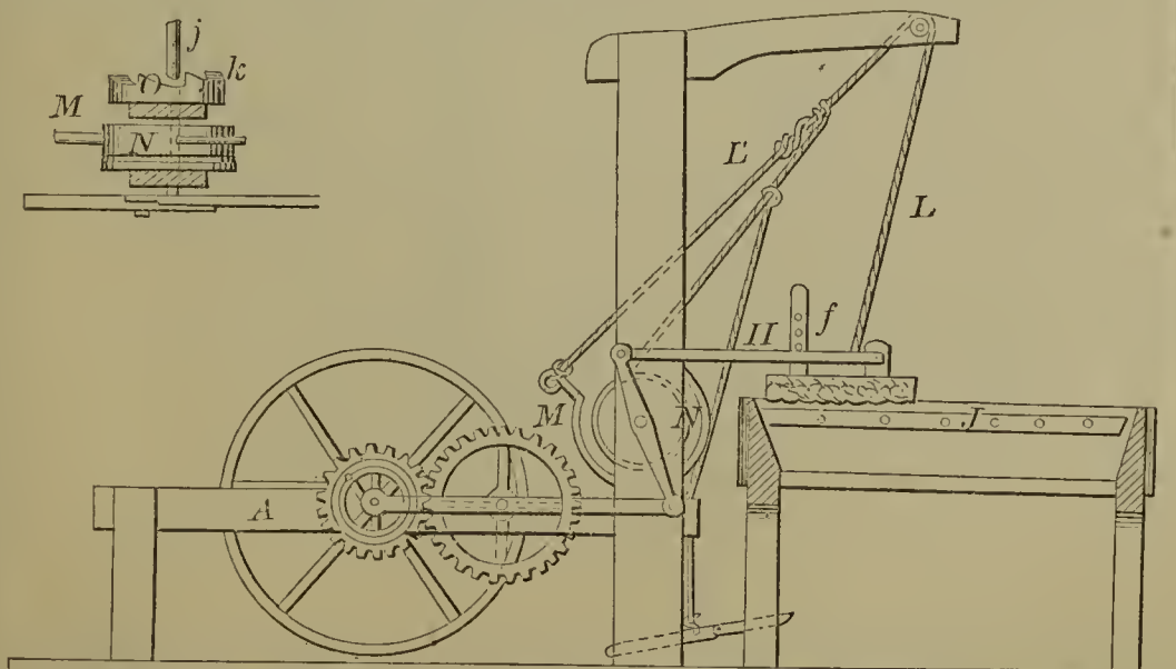
56733—A. L. Drake—Washing Machine.
