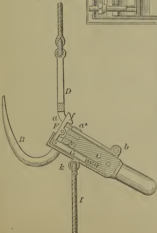
53288—T. Foster—Horse Hay Fork.
