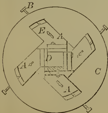
59731—J. Turner— Adjustable Nut Box.
