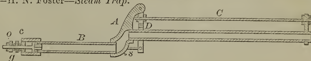
52038—H. N. Foster—Steam Trap.
