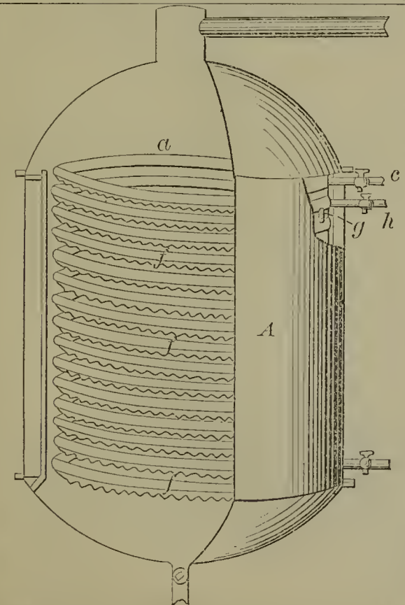
52197—G. R. Percy— Vacuum Pan.
