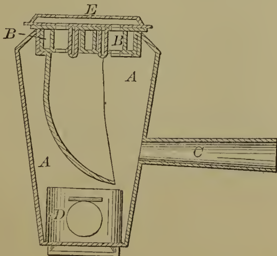
58238—B. Fish— Tuyere.
