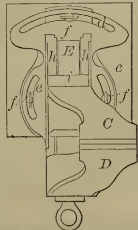
55656—J. S. Hoar— Bench Vise.
