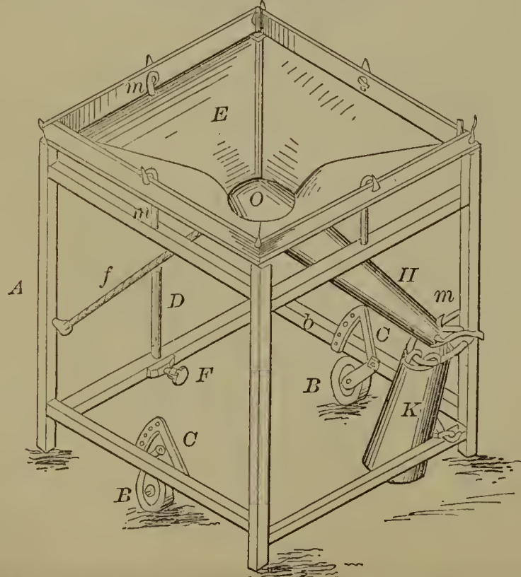
54696—J. A. Daum— Fruit Gatherer.
