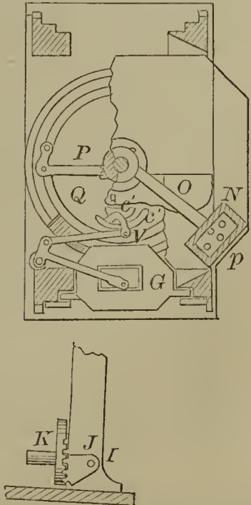
55841—J. S. Elliott— Brick Machine.
