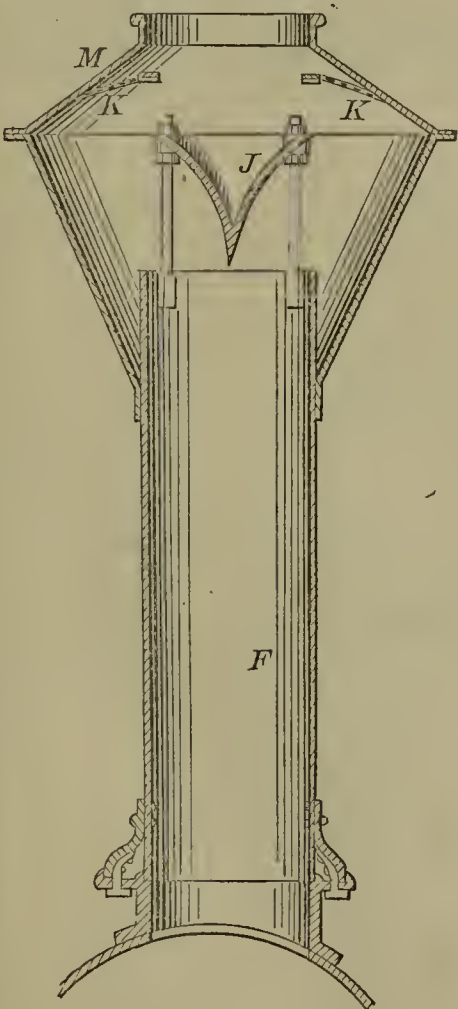
52362—C. F. Jauriet—Spark Arrester.
