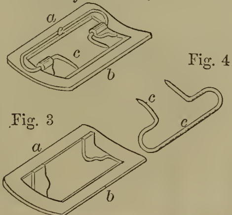
55311—G. R. Kelsey—Buckle.
