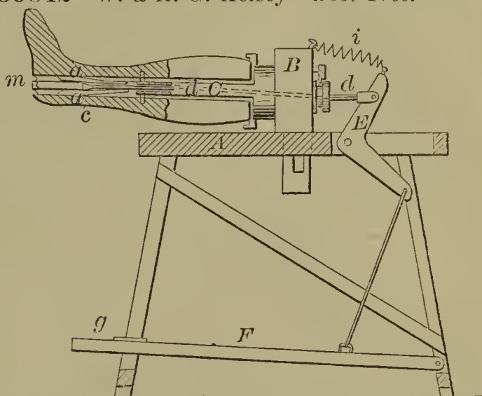
59842—W. & A. G. Kelsey—Boot Tree.
