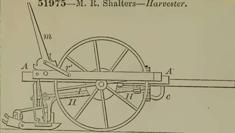
51975—M. R. Shalters—Harvester.
