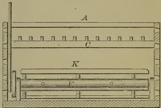
54647—W. La Dew— Vat for Tanning.
