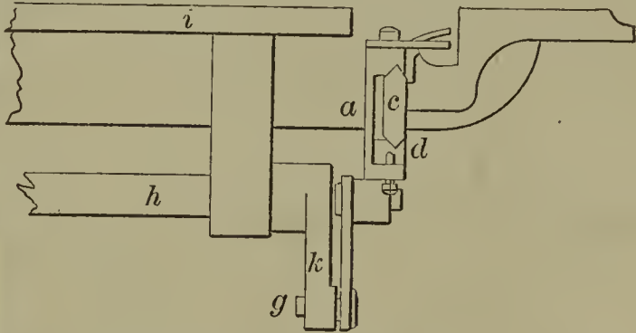
60418—F. A. Pratt—Sewing Machine.
