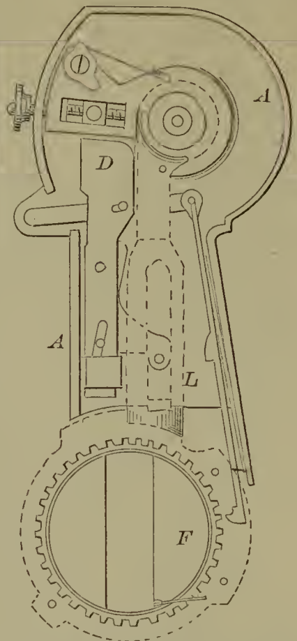
55866—J. A. & H. A. House—Sewing Machine Clamp.
