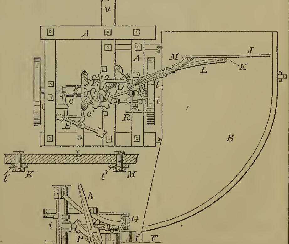
55059—W. J. & R. Case— Harvester Rake.
