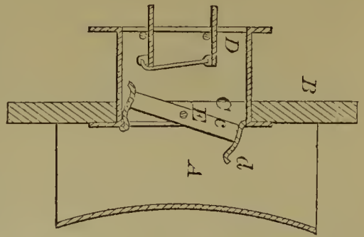
55094—G. Hardy—Car Ventilator.
