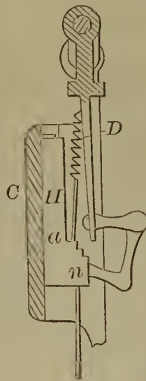
56247—J. Minter—Bolt Heading Machine.
