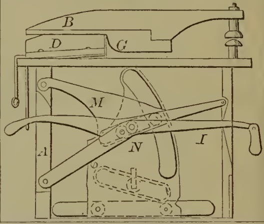
59669—J. N. Smith—Foot Press.
