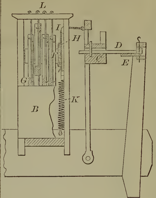
52160—J. S., E. J. & R. Godfrey—Washing Machine.
