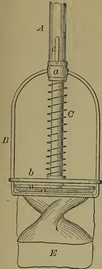
54146—G. H. Hammer— Mop Head.
