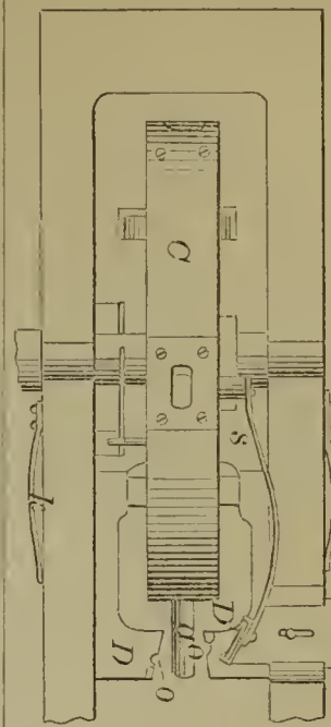
57043—E. L. Keeler— For Bending Chain Links.
