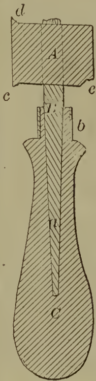
60563—F. M. Schmitt— Sole Edge Finishing Tool.
