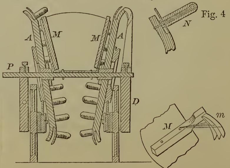
52880—W. E. Prall—For Picking Cotton.
