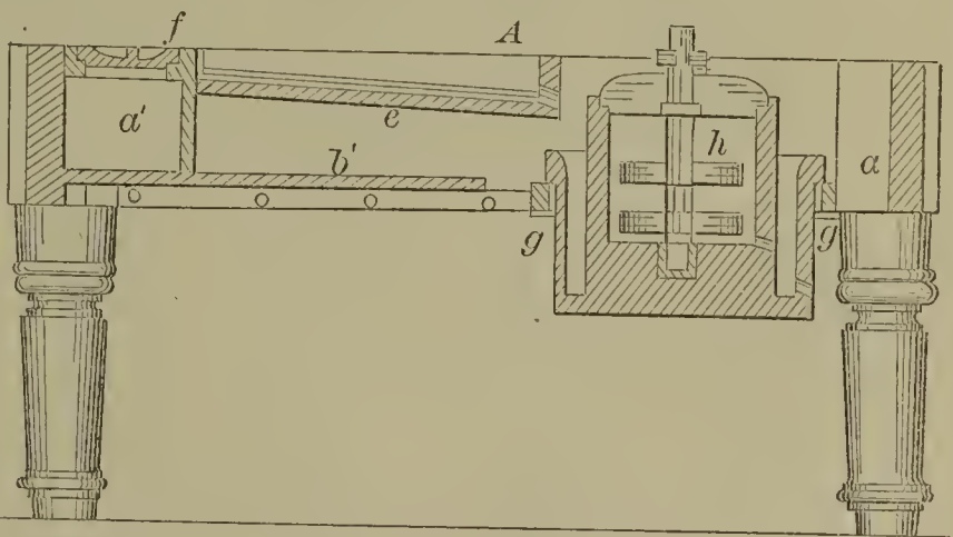
55857—W. H. Hart— Butter Worker.
