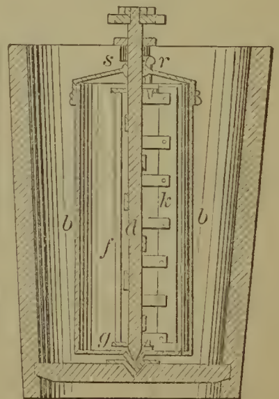
59366—M. G. Crane—Ice Cream Freezer.
