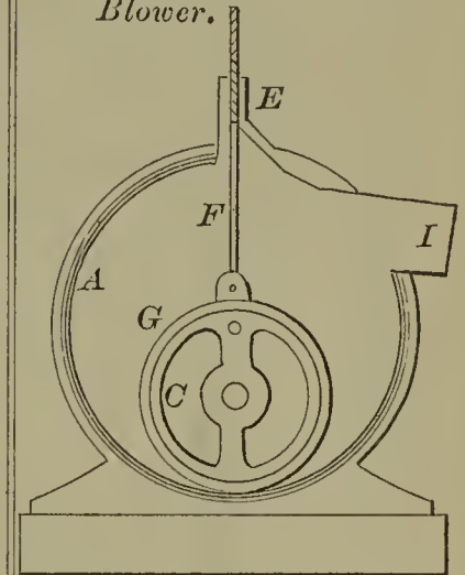
60350—J. A. Evarts—Blower.
