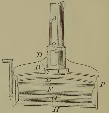
55434—J. G. Wilson—Knitting Machine.
