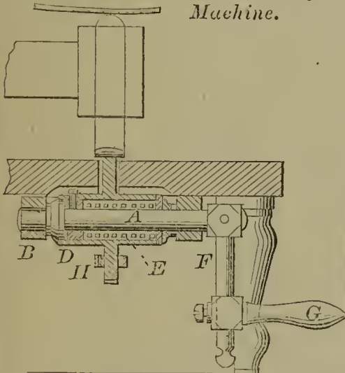
56733—A. L. Drake—Washing Machine.
