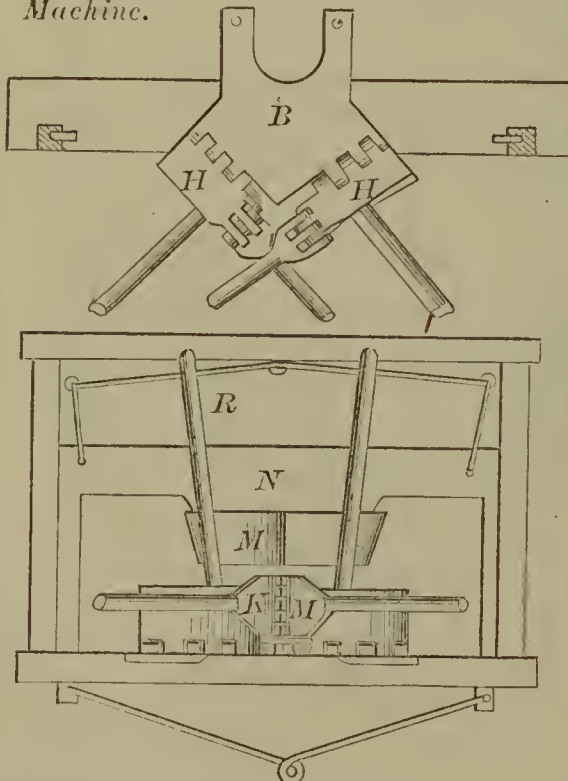
57261—M. S. Sager—Sheet Metal Pan Machine.
