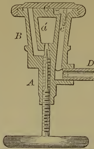
58261—J. S. Hull— Vapor Lamp Burner.
