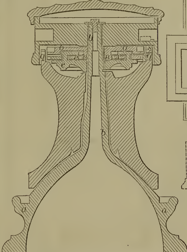
57302—J. Edson—Capstan.
