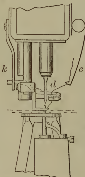
52368—T. K. Reed—Sewing Machine.
