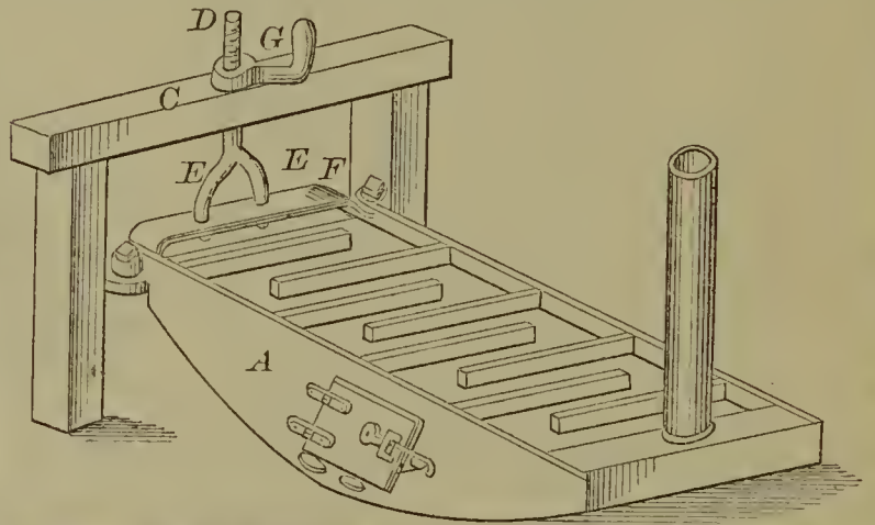
53422—J. A. De Tar—Adjuster for Evaporator.
