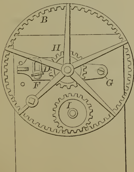
56771—A. E. Mason— Churn.
