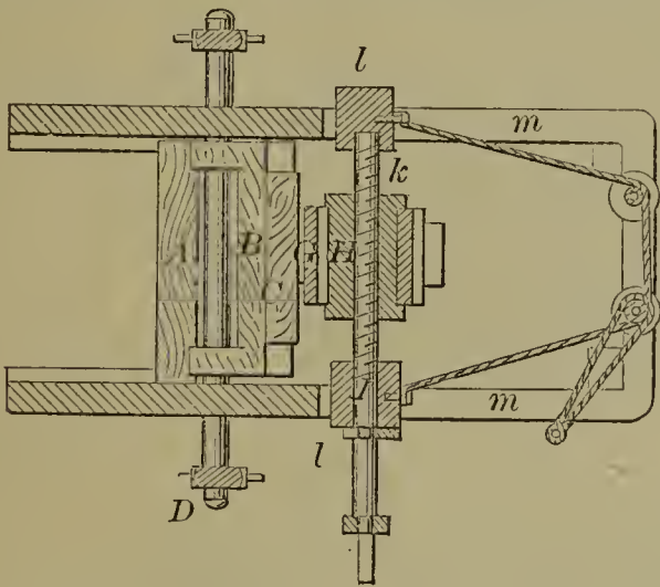
54163—A. J. Homan— Slide Valve.
