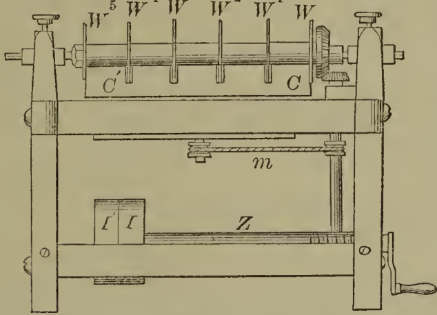
52626—C. Unverzagt— Hand Loom.
