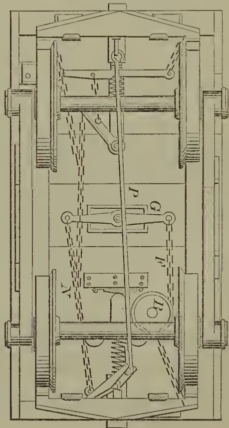
52063—G. F. Lynch— Car Brake.
