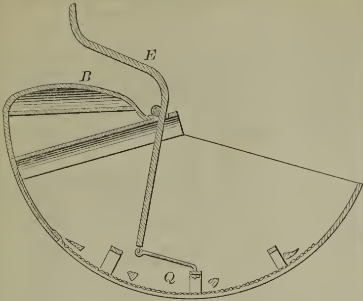
51901—D. T. Robinson— Flour Sifter.
