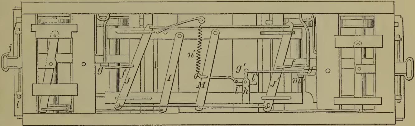
53971—J. W. Gibbs—Car Brake.
