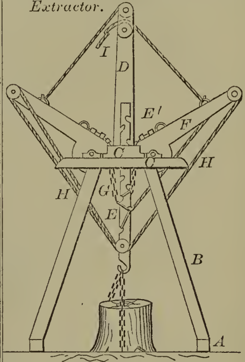
60372—N. M. Healy— Stump Extractor.
