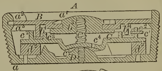
60011—Hufendick & Spangenberg—Bung.
