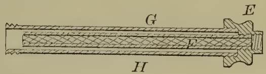
55383—W. H. Smith— Vapor Burner.
