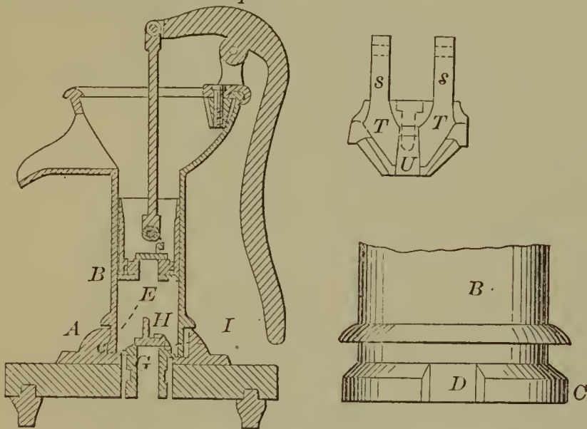
54289—A. Burr— Pump.
