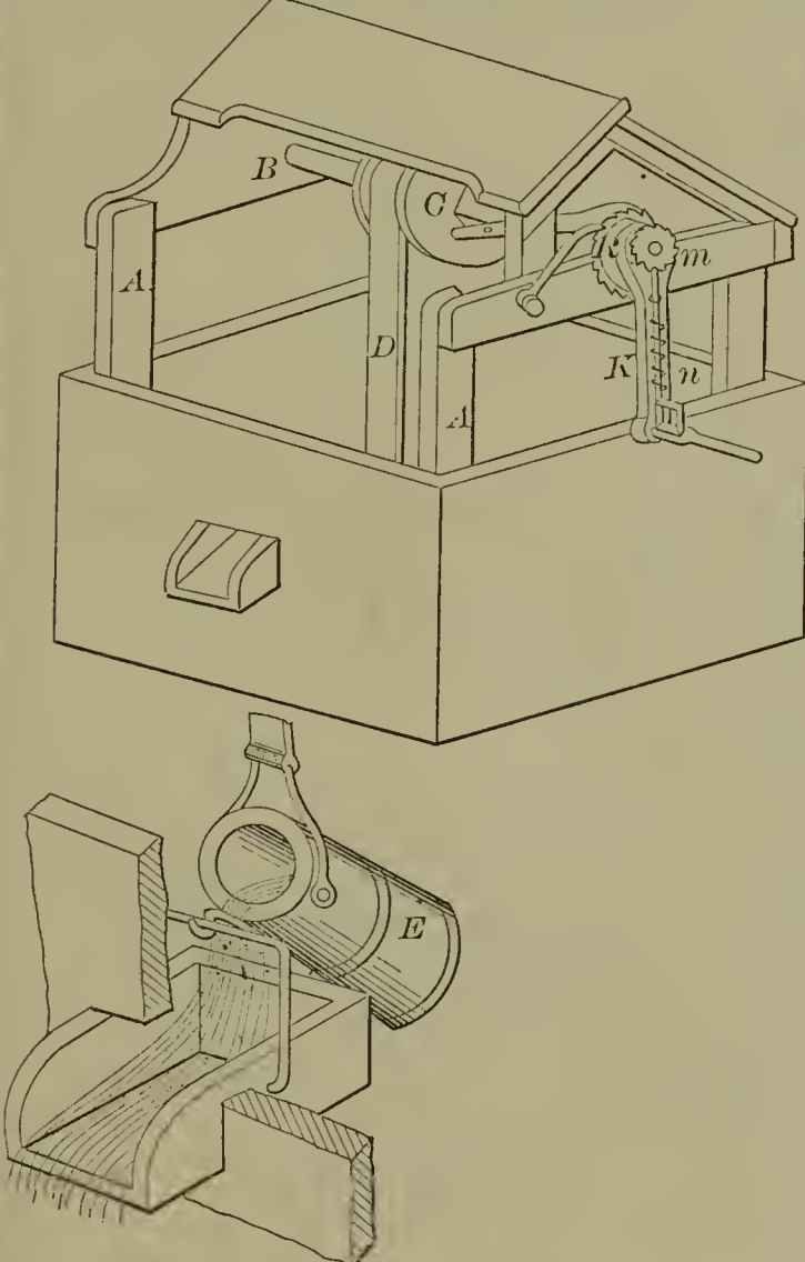
57546—J. E. Moeller— Water Elevator.
