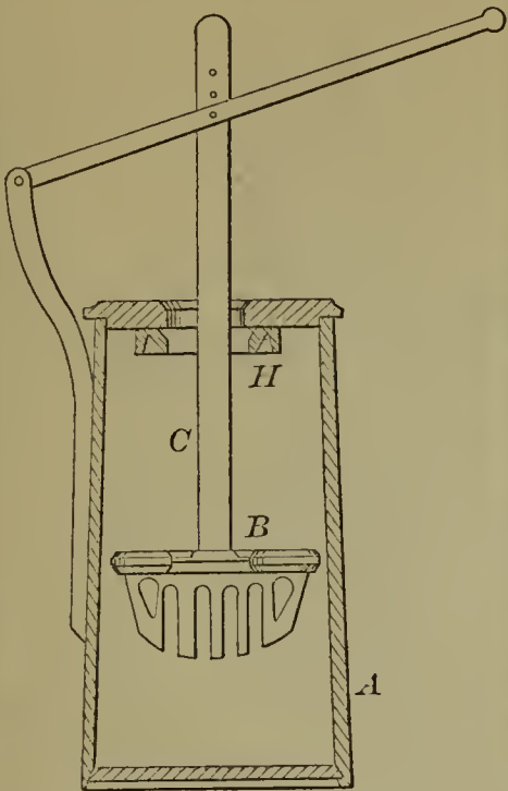
53432—D. A. Fiske—Churn.
