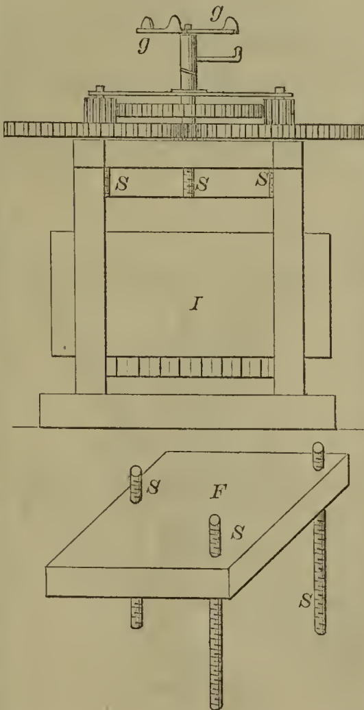
57331—I. H. Johnson— Hay Press.
