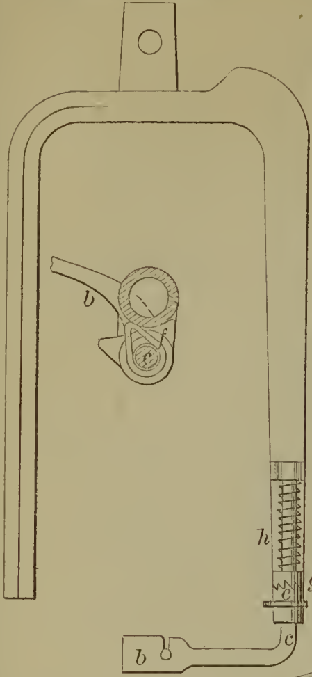
57065—B. A. Bailey— Spinning Flyer.
