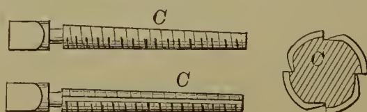
54096—B. F. Bee— Screw Tap.
