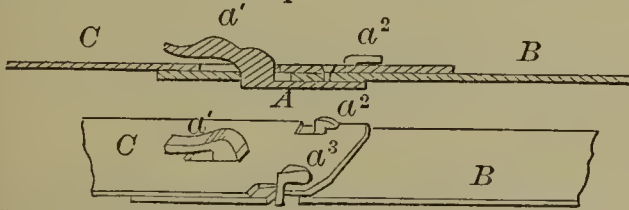
54675—J. Booth— Cotton Bale Tie.
