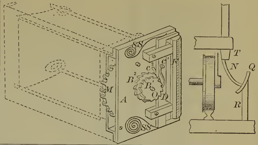
53604—J. T. Greenwood, Sr.—Washing Machine.
