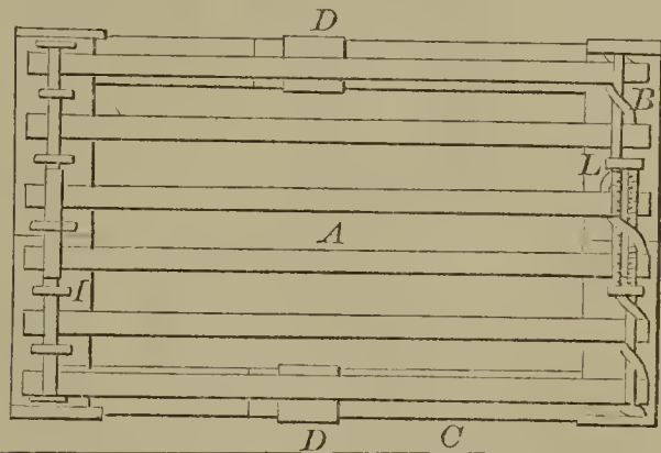
52663—S. R. Boure—Sled.
