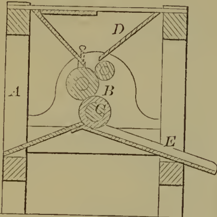
59700—J. H. Williams— Cider Mill.
