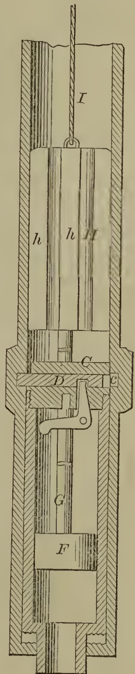
52364—T. Mayhew—Pump.
