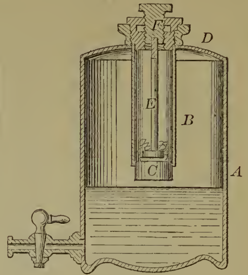
59847—J. R. Laurent—For Extinguishing Fires.
