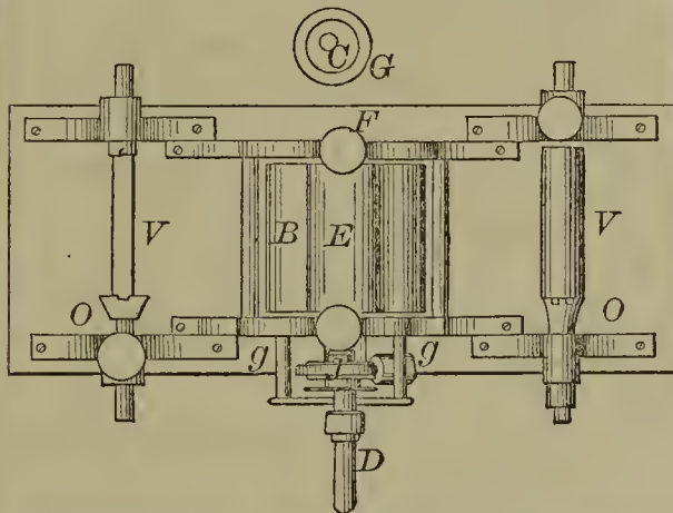
52383—Burnett & Vandevort— Wind Wheel.
