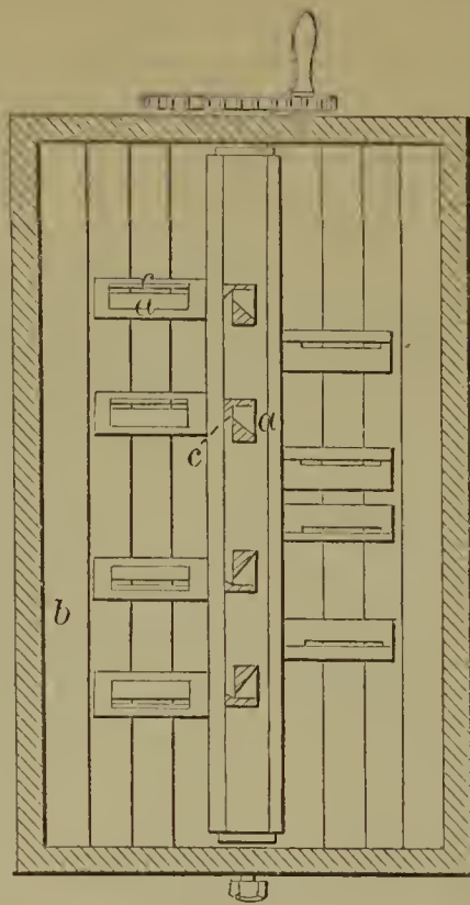
57730—J. D. Kellogg Churn.
