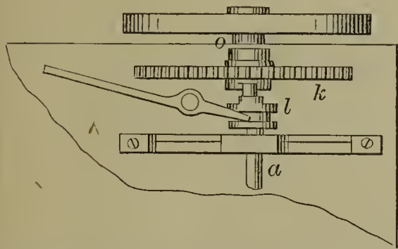
54222—J. M. Seymour— For Tenoning Blind Slats.
