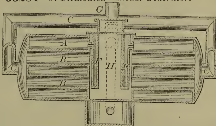
53285—A. Fischer—Beer Cooler, &c.
