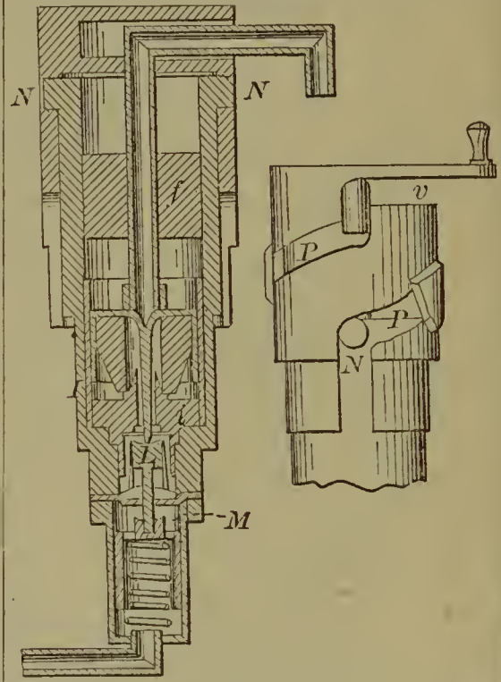
59670—J. N. Smith—Hydrant.
