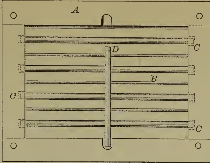
52856—E. A. Jeffery— Coal Hod.
