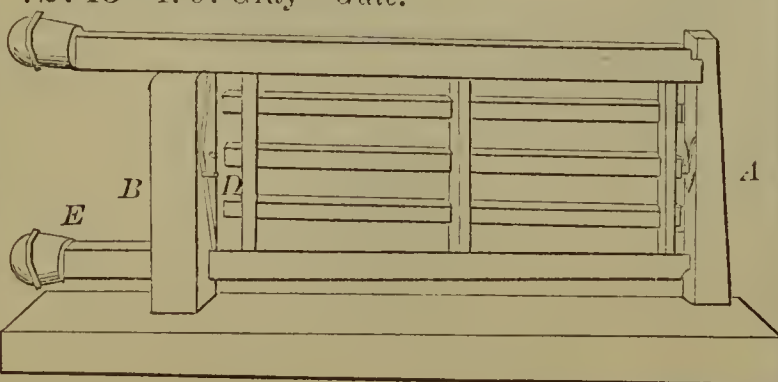
72743—I. J. Gray—Gate.
