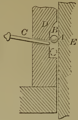
58322—W. S. Van Hoeseon— Sash Supporter.
