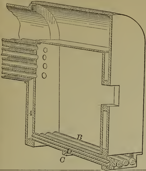
59130—W. A. L. Kirk—Water Grate.
