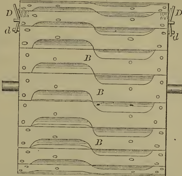
57078—Blinn & Hewitt— Flooring Clamp.
