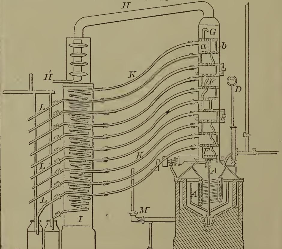
60477—J. A. Coffey—Distilling Apparatus.
