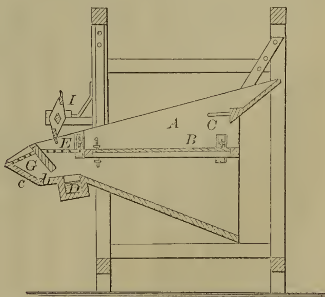
56194—J. F. Dunham—Grain Separator.
