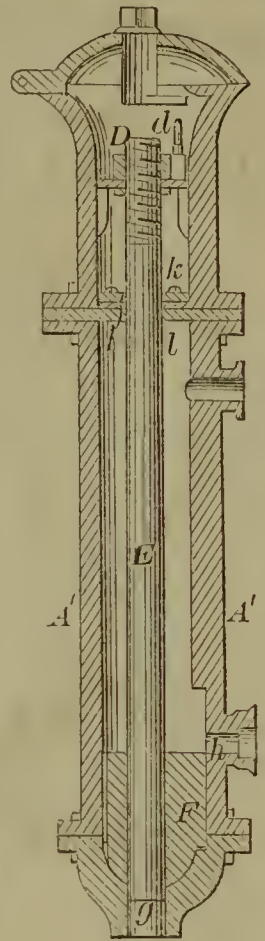
57449—J. M. Ward— Hydrant.
