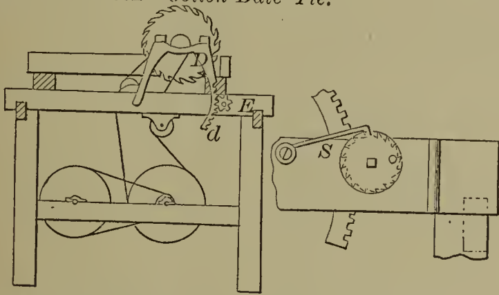
54675—J. Booth— Cotton Bale Tie.
