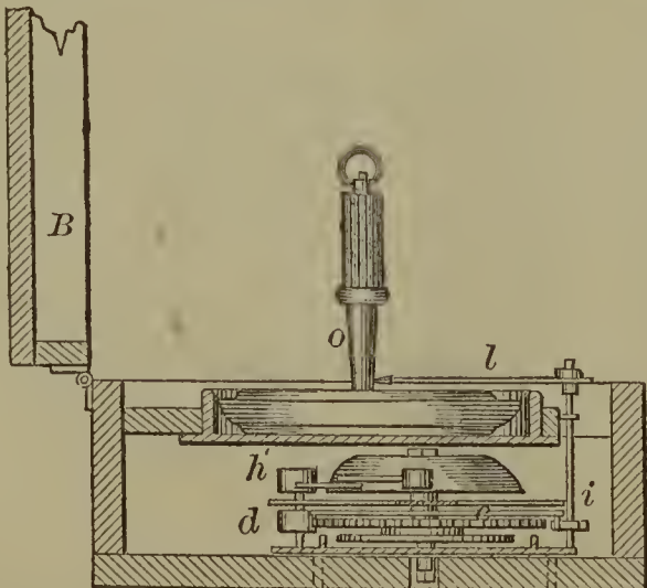
58058—J. E. Buerk—Alarm Clock.
