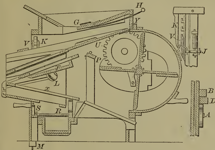
52841—J. W. Free— Grain Separator.
