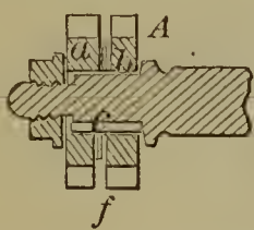
53496—J. F. Smith— Milling Tool.
