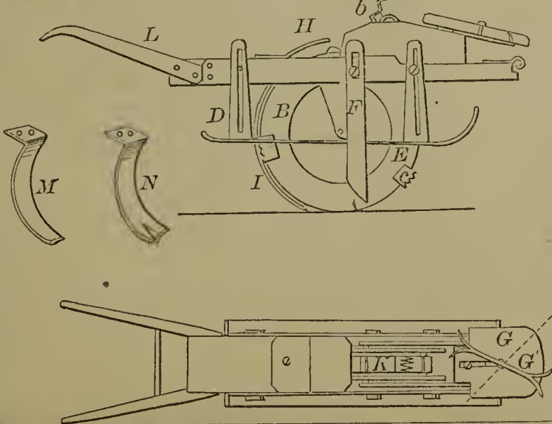
58334--W. H. Burridge--Potato Digger.
