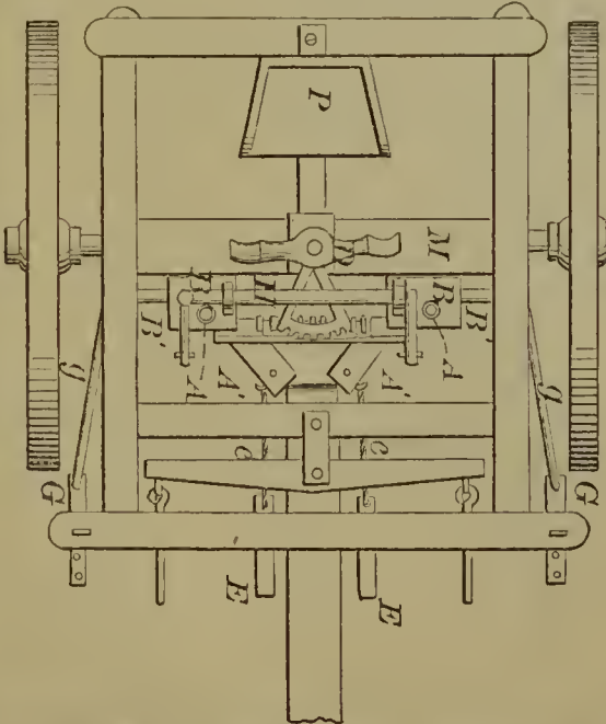
54669—Barr & Cox— Cultivator.
