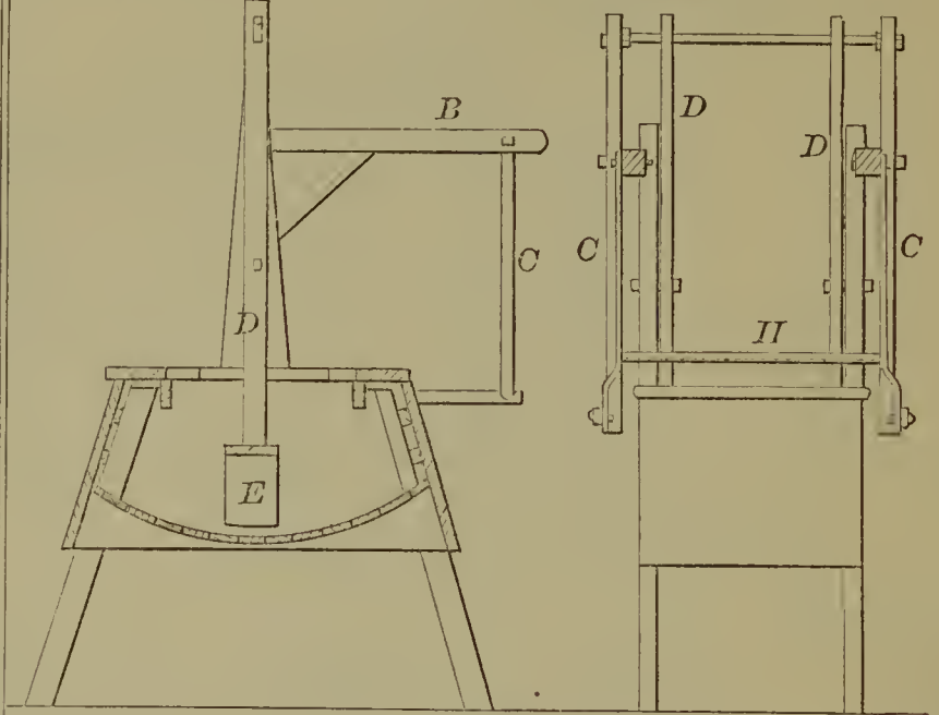
56911—Durant & Grissirn—Washing Machine.
