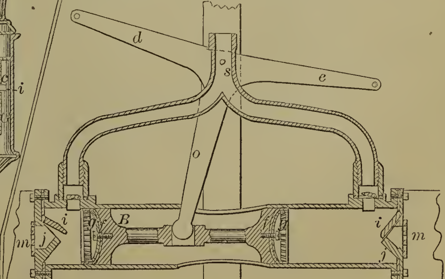
58360—L. Drescher— Pump.
