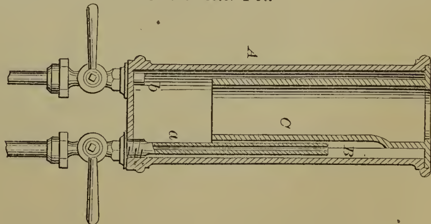
54073—G. Sewell—Saline Meter Pot.
