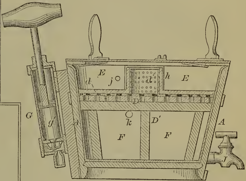
53606—J. P. Gruber—Filtering Apparatus.
