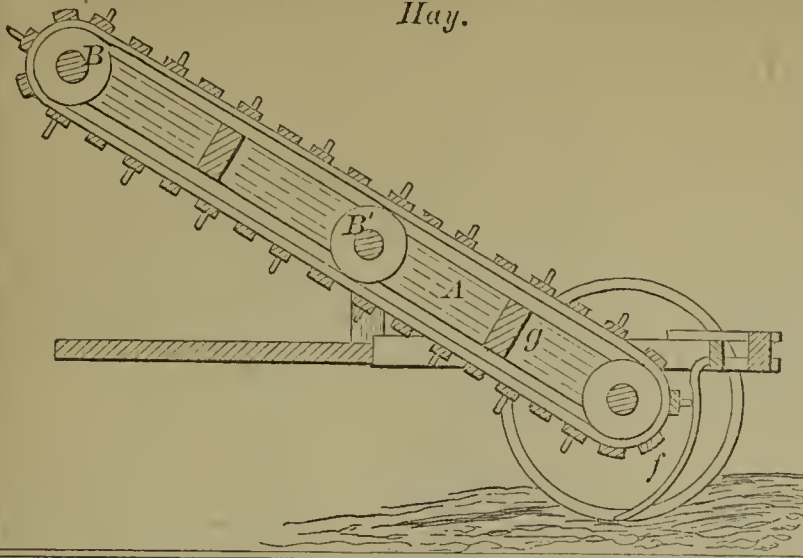
59117—J. H. Yager—Manual Power.
