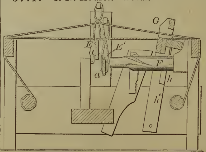
57717—I. N. Hodson—Loom.
