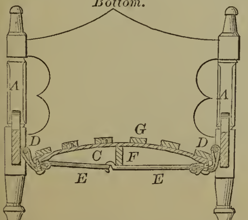
58994—G. B. & C. B. Davis— Bed Bottom.
