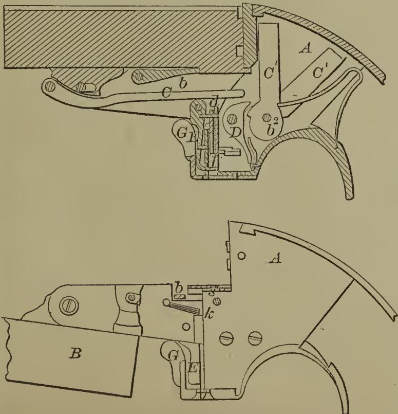
58064—W. J. Christy—Fire Arm.
