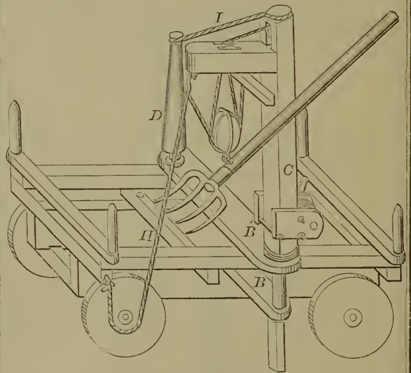
56924—A. Fuller— Hay Loader.
