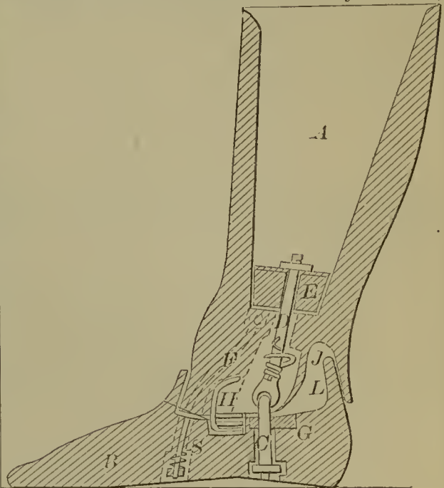
56983—R. H. Nicholas— Artificial Leg.
