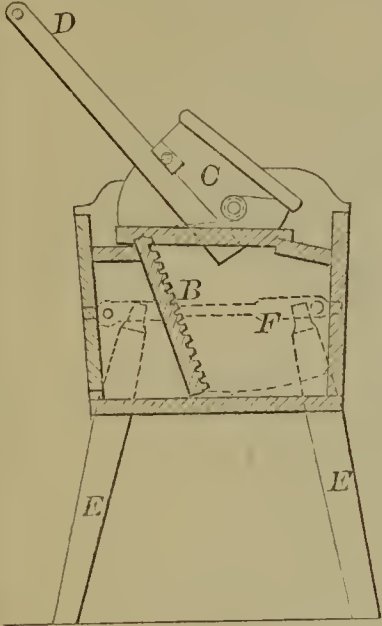
56910—W. M., E. P. & E. Doty—Washing Machine.
