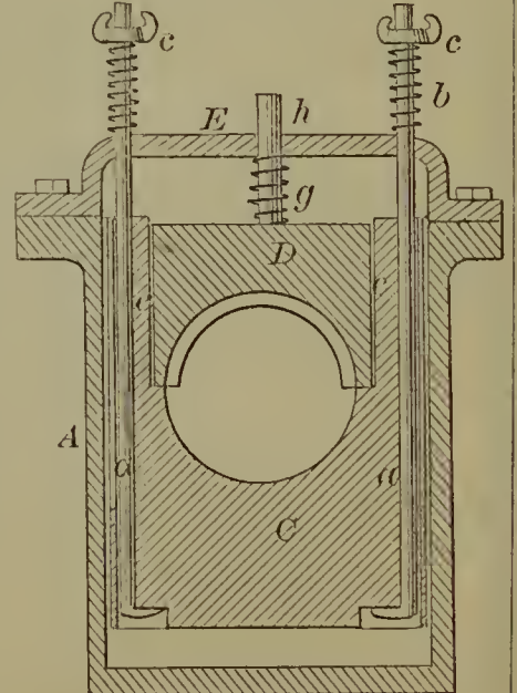
53588—D. H. Dotterer— Axle Box.
