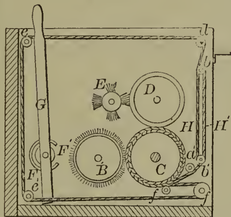
57527—J. K. Lowe—Bronzing Machine.
