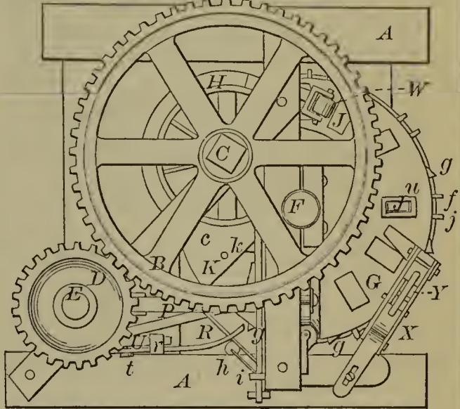
53223—J. Hotchkiss—Brick Machine.
