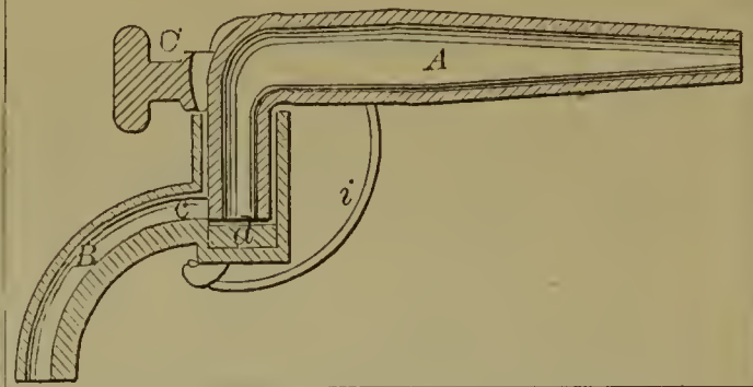
59670—J. N. Smith—Hydrant.
