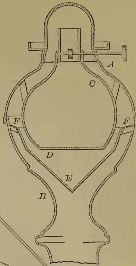
55075—M. B. Dyott—Lamp.
