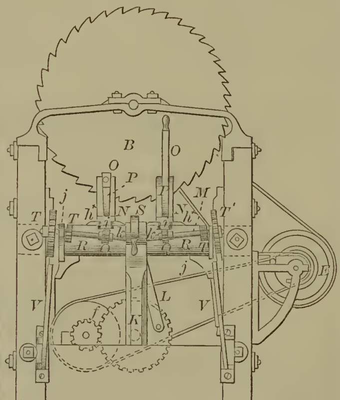
52507—T. H. Cox— Shingle Mill.
