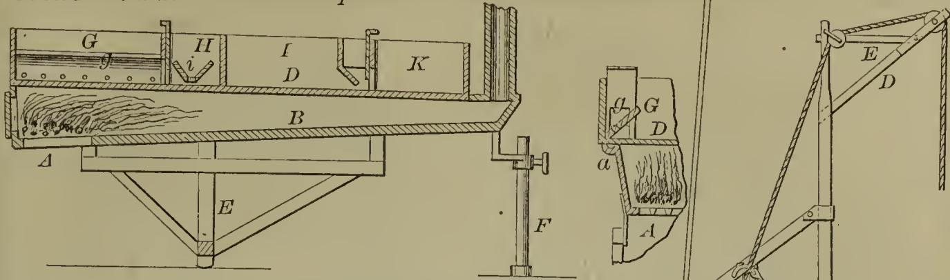
57527—J. K. Lowe—Bronzing Machine.
