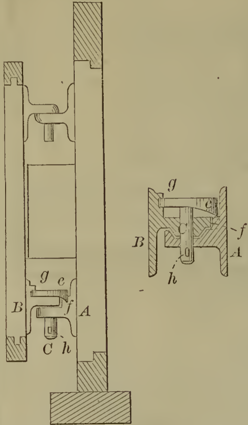
55646—A. B. Glover— Bolt Heading Machine.
