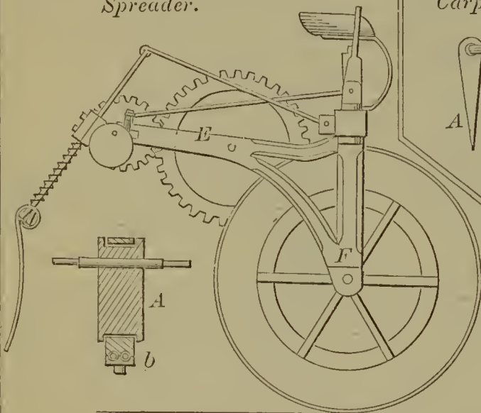
59001—C. R. Frink— Hay Spreader.
