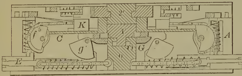
56793—H. Pearce—Quartz Mill.
