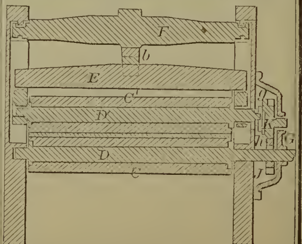
59041—J. S. Lash—Clothes Wringer.
