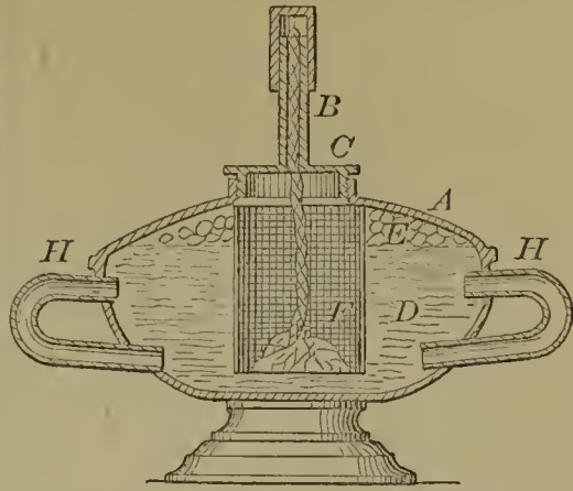
58481—K. Riedel— Lamp.
