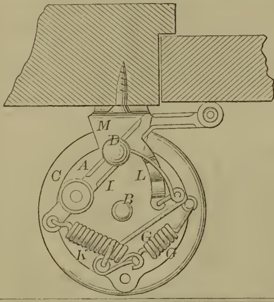
56264—J. B. Pratt— Knife Sharpener.
