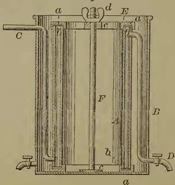
54708—A. Fischer— Liquid Cooler.
