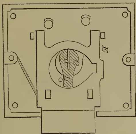
53941—T. A. Auferlin— Lock.
