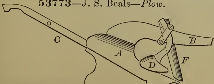
53773—J. S. Beals— Plow.
