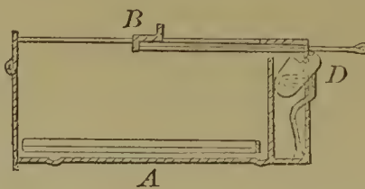
58540—T. B. De Forrest— Hoop Skirt Clasp.
