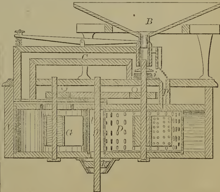
57001—A. & G. Smith— Smut Machine.
