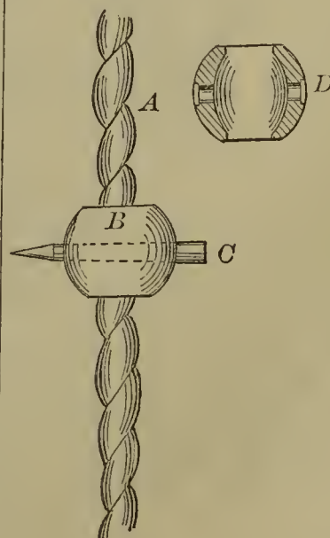
55506—O. B. Latham— Rope Guard.
