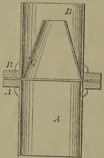
60378—G. G. Hunt— Steam Valve.
