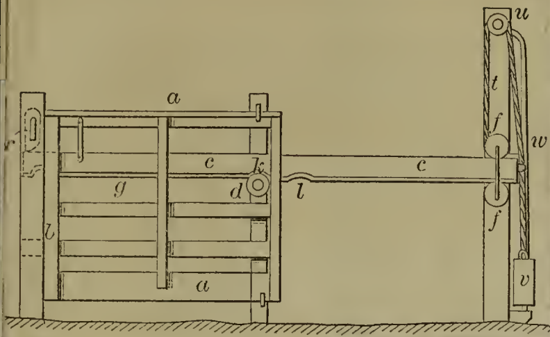
56039—J. H. Graves—Gate.
