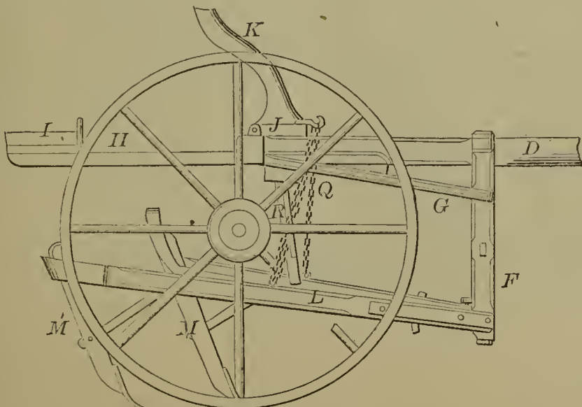
59012—J. B. Herman— Cultivator.
