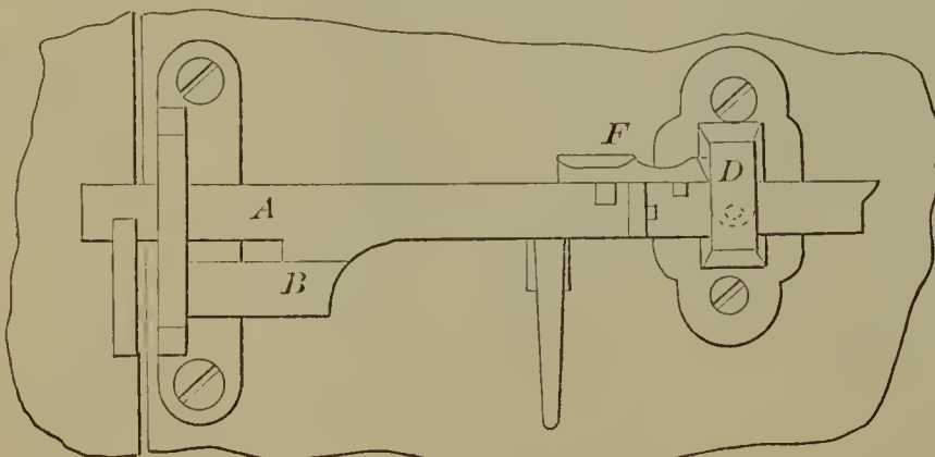
53585—H. L. De Zeng— Door Latch.
