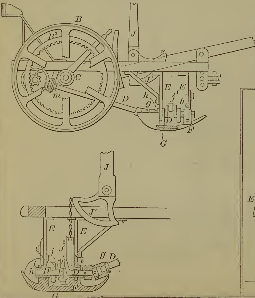
54372—E. M. Krum—Harvester.
