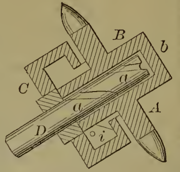
55035—T. H. Arnold— Horse Hay Fork.
