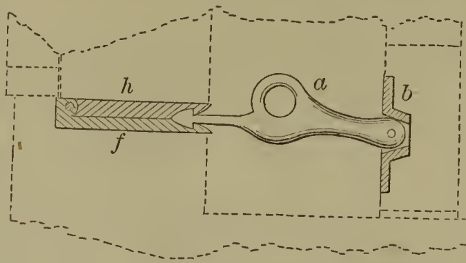
52443—H. L. Parker—Brad Awl Handle.
