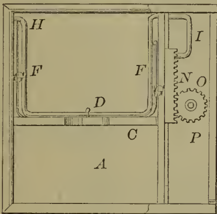
59287—Sterrett & Farrell— Letter Box File.
