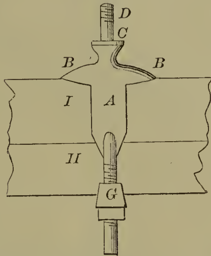
59642—J. Phelps—Carriage King Bolt.
