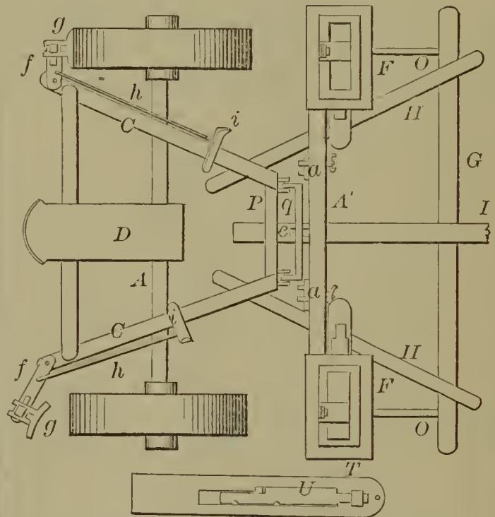
59285—T. G. Springer— Wagon Brake.
