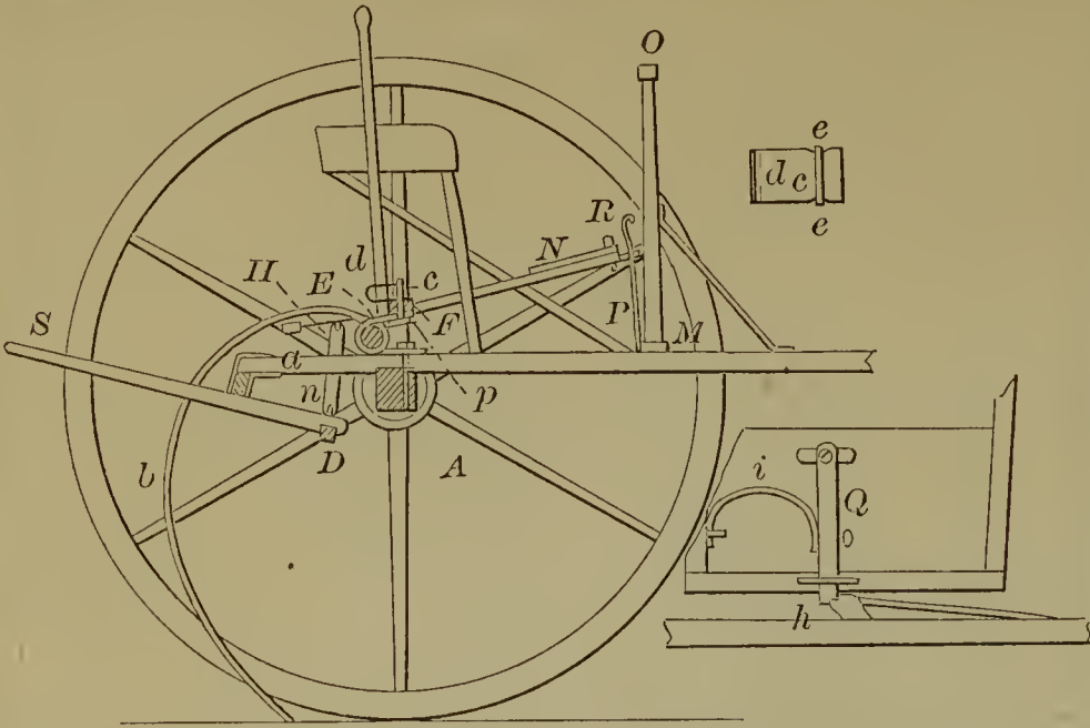
54151—H. R. Hawkins—Horse Rake.
