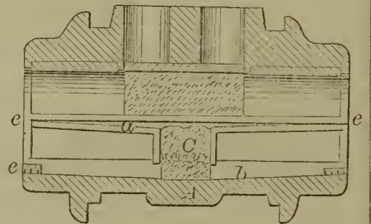
57343—E. F. Leight— Journal Box.
