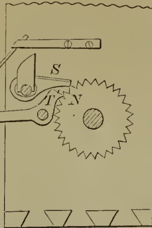
54647—W. La Dew— Vat for Tanning.
