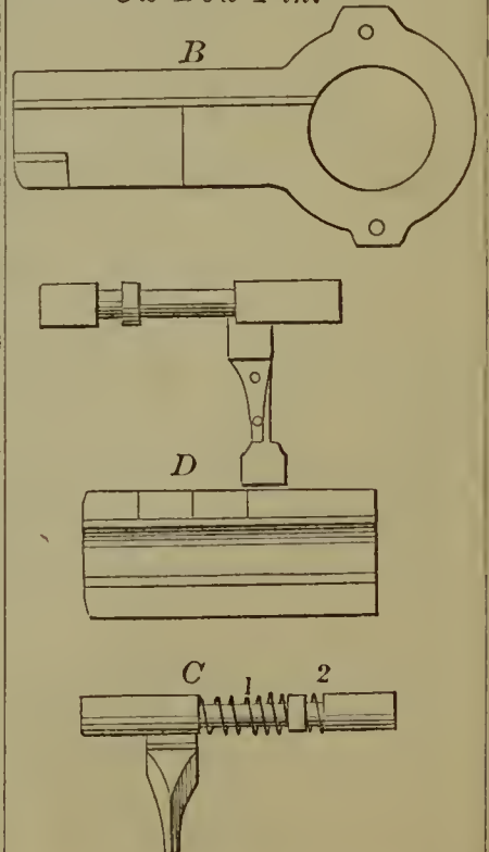
52923—E. S. Woodford—Ox Bow Pin.
