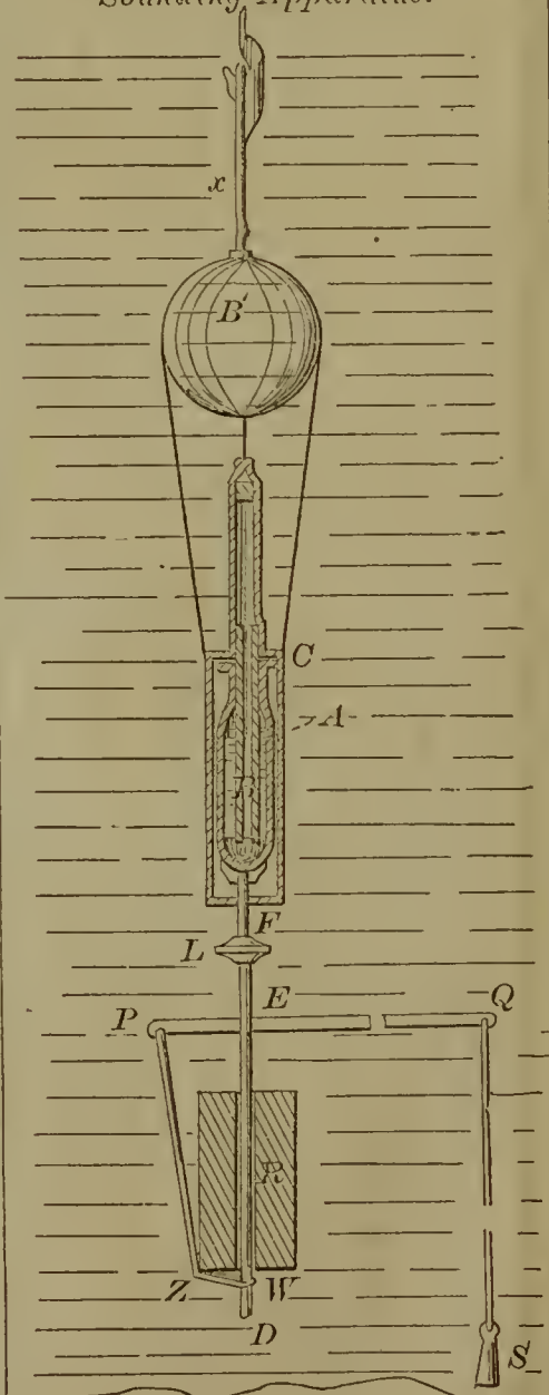
56436—S. E. & G. L. Morse— Sounding Apparatus.
