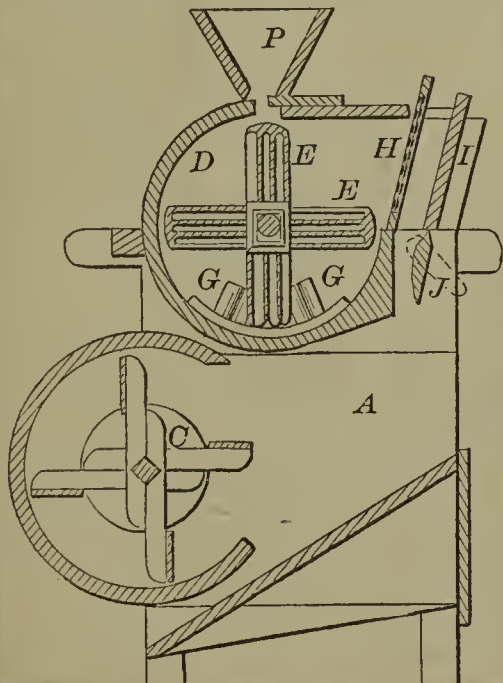
60385—B. Kemp—Homing Mill.
