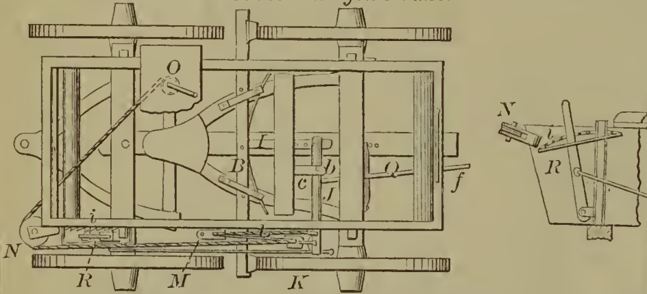
59831—E. R. Gard— Brick Machine.
