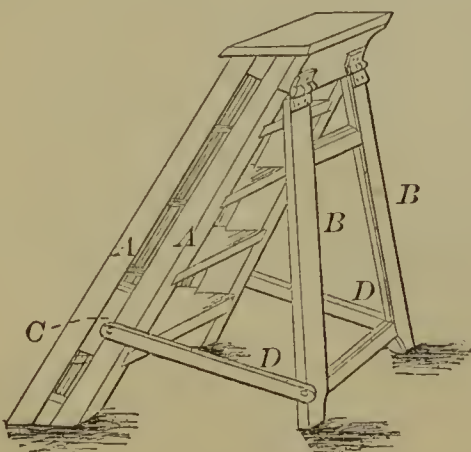
54387—A. Moore, Jr.— Step Ladder.
