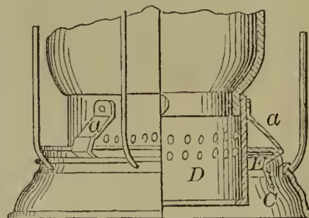
56567—E. N. Jenkins— Lantern.
