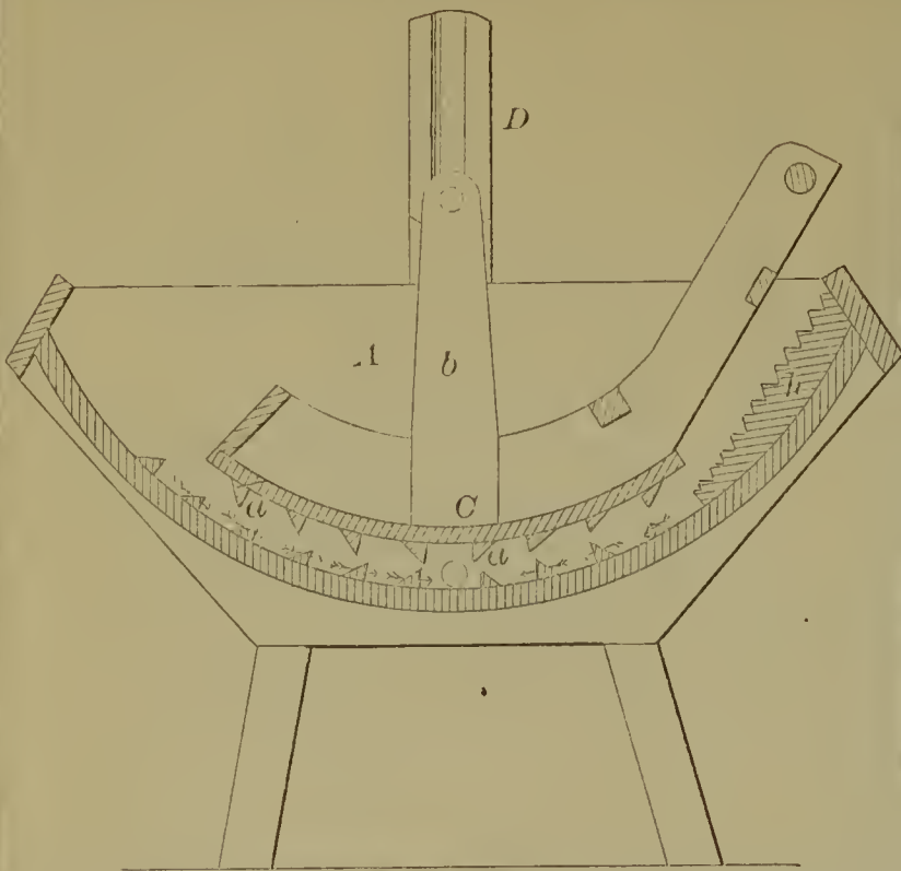
59477—W. C. Taggart— Washing Machine.
