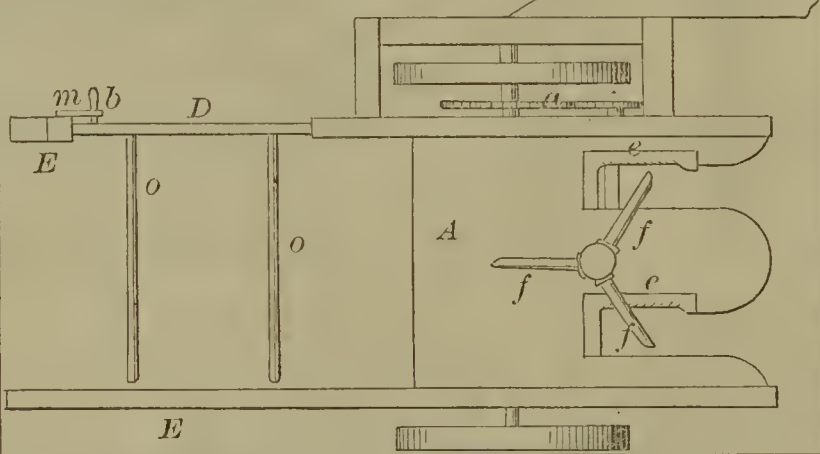
56237—A. J. & H. Linebarger—Grain Separator.
