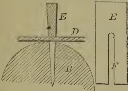
59072—T. B. Raymond— Rafting Pin.
