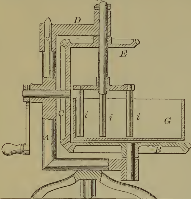
56382—J. Davis—Egg Beater.
