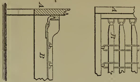
58679—R. S. Sanborn—Bed Bottom.
