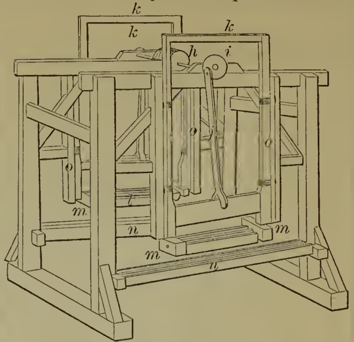
52821—G. M. Campbell—Hemp Brake.
