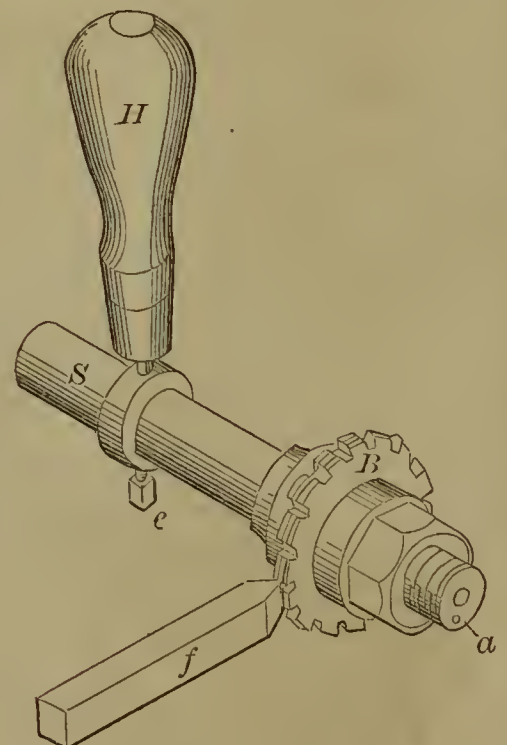
56495—L. F. Grant— Gear Cutter
