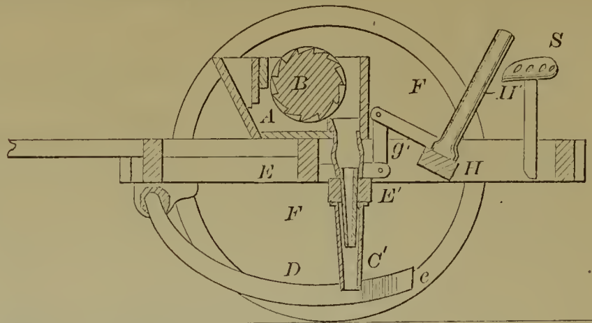
54992—J. Wootton— Flying Machine.
