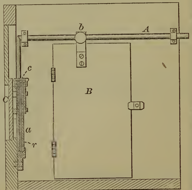
52999—W. O. Hills—Burglar Alarm.
