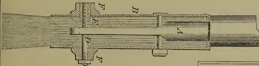
55766—O. S. Pettit—Water Closet.
