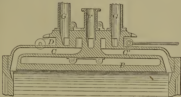
58699—J. H. Wait— Balance Slide Valve.
