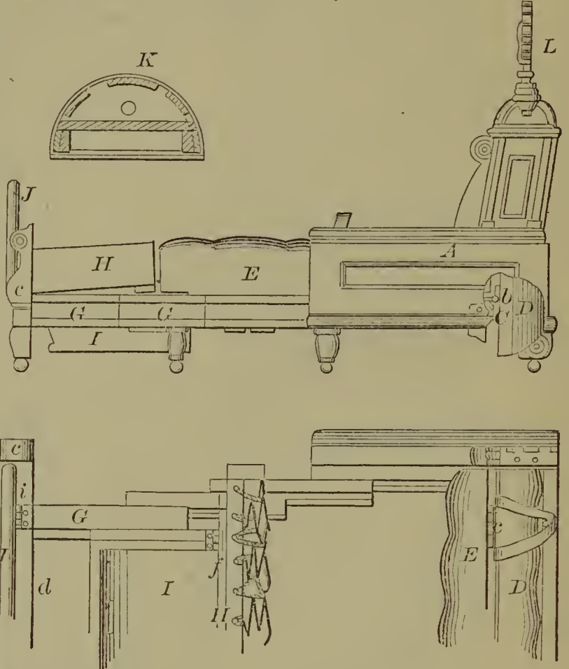
54592—J. F. C. Pickhardt—Sofa Bedstead.
