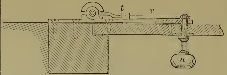
53389—J. W. Allen— Hinge.
