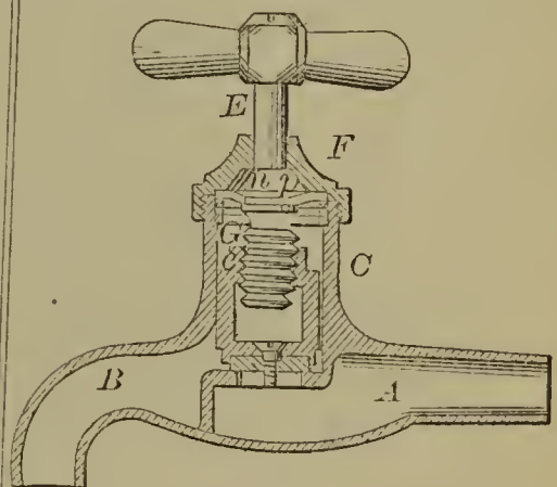
59122—W. S. Cooper—Faucet.
