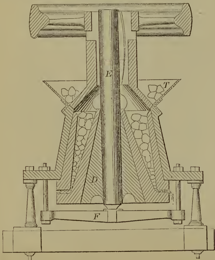
56793—H. Pearce—Quartz Mill.
