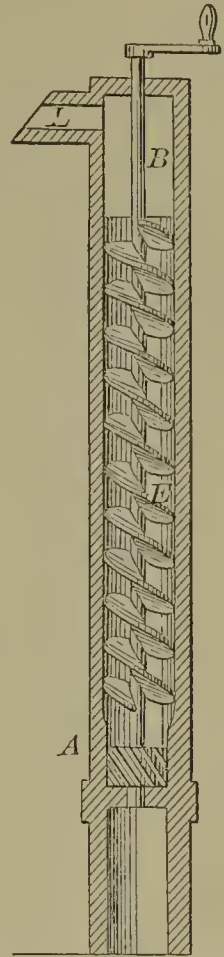
60147—H. D. Dann— Seeding Machine.
