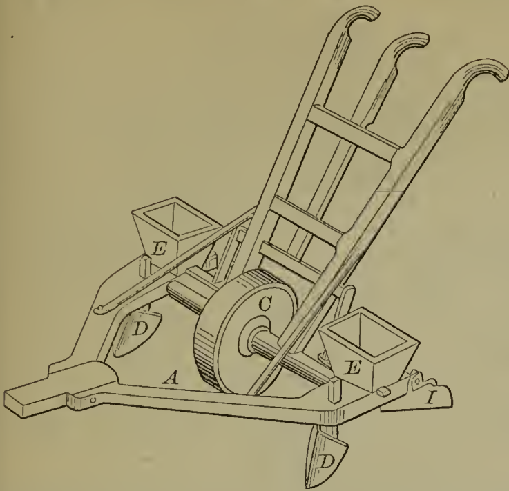
53635—J. N. Lane—Seed Planter.
