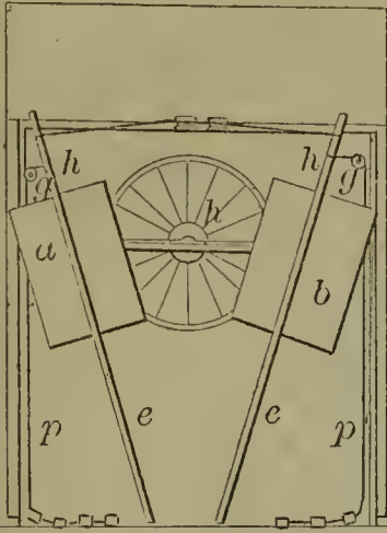
57131—J. H. Heyser— Wind Mill.
