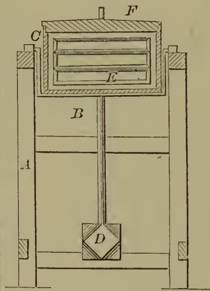
59637—J. D. Parrot— Churn.
