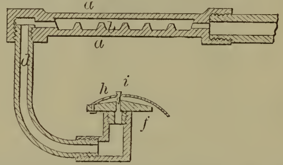
57502—M. E. Hanson—Gas Generator.
