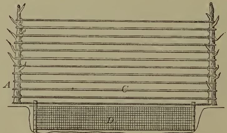
59953—A. Brear—For Trapping Wild Fowl.
