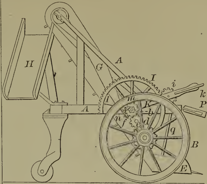
60025—J. H. Marshall—Ditching Machine.
