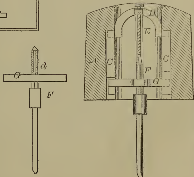
54486—J. W. Baldwin— Grinding Mill.
