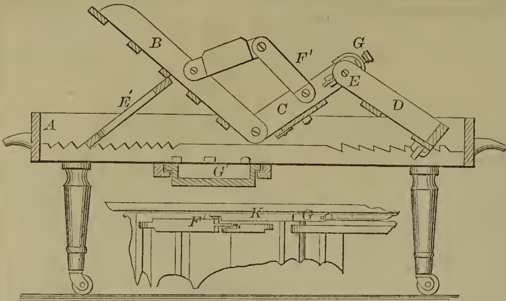
56211—W. A. Guyer—Invalid Bedstead.
