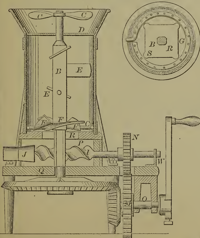
55018—J. H. Rae—Peat Machine.
