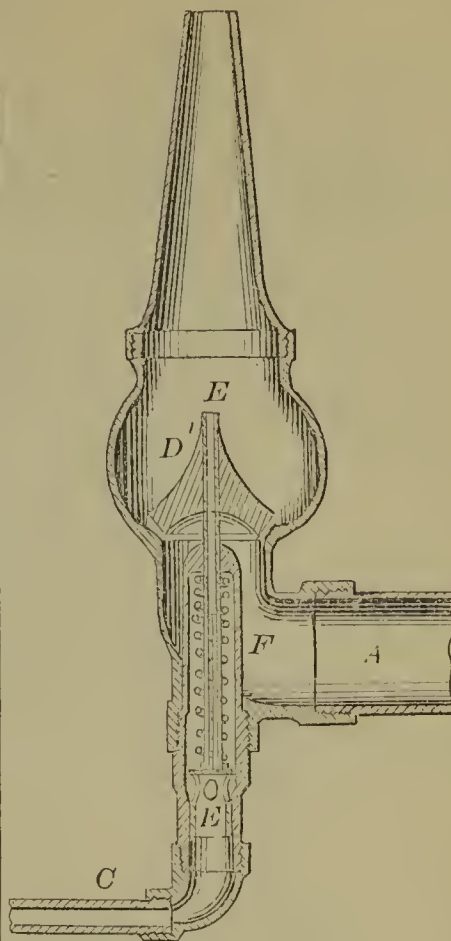
59602—P. C. Heinz— Injector.
