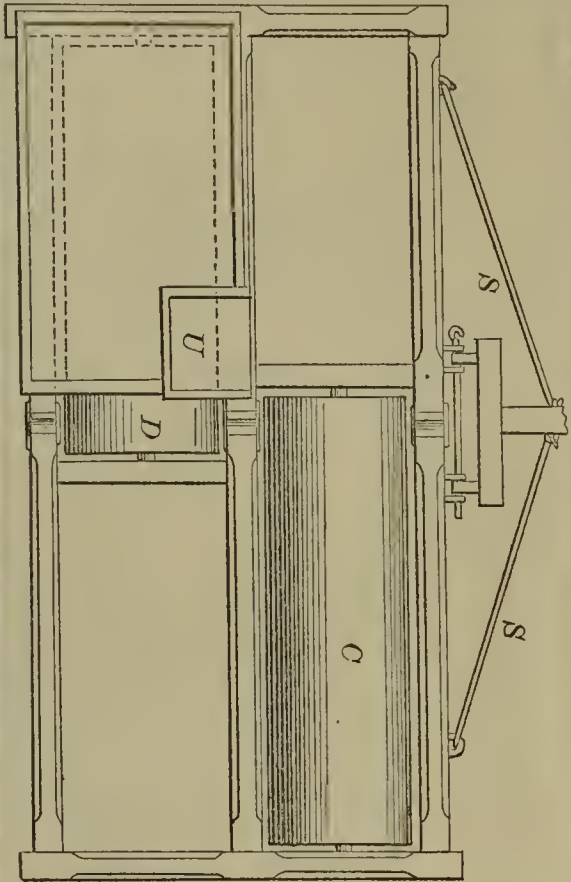
54425—A. S. Skiff— Lead Roller.
