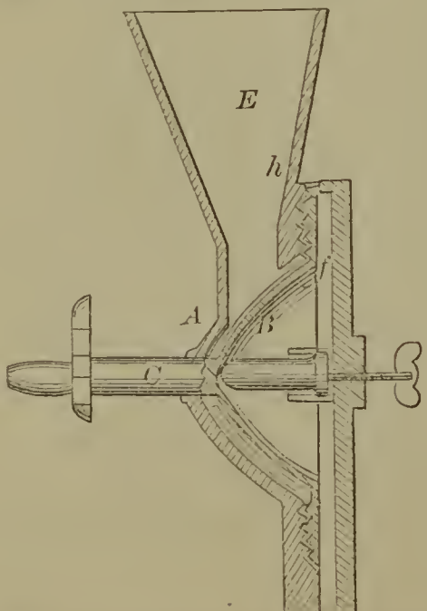
58946—J. G. Lane—Coffee Mill.
