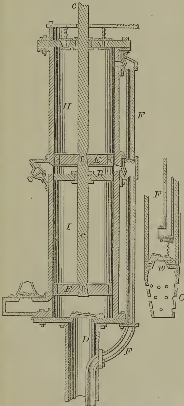
52019—J. A. Bloom— Deep Well Pump.
