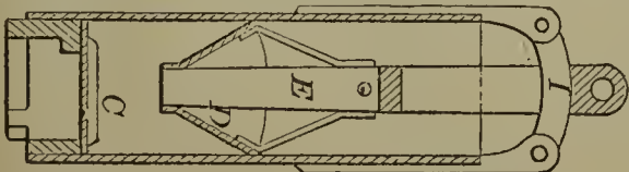
58579—J. Benson— Sand Pump.
