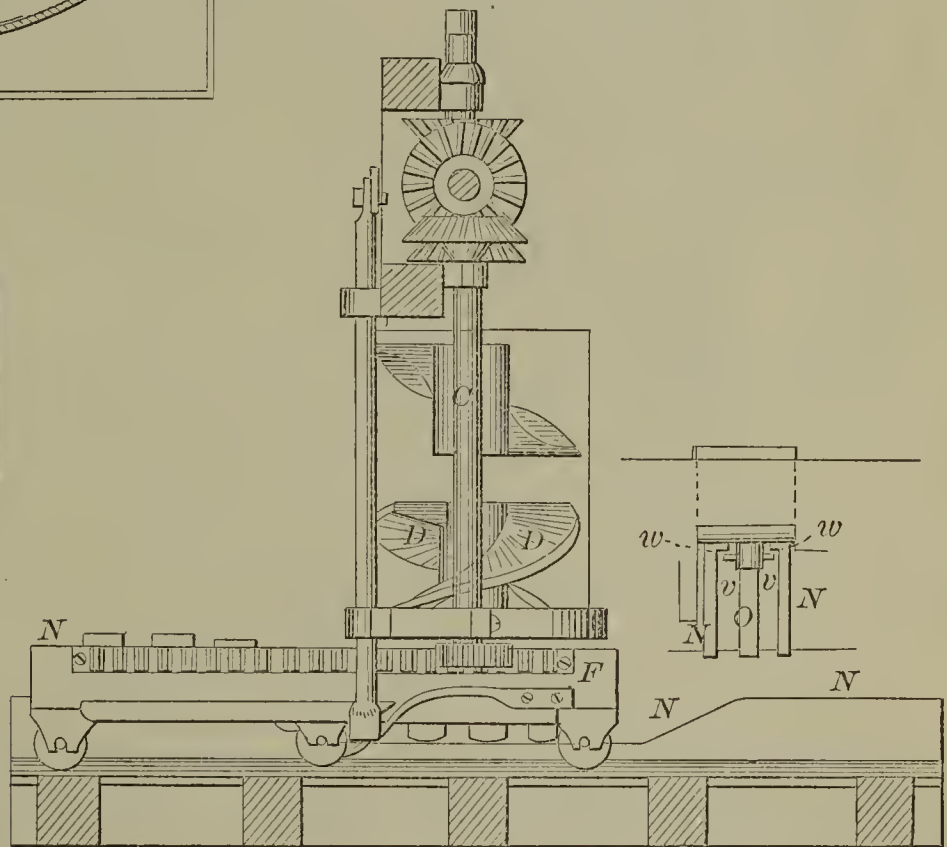
52156—E. R. Gard—Brick Machine.
