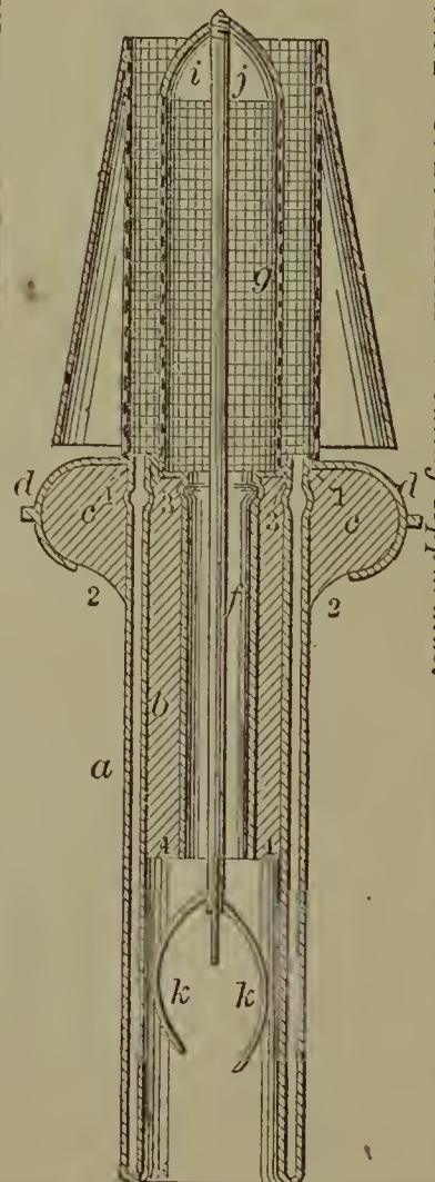
60224—O. F. Morrill—Heating Apparatus.
