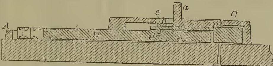
57249—J. Decker— Slide Bolt.
