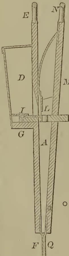
55850—W. Gilbert—Hand Corn Planter.
