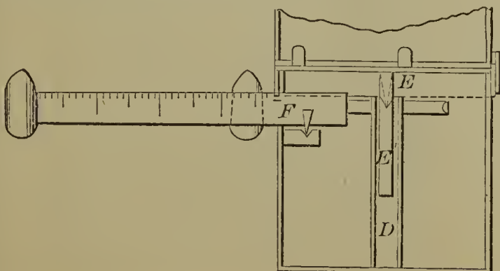
59213—H. Haak—Grain Gauge.
