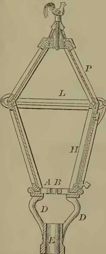
60377—A. R. & E. A. Hunt— Street Lantern.
