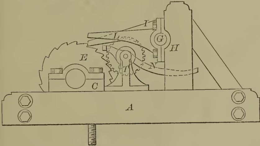
54467—Goodsell & Frisbie— Hoisting Apparatus.
