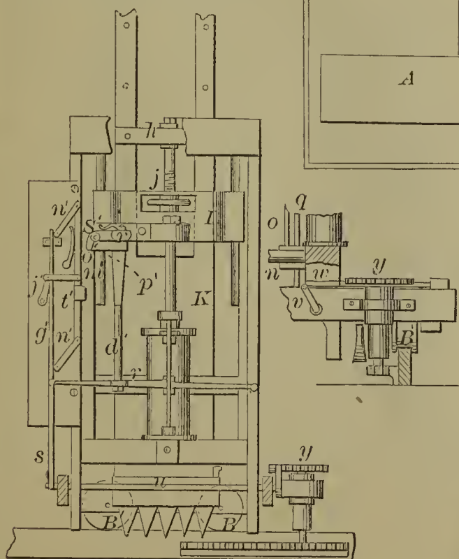
59856—Merriman & Ross—For Channeling Stones.
