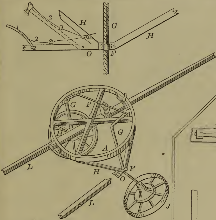
56022—T. E. Ellett—Cultivator.
