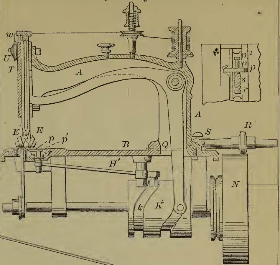
53743—J. S. McCurdy—Sewing Machine.
