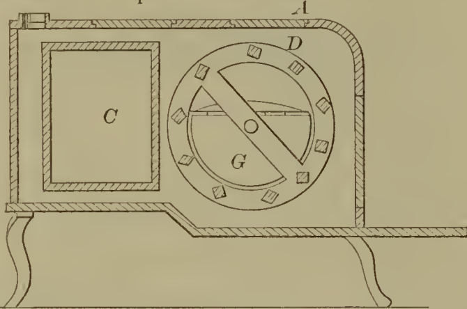
52550—J. & J. Ehart—Washing Machine.
