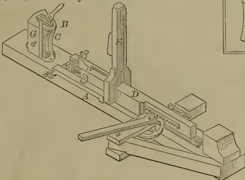
55708—J. J. Ralya— Stave Machine.
