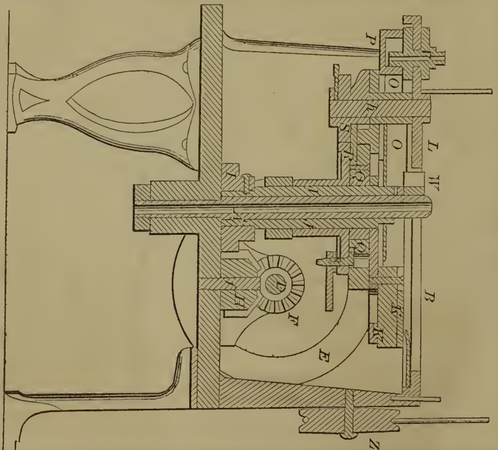
56485—J. A. Bazin—Cordage Machine, &c.
