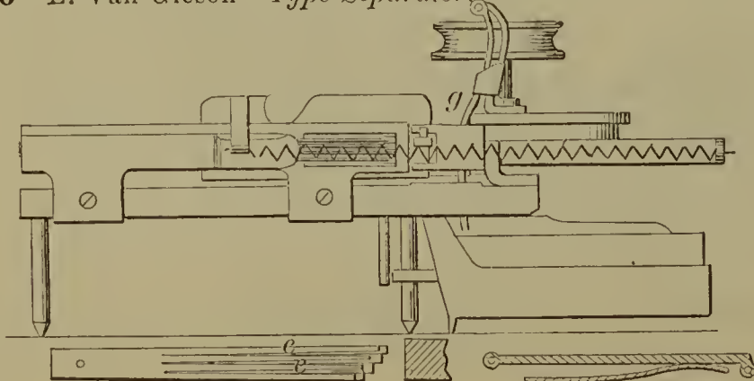
59786—E. Van Gieson— Type Separator.
