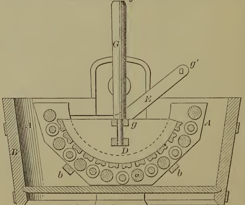
53311—J. S. Lash— Washing Machine.
