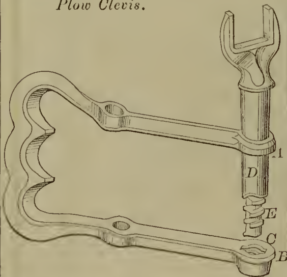
57436—G. P. Darrow— Plow Clevis.
