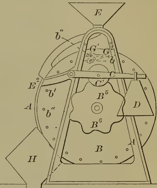
54074—T. Tripp—Amalgamator.
