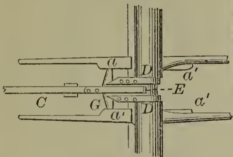
52102—G. L. Witsill—Well Boring.
