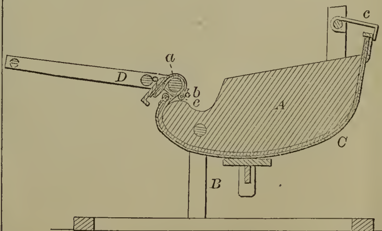
58873—C. Moyer, Jr.— Wood Bending Machine.
