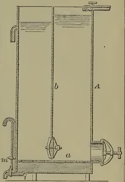
58868—C. F. Mietzsch— Filter.
