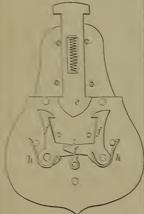
60257—E. A. G. Roulstone—Lock.
