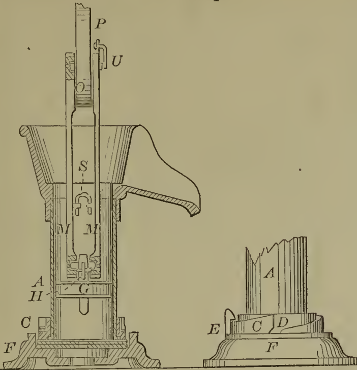
58801—A. F. Fletcher—Pump.
