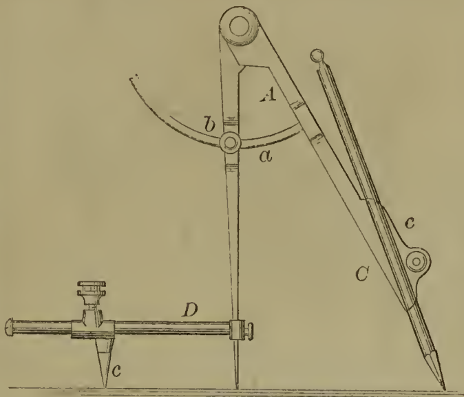
60609—H. M. Albee— Ellipsograph .
