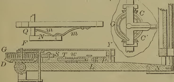
59355—G. E. Burt—Car Brake.
