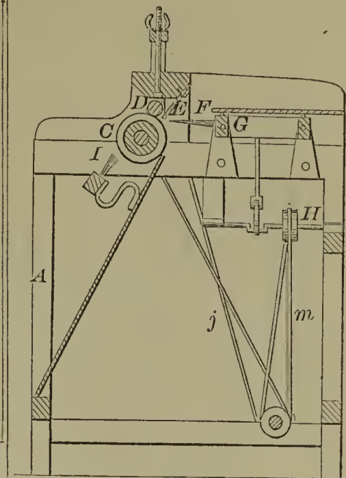
60404—J. M. Miller— Grinding Mill.
