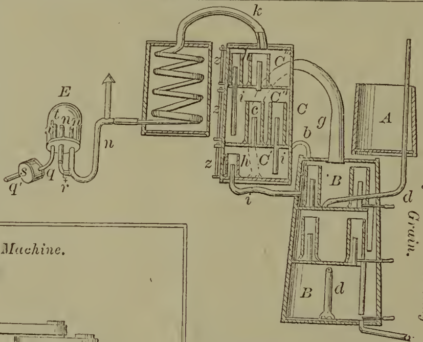
60327—Beebe & Lloyd—For Distilling Grain.
