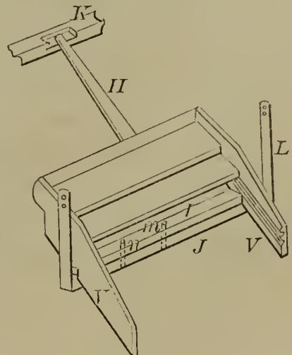
57483—H. W. Curtis—Fanning Mill.
