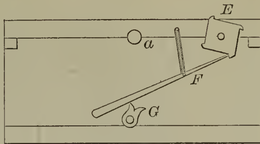
51933—J. H. Elward—Animal Trap.
