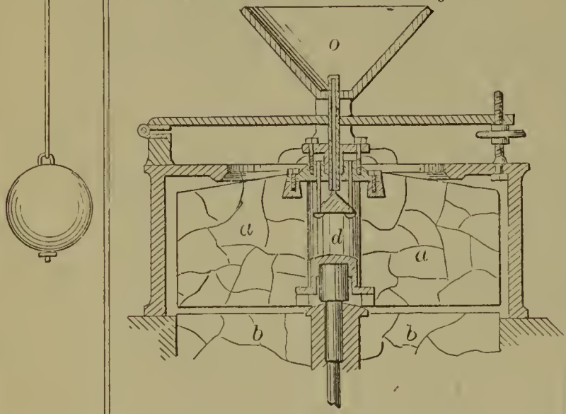
59671—J. N. Smith—Hydrant.
