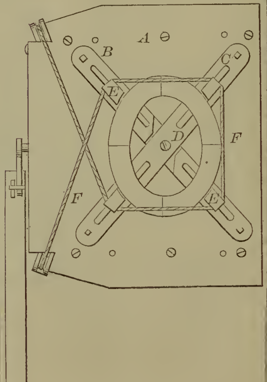
54463—J. A. H. Dunne— Picture Frame Clamp.
