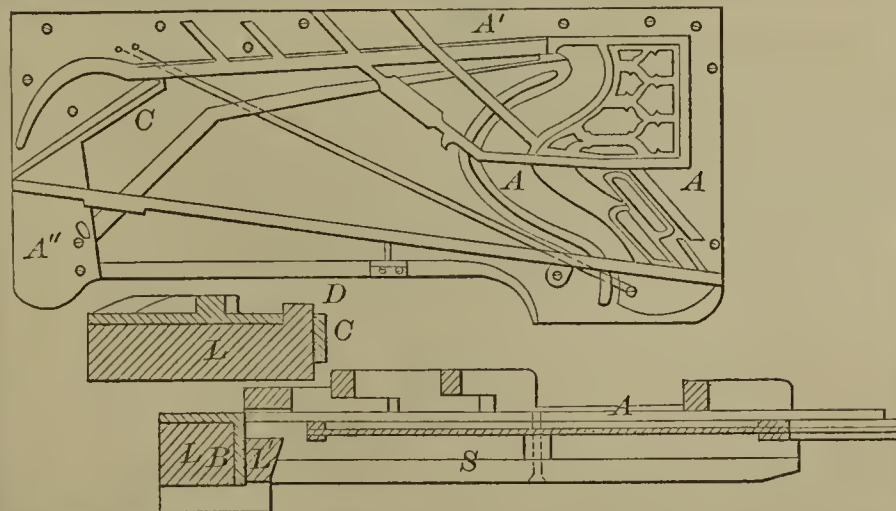
52725—A. Ludolf—Iron Frame for Piano Forte.
