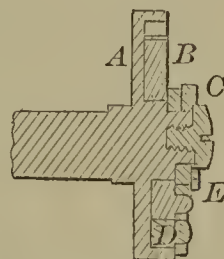
57287—W. Chieken—Sewing Machine.
