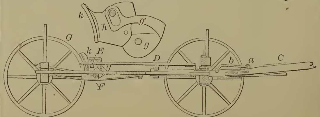
59285—T. G. Springer— Wagon Brake.
