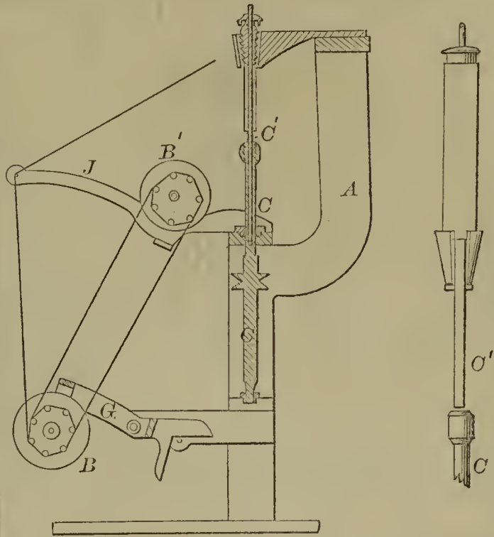
57330—B. H. Jenks— Cop Winding Machine.
