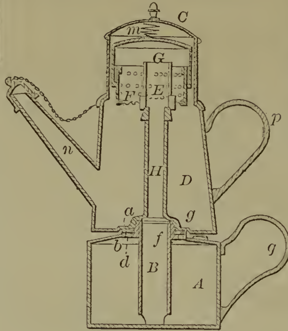
60204—J. H. Lee—Coffee Pot.
