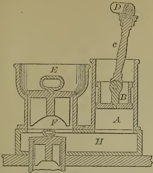
55147—G. Moulton, Jr.— Ship's Pump.
