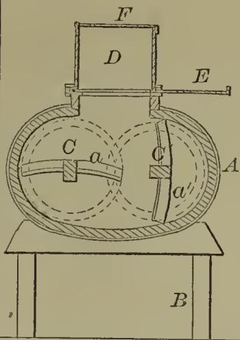
60058—J. K. Reiner—Churn.
