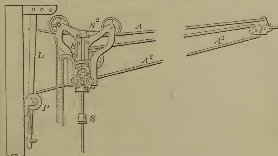
52676—E. H. Carpenter— Track Rope Hay Elevator.
