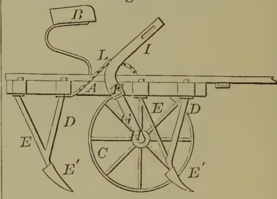
57619—J. Bergen—Cultivator.
