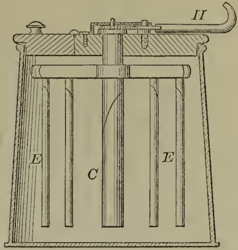
52066—J. O'Donald— Churn.
