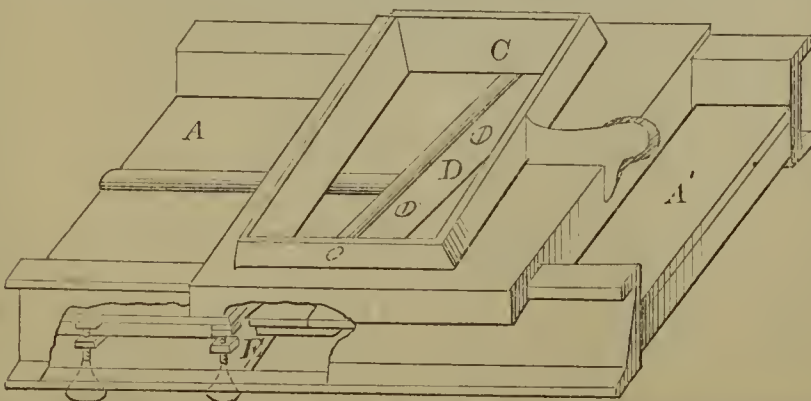
56883—J. Bell—Stave Cutting Machine.
