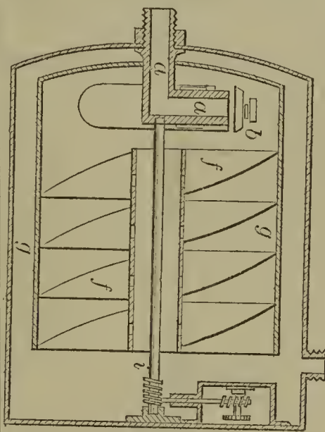
57268—J. T. Scholte—Gas Meter.
