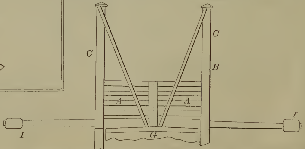
55914—J. H. Schenek—Automatic Gate.
