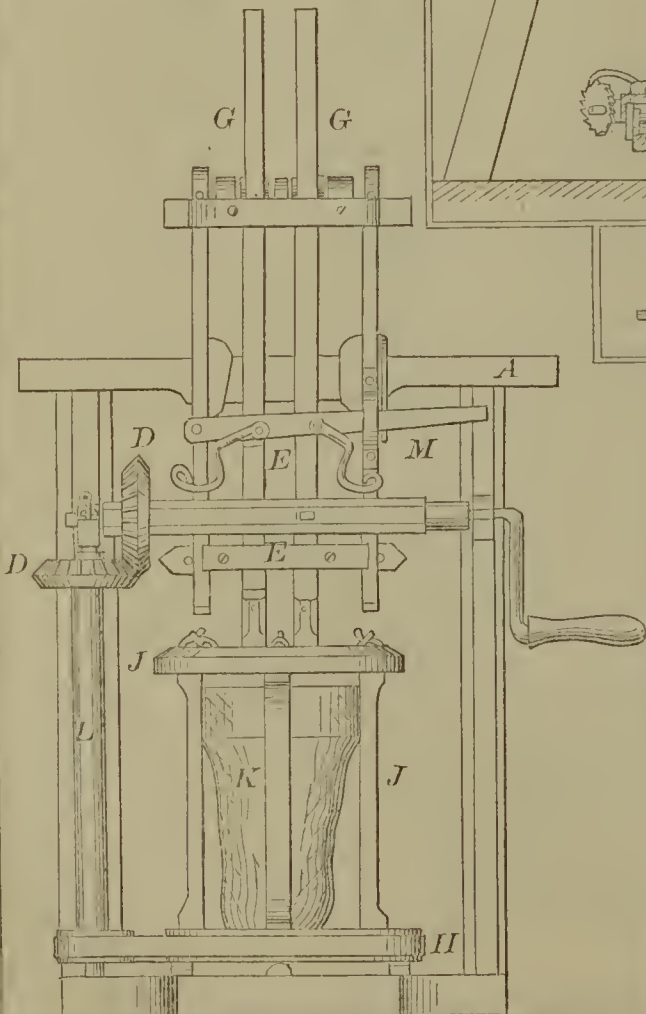
55885—J. Musser—Flour Packer.
