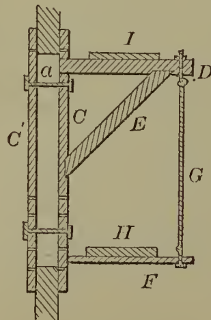
58571—W. Arrouquier— Staging.
