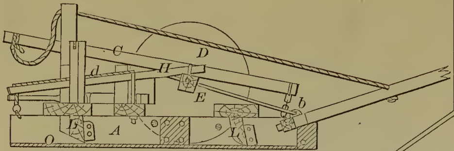
54003—F. Monroe— Land Leveler.
