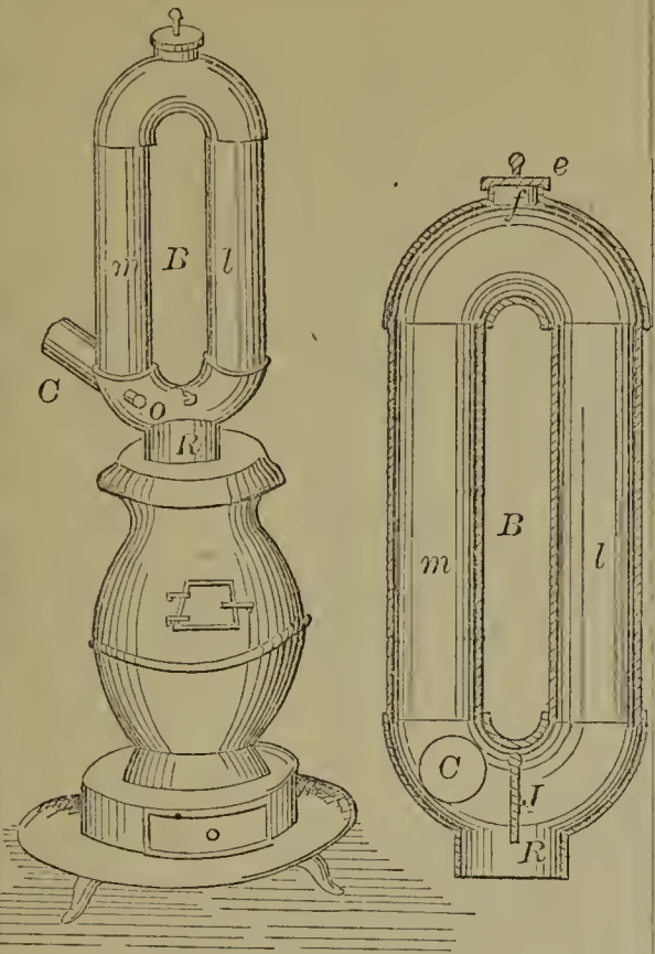
59173—E. S. Blake— Stove Pipe Drum.
