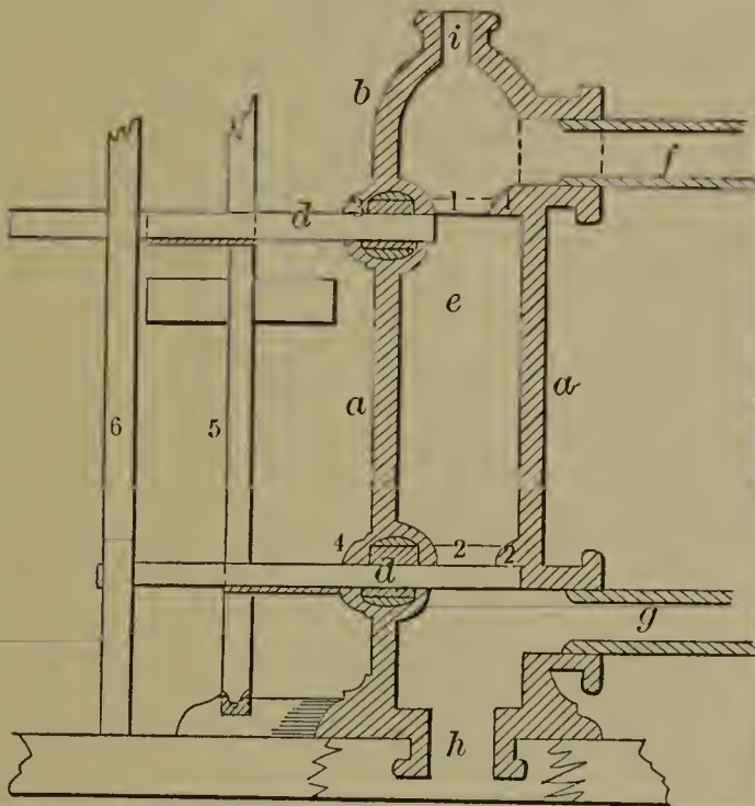
53044—F. Rumpf— Crane.
