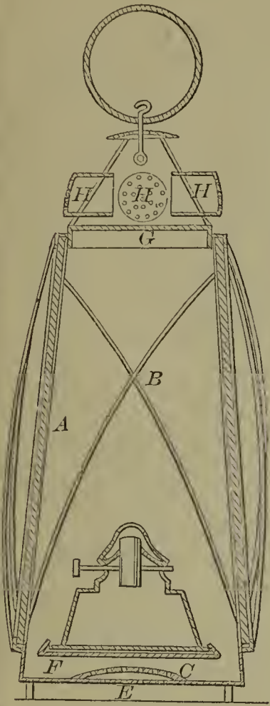
60140—R. Chester— Lantern.
