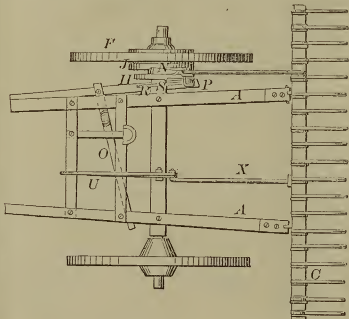
57488—Dunham & J. & A. Webb— Horse Rake.
