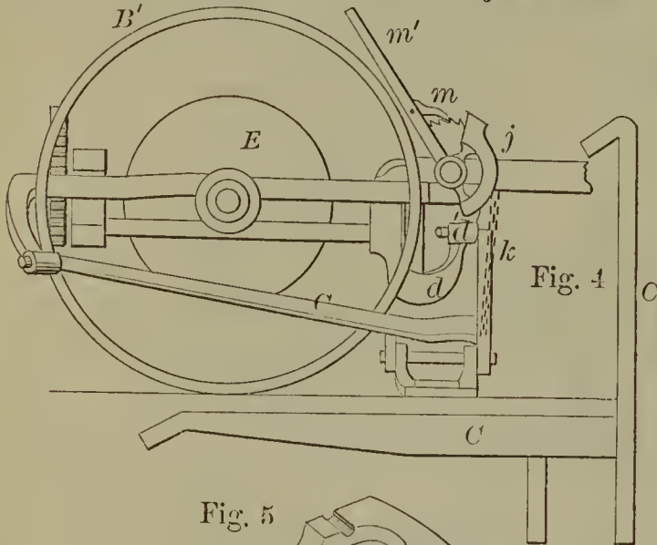
52264—W. H. Burkhart— Harvesting Machine.
