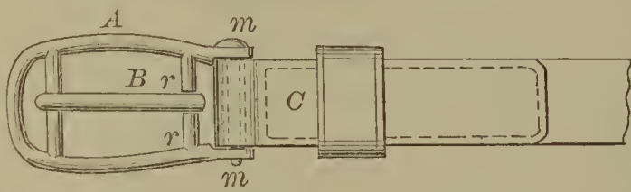
54504—C. S. Cissna—Buckle.
