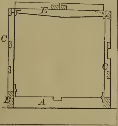
56541—B. F. Elliott— Grape Trellis.
