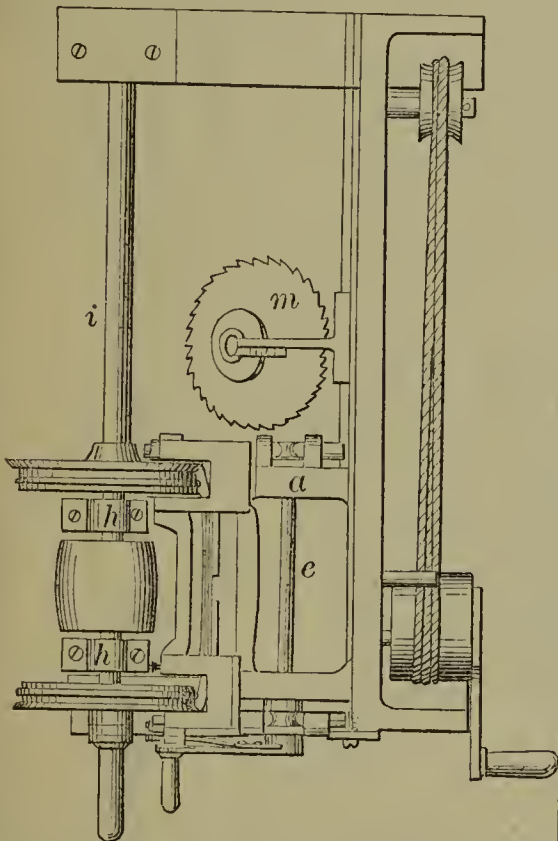
53618—A. H. Hook— Stave Machine.
