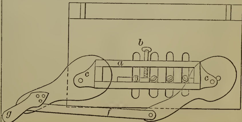
55223—J. S. L. Babbs—Dovetailing Machine.
