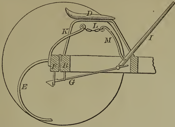
58075—J. Dillier— Horse Rake.
