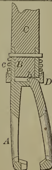
58872—W. Morehouse— Mop Holder.
