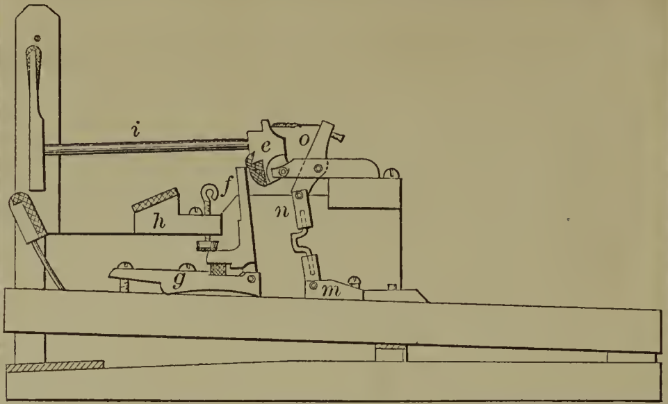
60519—G. H. Hulskamp— Piano Forte.
