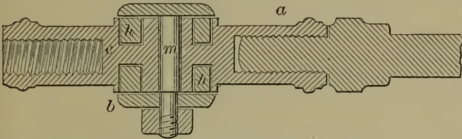
52969—J. K. Collins— Knuckle Joint.
