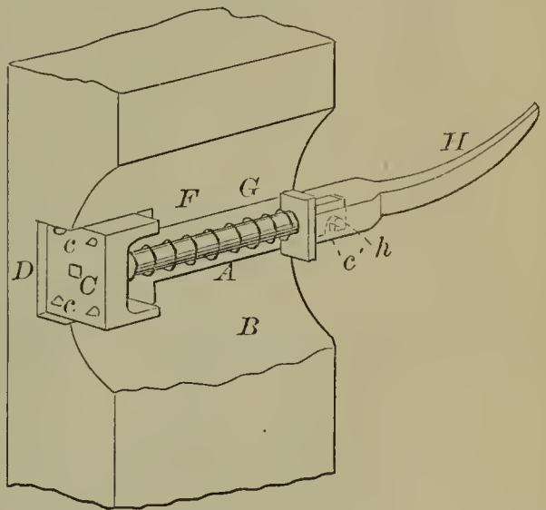
55475—J. W. Elliot— Sash Fastener.
