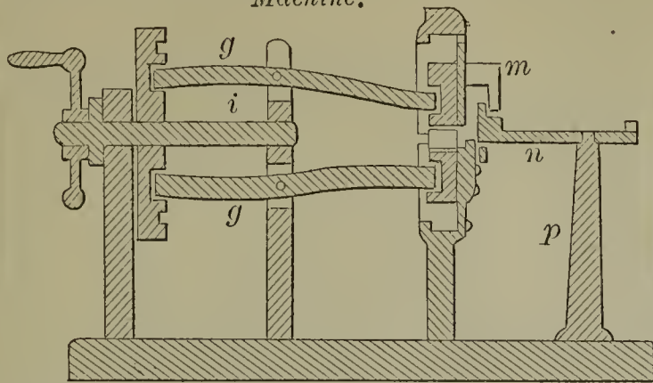
52084—J. N. Smith—Hay and Cotton Press.
