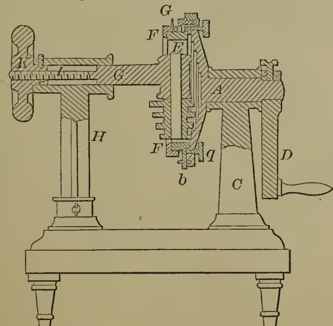
54621—C. F. Spaulding— Spinning Metal.
