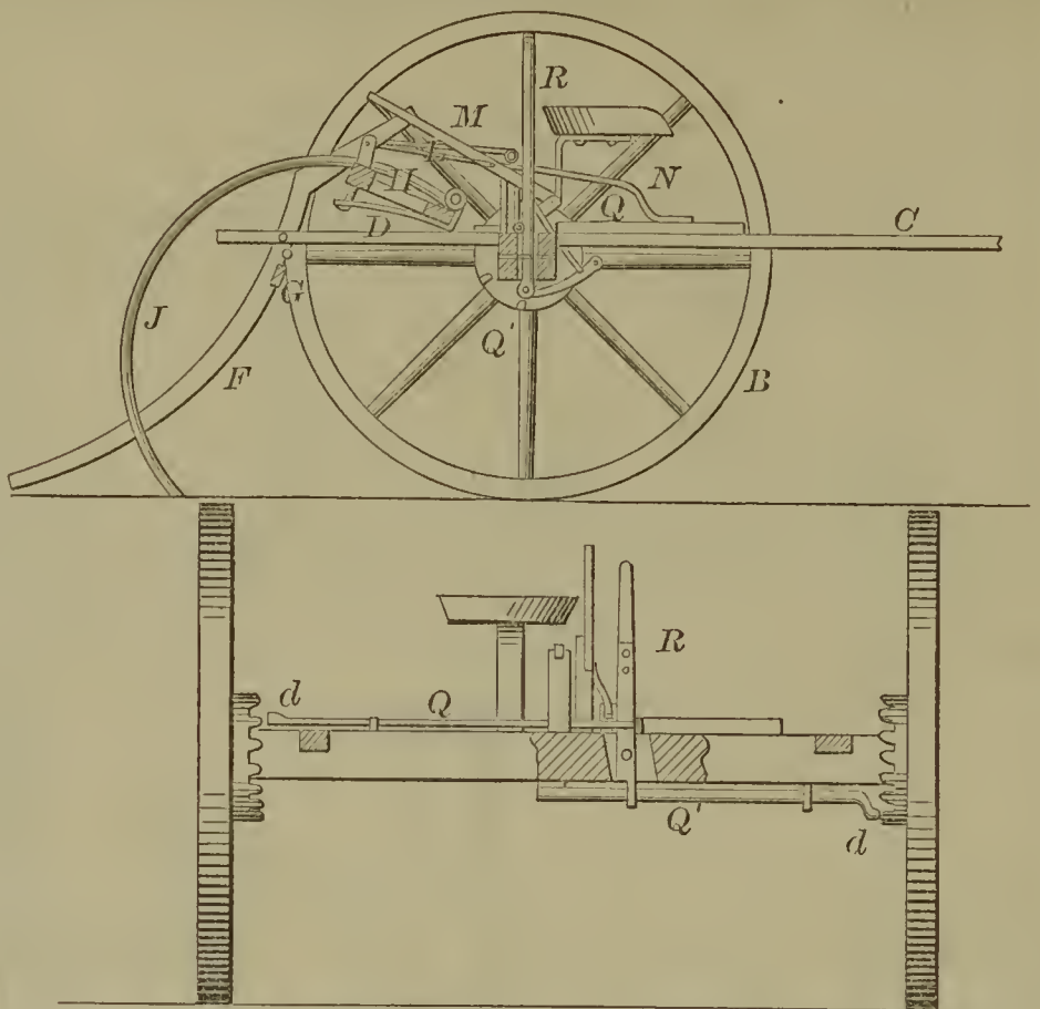
52458—F. Stewart— Horse Rake.
