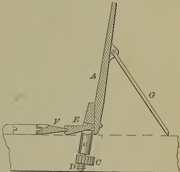
55424—A. Lloyd—Floor Clamp.
