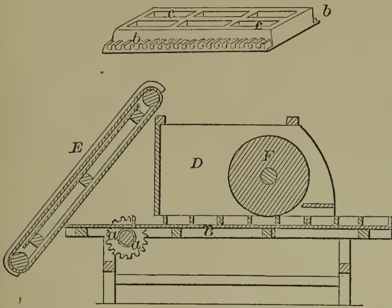
60397—J. B. Lyons— Peat Machine.
