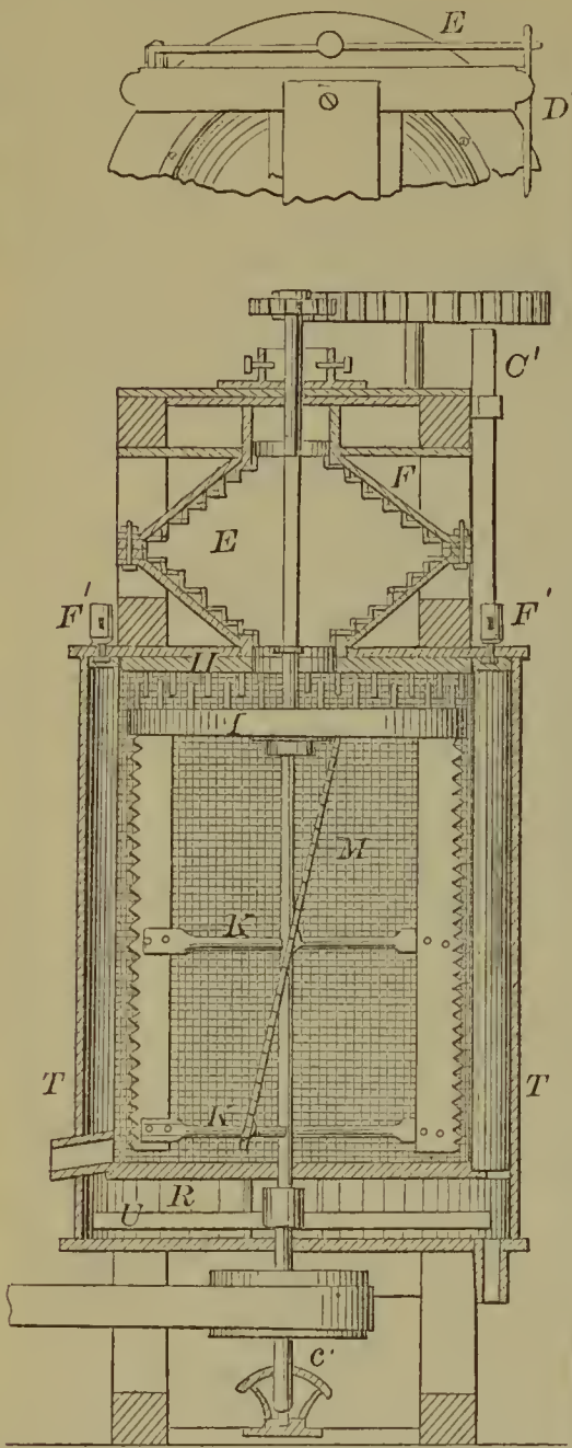
59862—G. H. Reynolds— Bran Duster.
