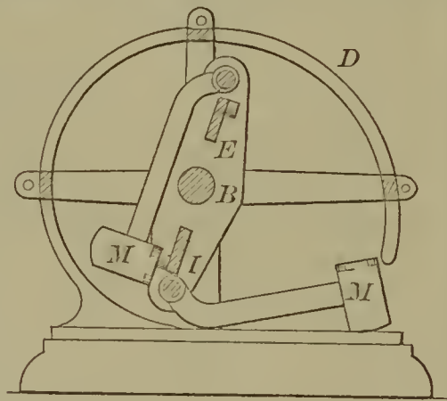
52447—A. Rix—Forging Apparatus.
