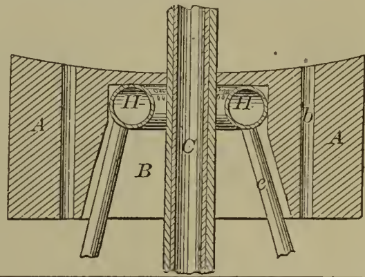
56626—M. B. Stafford— Peat Machine.
