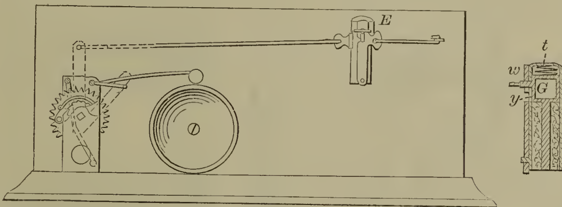
55957—C. D. Kubach— Fire Alarm.
