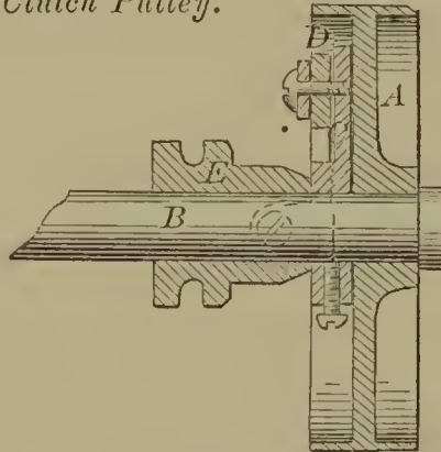
58768—T. W. Brown— Grindstone Journal Box.
