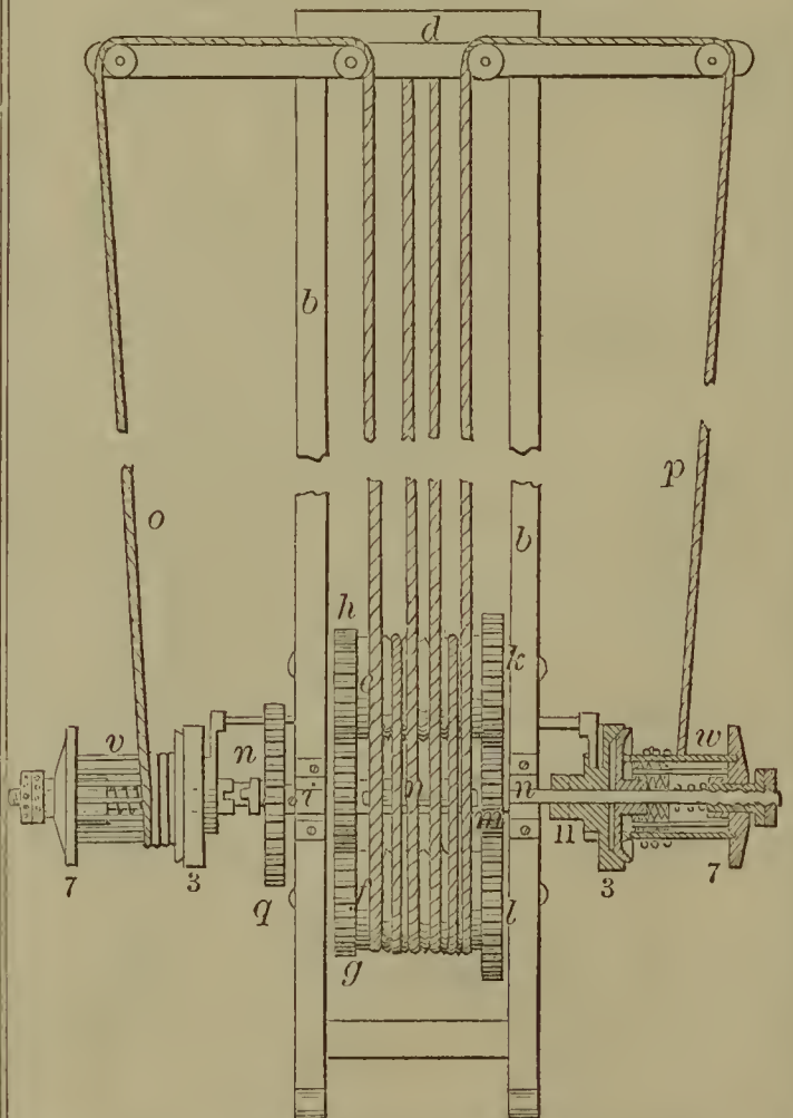
52777—D. D. Winant—Derrick.
