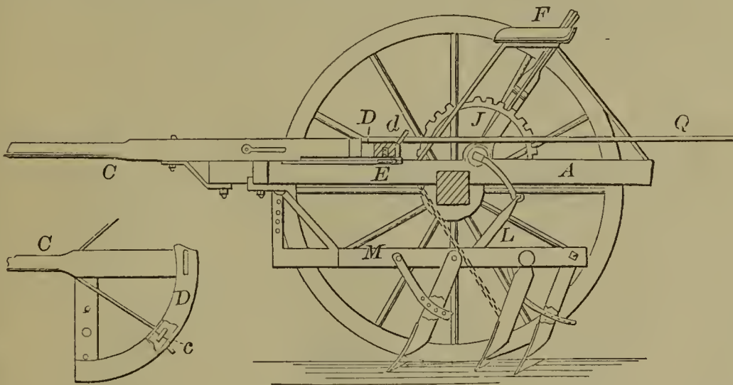
59643—W. W. Philler—Cultivator.
