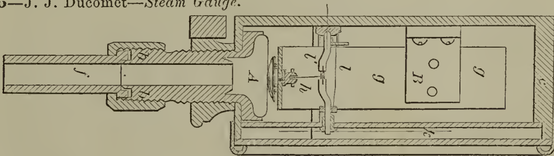
52006—J. J. Ducomet—Steam Gauge.
