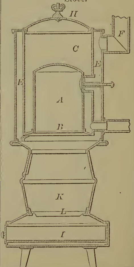
59563—H. G. Dayton— Coal Stove.
