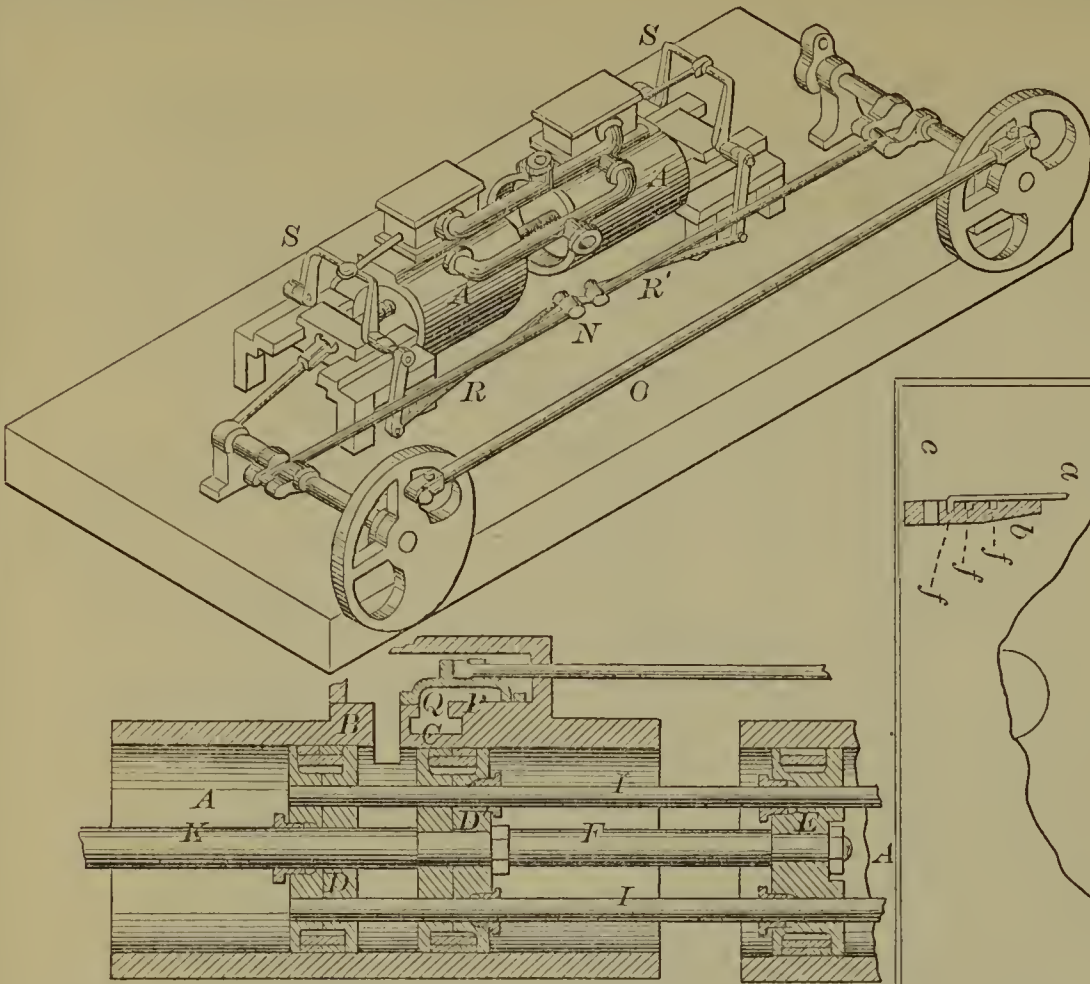
53597—J. T. Forrer—Mash Machine.
