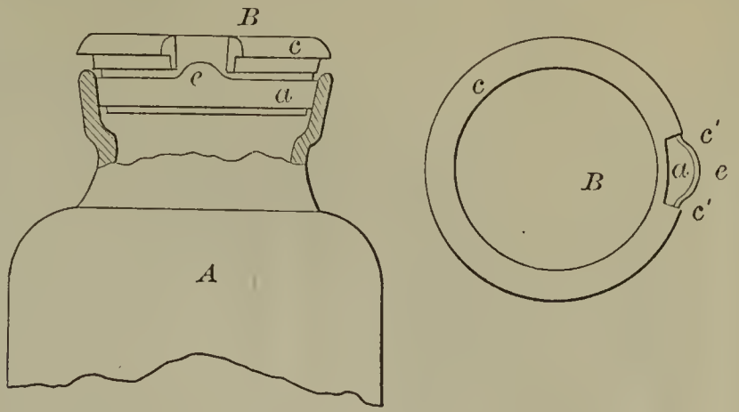
51785—J. Adams— Preserve Jar .
