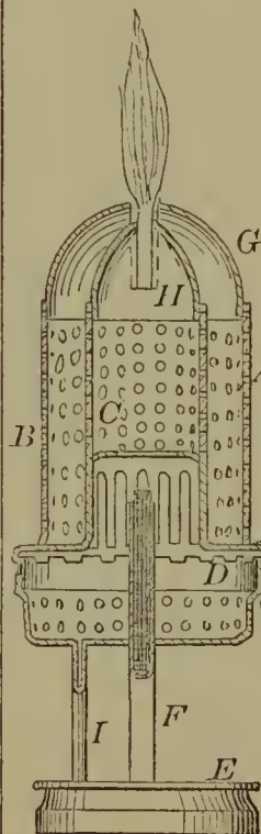
59704—J. K. Andrews—Lamp Burner.
