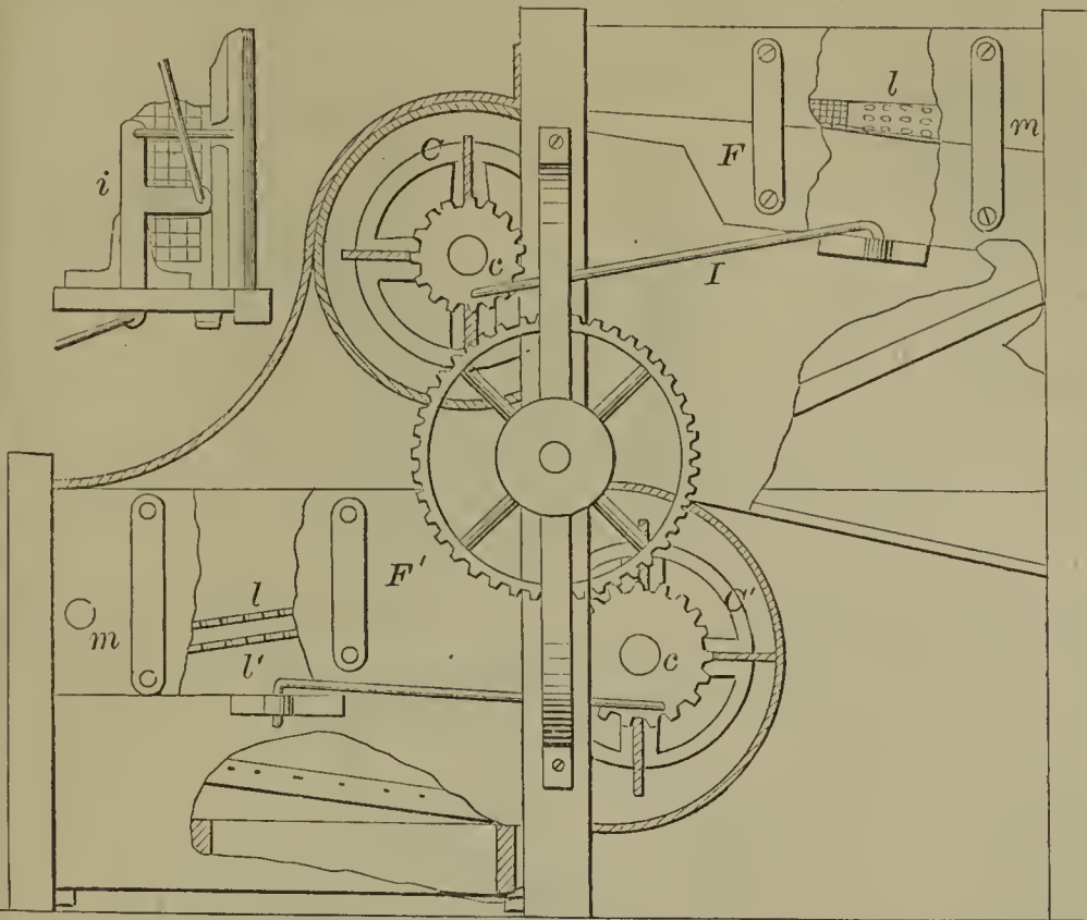
55956—J. L. Kendall— Clothes Sprinkler.
