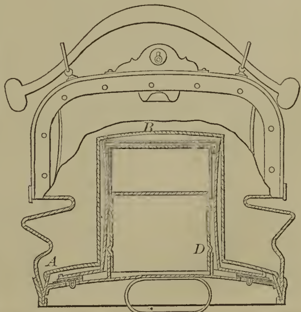
58792—Z. S. Durfee—Hat Box and Valise.
