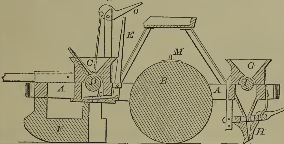
58049—W. N. Barr— Cane Stripper.
