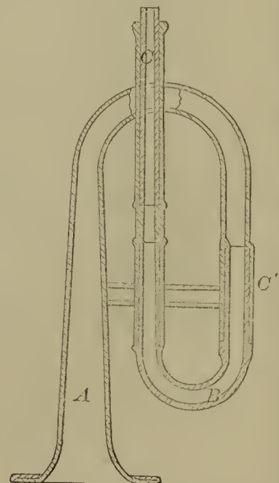
52580—H. G. Lehnert— Bugles, Horns, &c.
