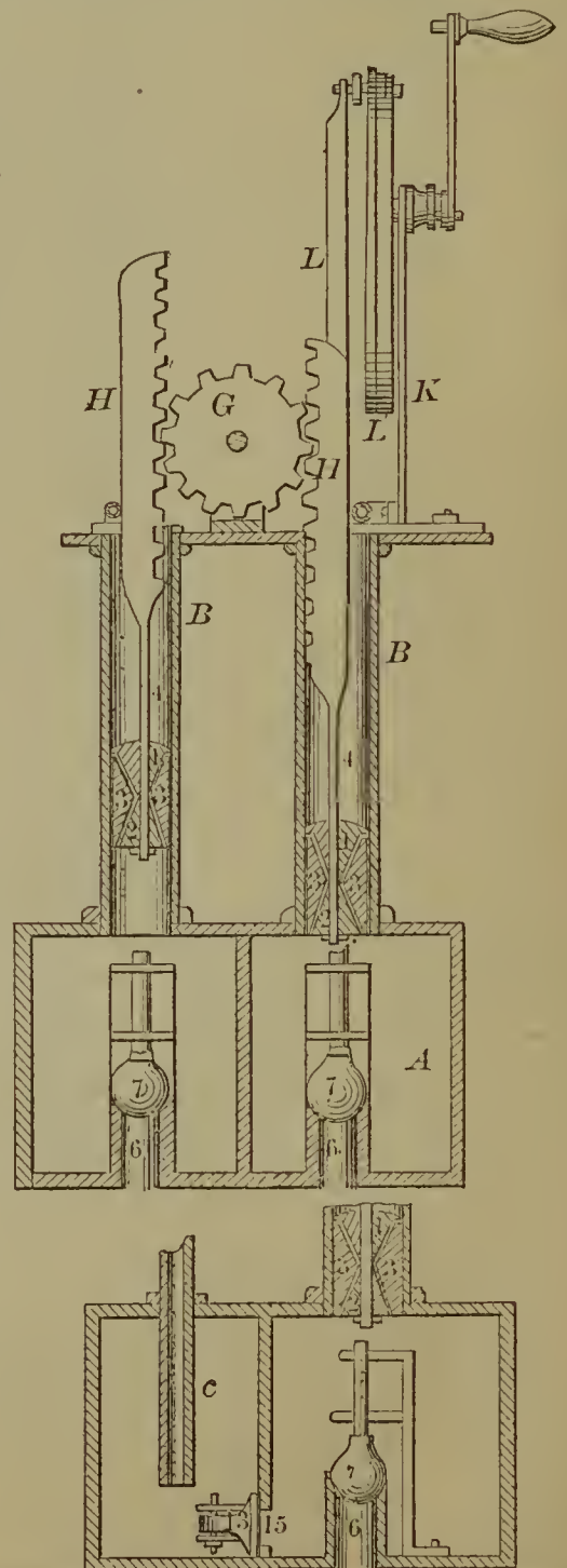
56387—S. S. Durbon—Pump.
