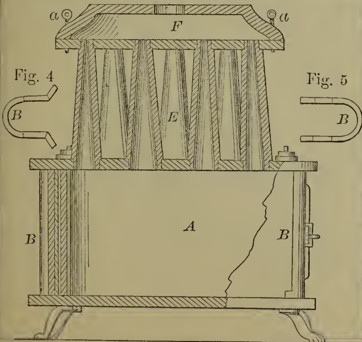
54319—J. H. Flagg— Soap Stone Store.
