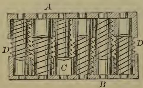
53292—J. J. Gest—Car Spring.
