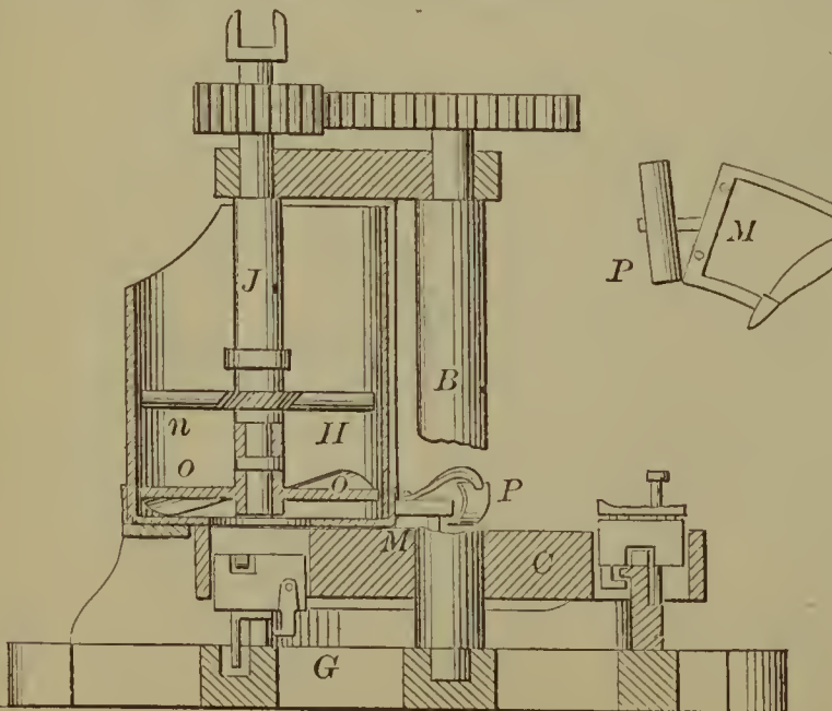
59831—E. R. Gard— Brick Machine.
