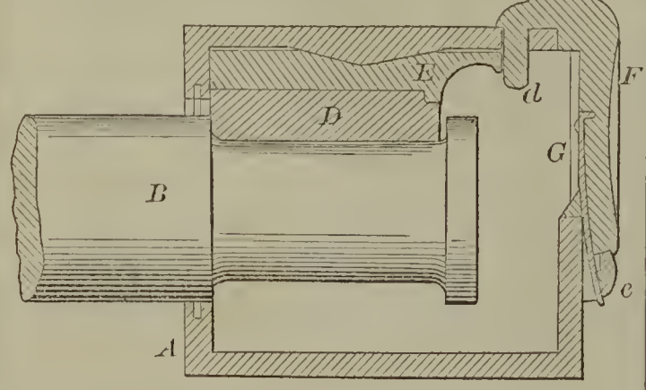
52029—J. Christy— Axle Box.
