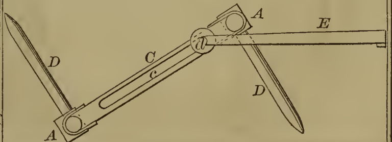
56517—J. N. Baxter—Horse Rake.
