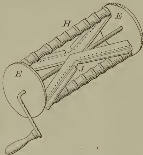
51881—H. Tilden—Flour Sifter.
