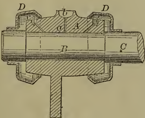
56624—A. R. Sherman— Lubricating Journal Boxes.
