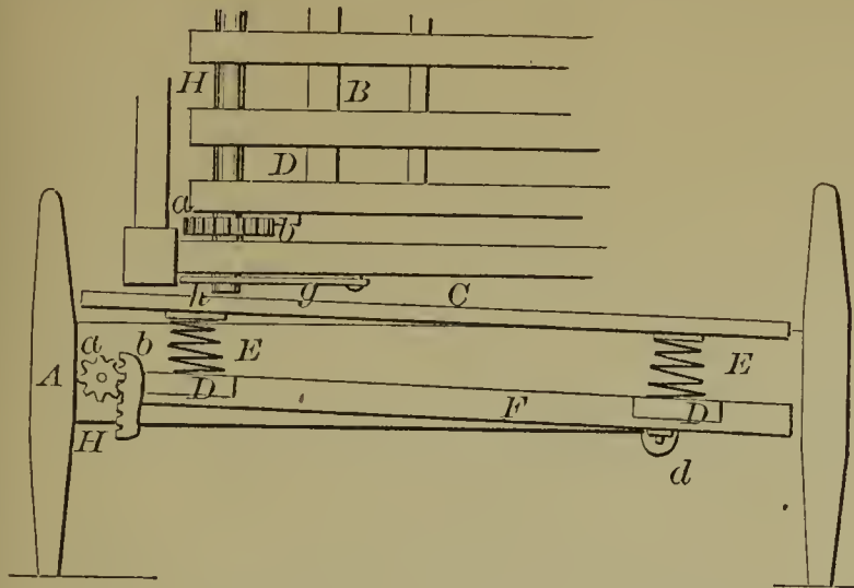
53706—E. W. Tucker— Bed Bottom.
