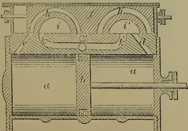
54163—A. J. Homan— Slide Valve.
