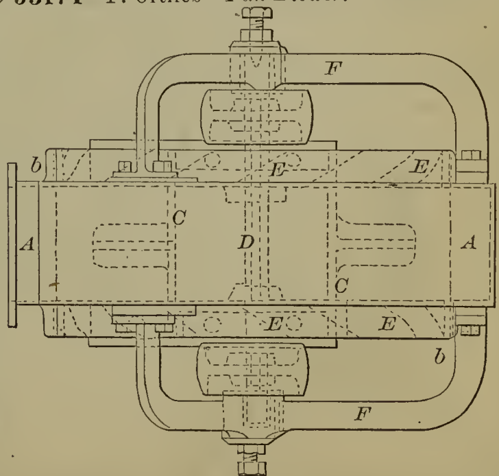
53174—F. Ortlieb— Fan Blower.
