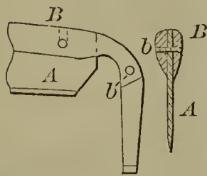
57440—C. M. Hodges— Scythe.
