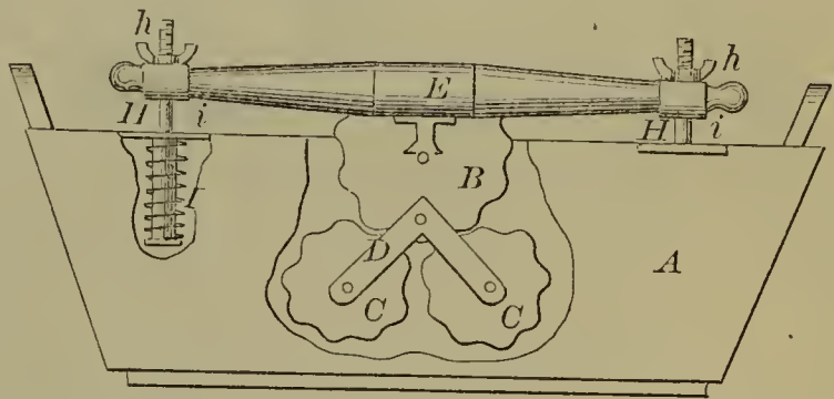
53604—J. T. Greenwood, Sr.—Washing Machine.
