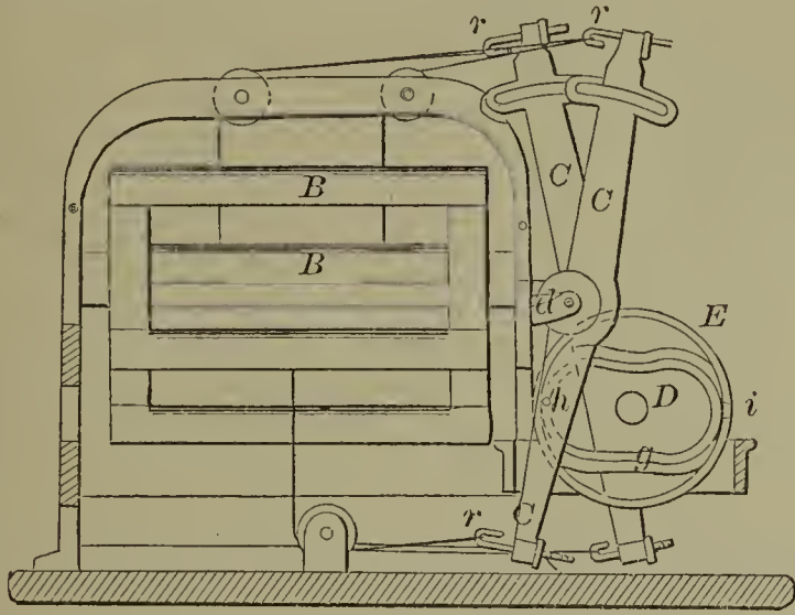
59987—H. A. Ellis—Loom.
