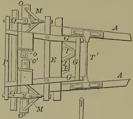
58689—J. A. Spear—Horse Rake.
