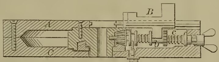
57383—R. & T. Ross—Chuck.
