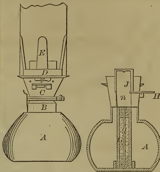
56503—W. M. Wright—Carburetted Gas.
