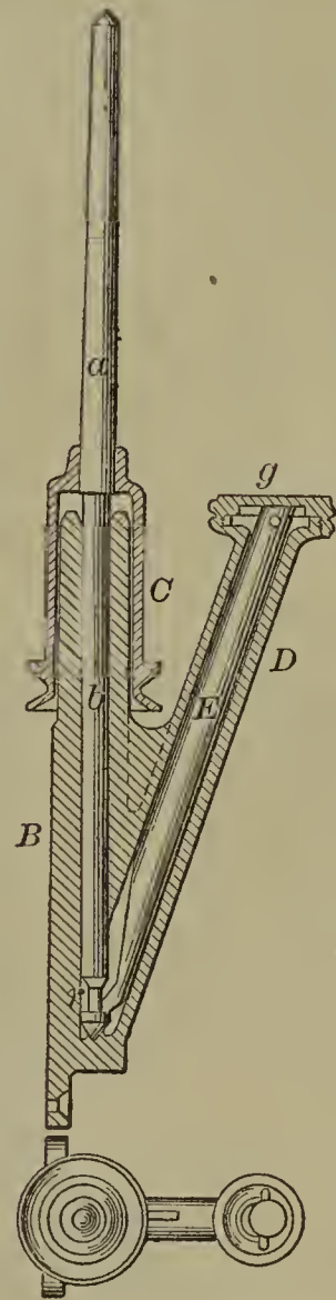
58046—J. E. Atwood— Spinning Frame Spindle.
