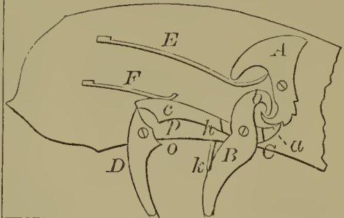
58445—J. McMurtry— Cotton Bale Tie.
