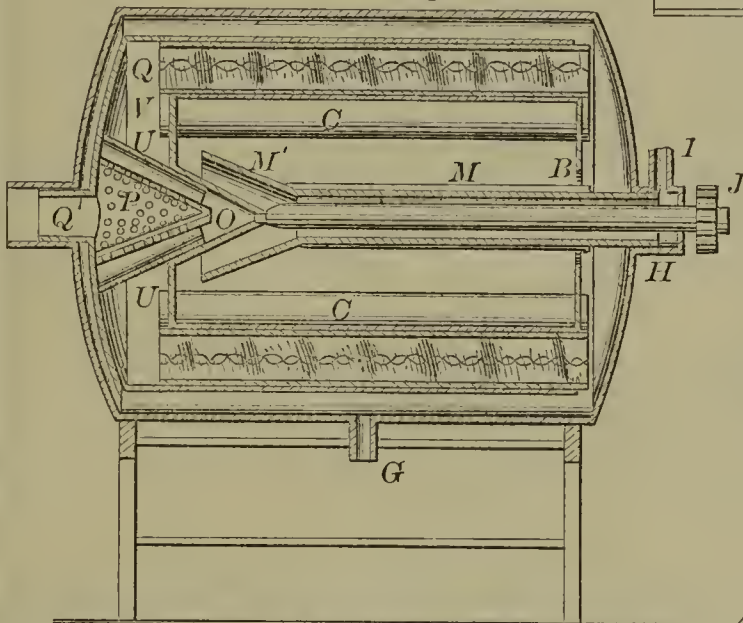
57546—J. E. Moeller— Water Elevator.
