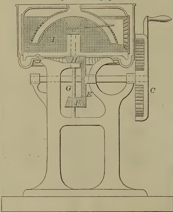
57517—J. O. Joyce—Centrifugal Machine.
