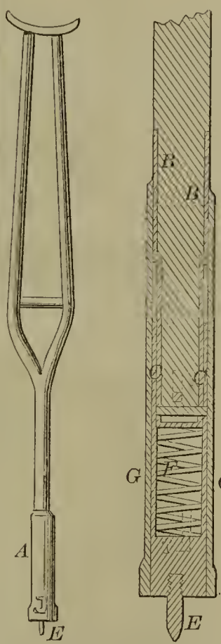
57416—R. W. Ware— Crotch.
