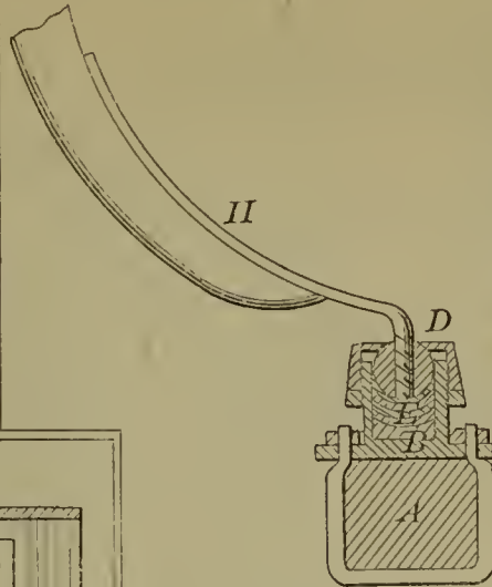
59728—T. S. Smith— Carriage Shackle.
