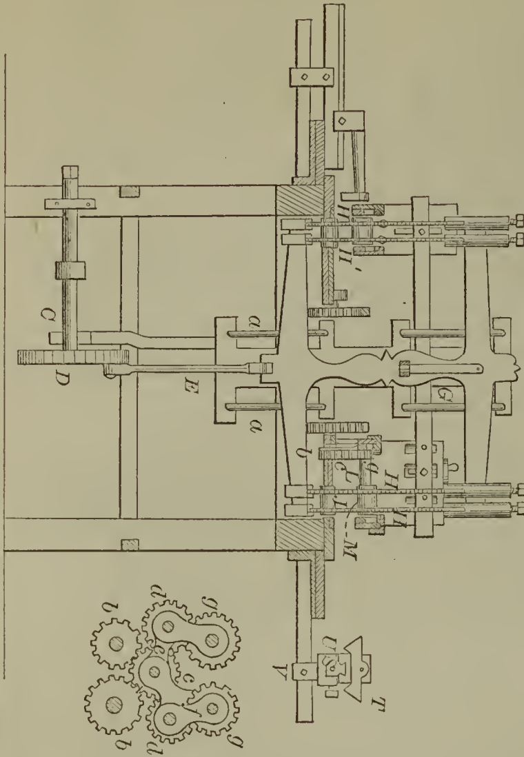
52039—J. A. Geer—Sewing Machine.
