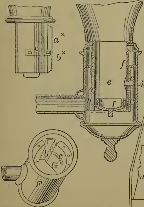
58361—G. Stobwasser— Lamp.
