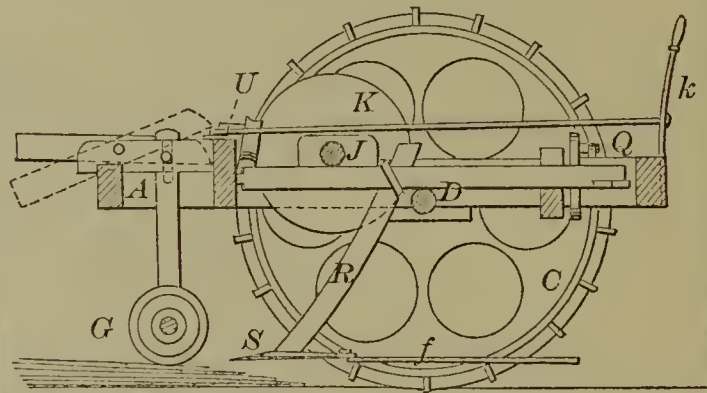
53349—L. F. Schanck—Potato Digger.
