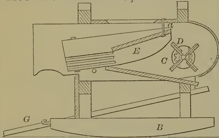
54405—J. N. Ray—For Bending Wood.
