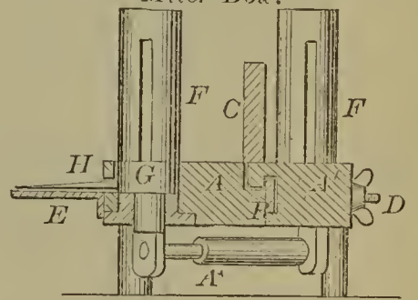
59046—J. A. McKinstry—Miter Box.
