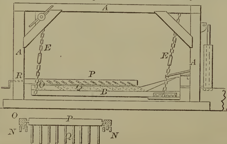
60089—H. A. Thompson—For Concentrating Ores.
