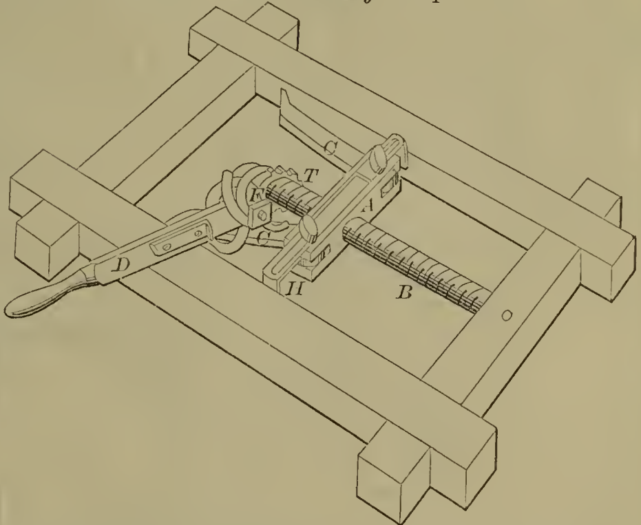
57078—Blinn & Hewitt— Flooring Clamp.
