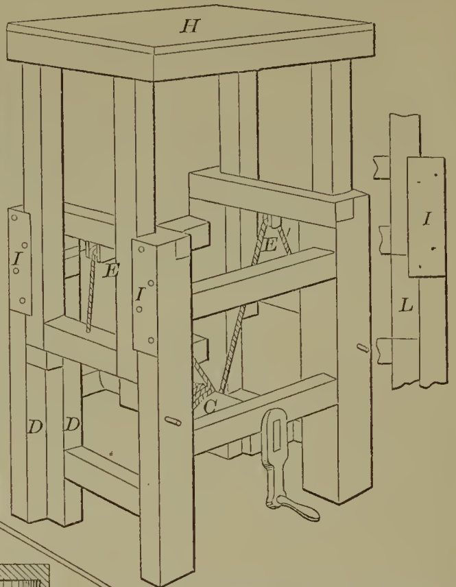
60088—G. L. Thompson—For Pressing Hats.
