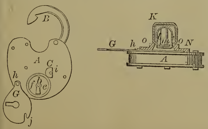
58278—E. M. & J. E. Mix—Padlock.
