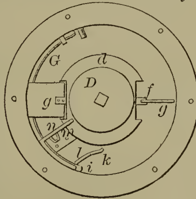
56627—J. A. Stansbury— Pump.
