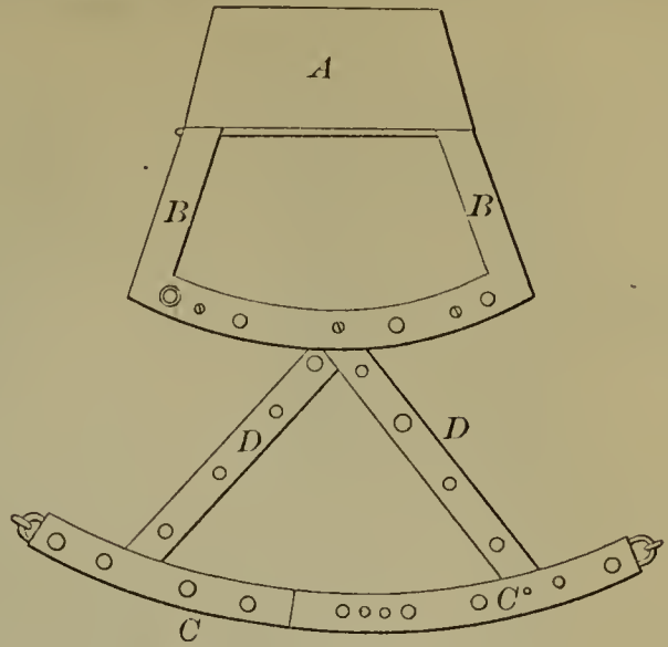
53654—J. H. Mumma—Broom Head.
