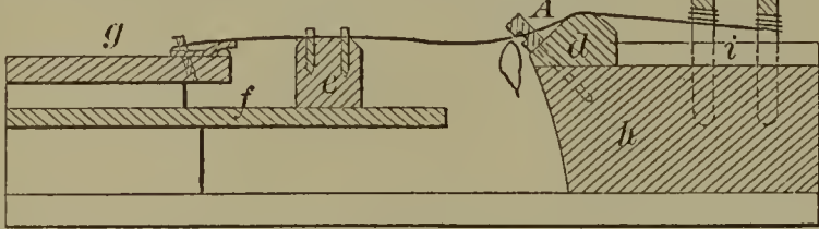
60519—G. H. Hulskamp— Piano Forte.
