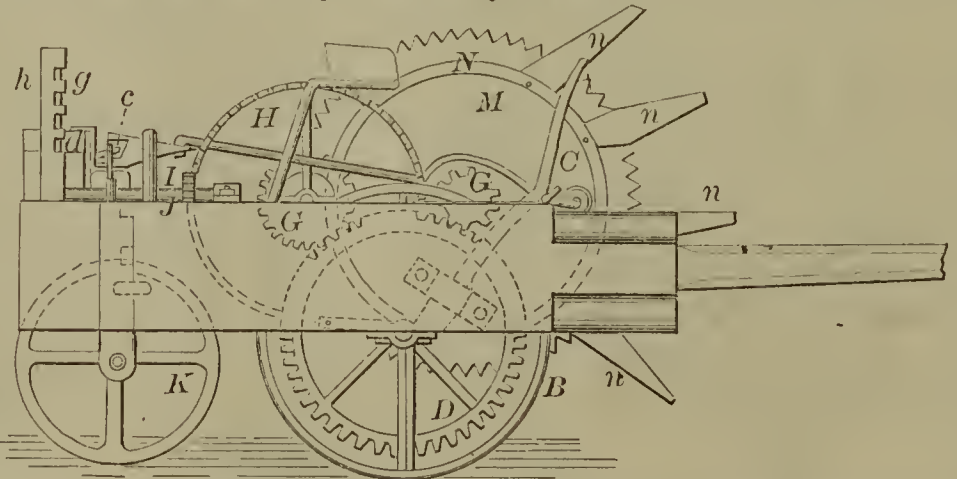
57590—W. & H. Sperry—Hedge Trimmer.
