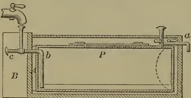
53829—J. K. Ingalls—Oil Tank.
