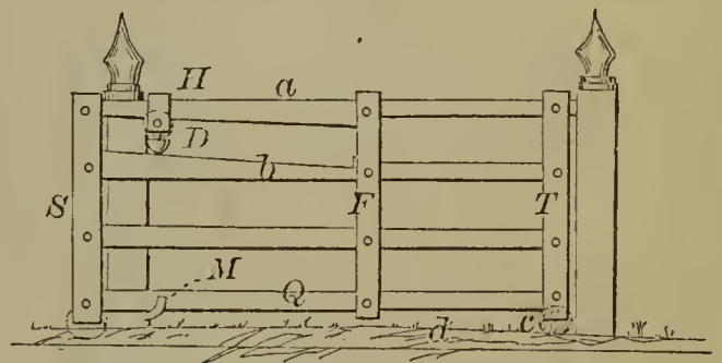
53856—J. C. Murphy—Farm Gate.
