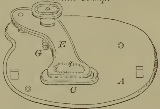
55866—J. A. & H. A. House—Sewing Machine Clamp.
