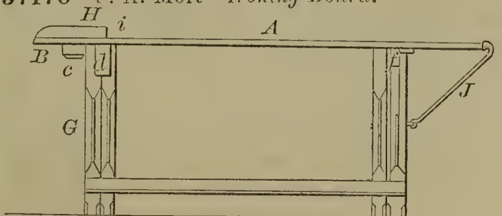
57170—S. A. Mort— Ironing Board.
