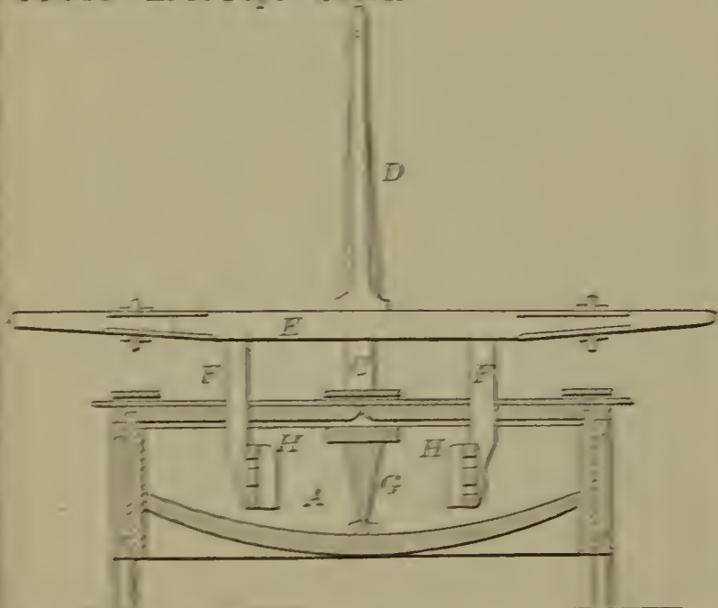
60240—A. J. Pope— Clamp.
