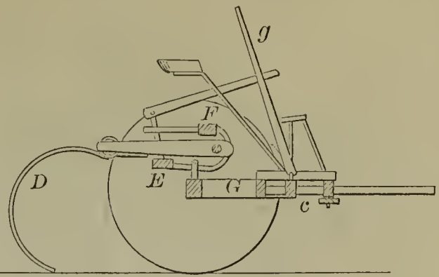
52152—C. H. Finson—Horse Rake.
