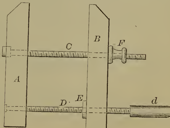
59861—W. Ormesby—Hand Screw Clamp.
