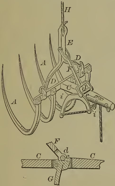
57609—F. Wicks—Horse Hay Fork.
