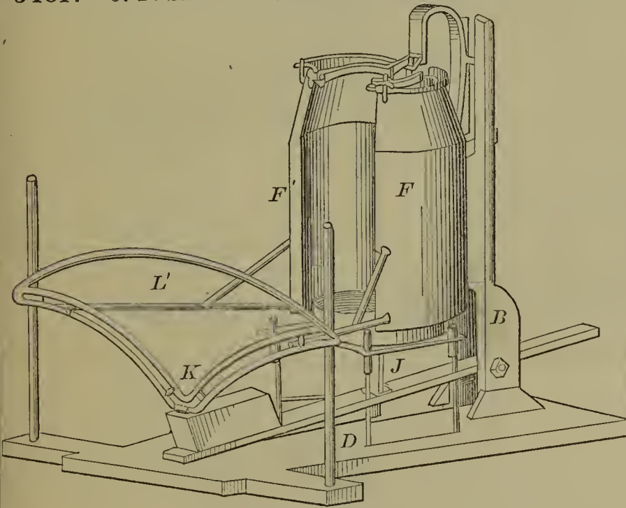
54621—C. F. Spaulding— Spinning Metal.
