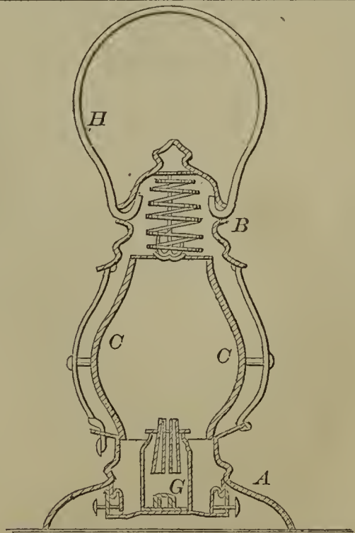
57914—J. H. Irwin— Lantern.
