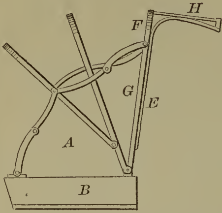
60066—W. F. Rundell— Carriage Top.
