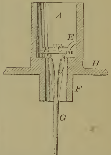
59366—M. G. Crane—Ice Cream Freezer.
