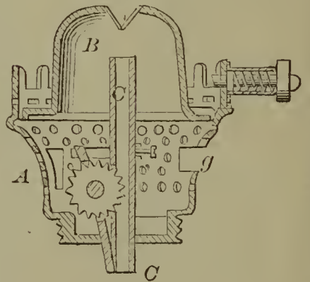
58893—J. F. Sanford— Lamp Burner.
