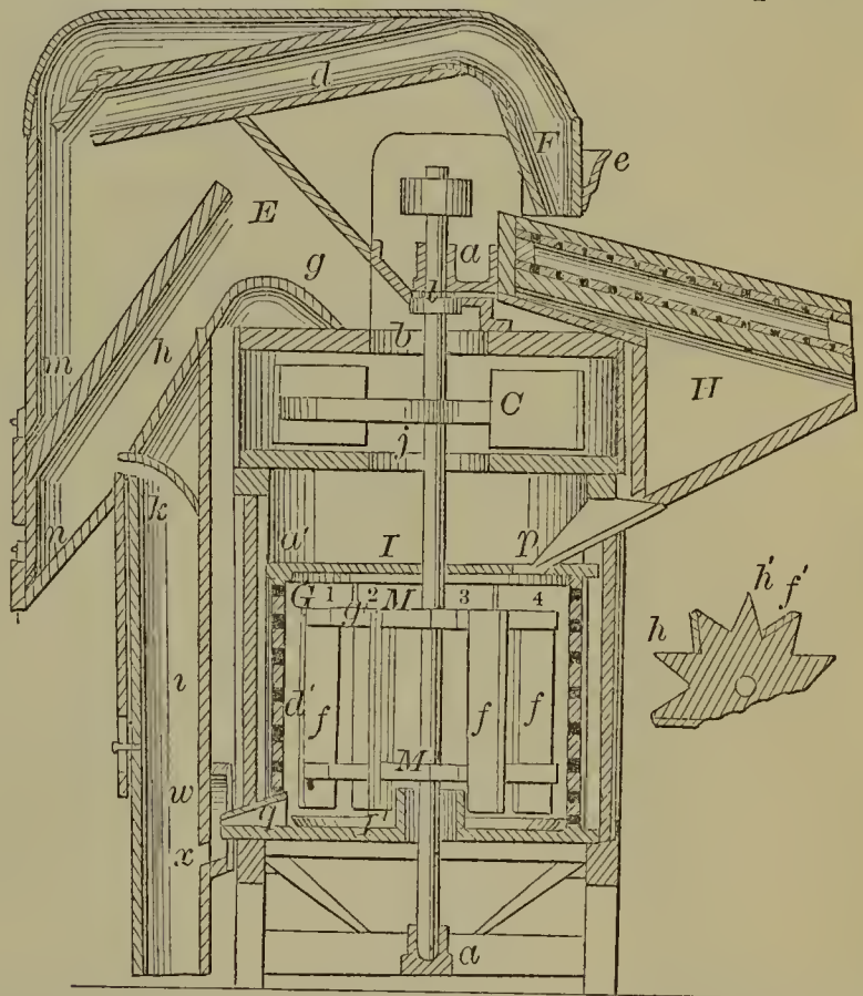
55180—F. Villard—Ventilator.
