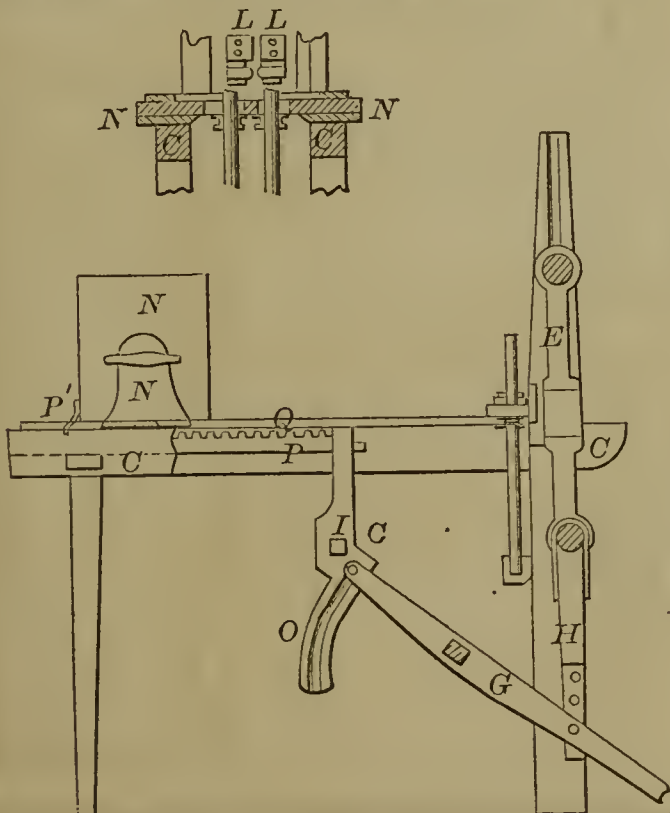
56445—W. Pruett—Tenon Machine.
