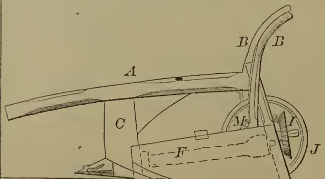
58177—J. A. Quick—Plow.
