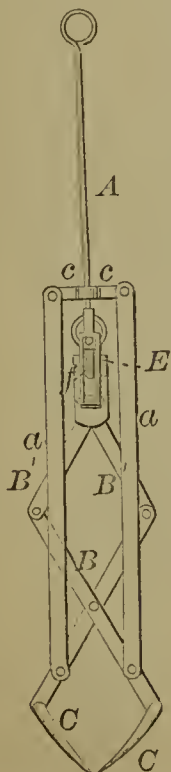
56936—S. & D. Harris—Horse Hay Fork.
