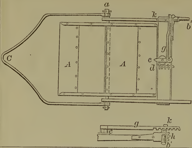
60326—E. Beckwith—Washing Machine.
