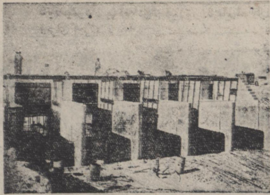
در عکس بالا بتون ریزی پایه ها و بل بویور محل تنظیم آب برسد کرخه دیده میشود
