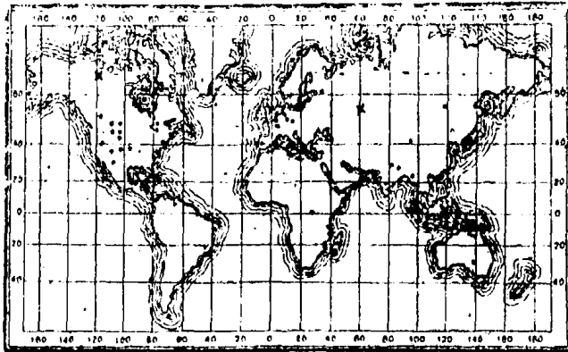
世界鈾錒礦之分佈圖 (圖中 × 代表發現最近之鈾礦但位置不甚確定)
