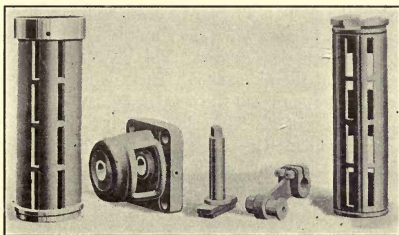
FIG. 279.—Bessemer Corliss air valve.
