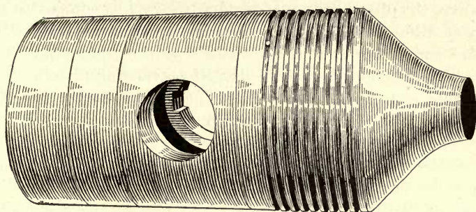
FIG. 55.—McEwen Diesel piston.
