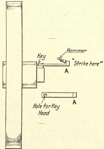
FIG. 287.—Key puller.
