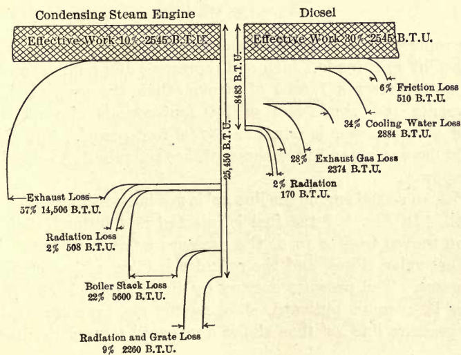
FIG. 195.—Heat balances.
