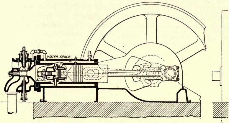
FIG. 234a.—De La Vergne type F.H. semi-Diesel engine.
