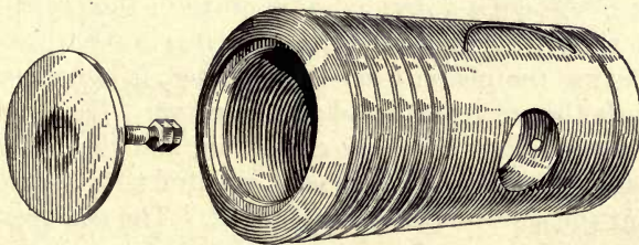
FIG. 54a.—Allis-Chalmers Diesel piston.
