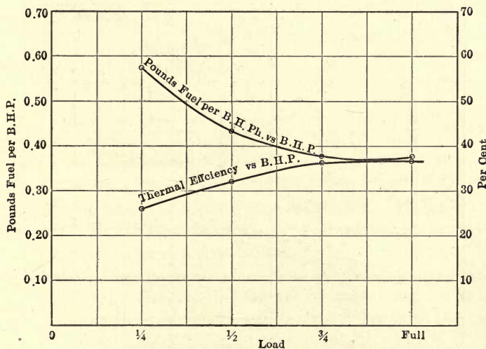
FIG. 187.—Test of 300 H.P. Körting Diesel.
