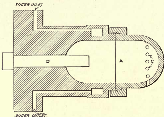
FIG. 224.—Nordberg semi-Diesel ignitor.
