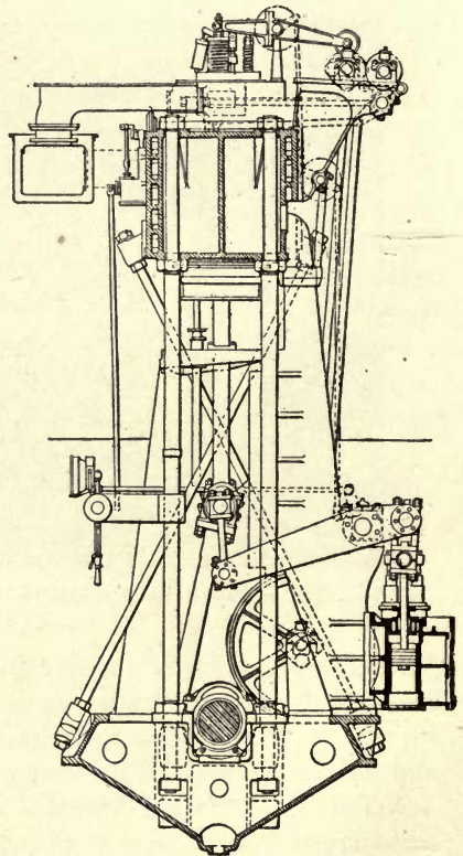
FIG. 18.—Werkspoor open frame marine Diesel.
