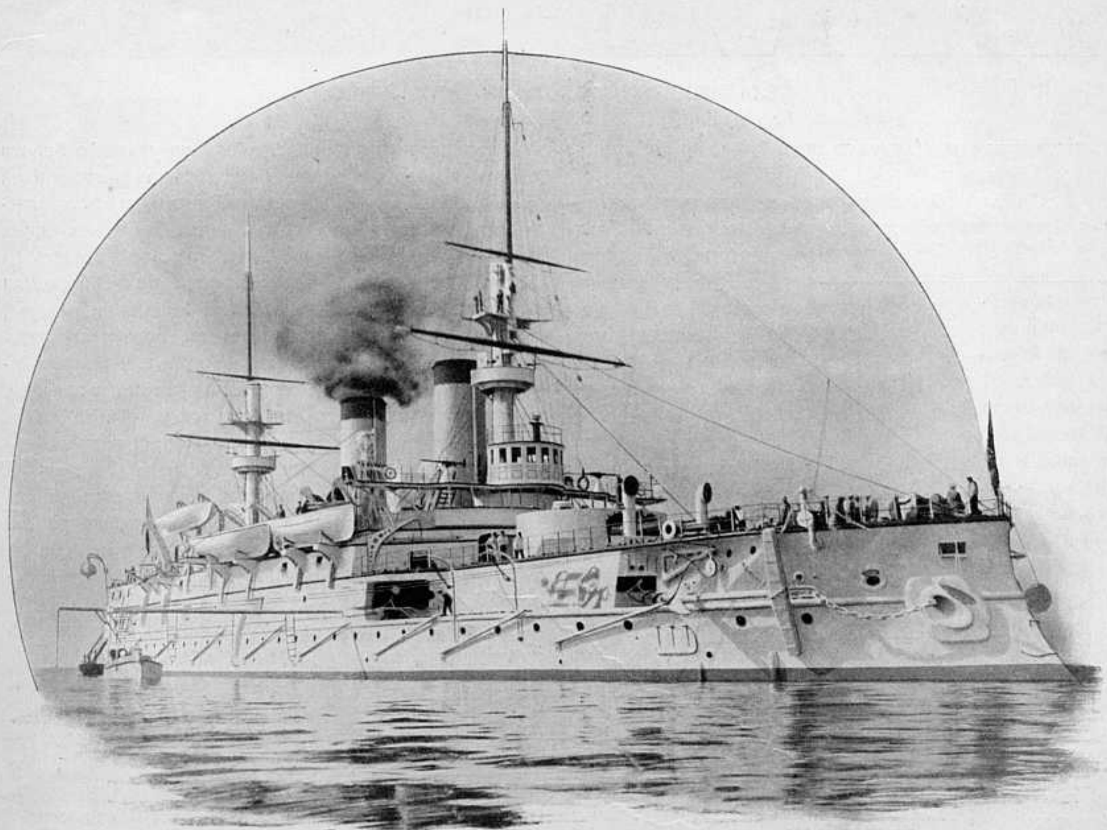
3-я ТИХООКЕАНСКАЯ ЭСКАДРА. БРОНЕНОСЕЦЪ «ИМПЕРАТОРЪ НИКОЛАЙ I».
