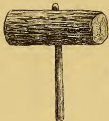
142. ábra. Furkó.
