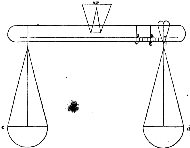
c. كفة الفضة ثابتة Bowl for Silver, fixed.
