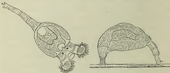
No. 21.— Philodina .
