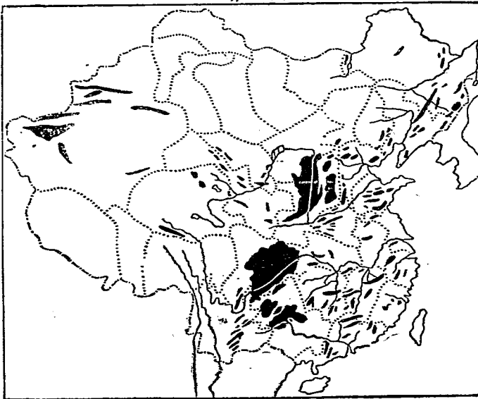
我國炭田分布
