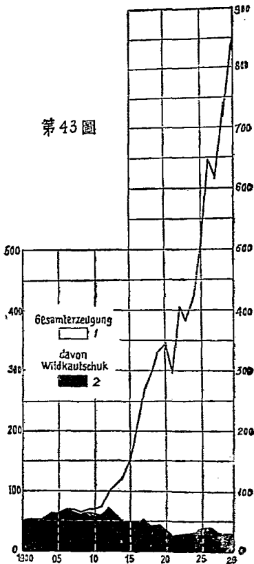
野生橡膠與栽培橡膠之產出關係 (1900-1929年)
