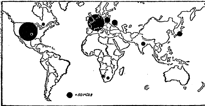
世界生鐵產地及產額
