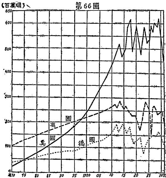
世界石炭主要出產國及產量(1870-1931)
