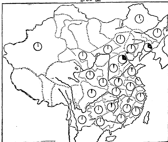
1931 我國各省煤產比較(百分比)
