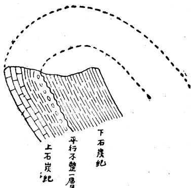
雲南東部地質剖面圖 第二
