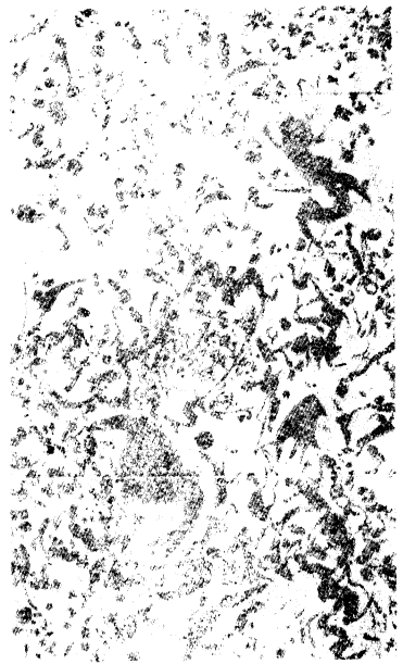
石化蟲葉三 圖二十第
