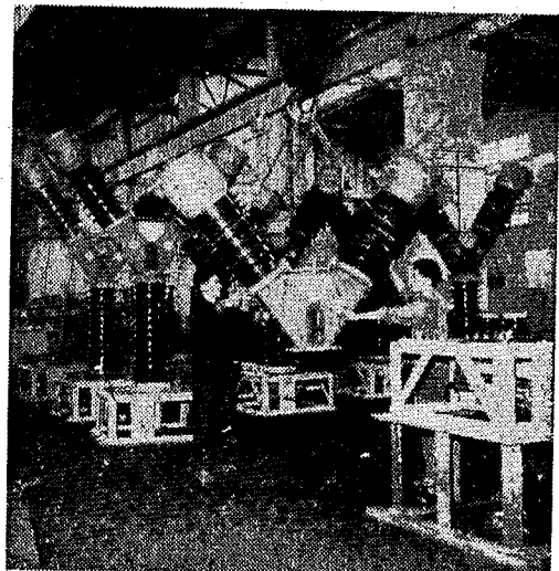
湖南开关厂七年间工人以大庆人为榜样，树雄心立壮志，积极生产十一万伏少油断路器，支援农业建设。这是他们正在总装十一万伏少油断路器。 湖南开关厂宣传组供稿
