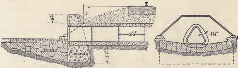
Fig. 40. C. P. R. Triangular Concrete Pipe.
