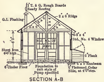
SECTION A-B
