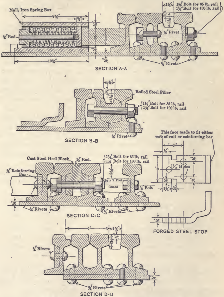
Fig. 69. P. R. R. Standard Spring Rail Frog.
