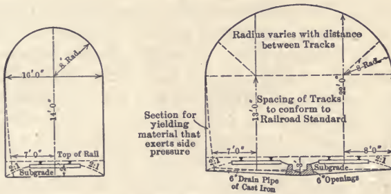
Fig. 1. A. R. E. A. Tunnel Clearances.
