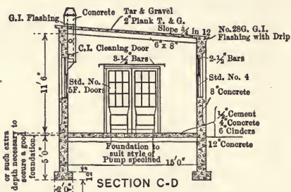
SECTION C-D
