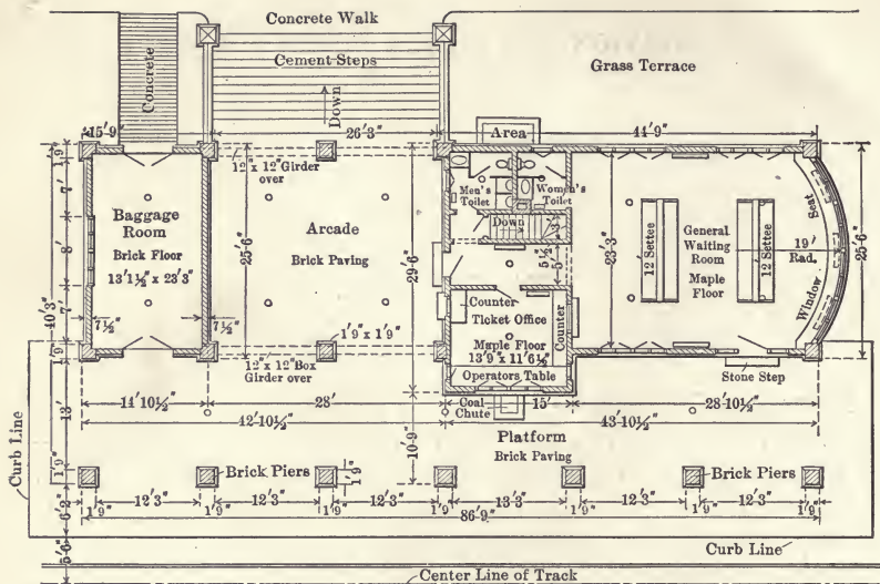
Fig. 129. Floor Plan, I. C. R. R. Station.
