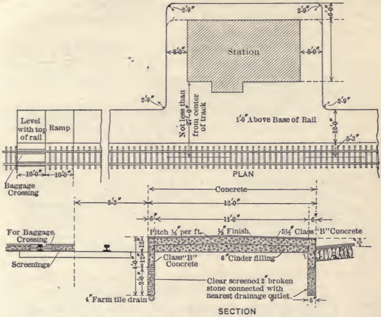
Fig. 187. N. Y. C. & H. R. R. R. Concrete Station Platform.
