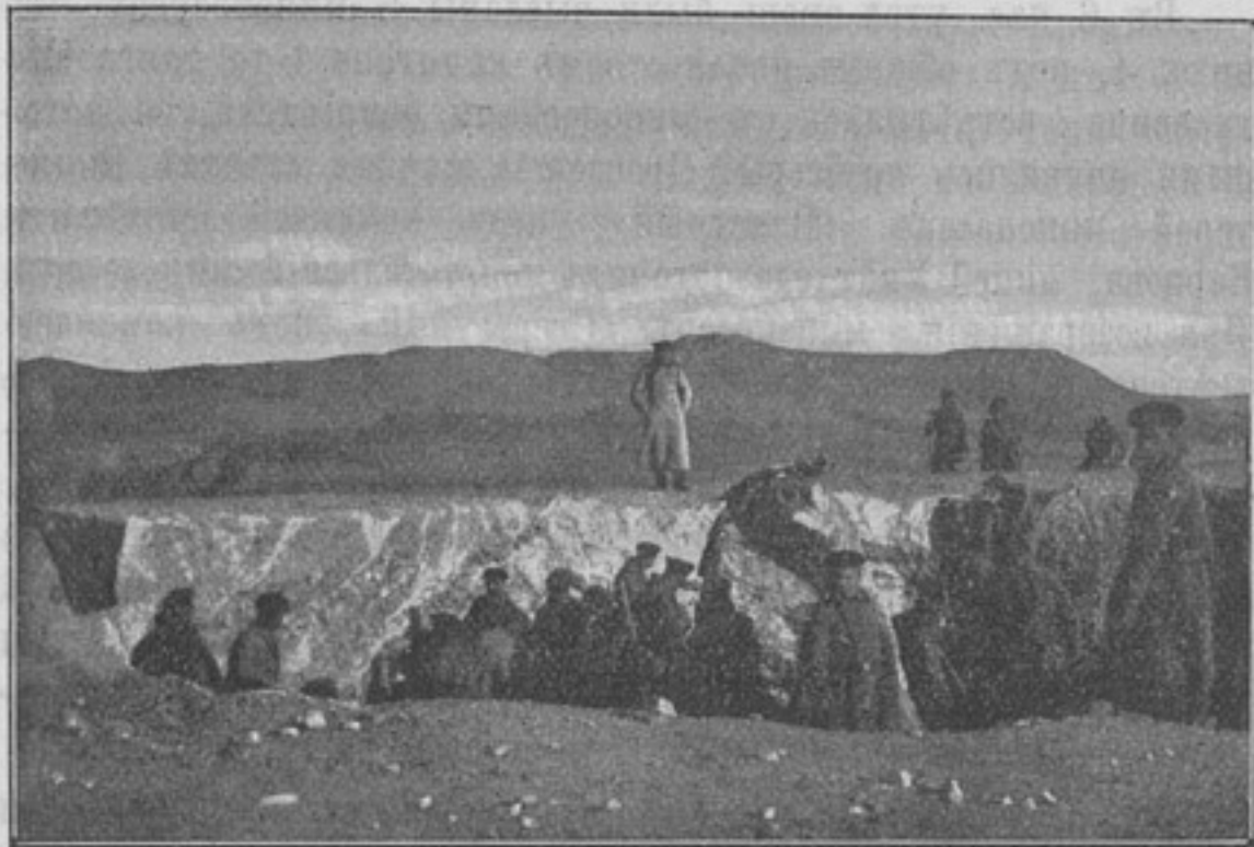
Портъ-Артуръ. Работы въ скаль (приготовленіе «постелей» для пушекъ).
