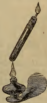
Burning Cyanogen.
