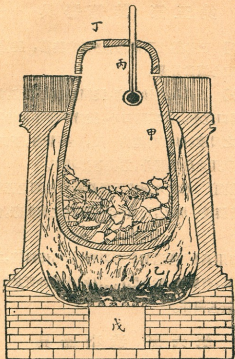
甲 坩 場 乙 爐 度 丙 溫 計 丁 氣 孔 戊 火 門 第二圖 石膏燒窯
