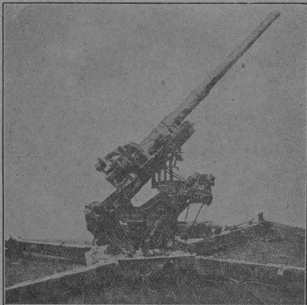
英國用以防守倫敦之新式高射砲，每分鐘能發射廿五發，高角射程達五英里半。
