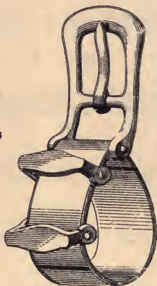
“Economy” Shaft Tug.
