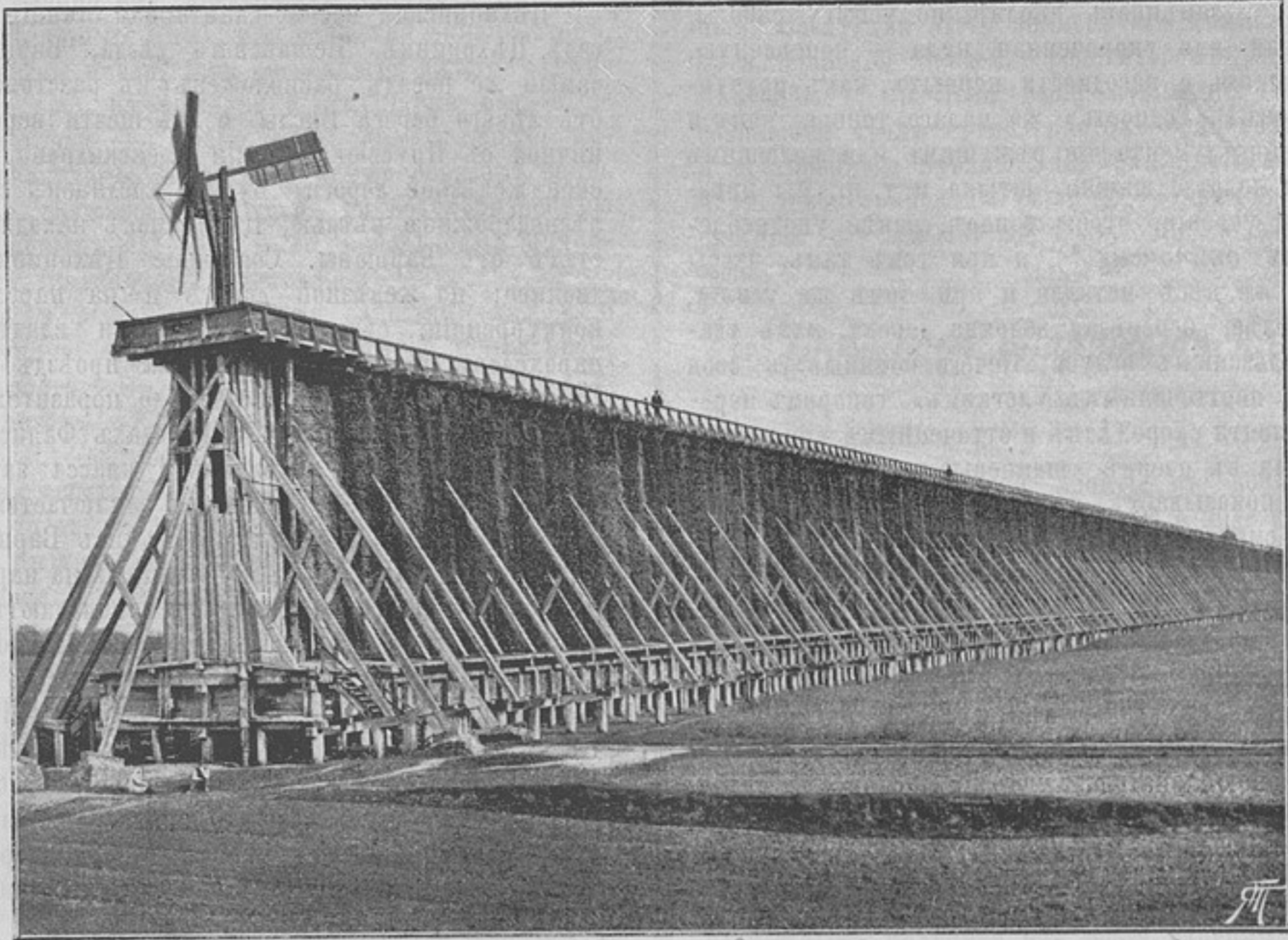
Градиря № 1, служащая для градировація трехпроцентной солянки.
