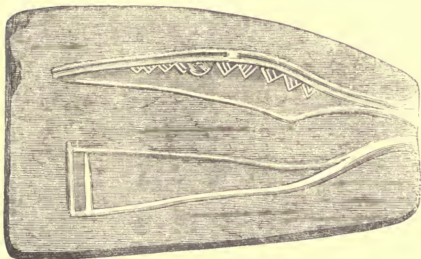
210. Form af sten för gjutning af två bronsknifvar. På stenslifvans andra sida är en form för fyra bronsågar. Sk. \frac{1}{2} .
