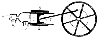
第四圖 汽油機構造
