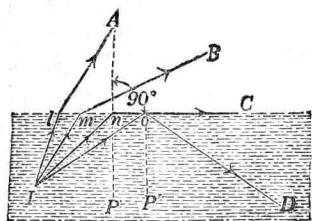
由空氣下水面之入射光線，其入射角為臨界角，普通稱某物質之臨界角為若干度者，均指光線由該物質進入空氣而言，故臨界角之定義可簡
