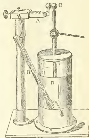
FIG. 1.—Lane's Jar.
