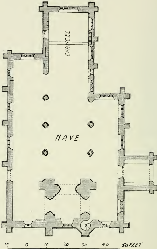
94. EWERBY
