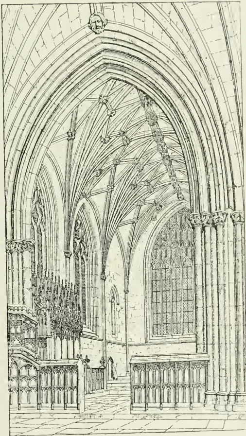
195. CHANCEL, NANTWICH
