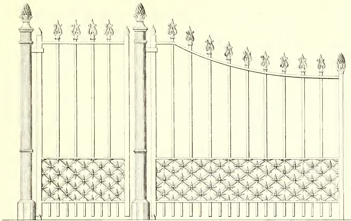
Op \frac{1}{20} der ware grootte. Schaal van 5 duim pr El.
