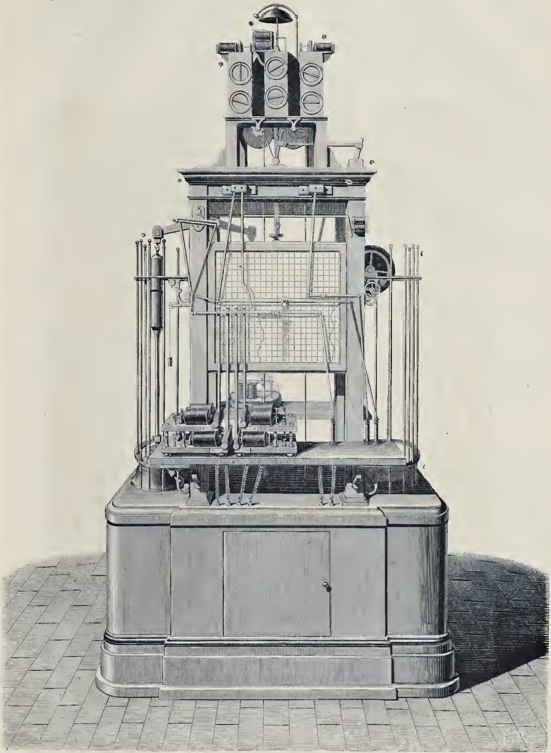
[LE METÉOROGAPHE DU P. SECCHI (Grand Prix). — Dessin de M. Noë.]
