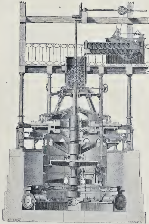
MACHINE A AGGLOMERER LA HOUILLE, de M. Félix Dehaynin (Médaille d'or.)
