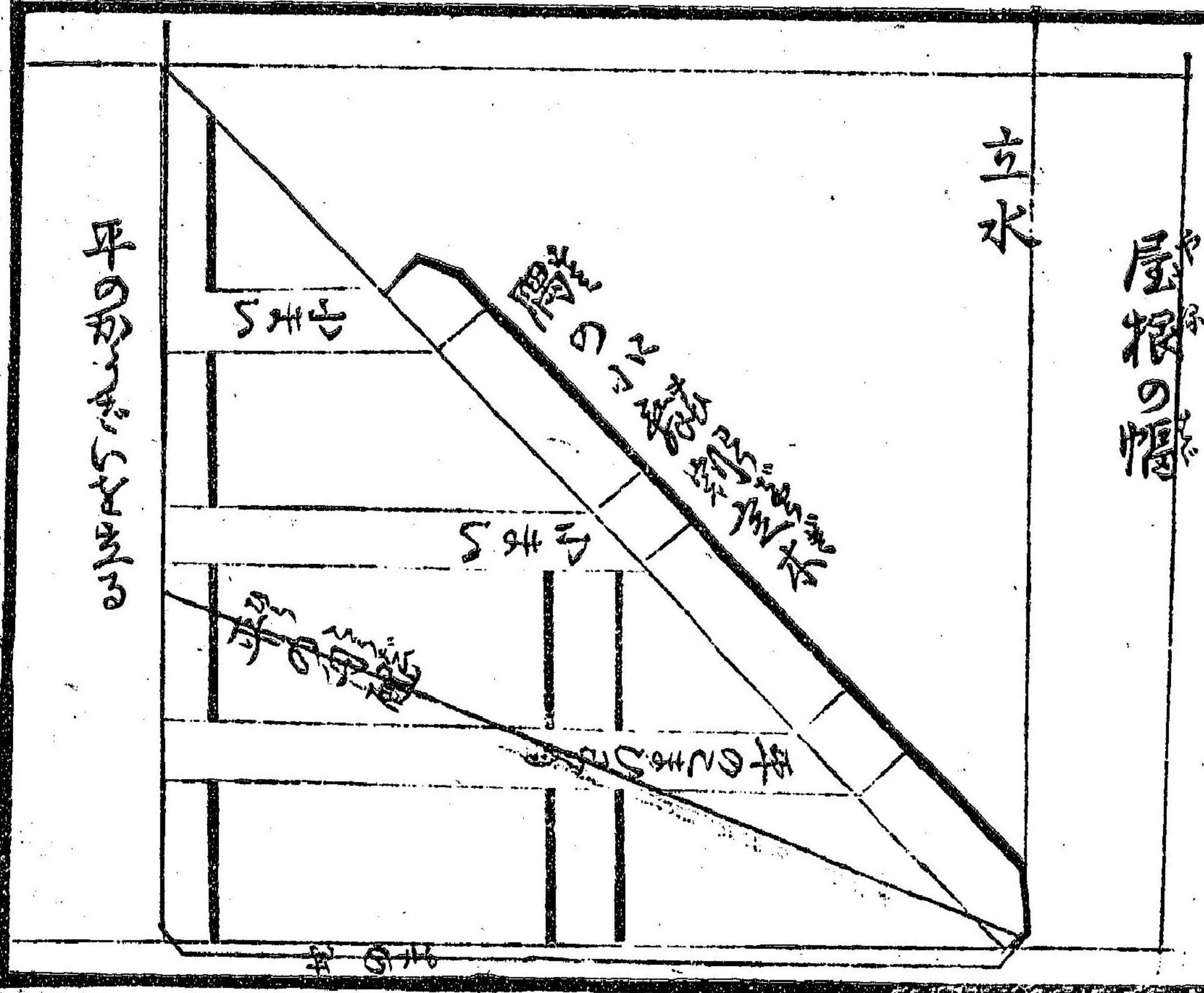
隅平小舞部の圖
