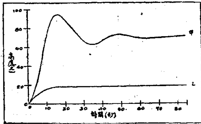
搖 動 之 機 行 飛 (圖 四 第)
