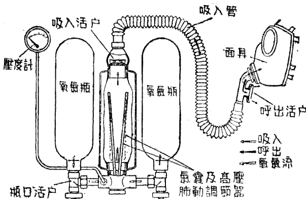
壓縮氧氣面罩
