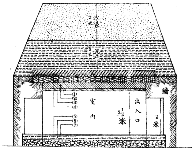
地下室立視圖
