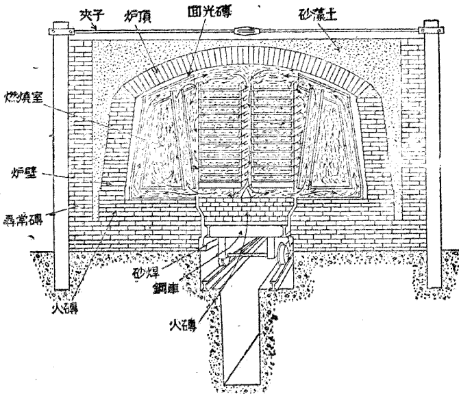
屈拉斯爾隧道窯
