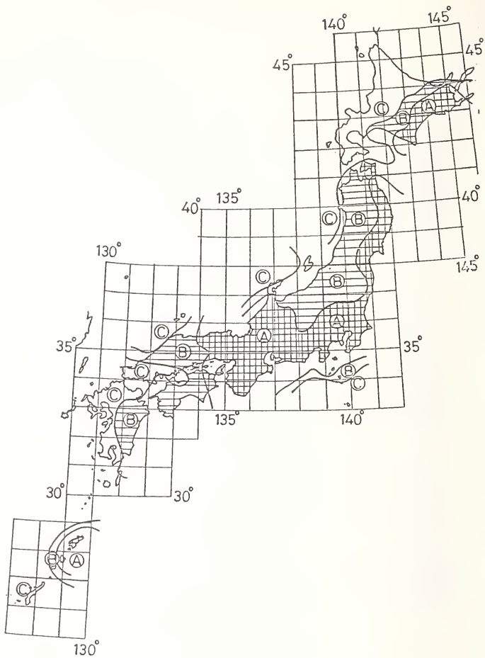
Fig. 4.1. Seismic Zoning
