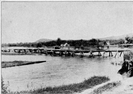
Мостъ черезъ Итунхэ у Люхэсана.
