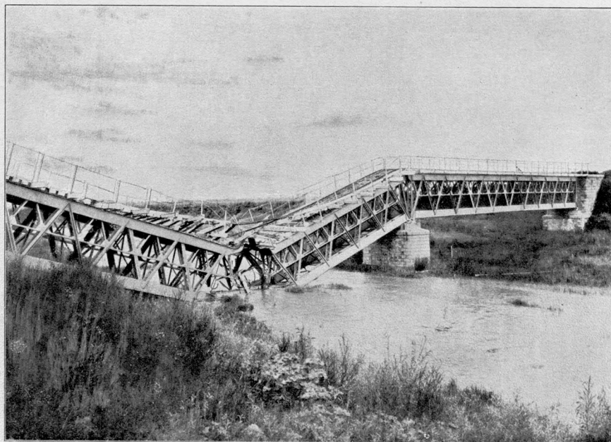
Разрушенные ж. д. мосты.
