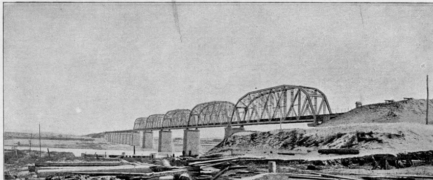
Железнодорожный мостъ черезъ р. Сунгари у Лошагоу.
