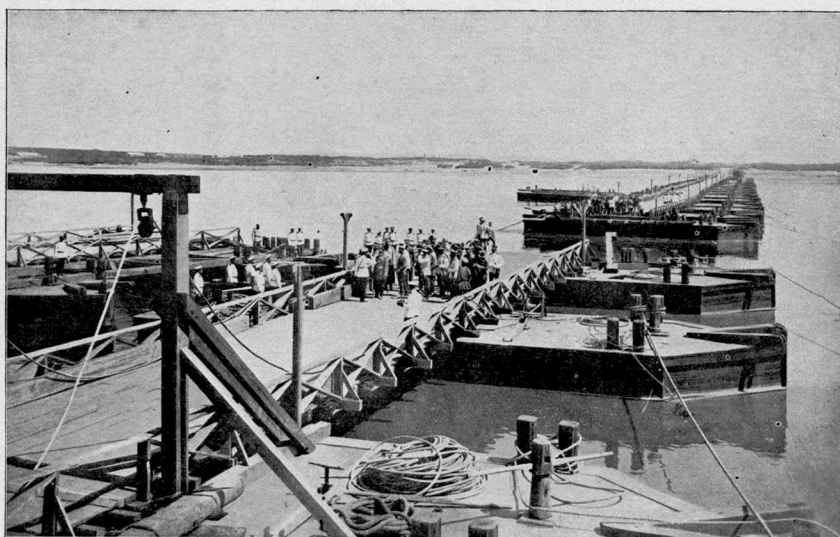
Понтонный мостъ, наведенный через р. Сунгари у Лошагоу.
