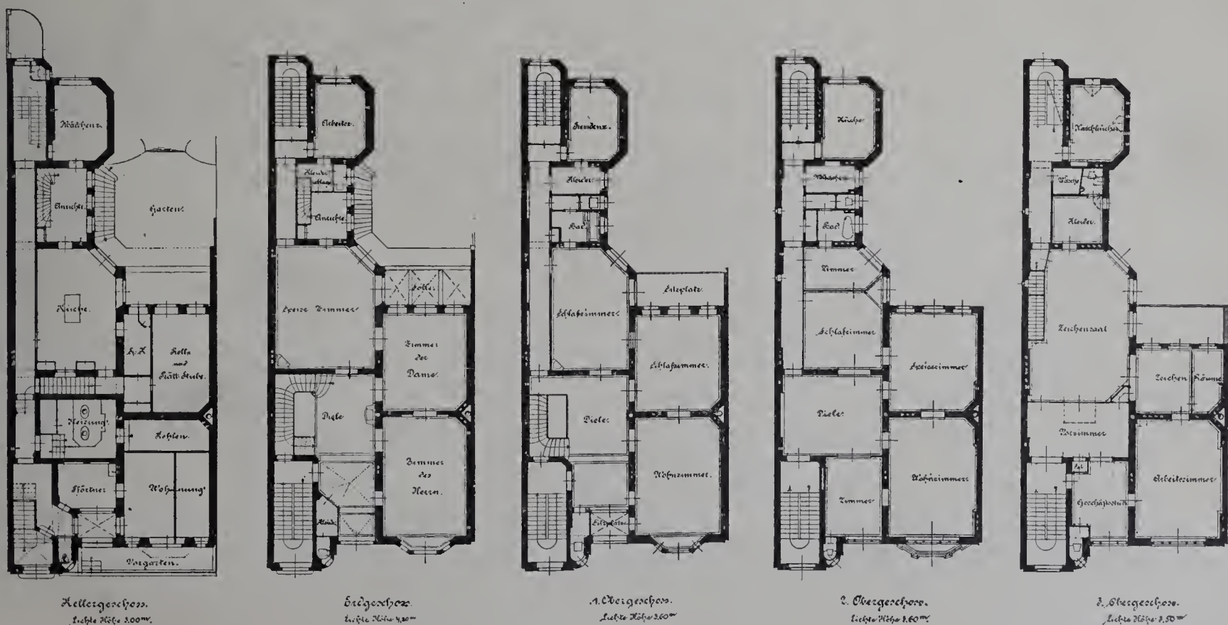
Wohnhaus W. Martens in Charlottenburg.
