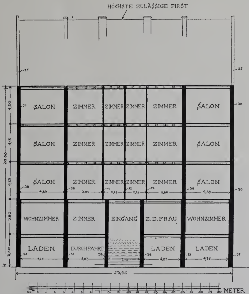
Ansicht des Hauses ohne seine Strafsenwand.
