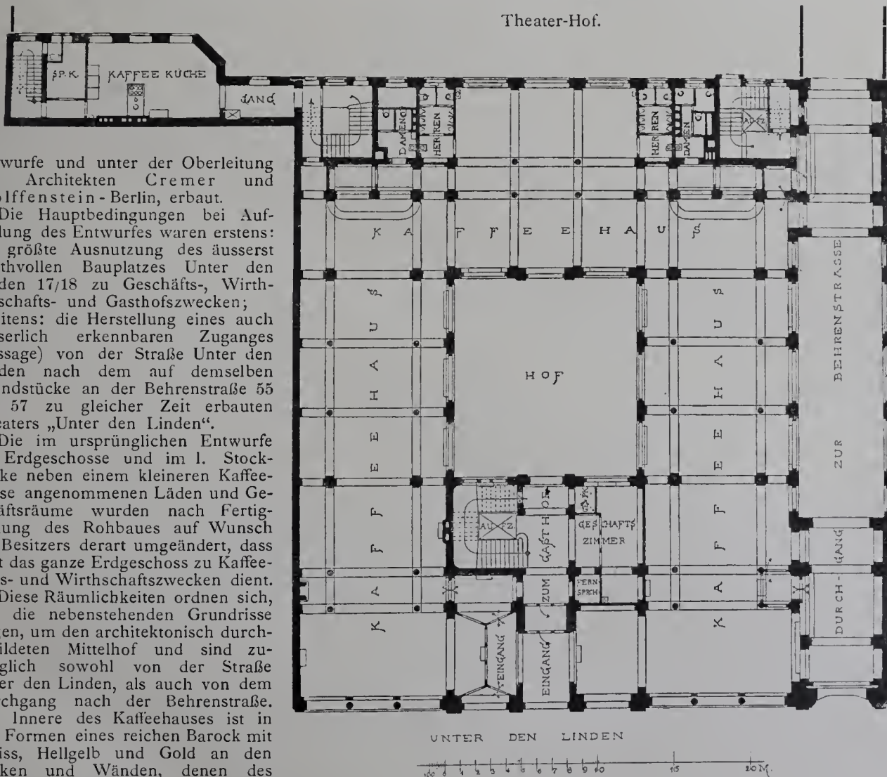
Der Gasthof „Unter den Linden“ in Berlin.
