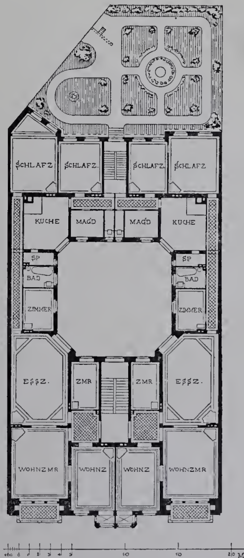
Wohnhaus in Berlin, Tauenzienstr. 12.
