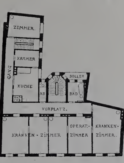
GRUNDRISS vom I. STOCK - KRANKENRÄUME.
