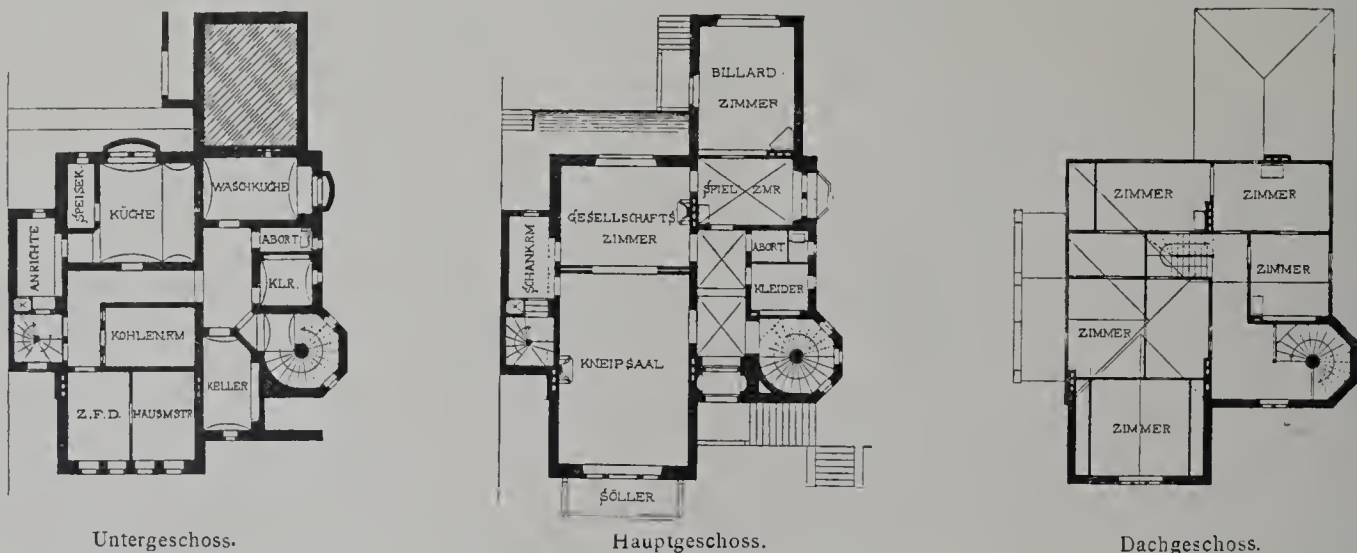
Das Forstkasino in Eberswalde.
