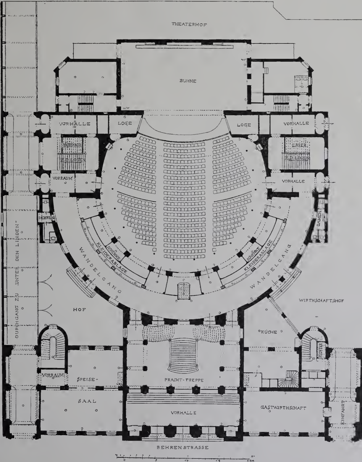
Das Theater „Unter den Linden“ in Berlin, Behrenstr. 55—57.
