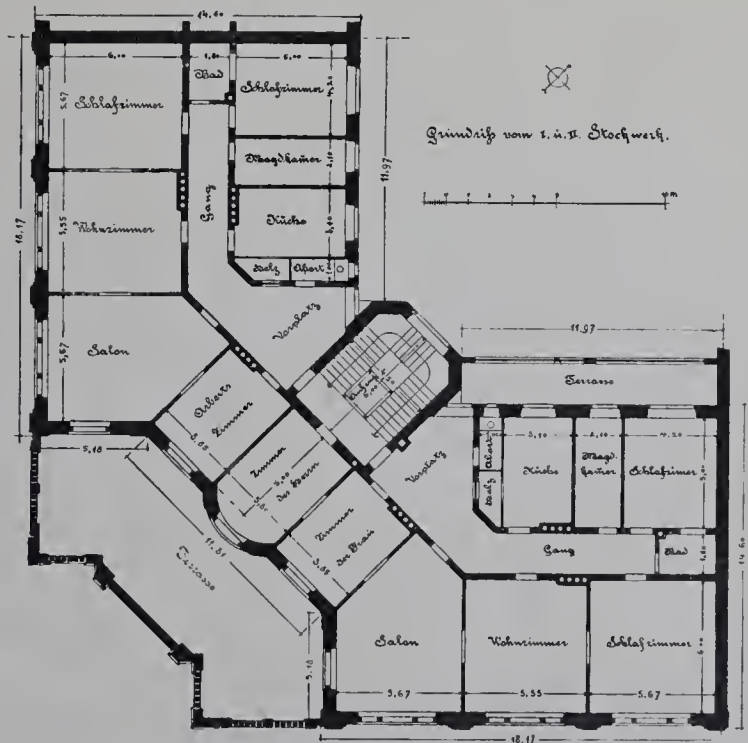
Wohn- und Geschäftshaus in München, Zweibrückerstrasse.
