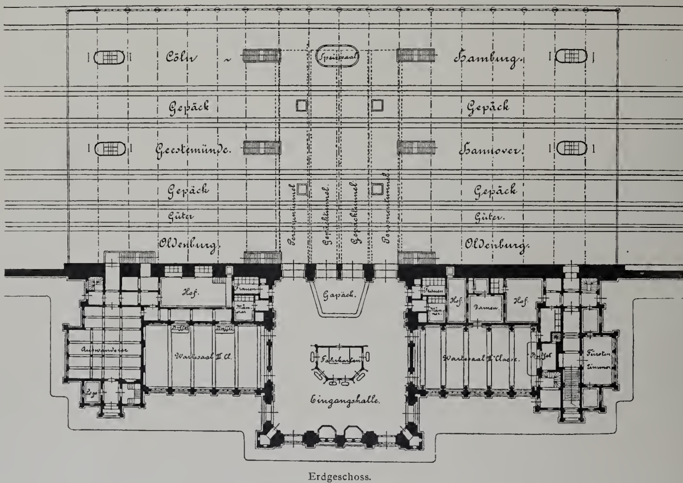
Das Empfangsgebäude des Bahnhofes in Bremen.
