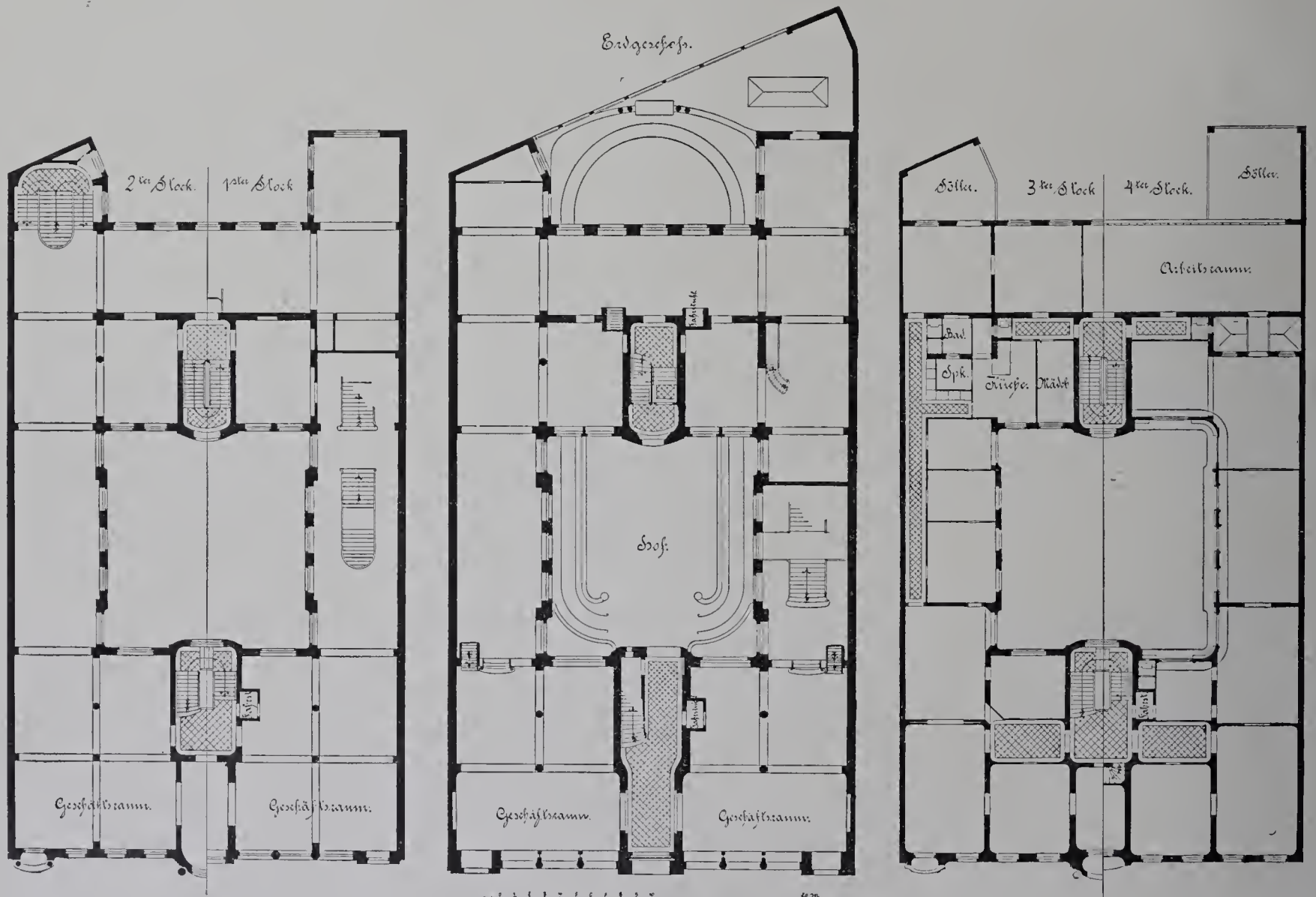
Kauf- und Wohnhaus Henckels in Berlin, Leipzigerstr. 117/118.
