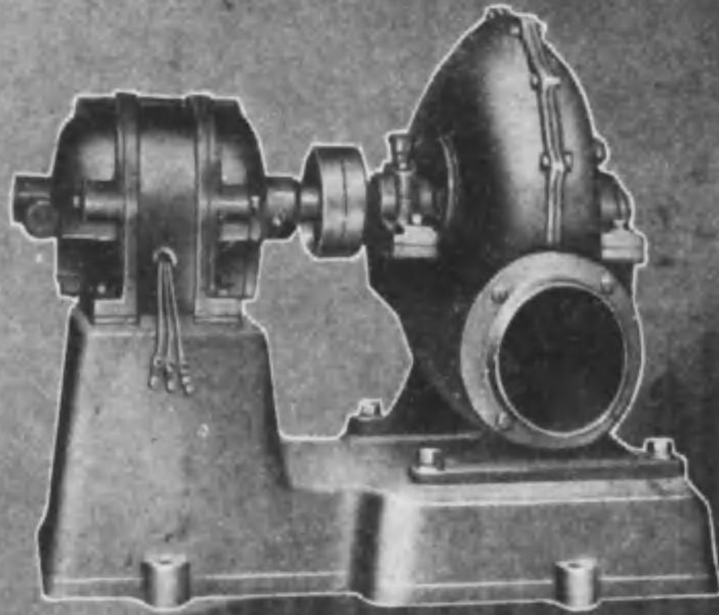
電動雜用送風機
