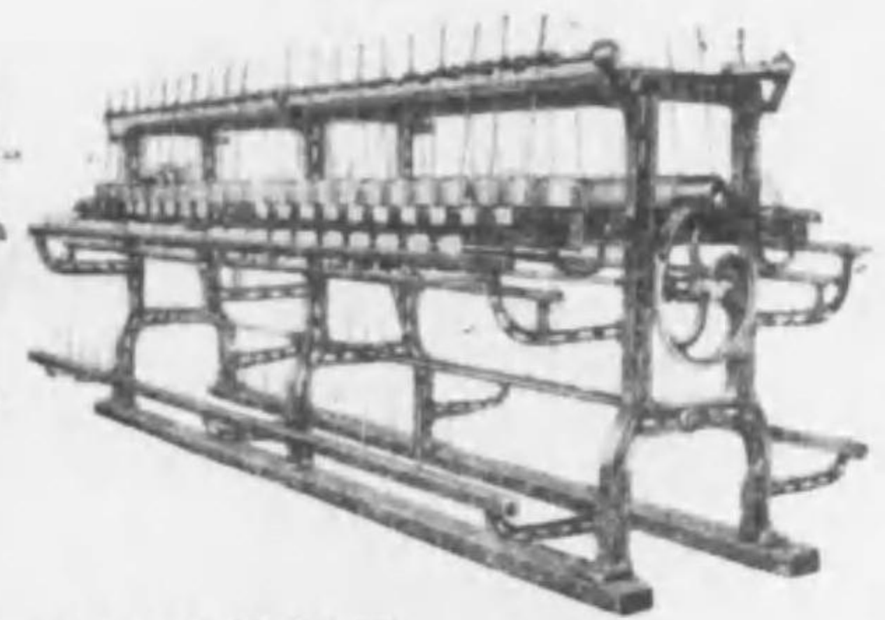
奥井式日型整經機
