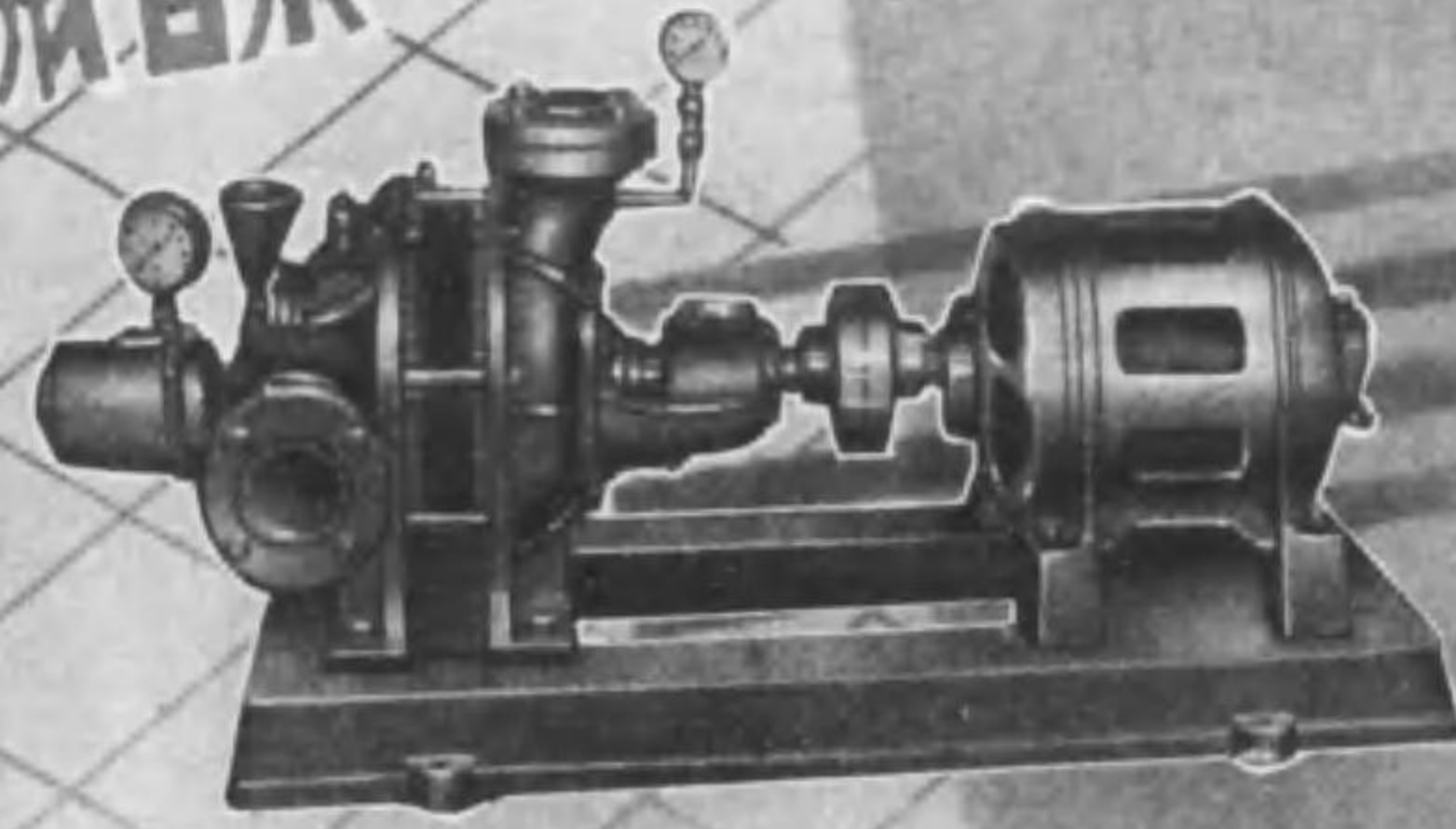
75hp 2段ターボポンプ
