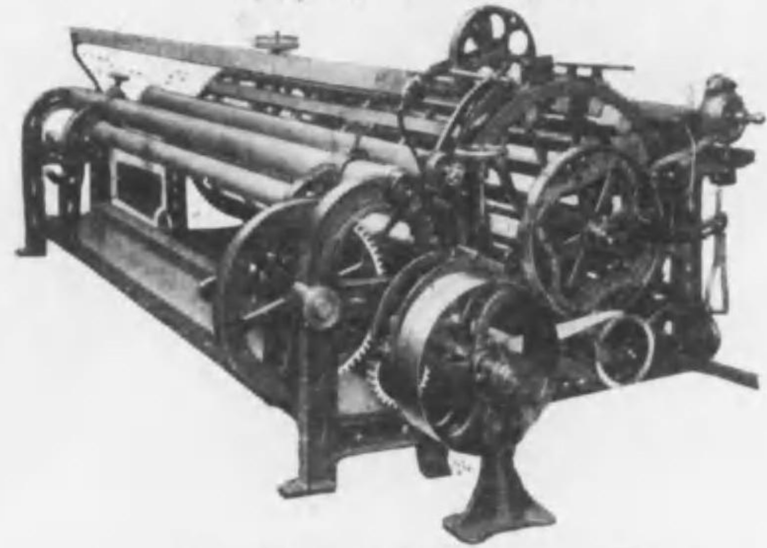
奥井式日型整經機
