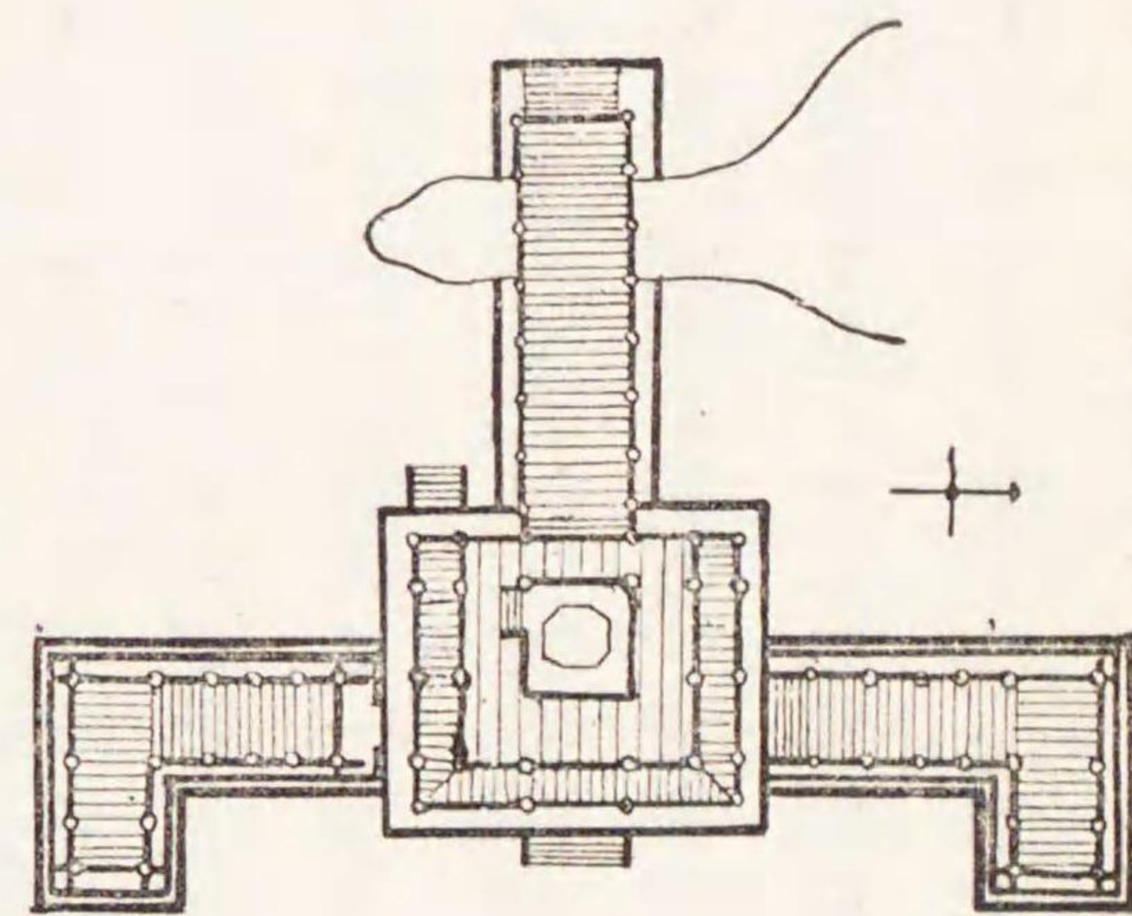
圖面平堂鳳凰 圖四十第
