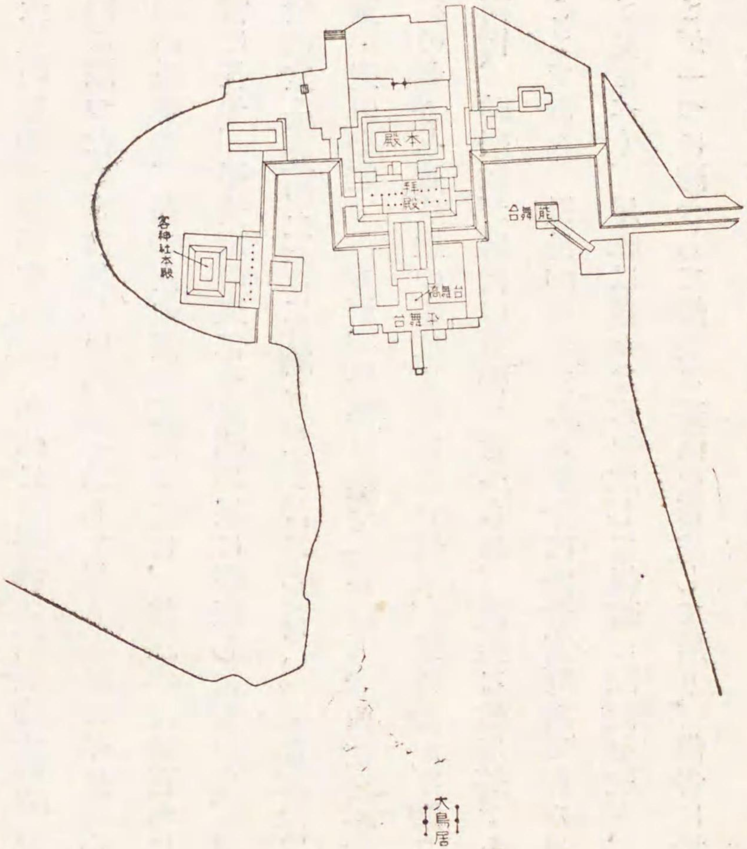
第七十圖 島神社平面圖
