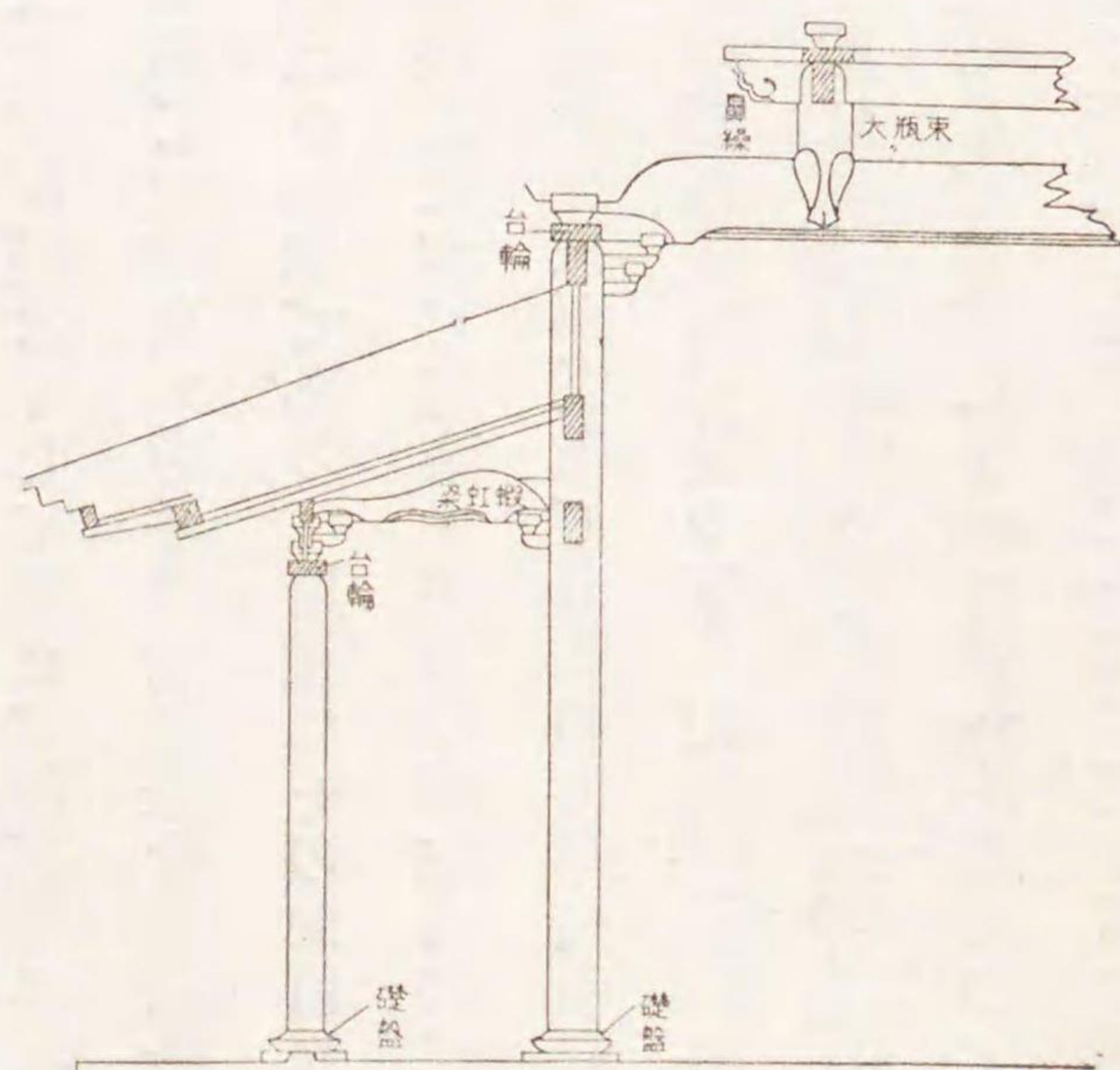
圖九十第 圓覺寺舍利殿建築圖
