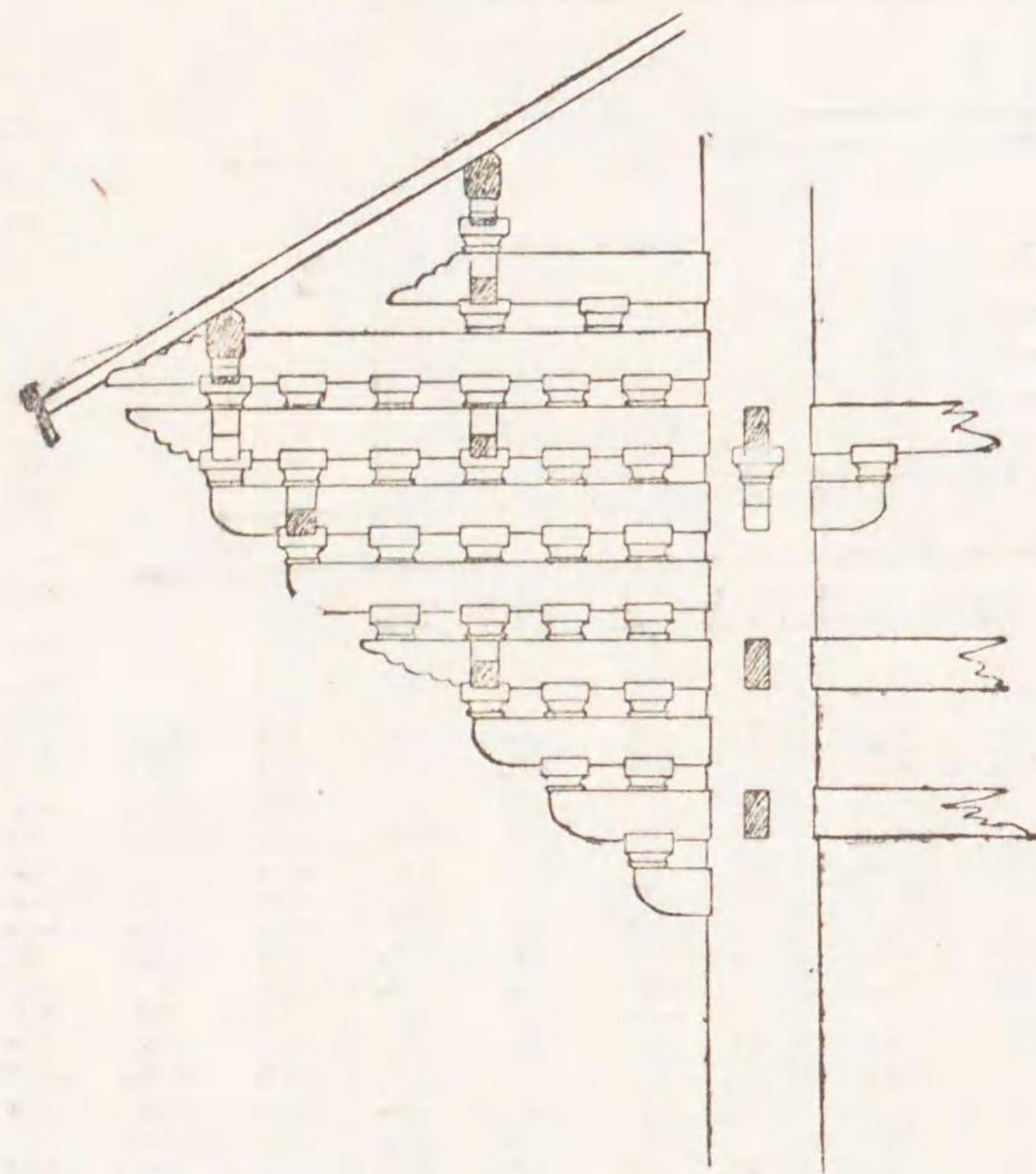
圖八十第 淨土寺七木手先組物 東大寺南大門
