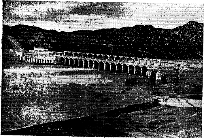
图为衡东县甘溪轮泵水电站全景。
