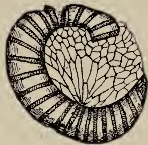
Fig. 38. — Sporange des quartz permien d'Autun, constitué comme ceux des Gleichéniées, grossi 35 fois.
