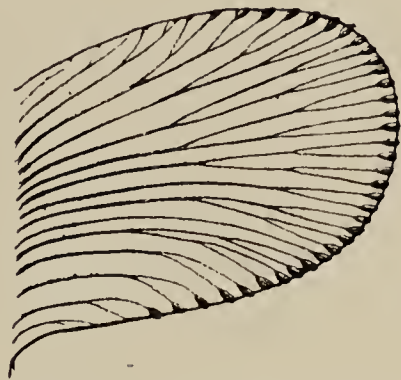
Fig. 74. — Odontopteris lingulata Goeppert (sp.), du Stéphanien. Pinnule fertile, grossie 4 fois (d'après Grand'Eury).
