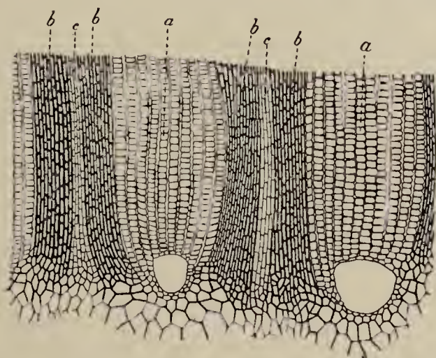
Fig. 109. — Calamodendron striatum Cotta (sp.), du Permien d'Autun. Coupe transversale, grossie, montrant deux coins ligneux : a, bois secondaire formé de trachéides rayées; b, bandes prosenchymateuses; c, rayons médullaires primaires (d'après Renault).
