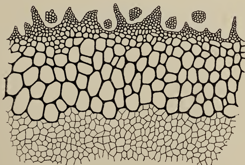
Fig. 124 — Lepidod. Harcourti Witham, du Houiller d'Angleterre. Coupe transversale montrant une partie de la moelle centrale et de l'anneau ligneux avec ses pointements trachéens et plusieurs faisceaux foliaires ; grossie 18 fois (d'après Williamson).
