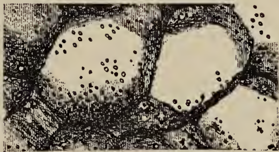
Fig. 12. — Micrococcus Guignardi Renault du Stéphanien de Saint-Étienne. Tissu cellulaire envahi par les Microcoques : très fortement grossi (d'après Renault).
