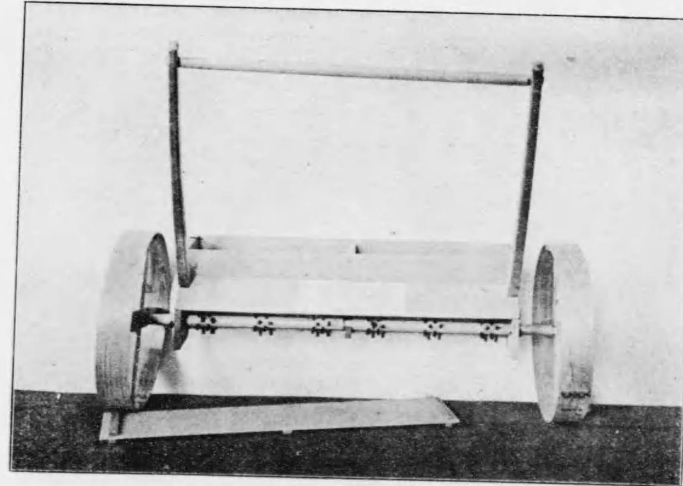
(類器種播) 圖二十三百第真寫
