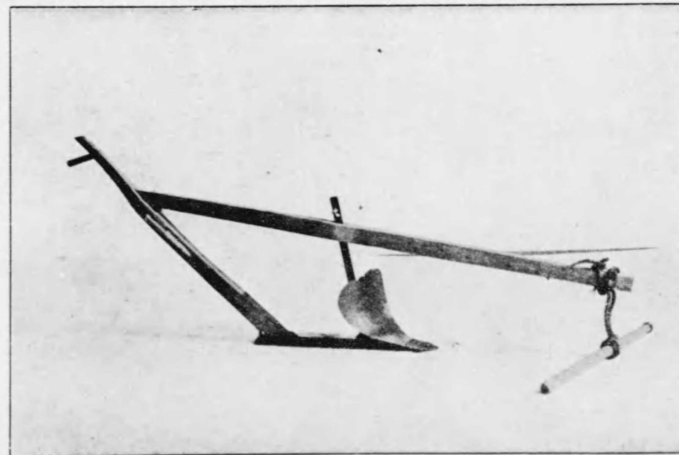
(類 犁) 圖二十三第真寫
