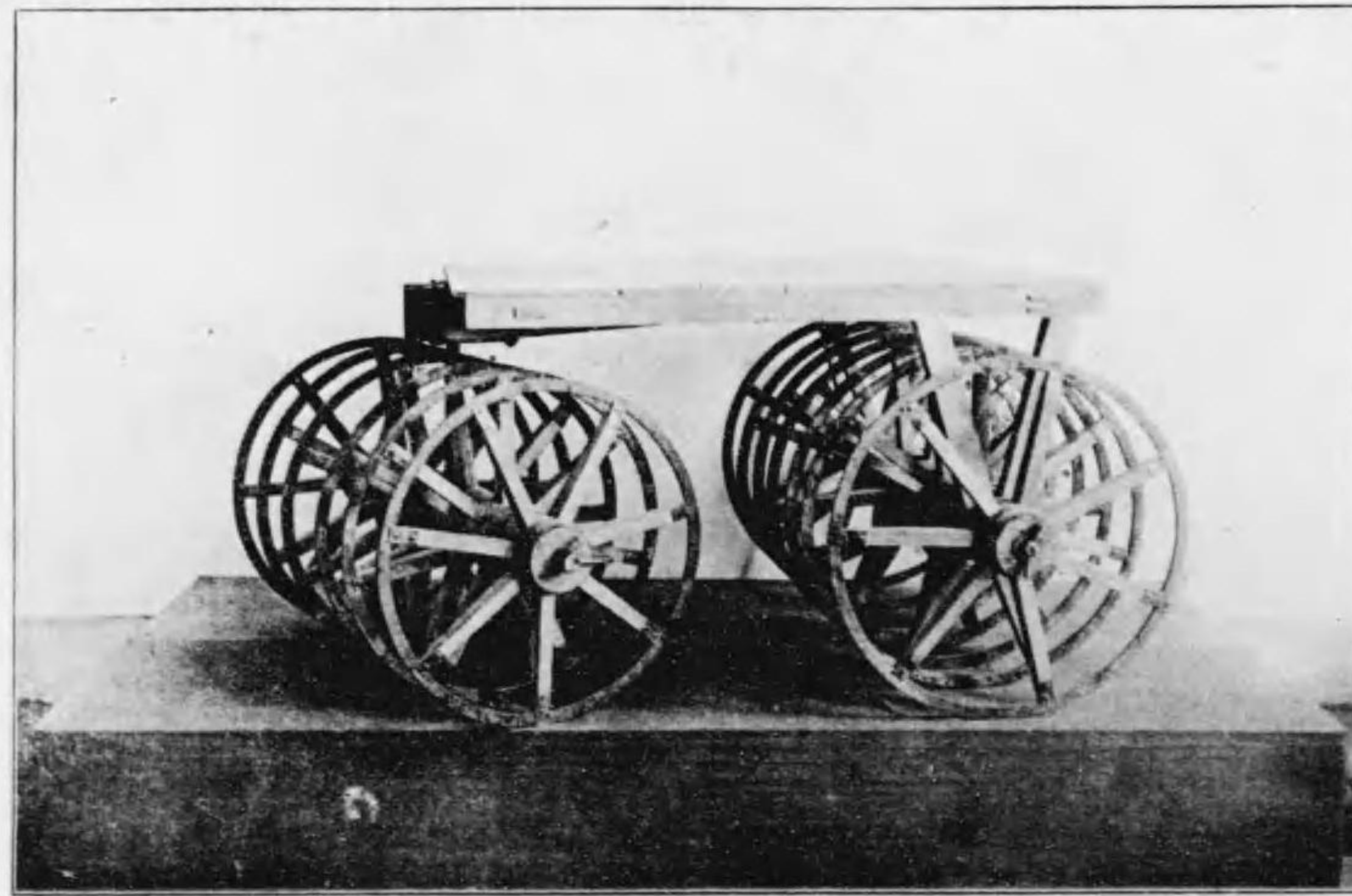
(類器土攪、器耙) 圖六十二百第真寫
