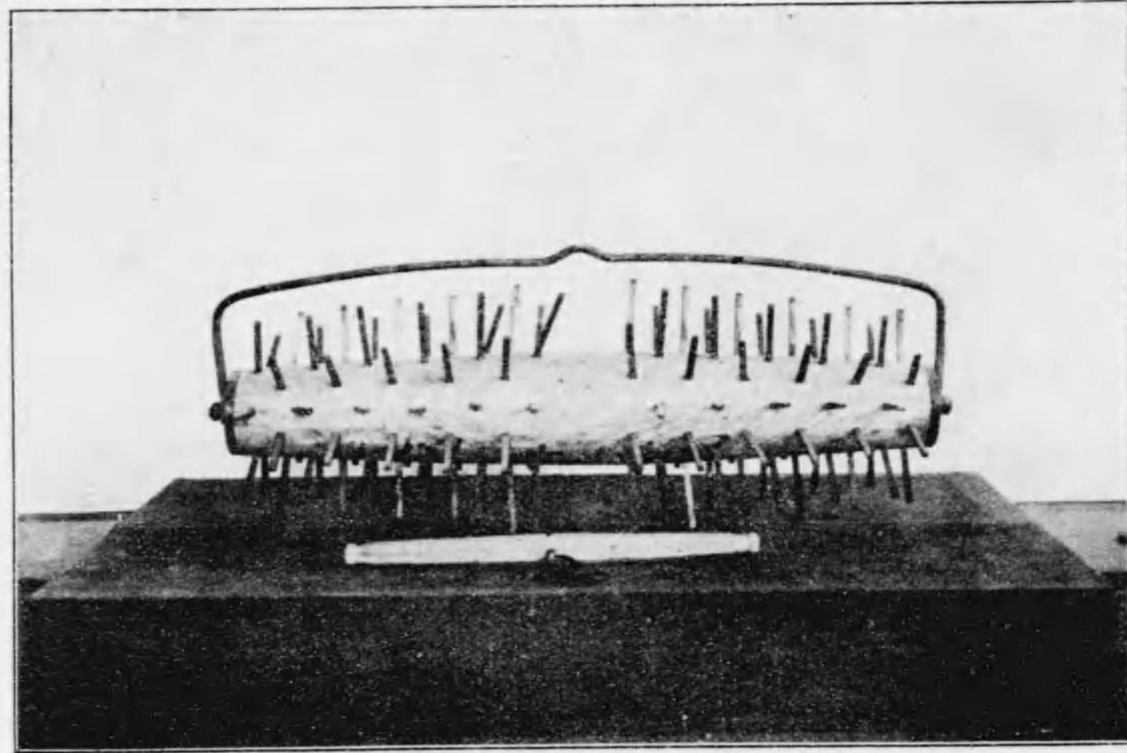
(類器土攪、器把) 圖一十二百第真寫
