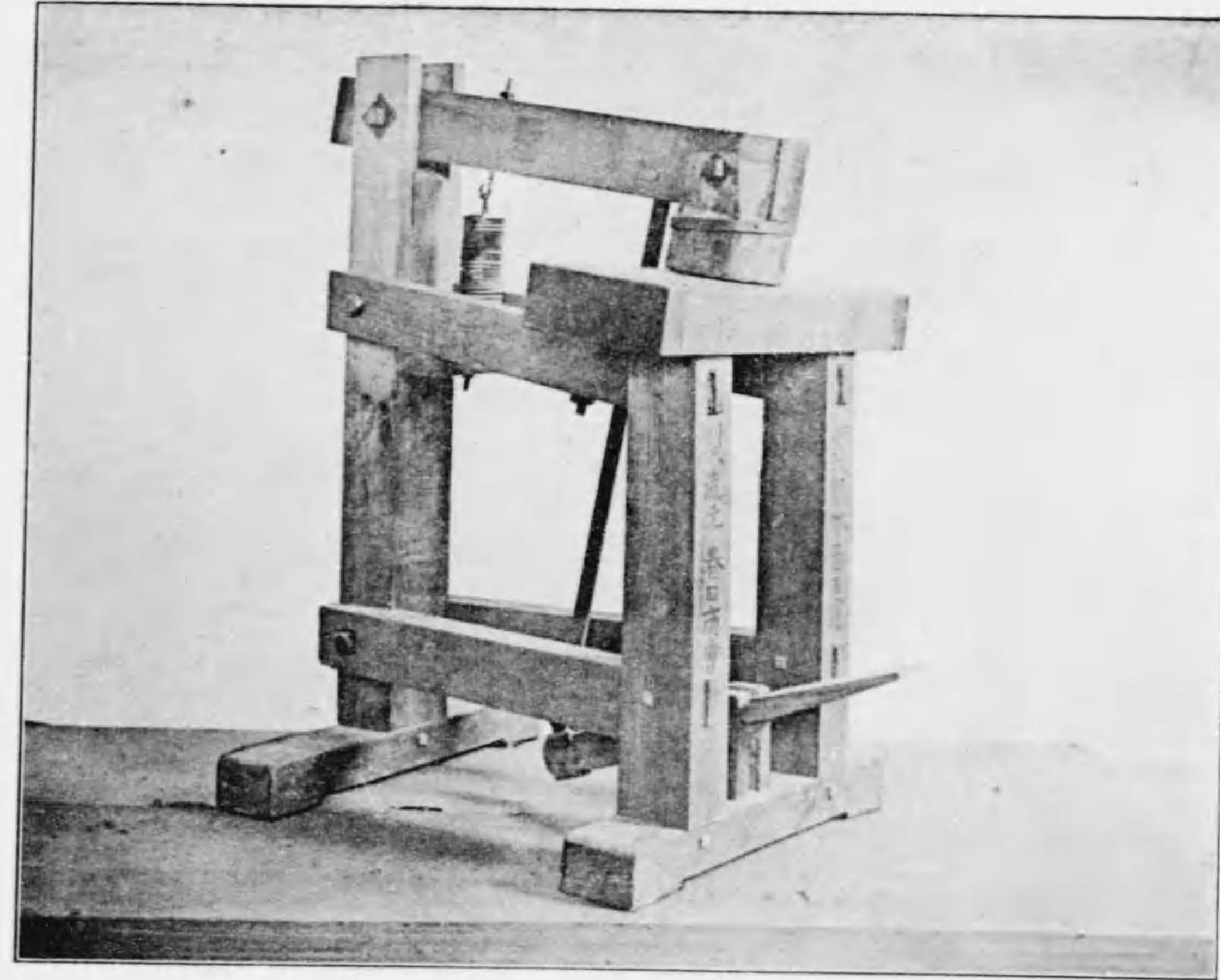
(類機打葉) 圖八十二百二第真寫
