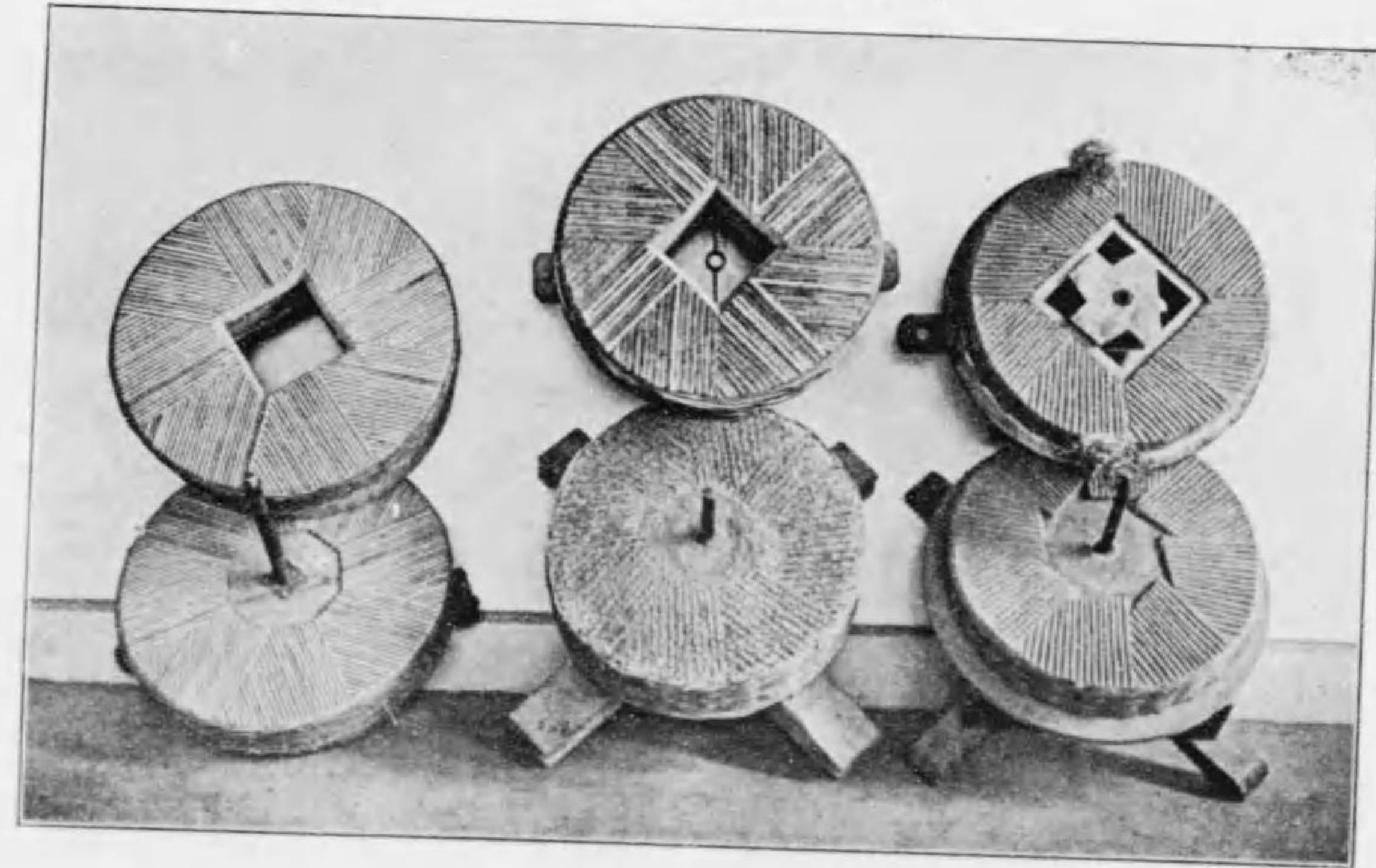
(類機摺穀) 圖四十八百第真寫
