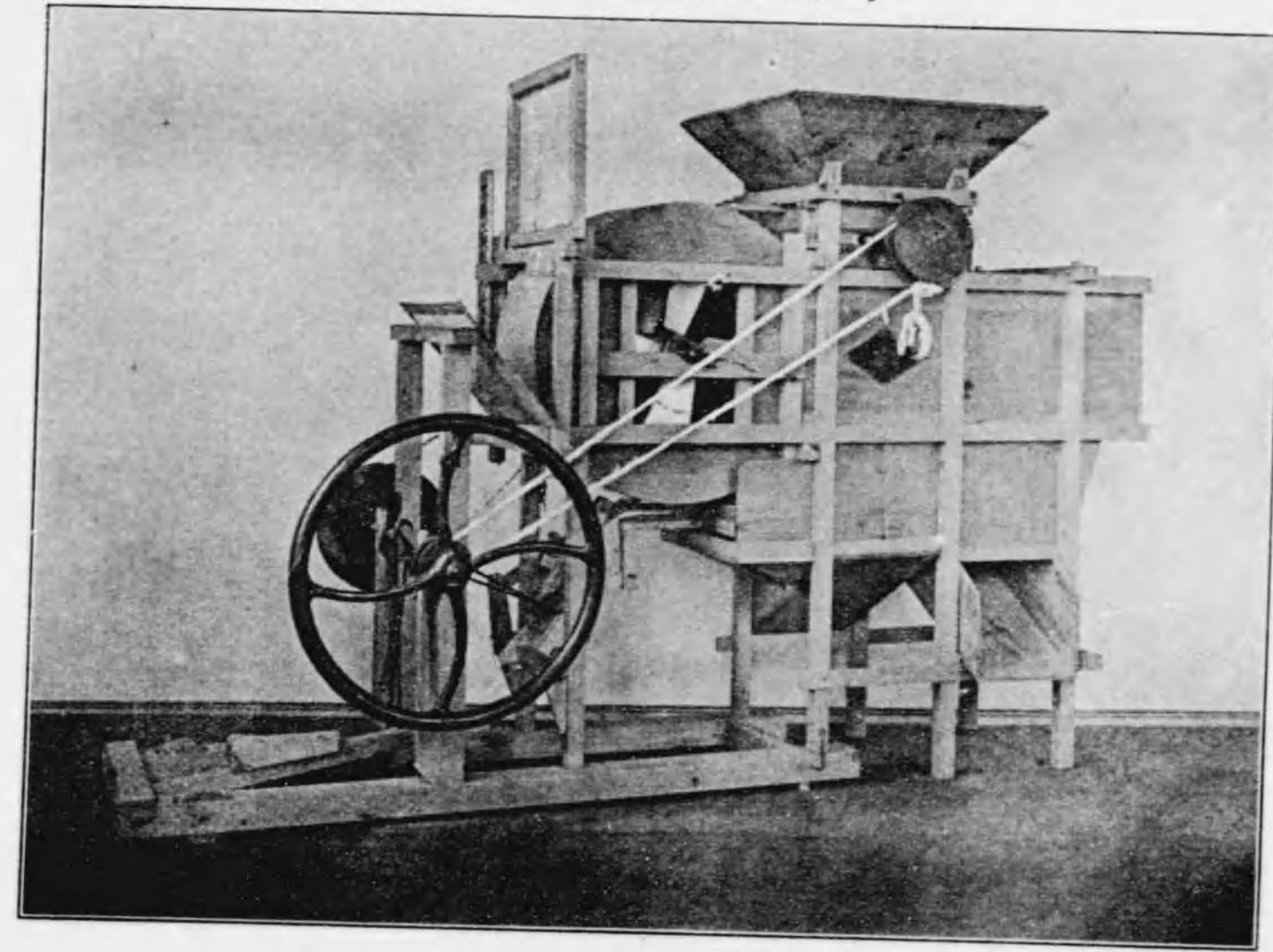
(類 箕 唐) 圖 五 十 九 百 第 真 寫
