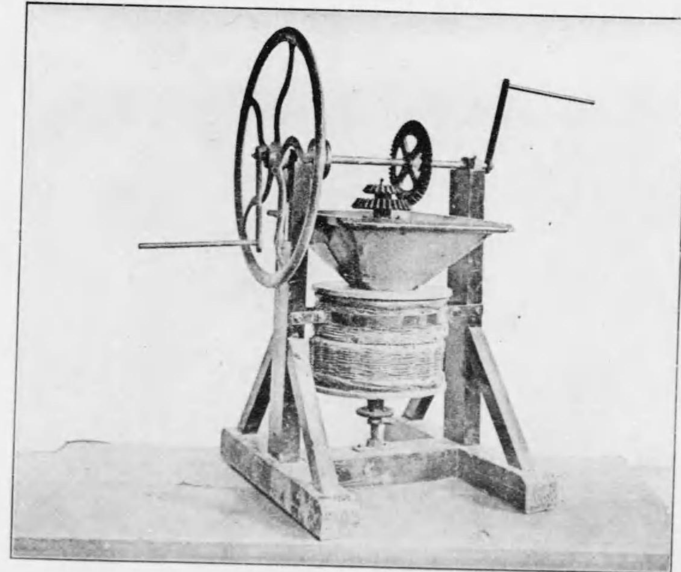
(類機擗穀) 圖八十八百第真寫
