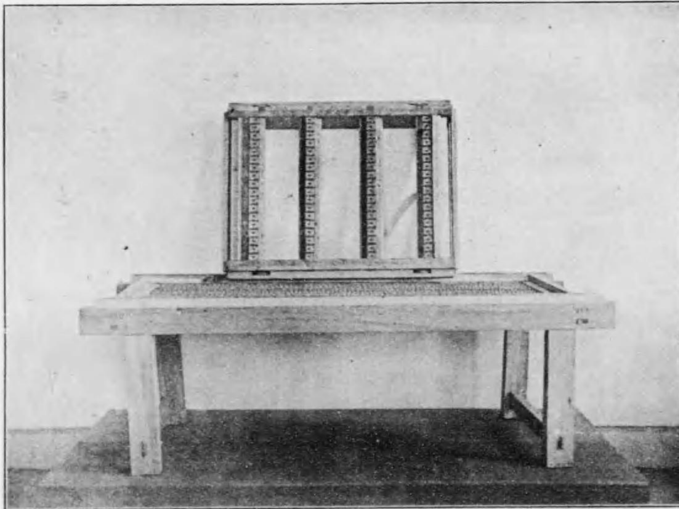
(類 機 粒 脫) 圖 八 十 七 百 第 真 寫
