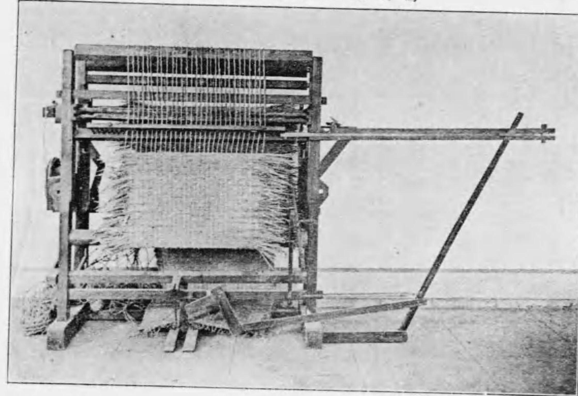
圖五十三百二第真寫 (類機蓬製)
