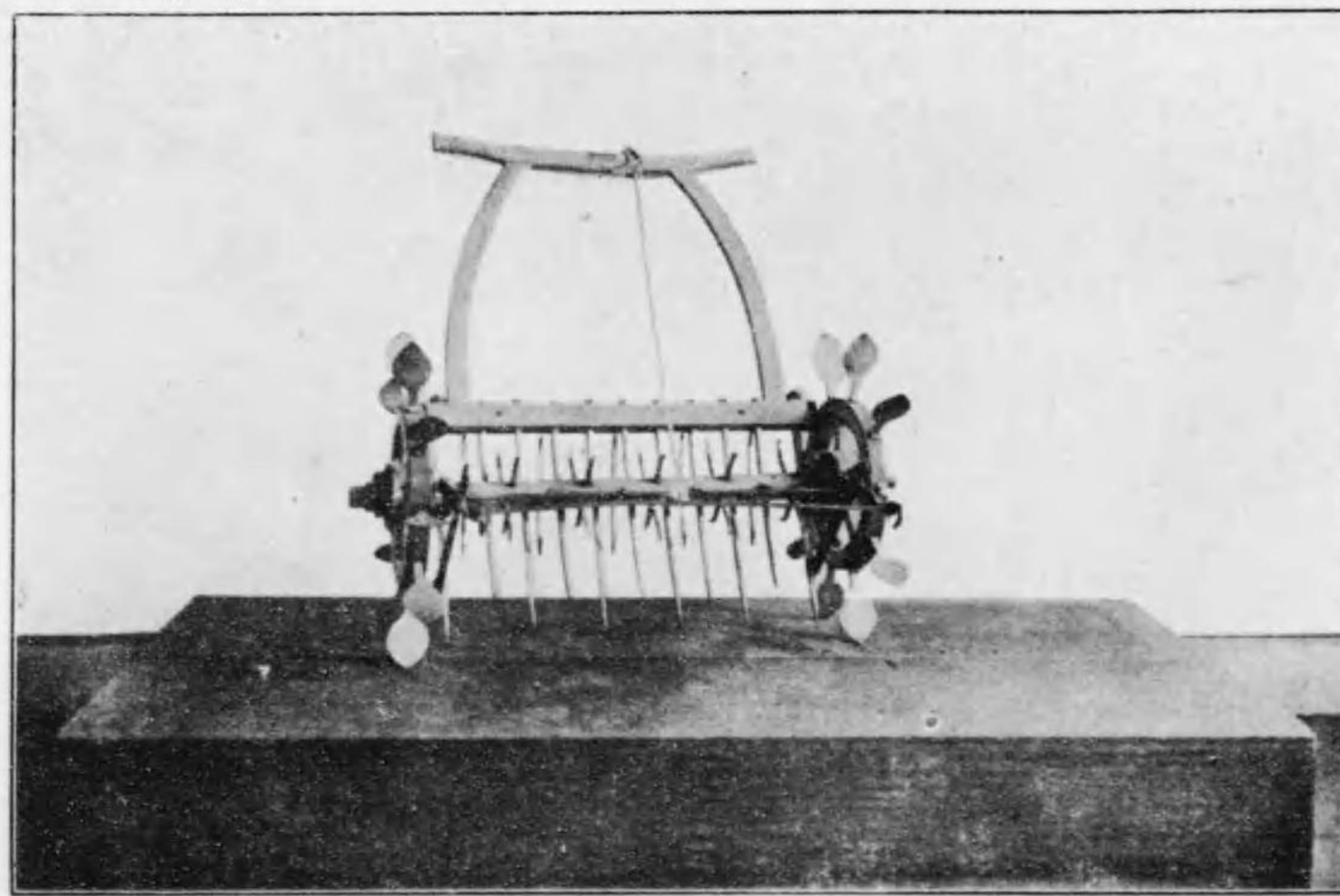
(類器土攪、器把) 圖八十百第真寫
