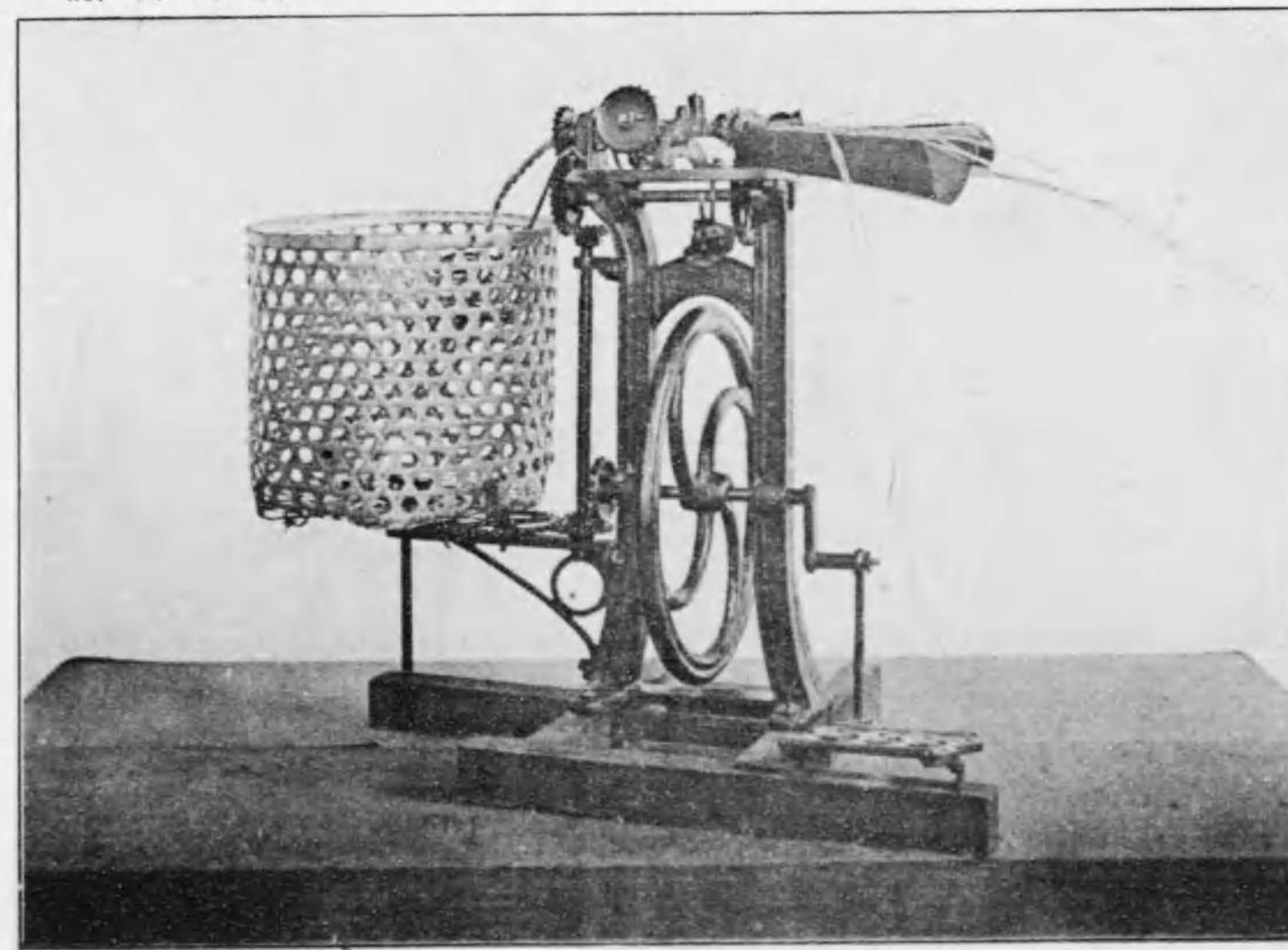
(類機繩製) 圖十三百二第真寫
