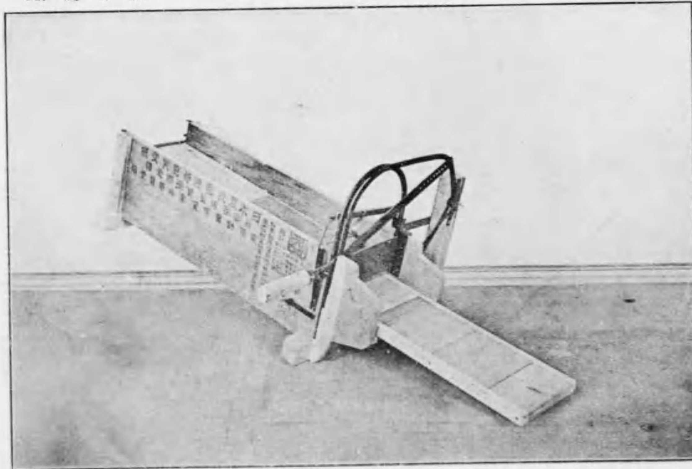
(類機切桑) 圖二百二第真寫
