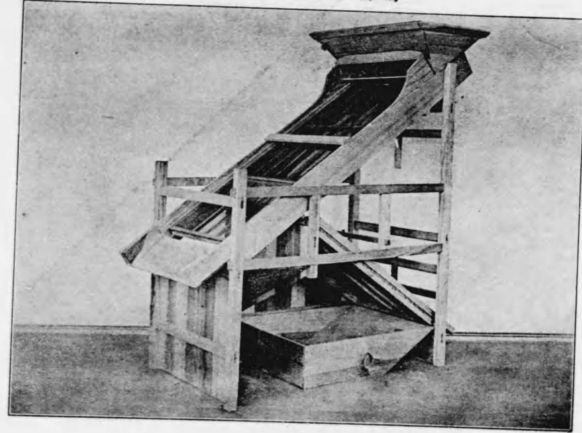
(類通石萬) 圖九十九百第真寫
