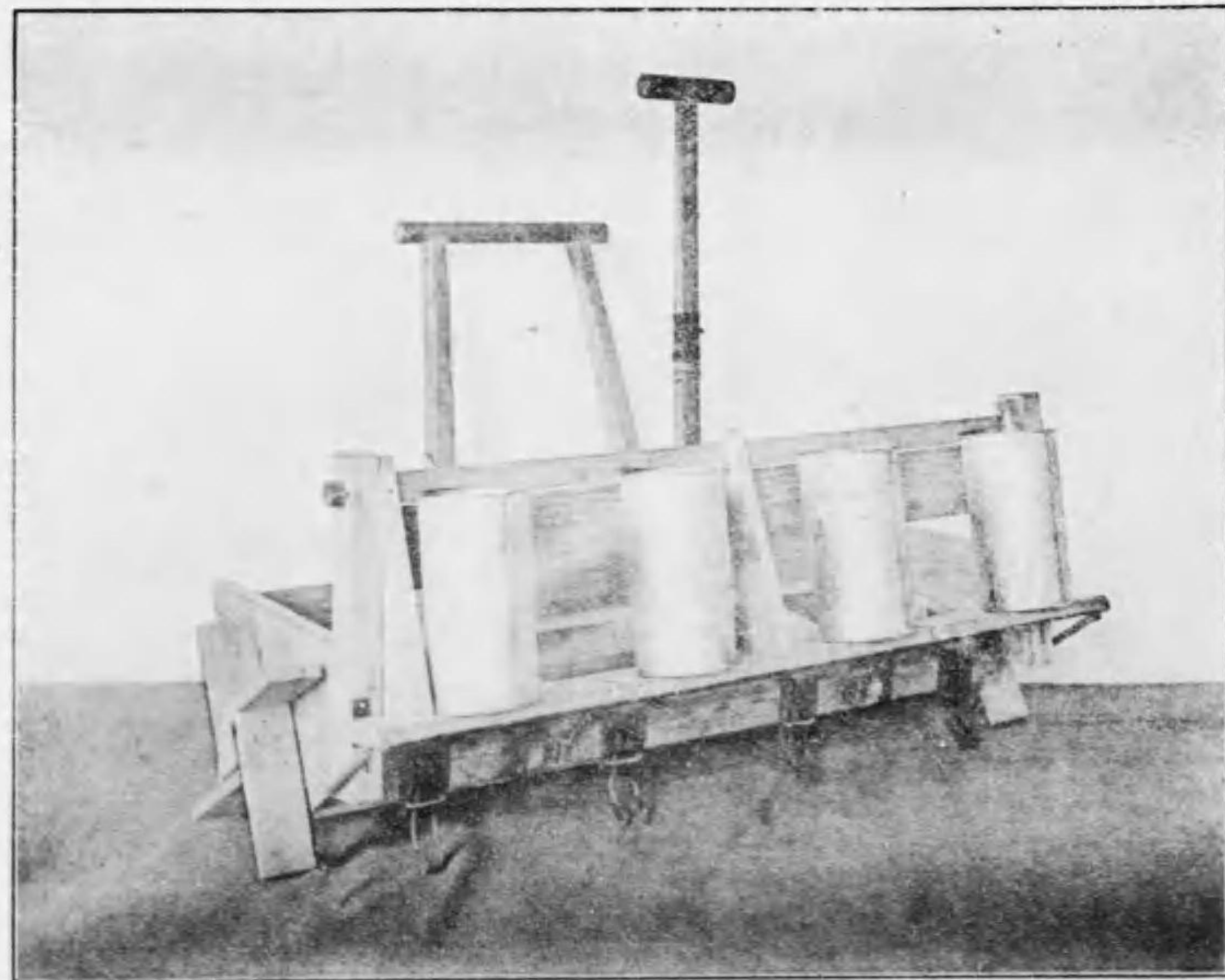
(類器秧插) 圖二十四百第真寫
