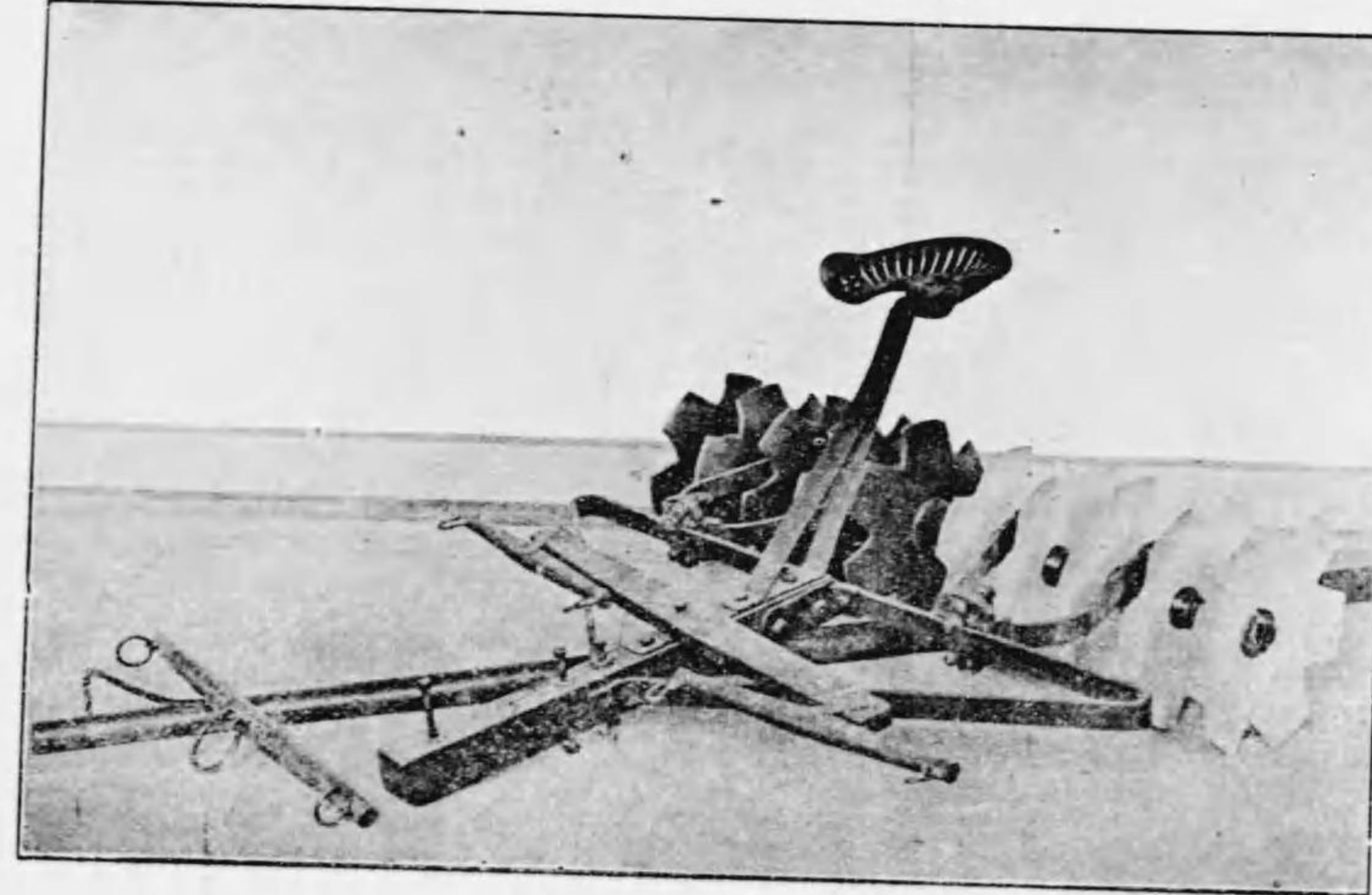
(類器土攪、器耙) 圖三十二百第真寫
