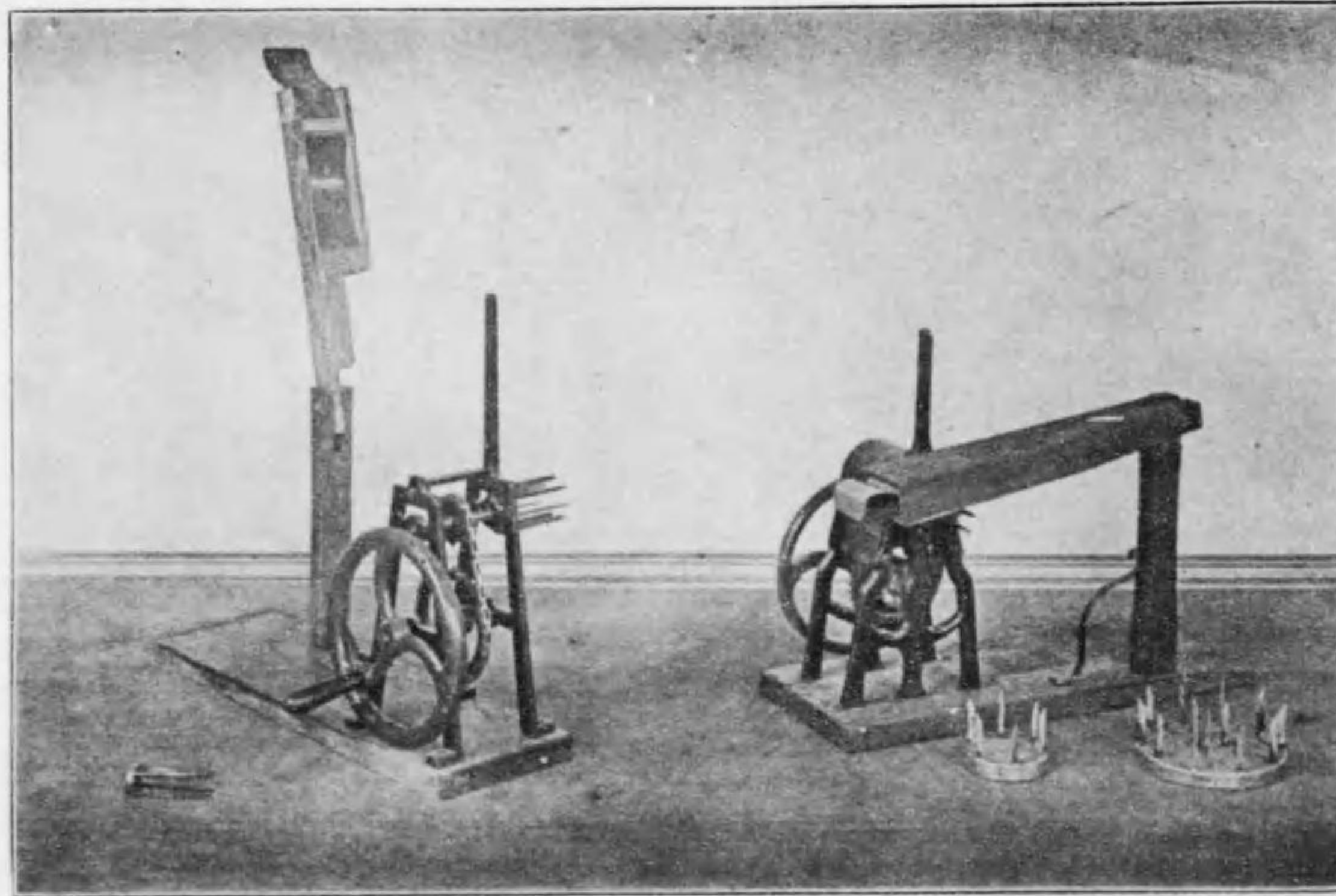
(類機切瓢干) 圖六十二百二第真寫
