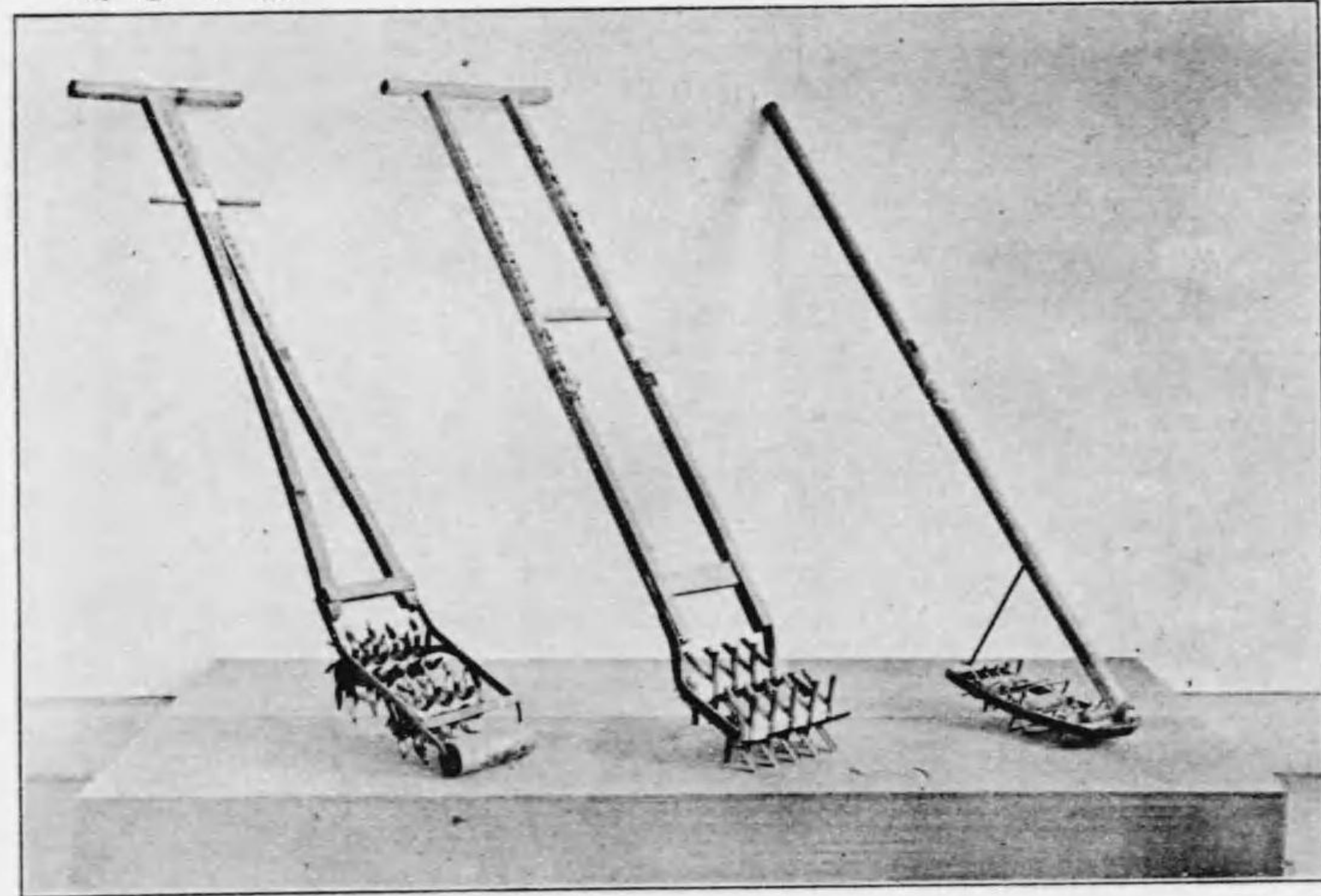
(類器草除) 圖七十五百第真寫
