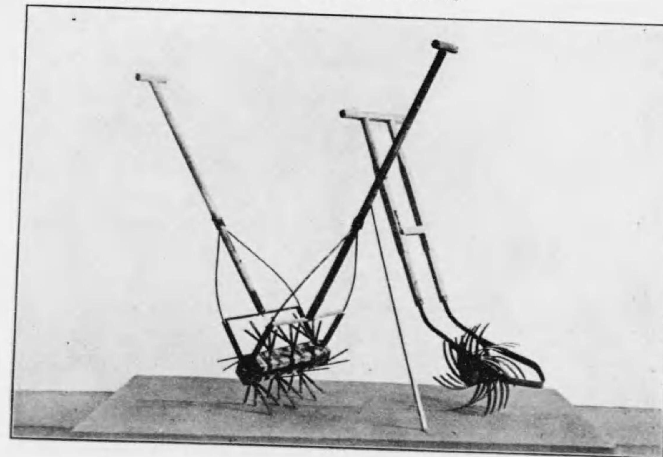
(類器草除) 圖六十五百第真寫
