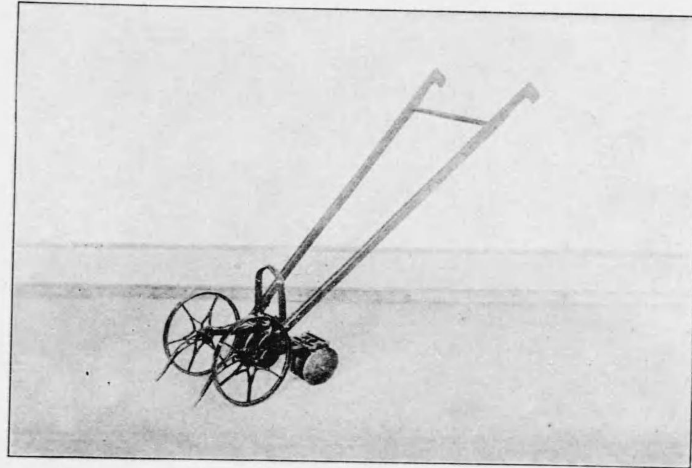
(類器耕中) 圖三十四百第真寫
