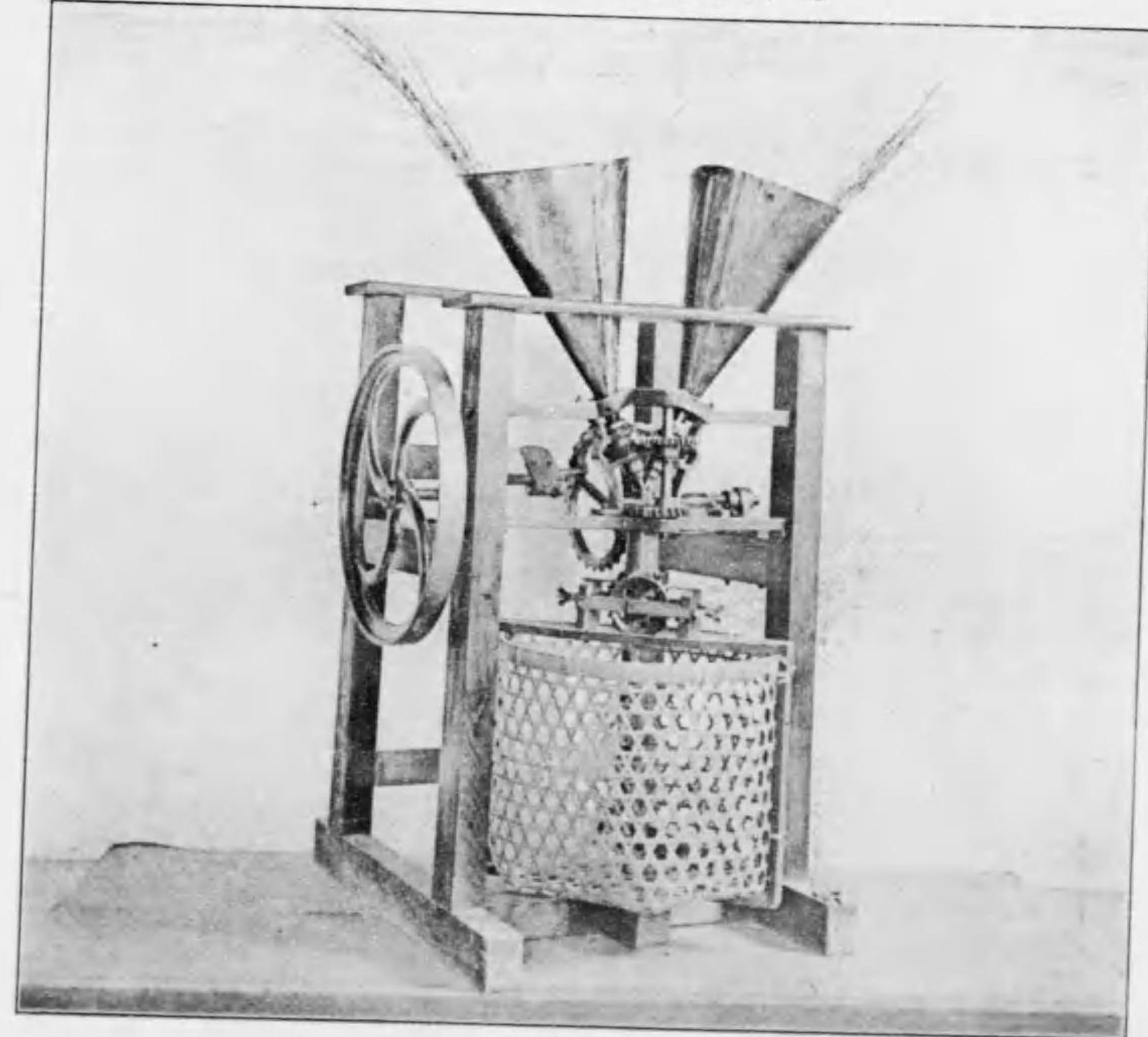
(類機繩製) 圖二十三百二第真寫
