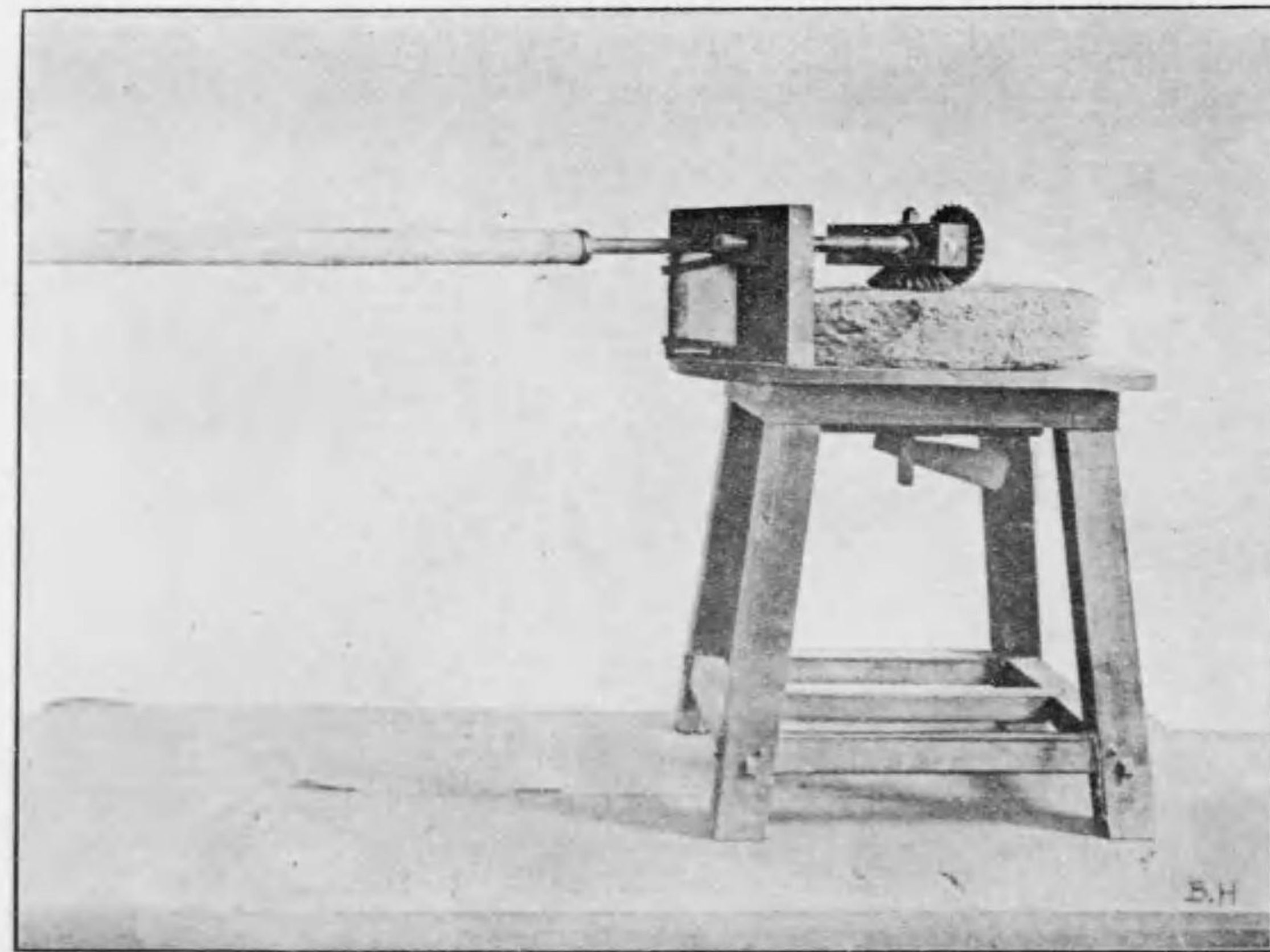
(類機碎粉料肥) 圖二十四百二第真寫
