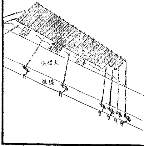
木龍八層縱木九層而梁
