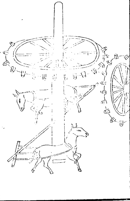
水輪車
