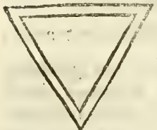
Isopleurus Rectus sub- ter constitutus.
