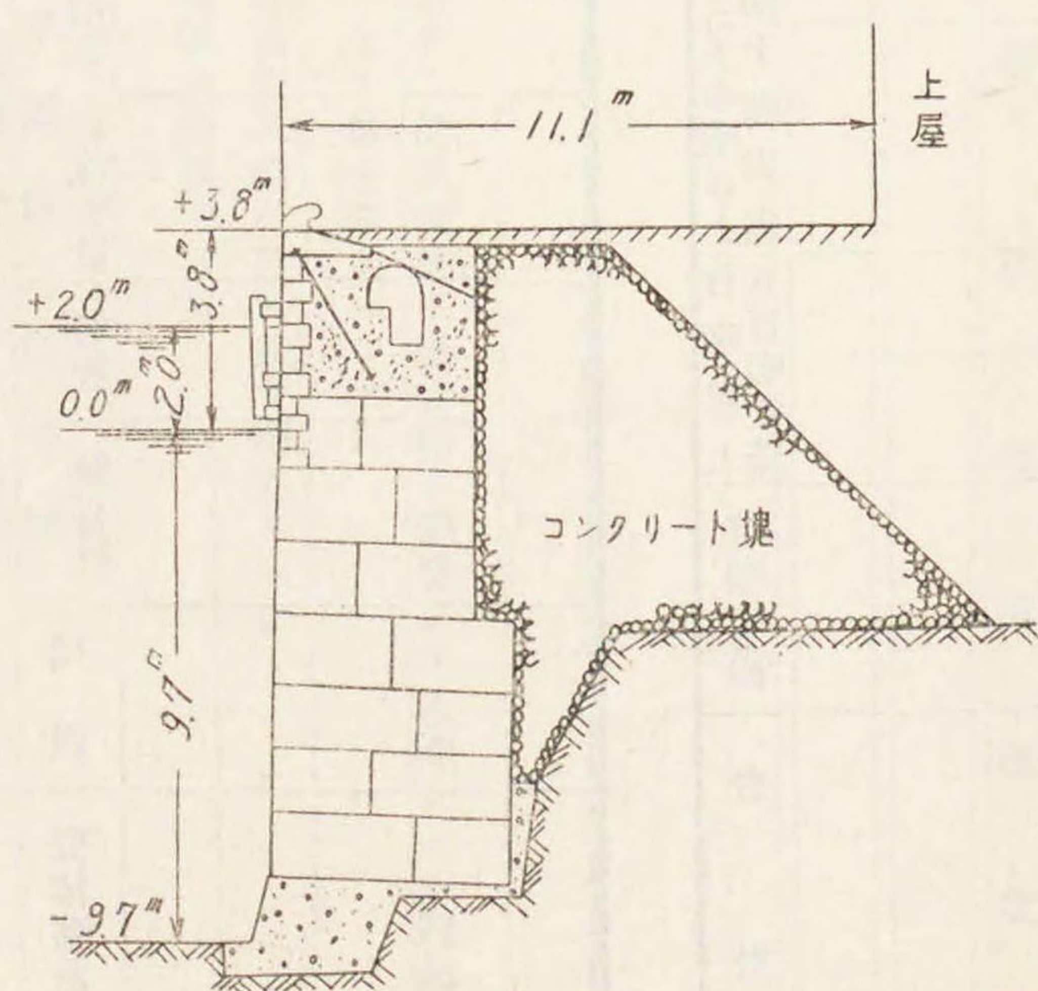
何繫船岸壁断面略圖
